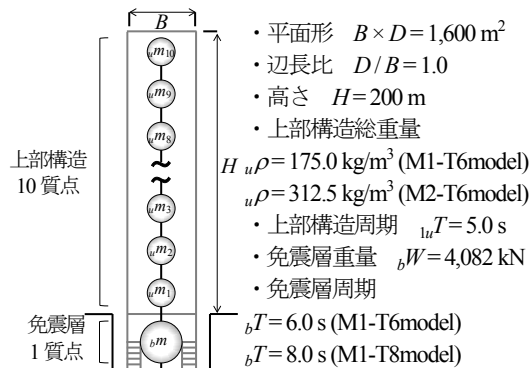
図1 弾塑性解析モデル概要
