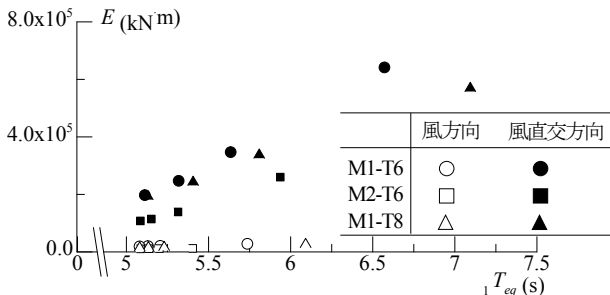
図3 {}_1 T_{eq} に基づく入力エネルギーの変化
