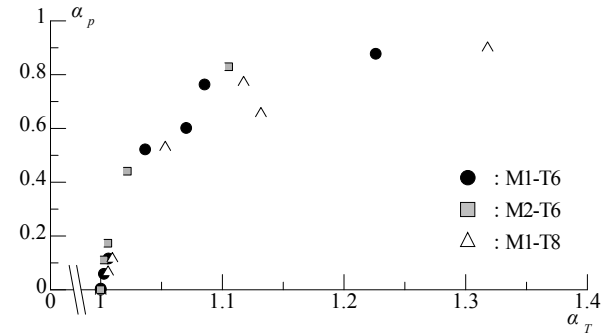
図4 \alpha_p と \alpha_T の関係
