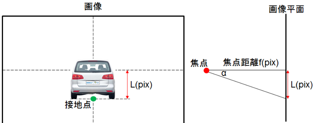
図 3.15： 接地点俯角 \alpha の計算
