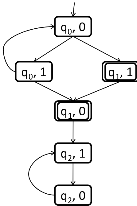
図 4.2: \mathcal{A}_{ex}, \sigma_{ex} の行程グラフ
