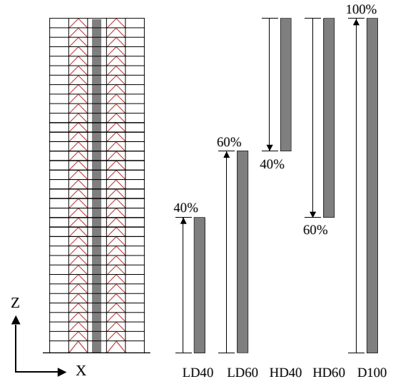
図1 粘性制振壁配置図（■：制振壁配置箇所）
