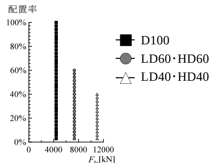
図2 粘性制振壁の粘性抵抗力
