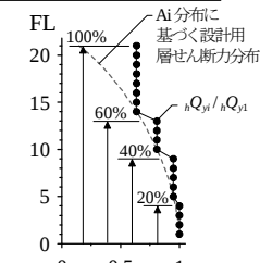
図2 降伏層せん断力の分布
