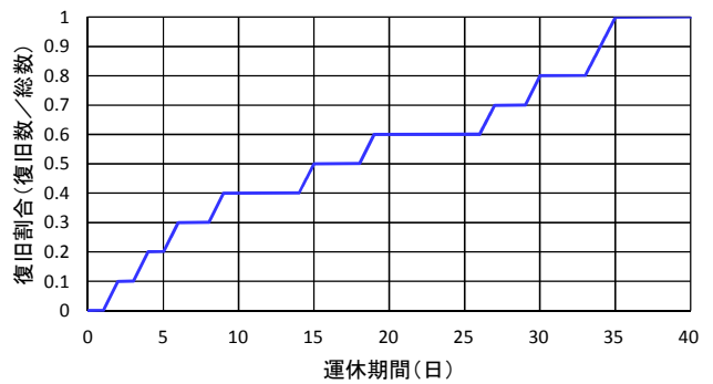
L8(2011東北以外・軽度被害・震度7)
