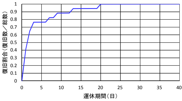
L1(2011東北・軽度被害・震度5強)
