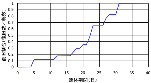
L3(2011東北・軽度被害・震度6強)
