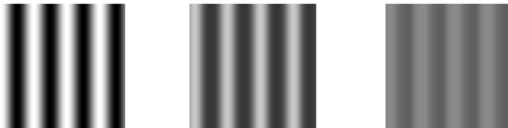
図 5.15 各収差の縦縞画像に対するコンボリユーション結果
