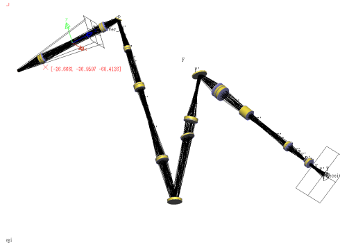
図 4.11 Code V による光学系の配置図
