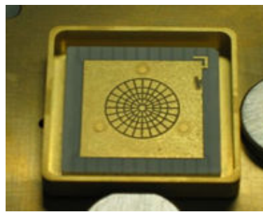
図 2.3 deformable Mirror (トプコン社提供)
