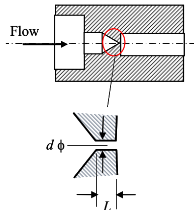
図 3.11 製作した短管ノズル
