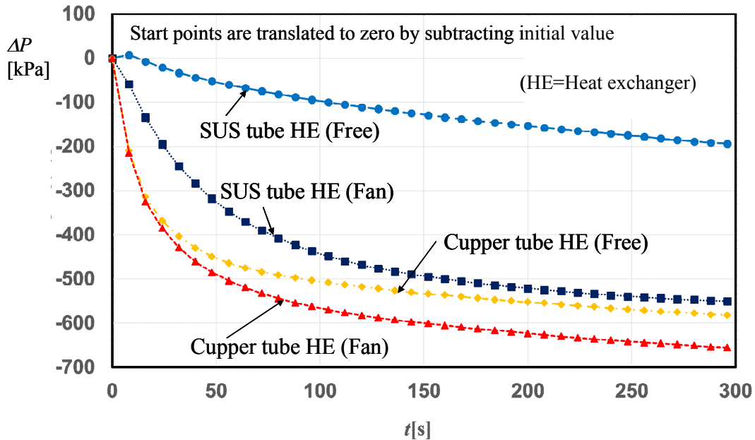
図 5.16 SUS 熱交換器と銅熱交換器, 漏れありのデータ
