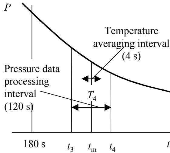
図 4.4 データ処理の時間間隔
