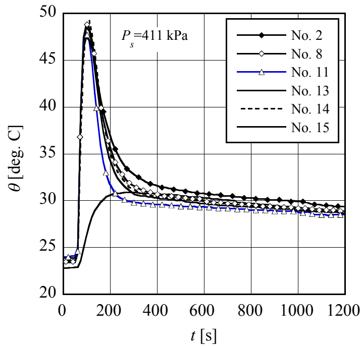
図 4.15 漏れがある場合の温度変化；チャージ圧力 411 kPa
