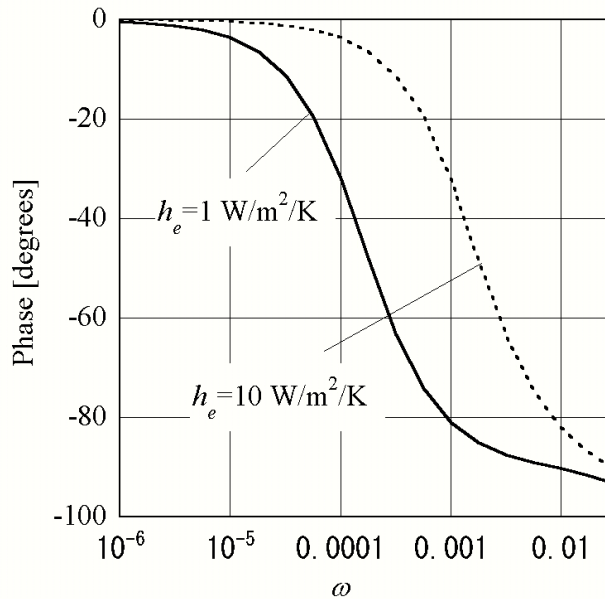
図 5.3 位相特性
