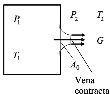
図1 オリフィスまたはノズル
