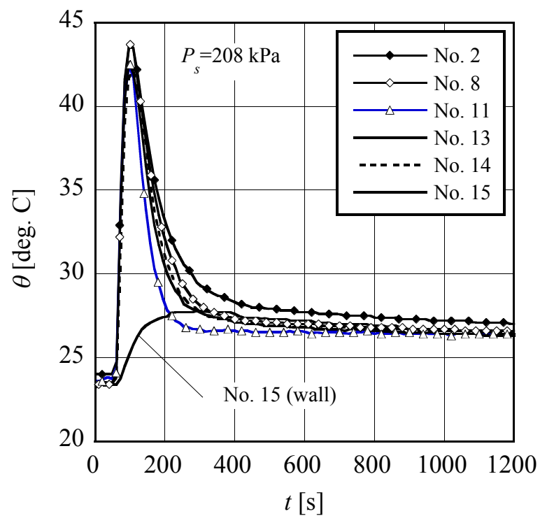
図 4.16 漏れがある場合の温度変化；チャージ圧力 208 kPa
