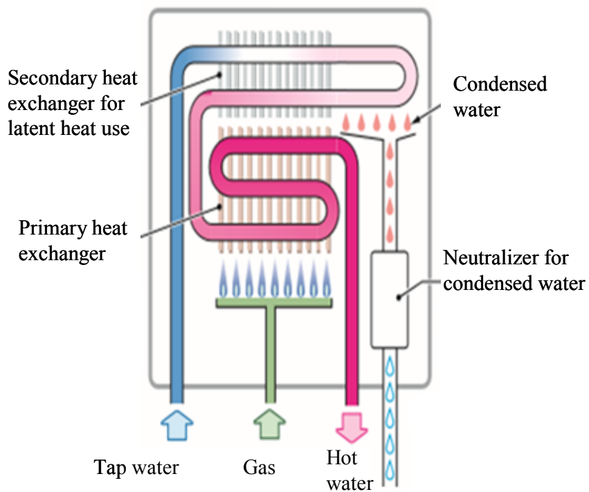
图 1.5 潜熱回収型高効率給湯機
