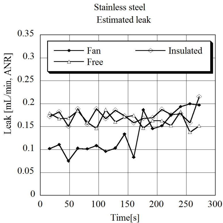
図 5.21 漏れ有りデータと漏れ無しデータの差の表示 (ステンレスコルゲート管熱交換器)
