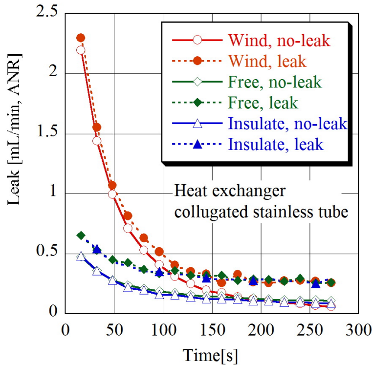
図 5.19 ステンレスコルゲート管熱交換器における見掛けの漏れ (平均曲線)
