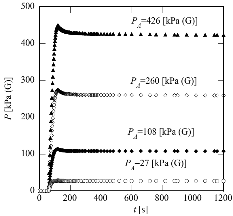
図 4.3 漏れの無い容器内の圧力変化
