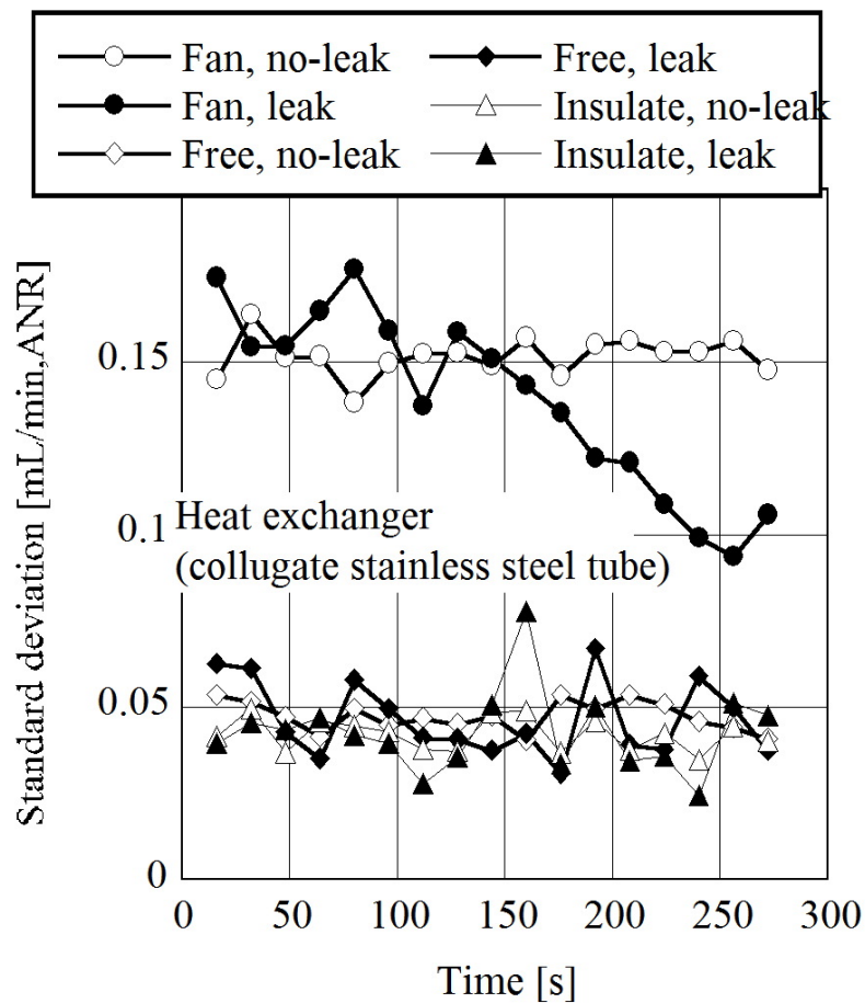
図 5.23 漏れ量推定値の標準偏差 (ステンレスコルゲート管熱交換器)
