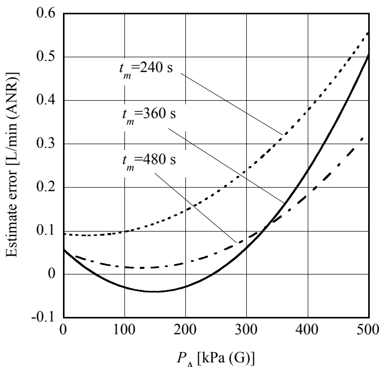
図 4.10 漏れの推定値の誤差
