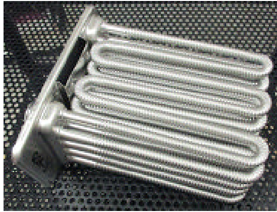
図 1.6 潜熱回収型高効率給湯機用ステンレス製二次熱交換器
