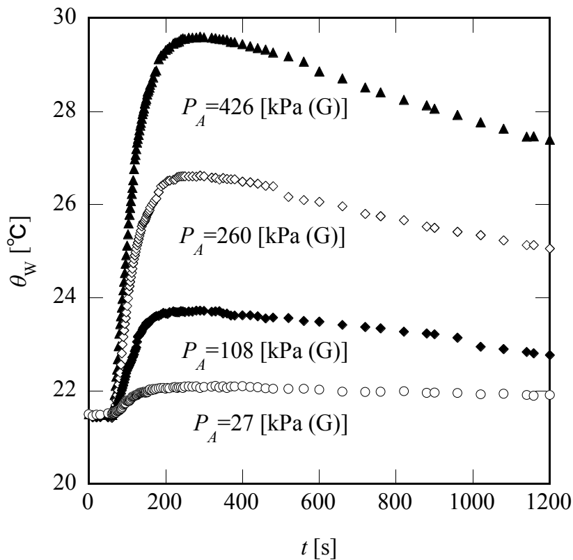
図 4.9 容器壁面温度
