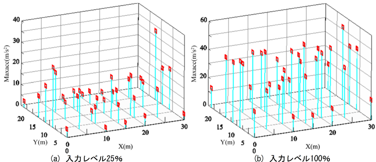
図7 屋根面加速度Z方向の最大値分布
