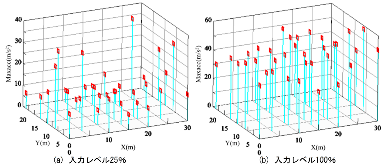
図6 屋根面加速度Y方向の最大値分布
