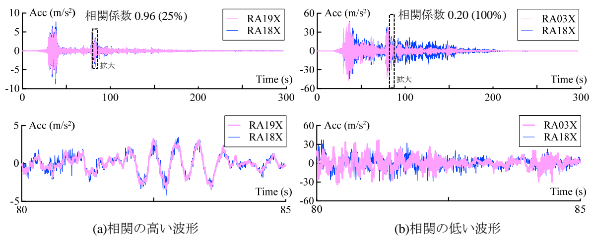
図11 X方向での加速度波形重ね合わせ
