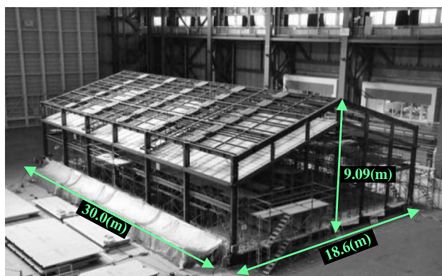
図1 実大体育館試験体 11)
