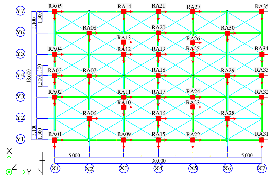
図2 屋根面加速度計測計画 12)
