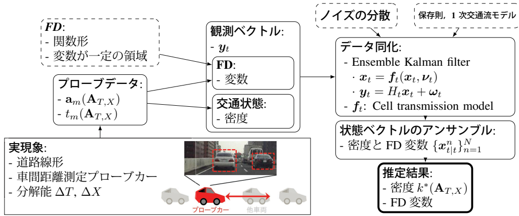
図-6: 交通状態・モデルパラメータ同時推定手法のコンセプト
