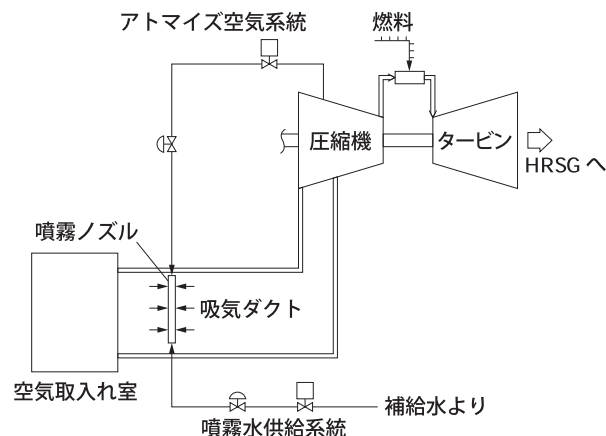
図4 吸気噴霧冷却システムの概要
