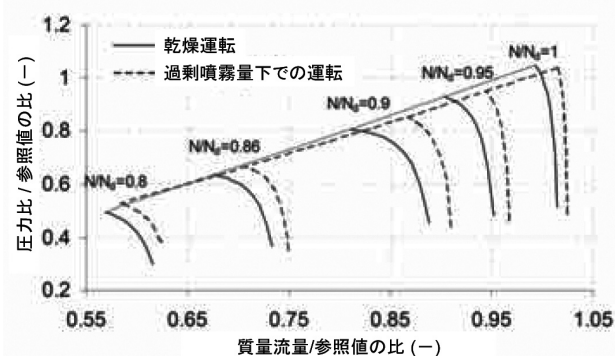
図12 過剰噴霧量1%での圧縮機運転マップ
