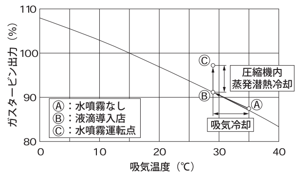
図1 ガスタービン出力の大気温度特性と吸気冷却による出力回復
