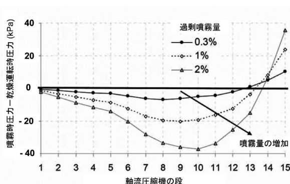
図16 乾燥運転との偏差で示した過剰噴霧時の圧縮器内圧力分布の変化
