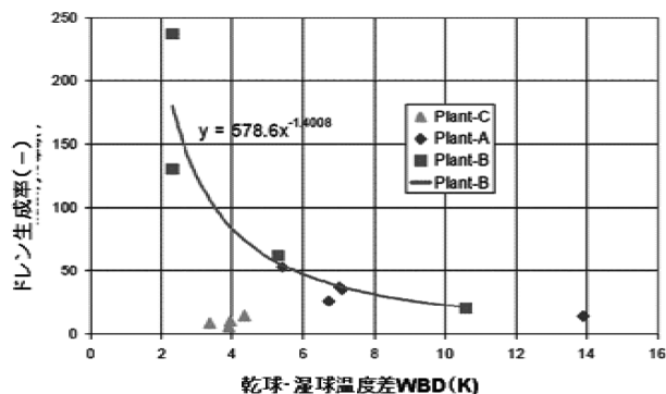
図11 ドレン生成の予測
