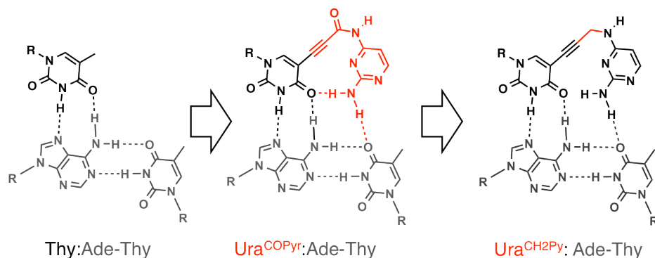
Figure 2. 第一章で設計した Ade-Thy 塩基対を認識する人工核酸塩基
