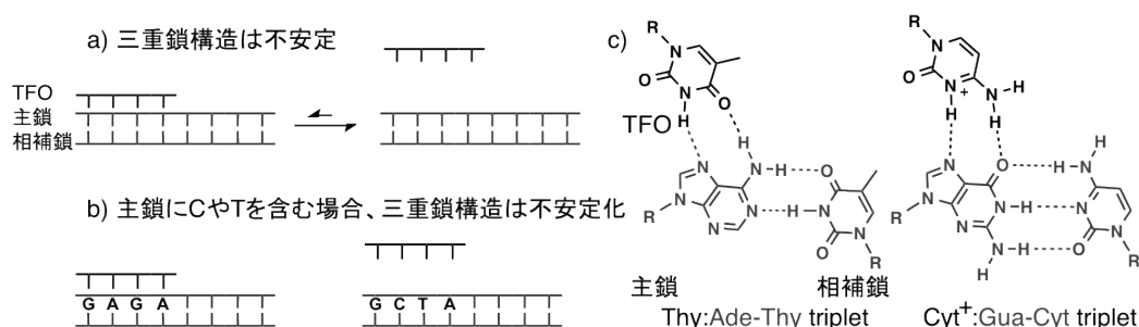
Figure 1. 天然型核酸で構成された核酸三重鎖の問題点
