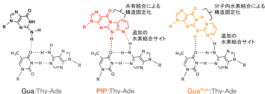
Figure 3. 第二章で設計した Thy-Ade 塩基対を認識し結合する人工核酸塩基
