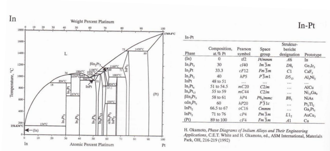
图 1-13. Pt-In 二元系状态图
