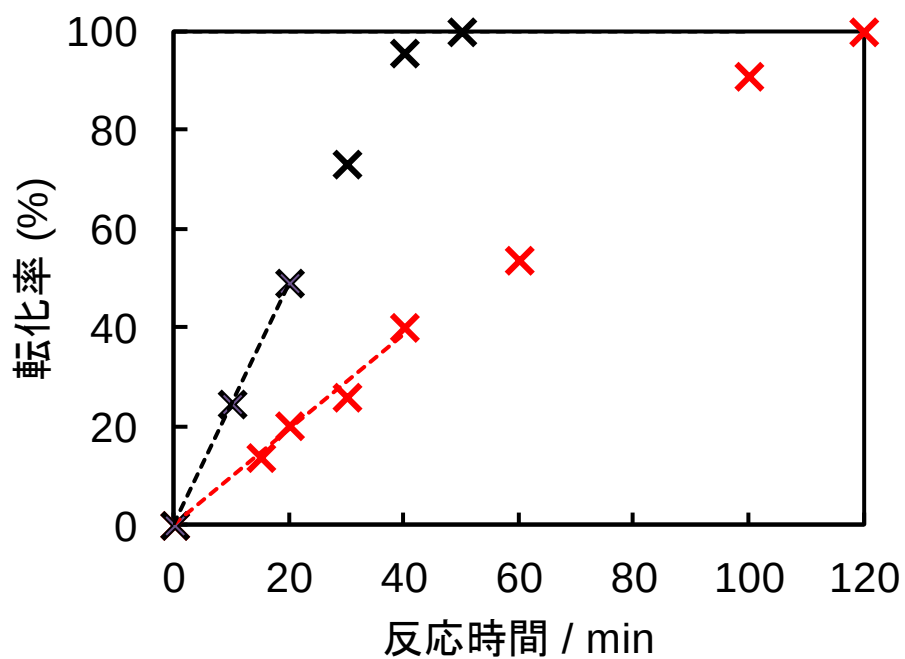
図 3-16. Pt/SiO 2 上での 4-CNBr 水素化における速度論的同位体効果 (× : H 2 雰囲気下、× : D 2 雰囲気下)
