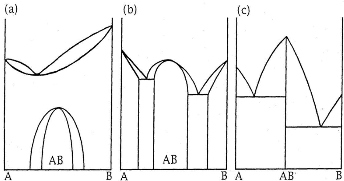
図 1-2. 平衡状態図による金属間化合物の分類
