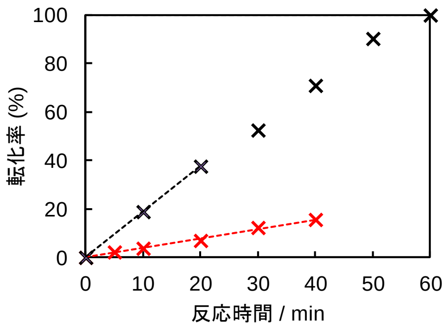
図 3-17. PtZn/SiO 2 上での 4-CNBr 水素化における速度論的同位体効果 (× : H 2 雰囲気下、× : D 2 雰囲気下)
