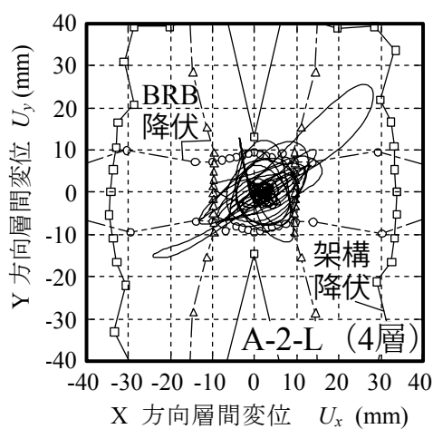
(ii) 層応答および降伏変位曲面
