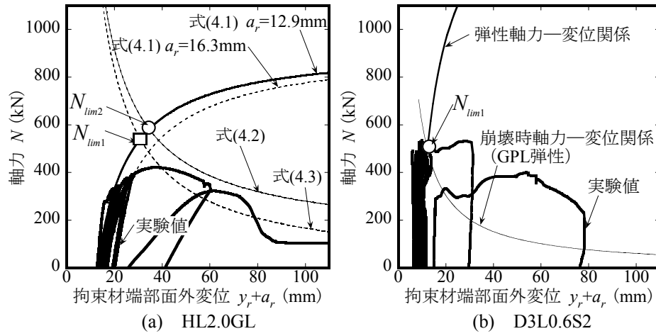
図 4.12 軸力—面外変位関係
