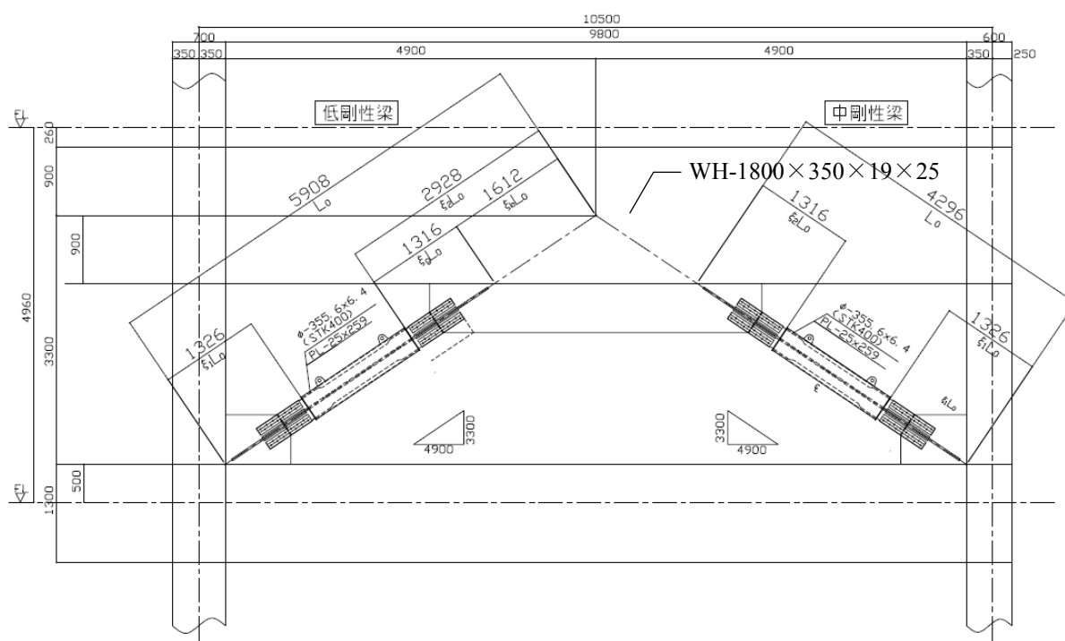
図 7.3 K 型配置された BRB の検討例 (取付く大梁成が非常に大きい場合)
