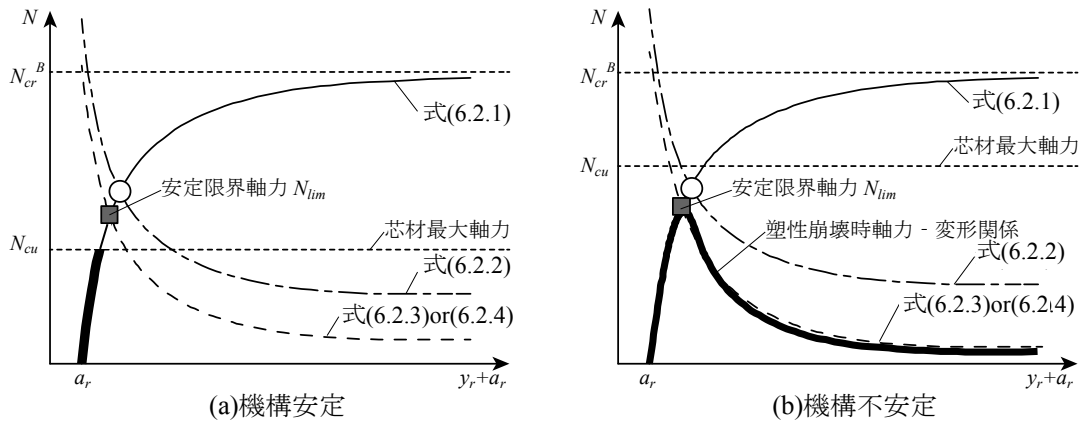
図 6.2.2 座屈拘束ブレースの機構安定条件
