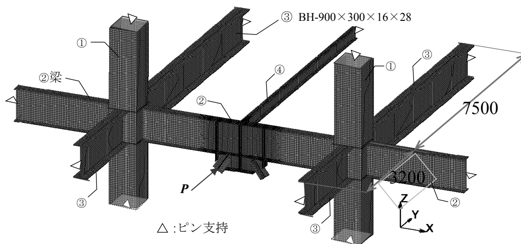
図 6.4.4 FEM 解析モデル図
