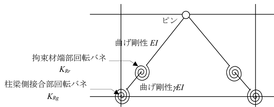
図 7.13 K 型配置用 BRB のモデル化
