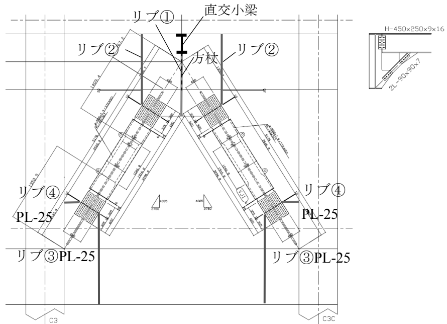
図 7.10 補強スチフナーの配置図
