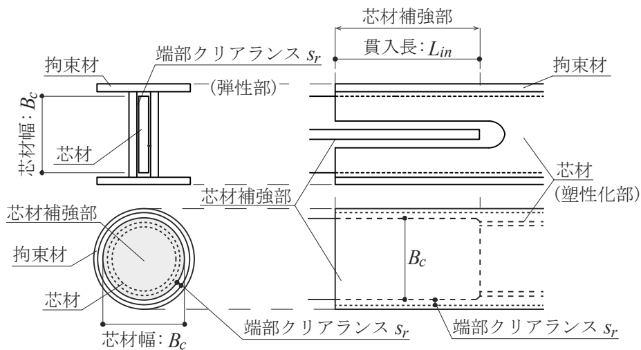
図 4.7 拘束材端部詳細図
