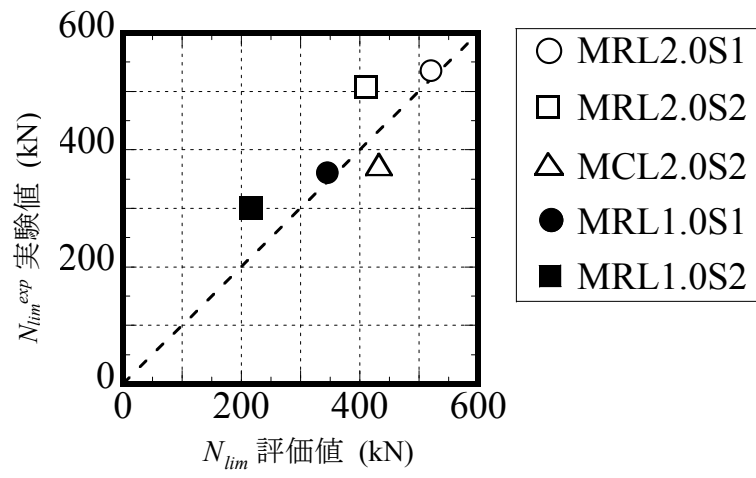
図 3.15 実験値と提案式の比較(崩壊時軸力)
