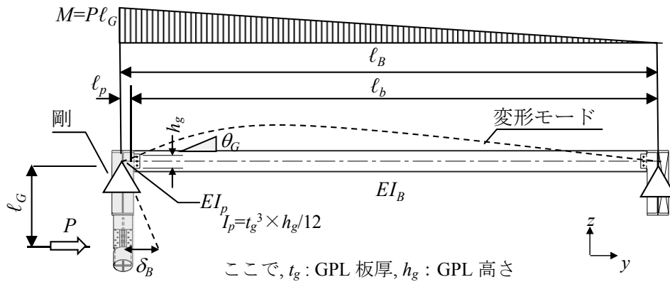
6.5.3 面外梁(ピン接合タイプ)の力学モデル
