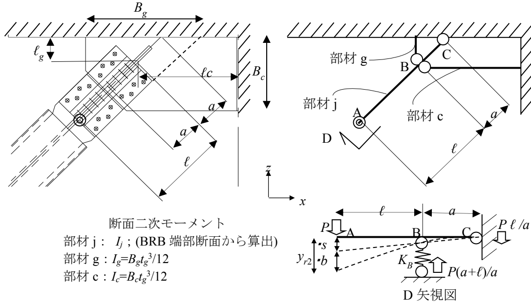
図 6.5.7 リブなし GPL の回転剛性算出用線材モデル
