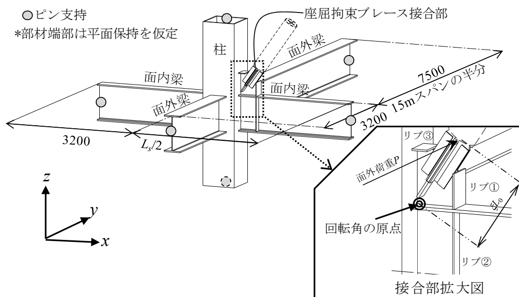
図 5.6 FEM 解析モデル
