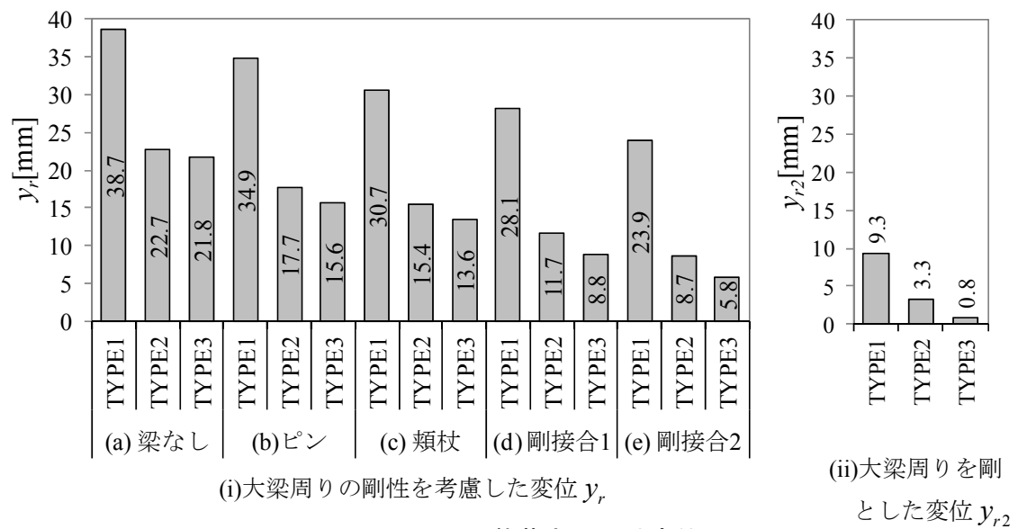
図 6.4.6 载荷点の面外変位
