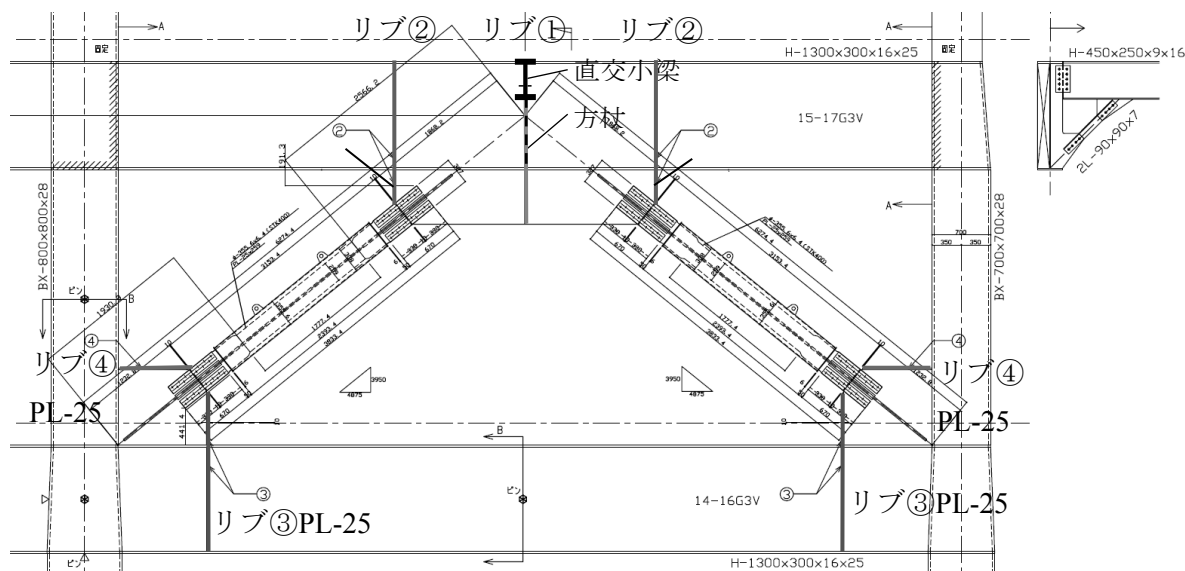
図 7.7 補強リブの配置図 (中剛性梁)
