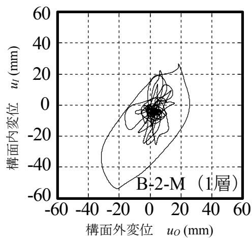
(iii) BRB 応答
