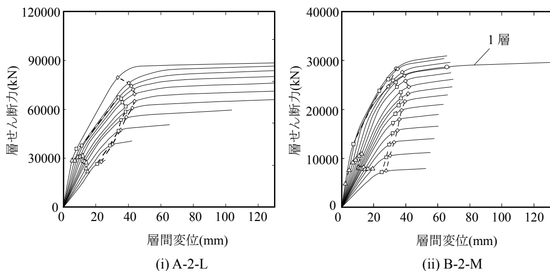
図 2.10 層せん断力-層間変位関係
