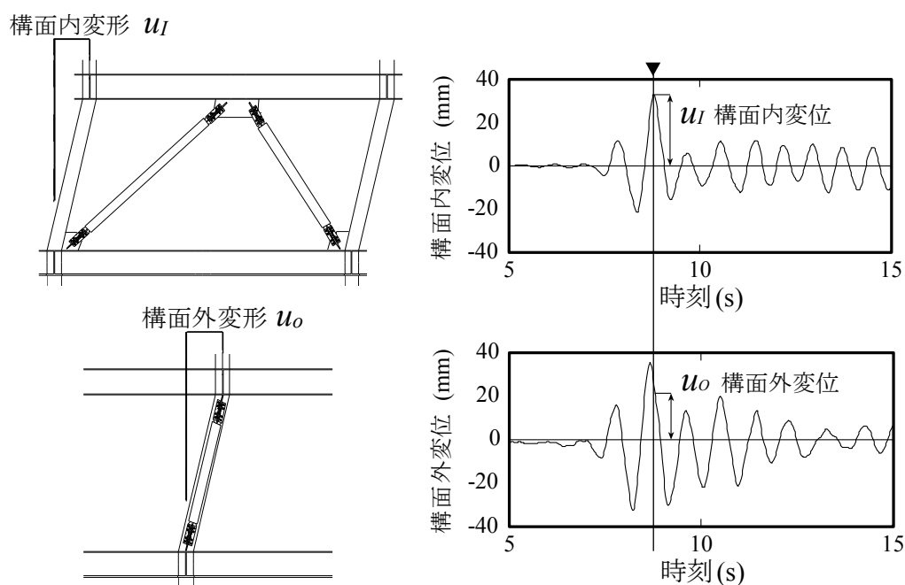
図 2.14 時刻歴応答解析結果抽出方法
