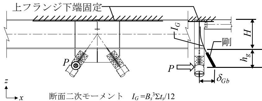
図 6.5.6 大梁ウェブの曲げ変形
