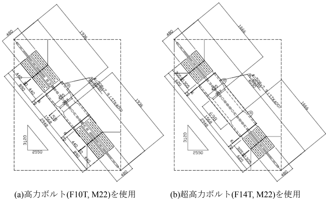
図 7.2 高容量 BRB の現場接合部検討例
