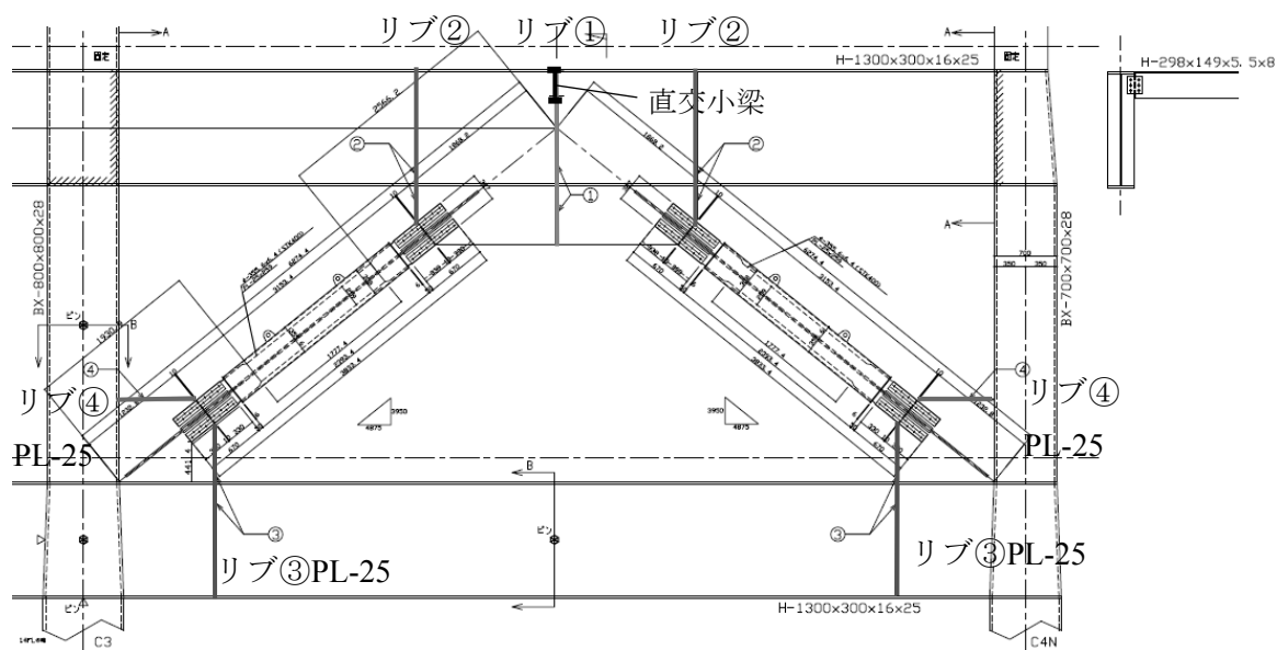
図 7.8 補強リブの配置図 (低剛性梁)
