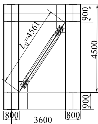
図 5.3 BRB の片流れ配置例
