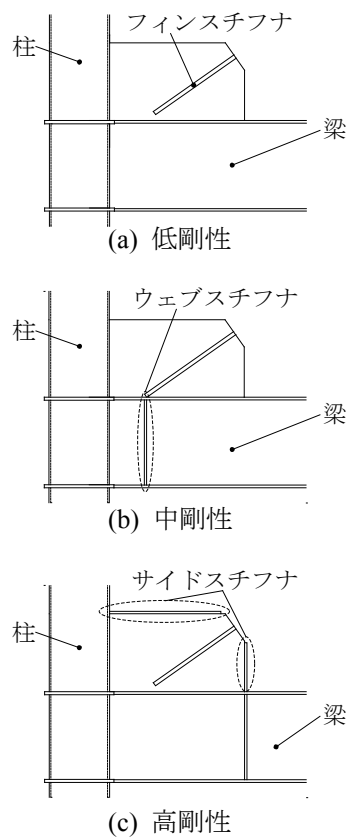
図 3.2 接合部ガセットプレート形式と構面外剛性
