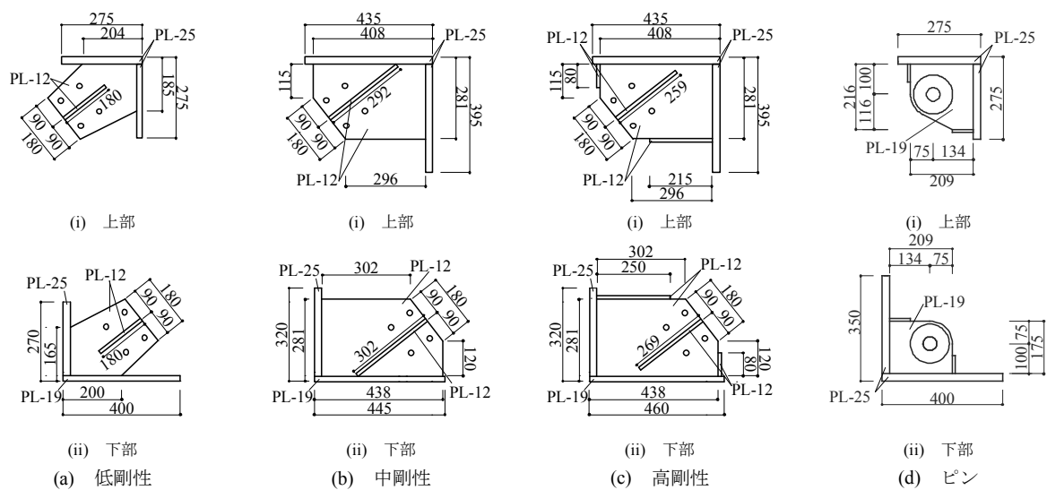
図 4.8 接合部ガセットプレート詳細図
