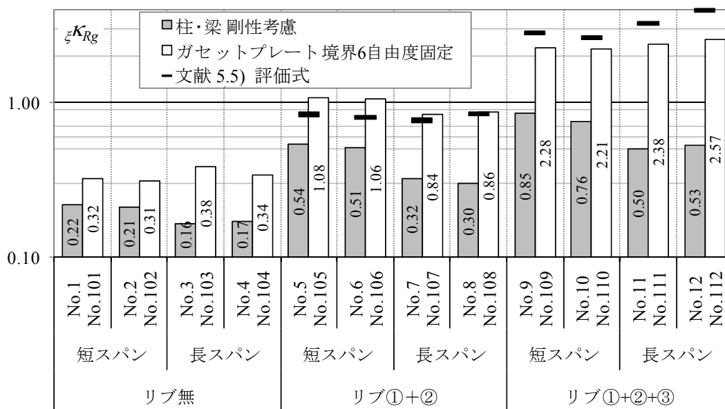
図 5.11 無次元化回転ばね剛性比 \xi \kappa_{Rg}
