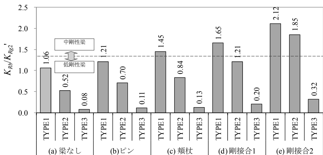
図 6.4.8 大梁の回転剛性と上部 GPL 回転ばねの比
