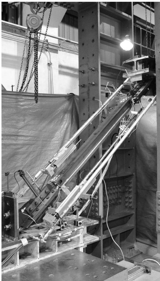
写真 4.1 HL シリーズ セットアップ
