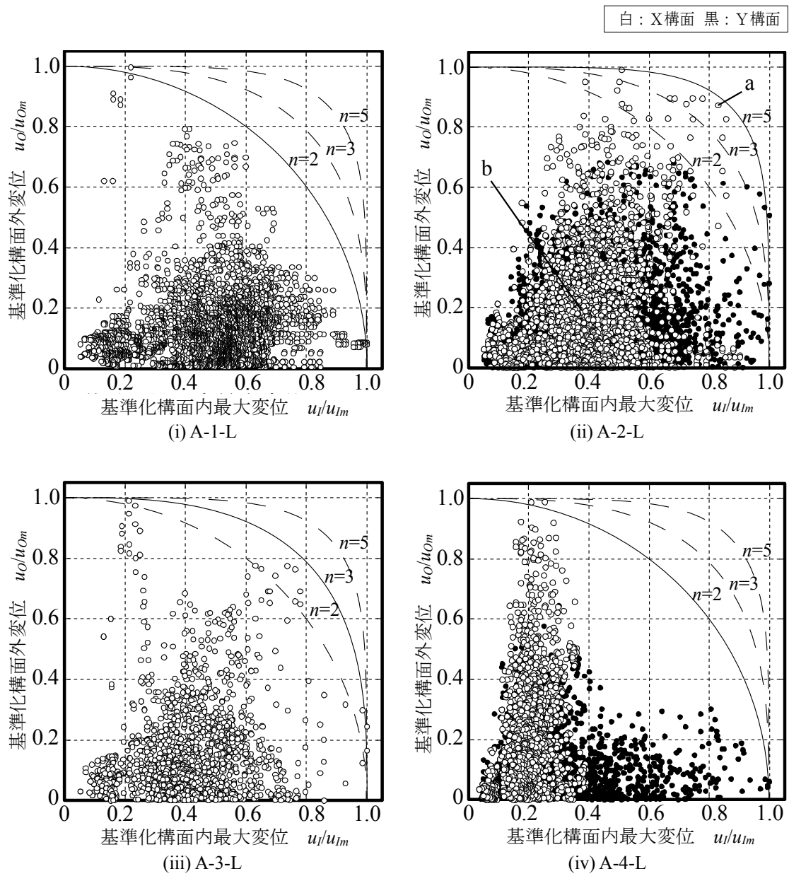
図 2.15 基準化構面内最大変位と同時刻における基準化構面外変位
