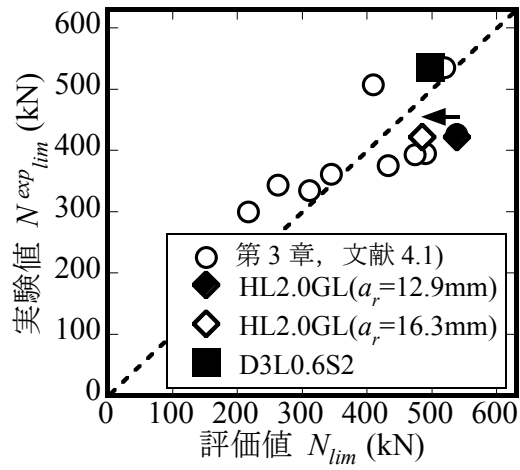
図 4.13 安定限界軸力評価精度
