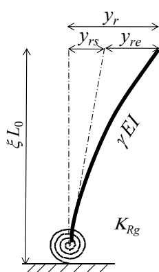
図 5.10 y 方向変位の設定
