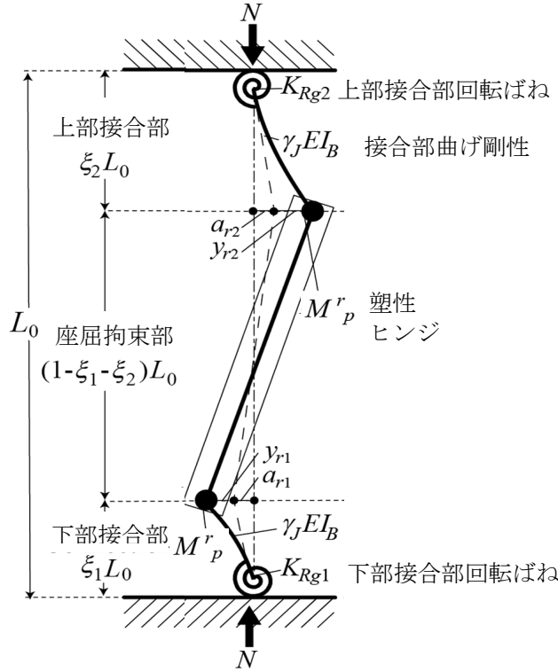
図 6.2.7 崩壊メカニズム（接合部：回転ばね，逆対称モード）
