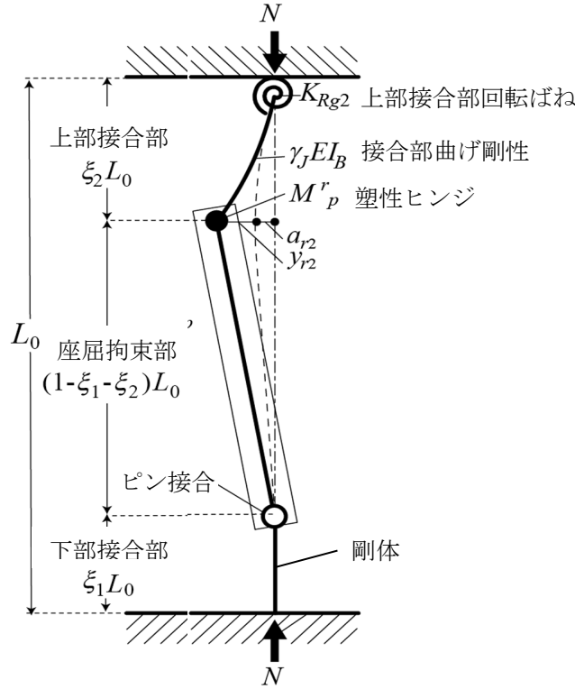
図 6.2.8 崩壊メカニズム（接合部：回転ばね，逆対称モード）
