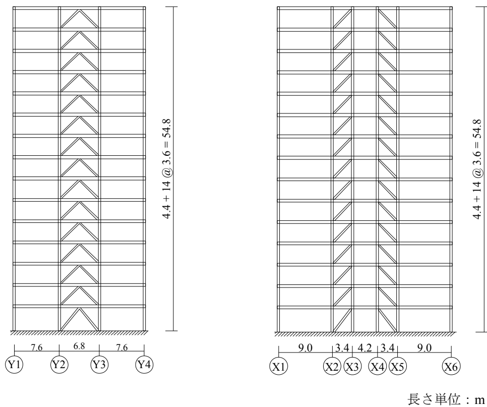
図 2.7 軸組図（センターコア形式）
