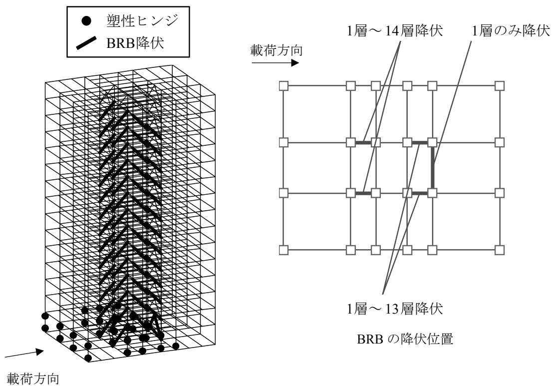
図 2.11 機構図 (B-2-M)
