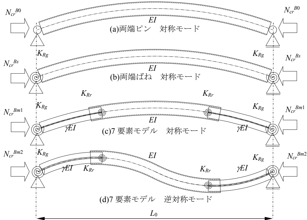
図 5.12 座屈検討モデルと座屈モード
