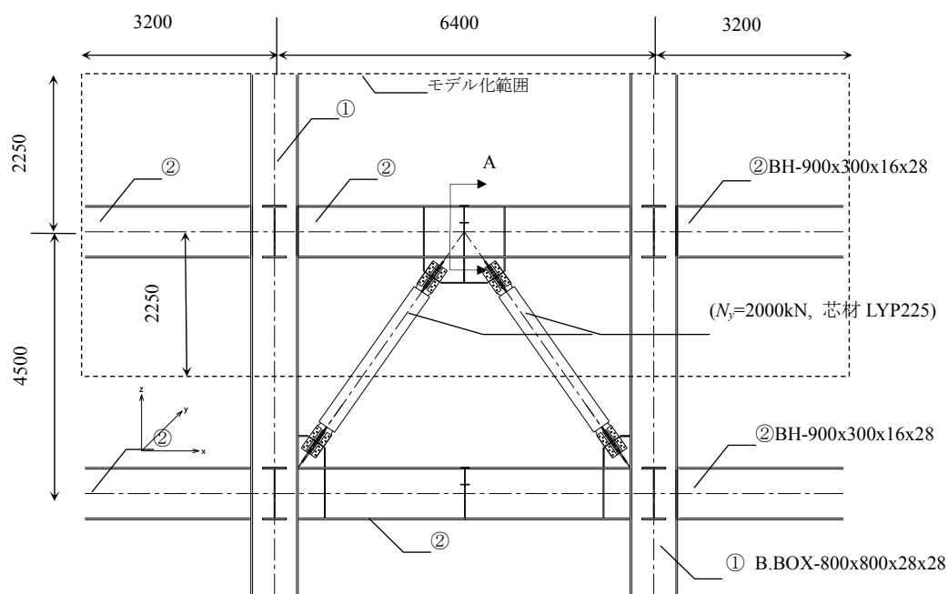
図 6.4.1 K 型配置 BRB 接合部の検討範囲
