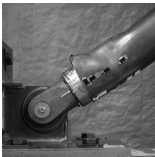
(b) 載荷後拘束材端部拡大
