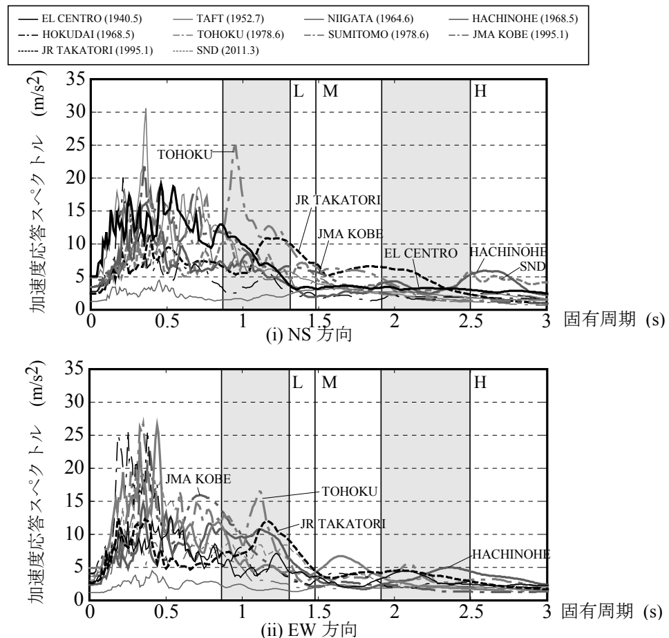
図 2.13 加速度応答スペクトル
