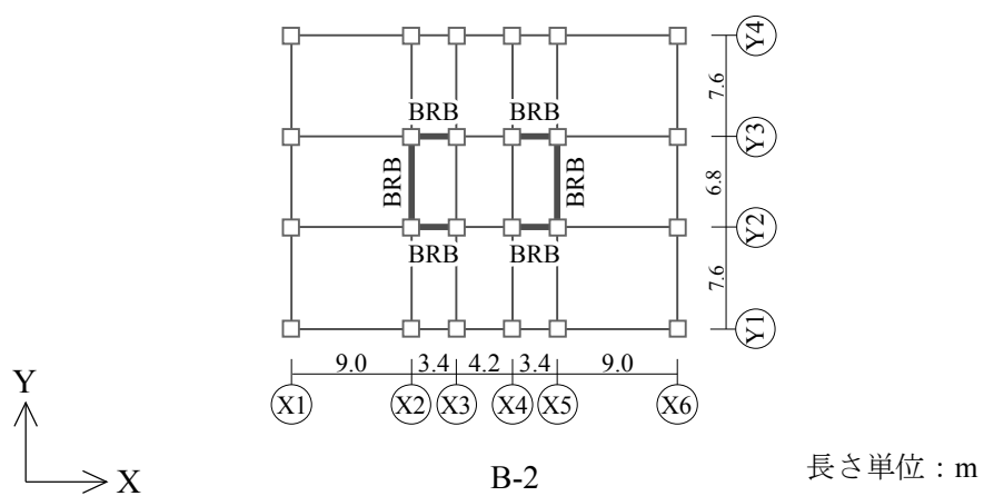
図 2.6 BRB 配置伏図（センターコア形式）
