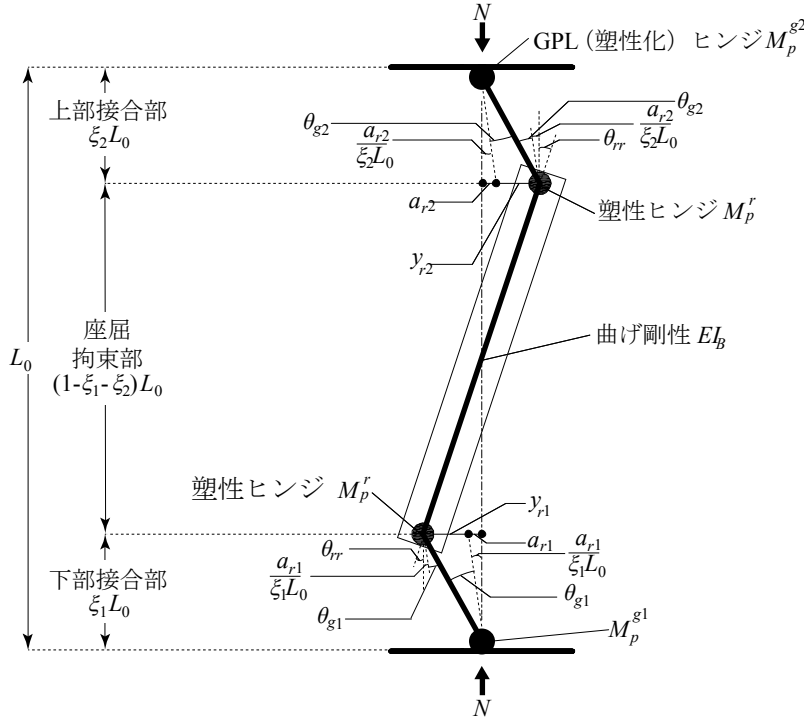
図 6.2.9 ガセットプレート塑性化後崩壊メカニズム（逆対称モード）
