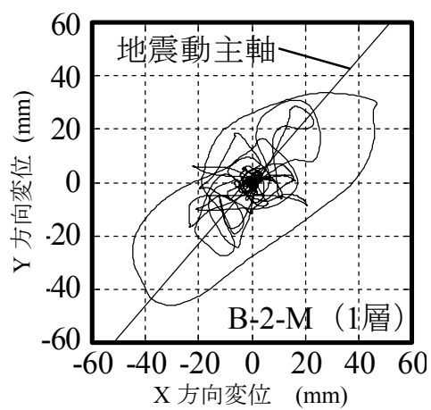
(i) 地震動変位オービット
