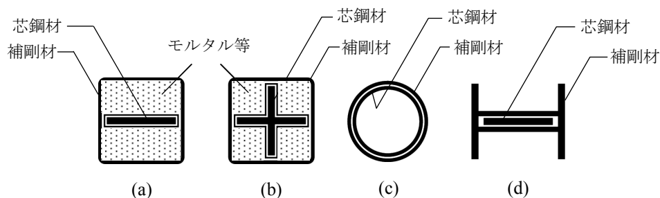
図 4.1 座屈拘束ブレースの座屈補剛形式例
