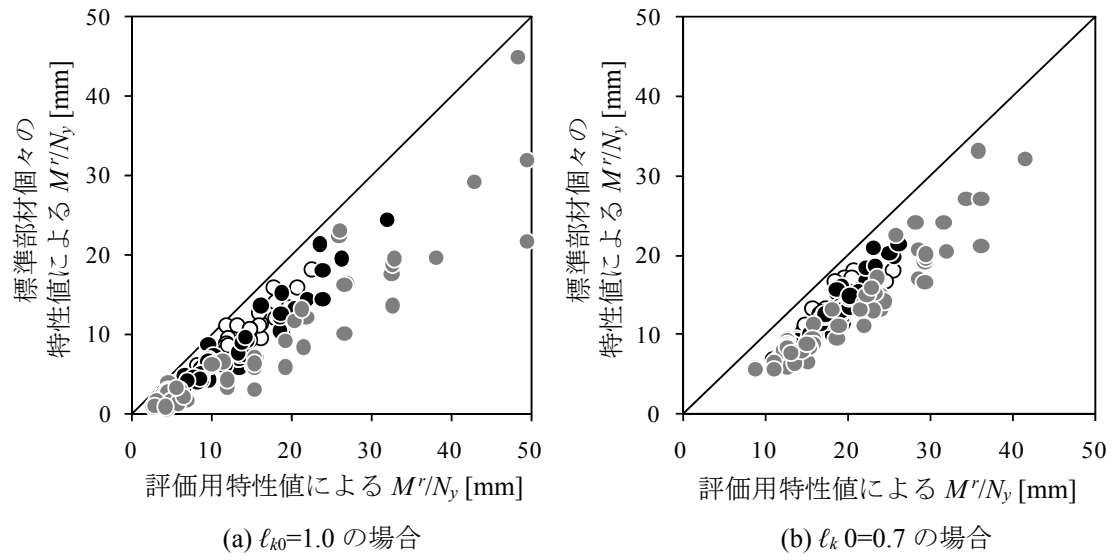
図 5.24 本検討範囲における M^r / N_y の精度
