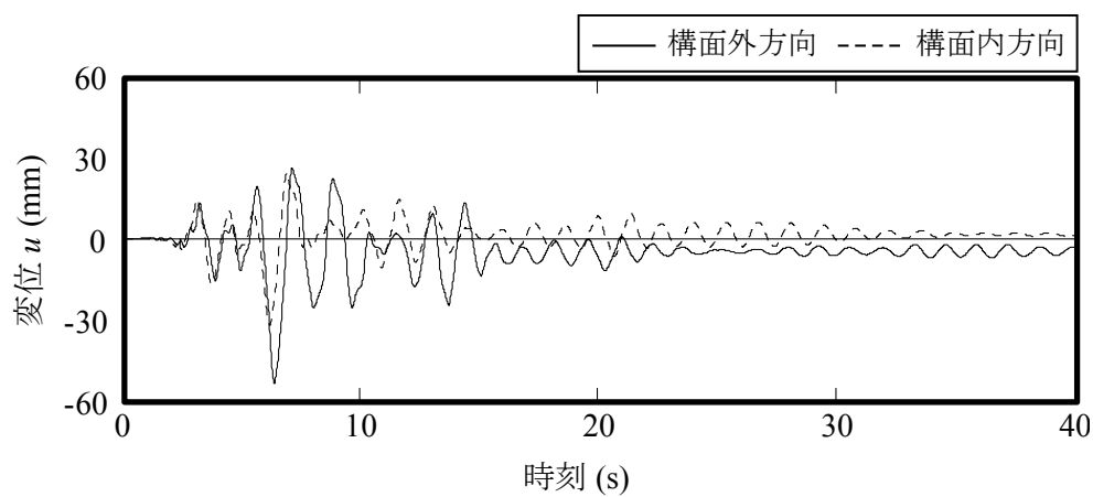
図 2.20 時刻歴応答変位波形 (B-2-M JR TAKATORI 波 90° 入力 1 層)
