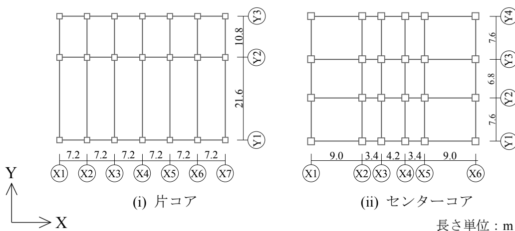
図 2.1 平面形状
