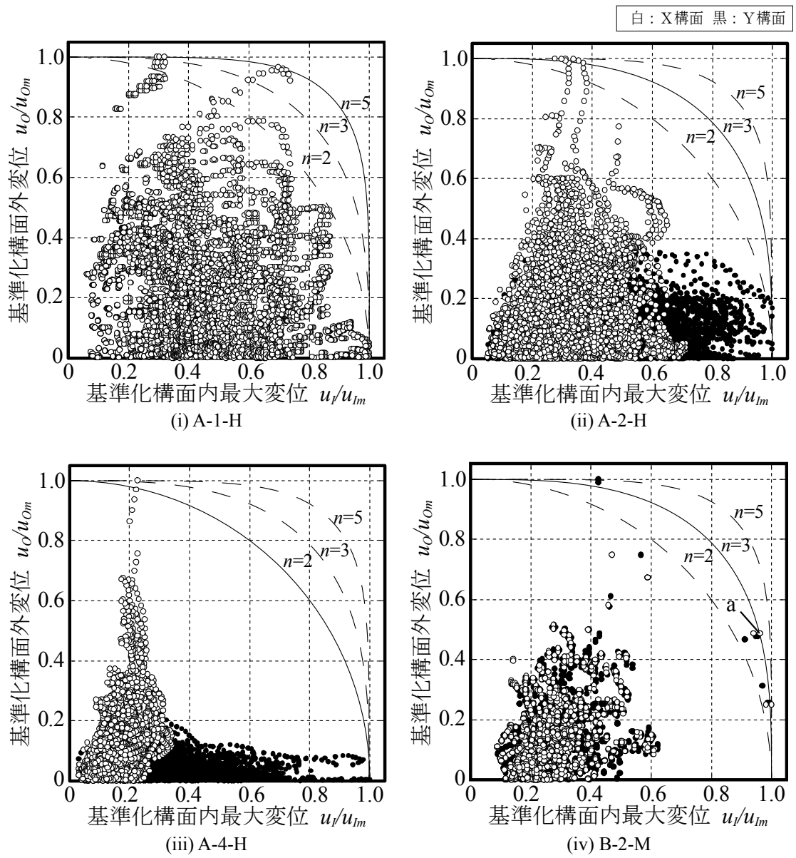
図 2.18 基準化構面内最大変位と同時刻における基準化構面外変位
