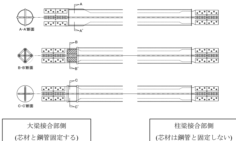
図 7.12 K型配置用 BRB
