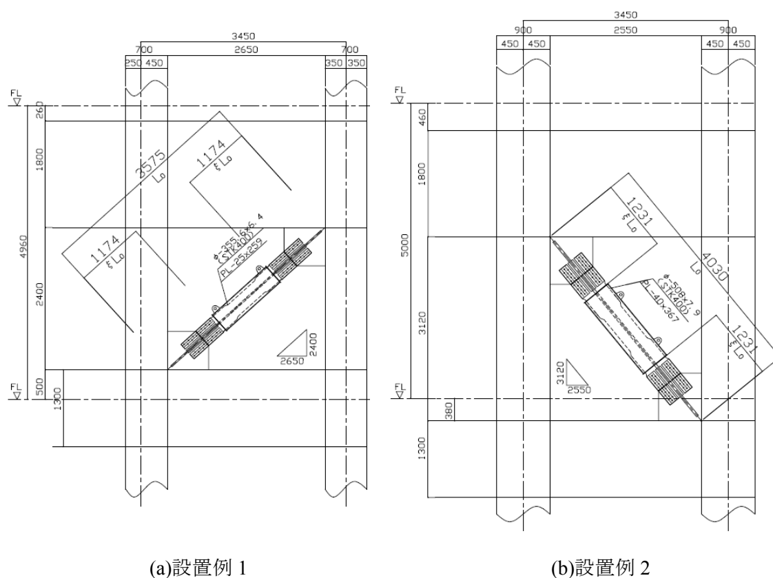
図 7.1 片流れ配置された BRB の検討例
