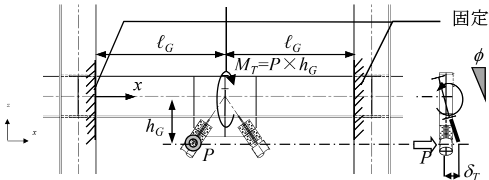
図 6.5.2 大梁の回転剛性の力学モデル
