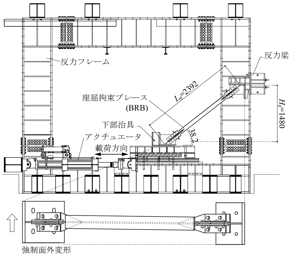
図 4.4 試験体セットアップ図
