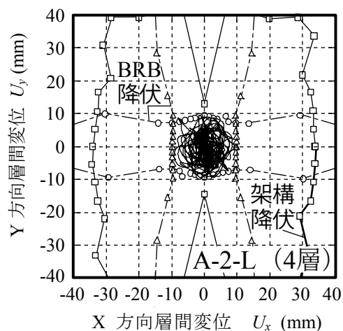
(ii) 層応答および降伏変位曲面
