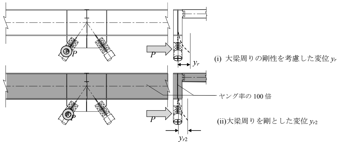
図 6.4.5 大梁周りの境界条件と面外変位記号
