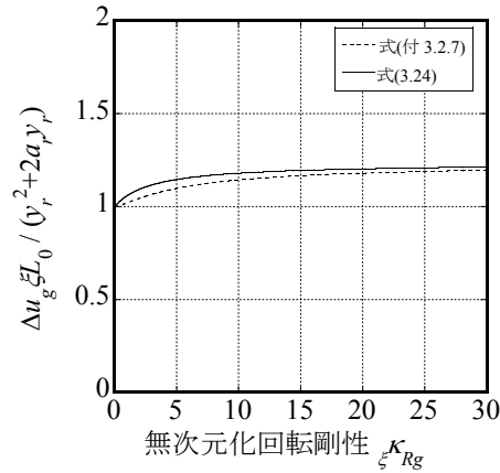
付図 3.2 式(付 3.2.7)と式(3.24)の比較
