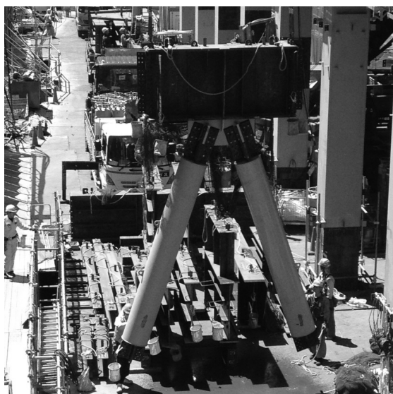
写真 1.1 超高層建物での高容量 BRB 採用例
