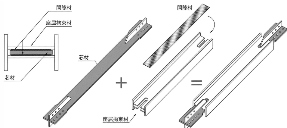
図 4.3 ダブルウェブ型 H 形鋼を拘束材に用いた BRB の機構
