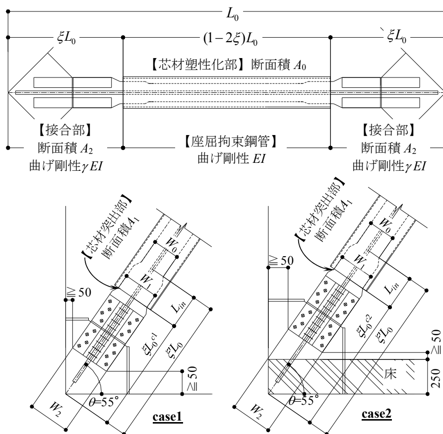
図 5.1 座屈拘束ブレース寸法および剛性と納まり例
