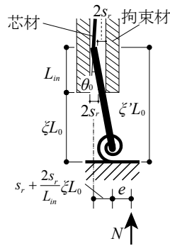
図 3.4 初期不整の設定
