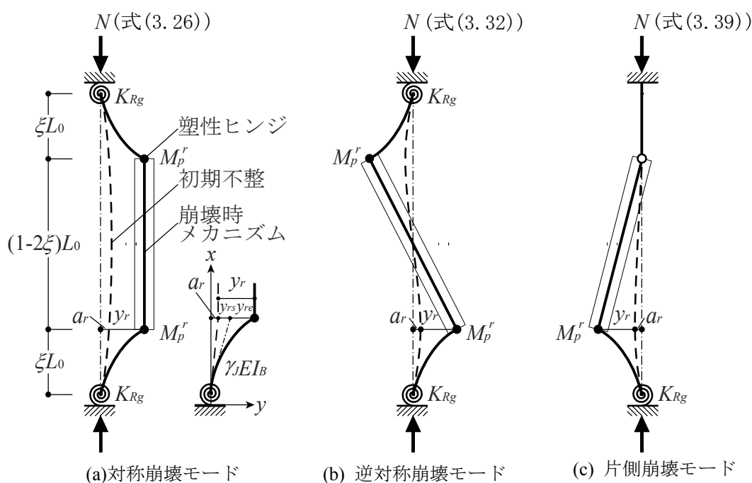
図 3.6 接合部を考慮した座屈拘束ブレースの崩壊メカニズム
