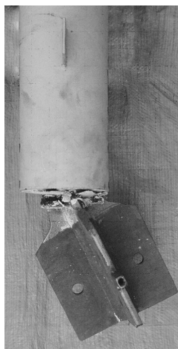
写真 3.3 載荷後 (MCL2.0S2)
