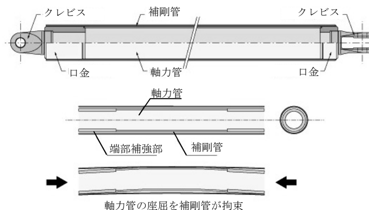
図 4.2 二重鋼管型 BRB の機構
