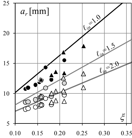
図 5.15 初期不整値 a_r と接合部長さ比 \xi
