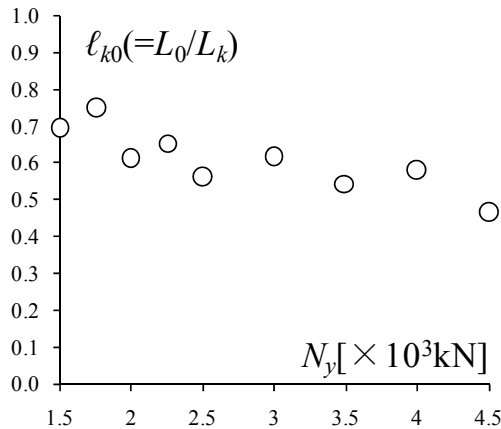
図 5.4 座屈長さ比 \ell_{k0} の分布
