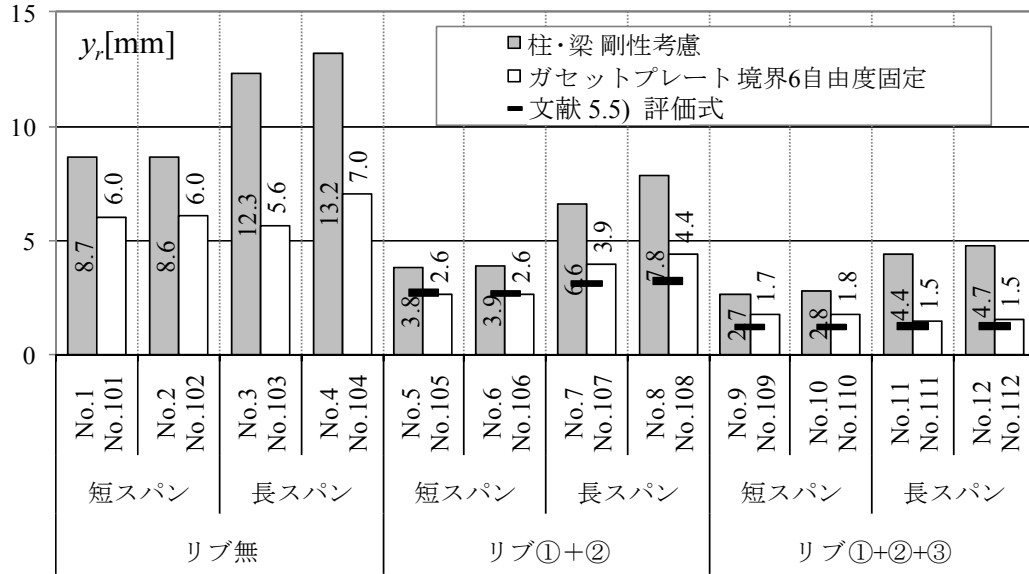
図 5.9 y 方向変位 y_r
