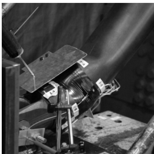
(a) 拘束材端部不安定時状況
