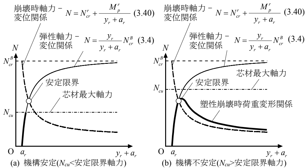
図 3.5 座屈拘束ブレースの機構安定条件
