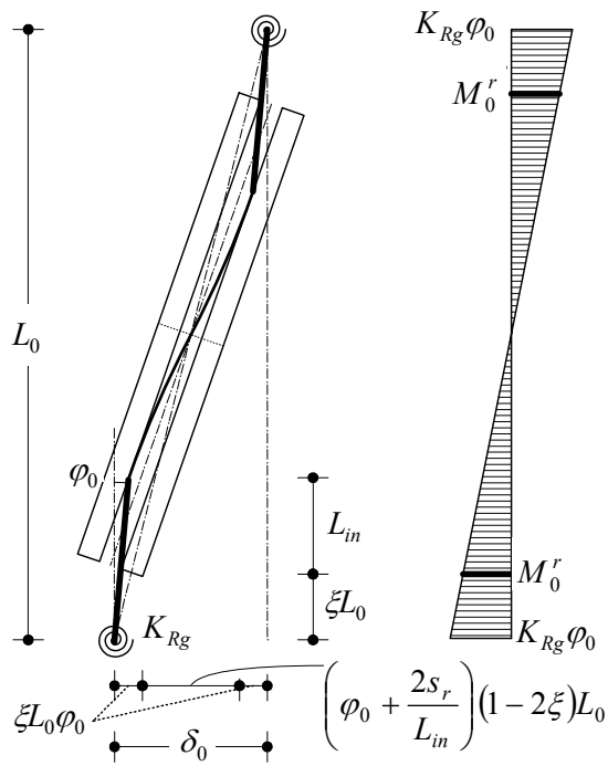
図 3.7 強制面外変形下の曲げモーメント分布仮定
