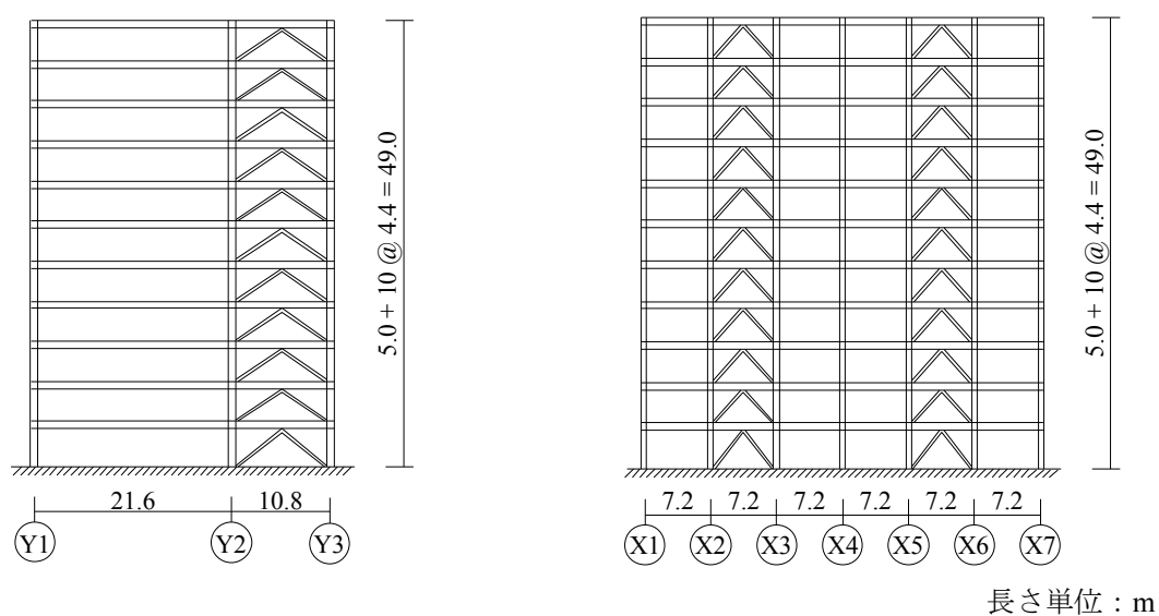
図 2.5 軸組図（片コア形式）
