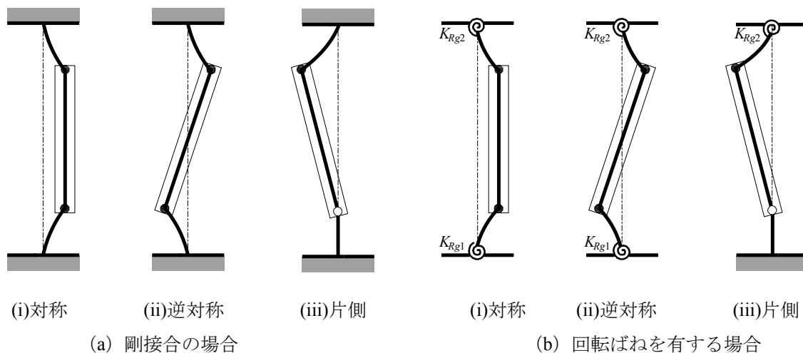
図 6.2.3 崩壊メカニズム 6.1)
