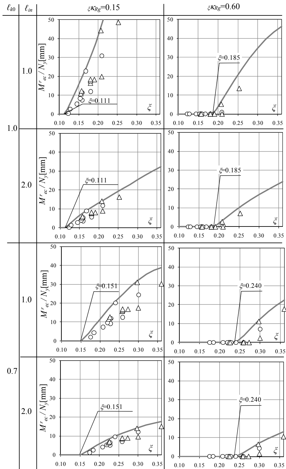
図 5.19 BRB の設計用偏心曲げモーメント M_{ec}^r / N_y
