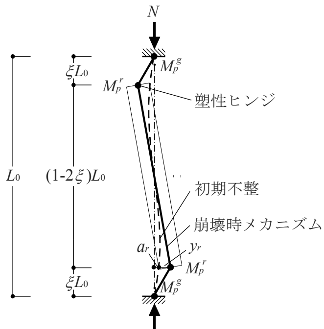
図 3.8 接合部端部に塑性ヒンジを有する場合の崩壊メカニズム
