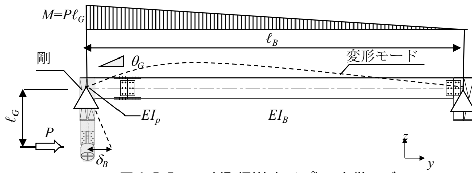
図 6.5.5 面外梁(剛節タイプ)の力学モデル
