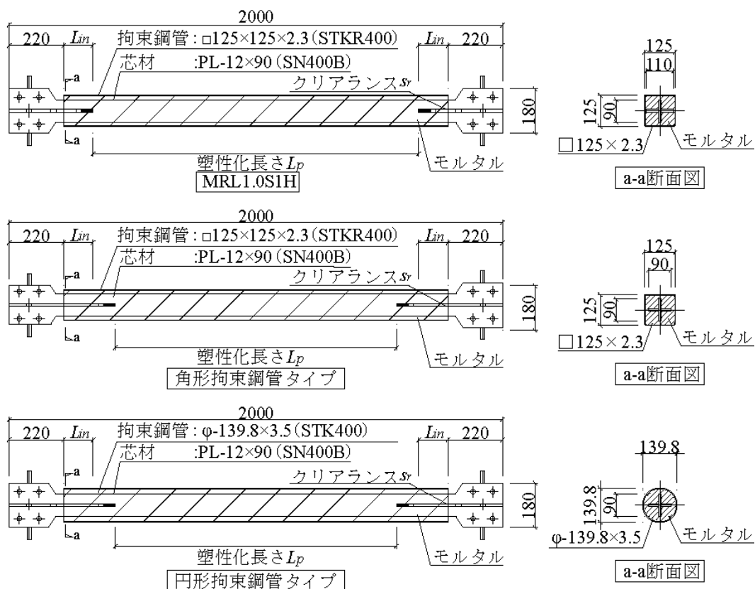
(c) 座屈拘束ブレース試験体
