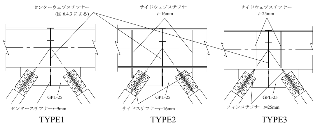
図 6.4.2 梁側接合部のディテール
