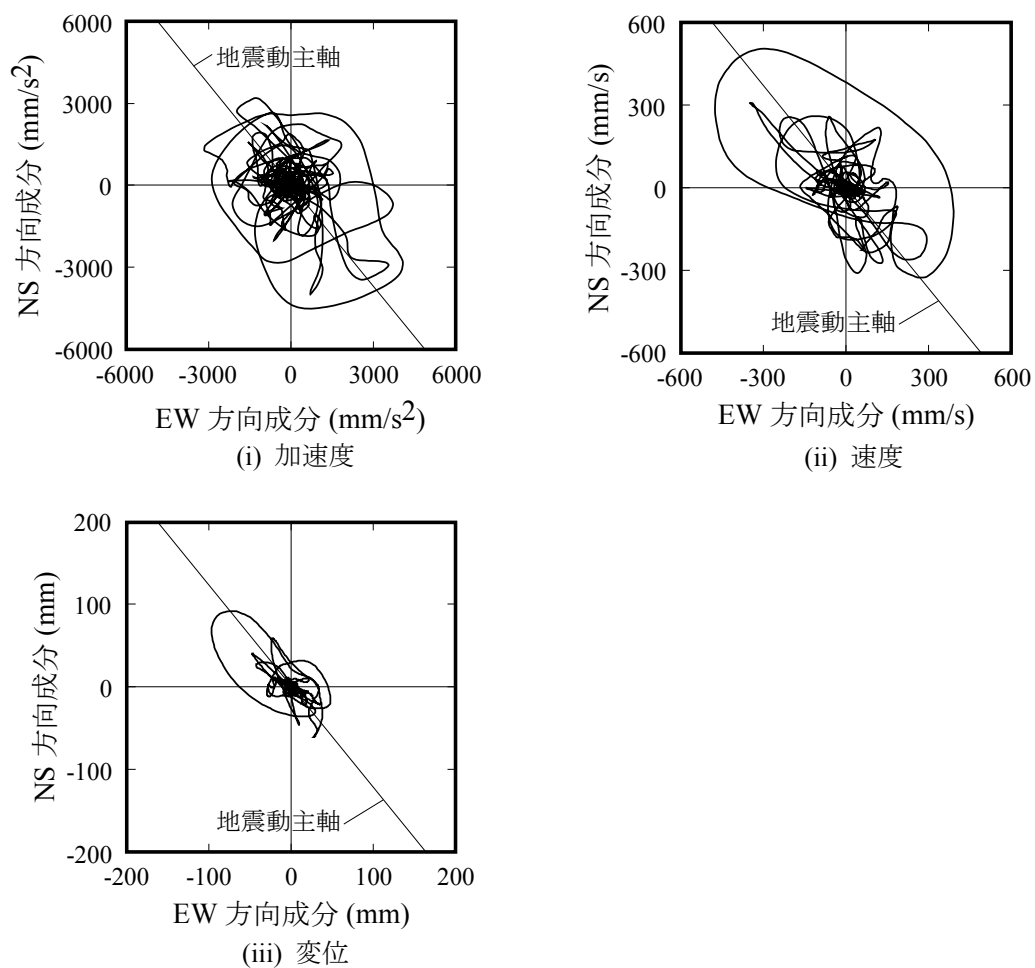
図 2.9 地震動オービットおよび地震動主軸 (JMA KOBE)
