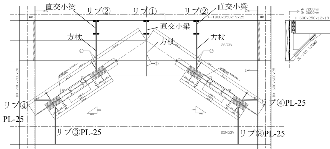
図 7.4 補強スチフナーの配置図
