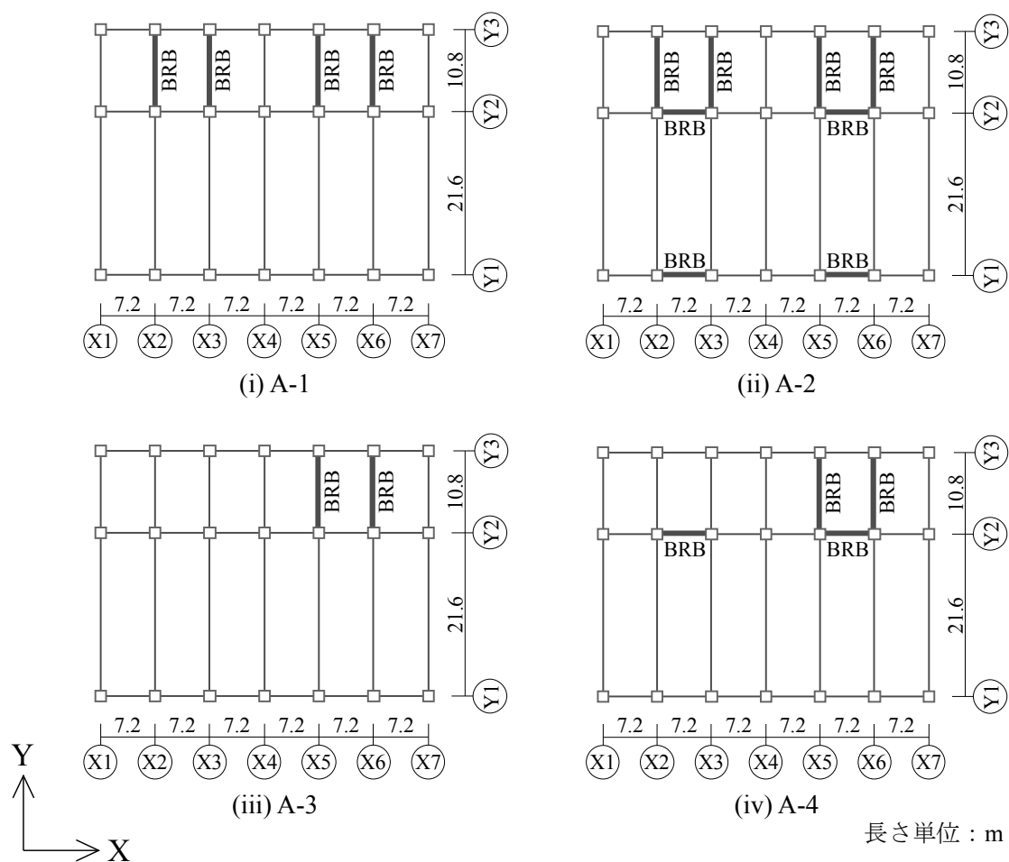
図 2.4 BRB 配置伏図（片コア形式）
