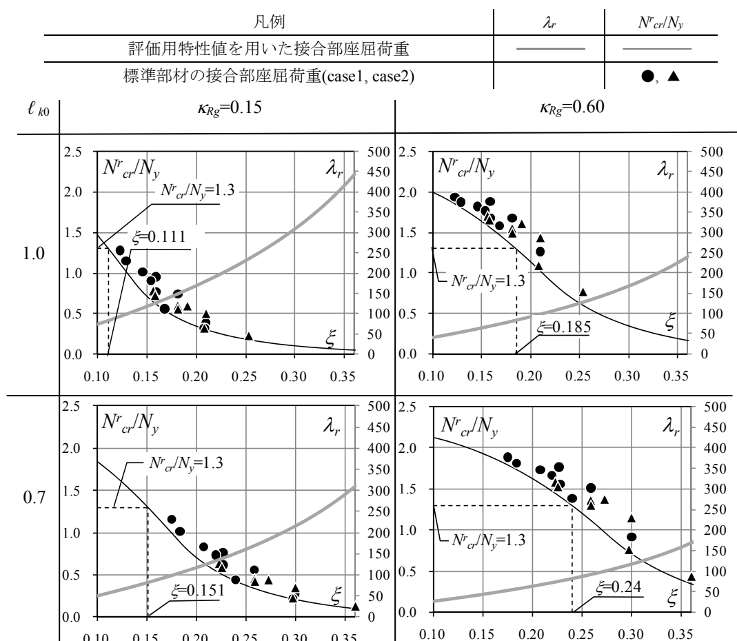
図 5.18 接合部の等価細長比 \lambda_r と規準化された接合部座屈荷重 N_{cr}^r/N_y
