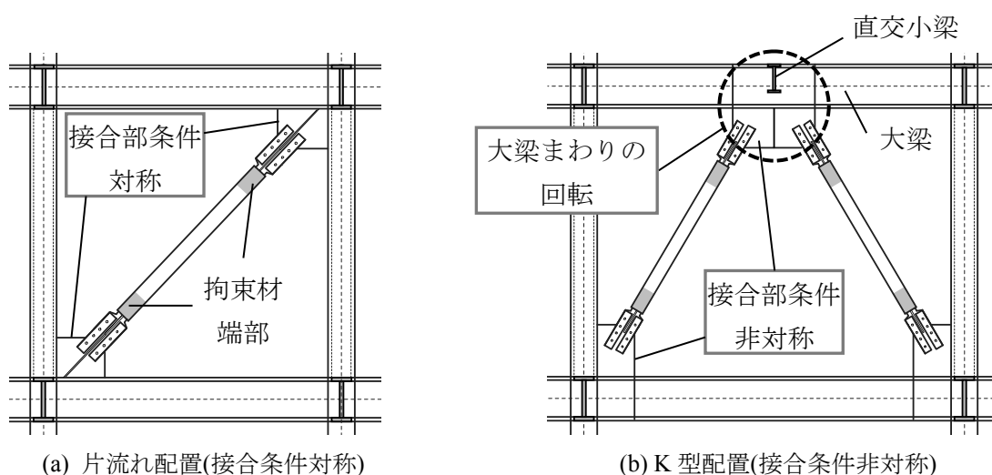
図 6.1.1 BRB の配置方法と接合部条件
