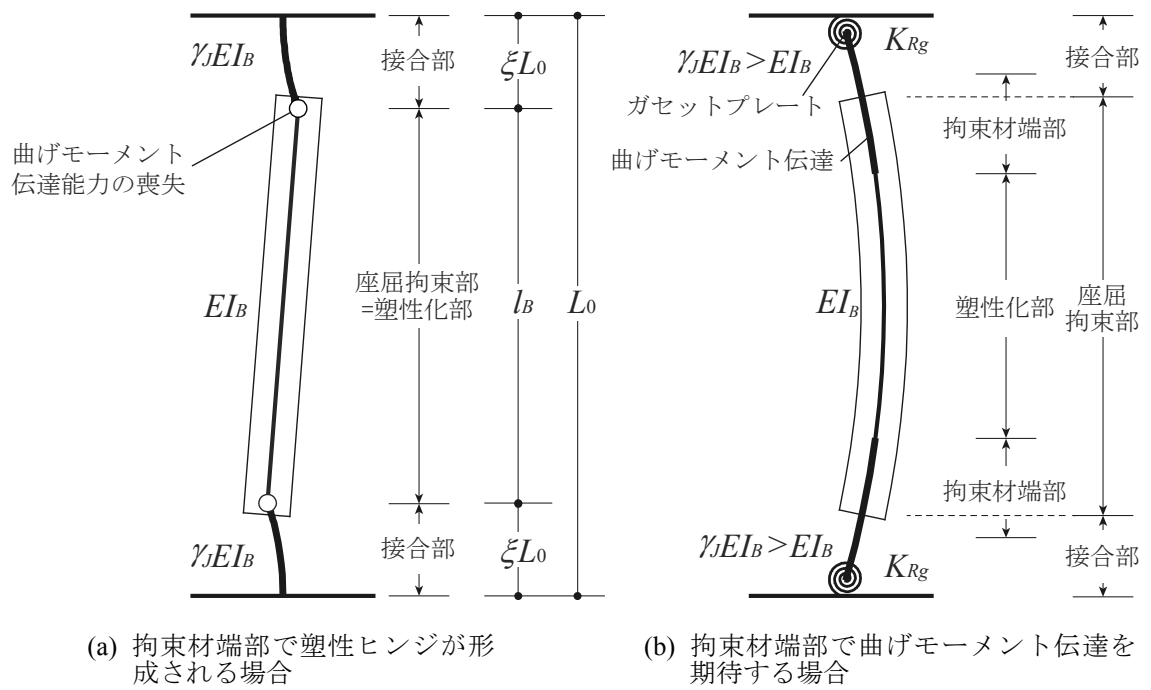
図 3.1 座屈拘束ブレースの機構安定性の考え方
