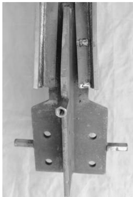
(b) 載荷後下部拘束材端部
