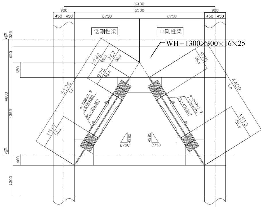
図 7.9 K 型配置された BRB の検討例 (高容量の BRB が取付く場合)
