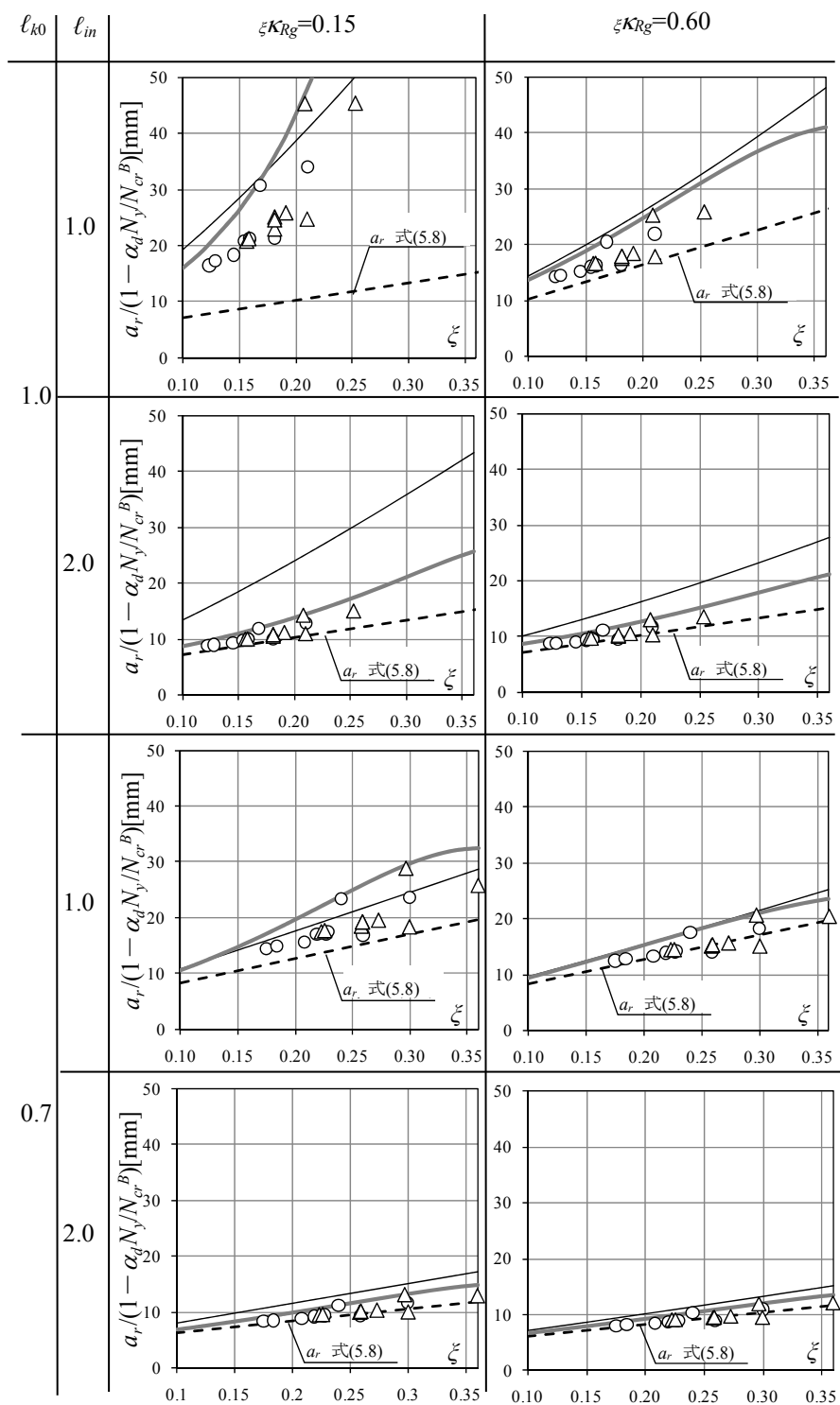
図 5.16 設計荷重時の座屈拘束材端部の変位
