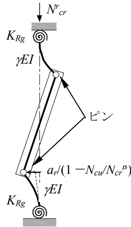
図 5.17 接合部座屈荷重のモデル図
