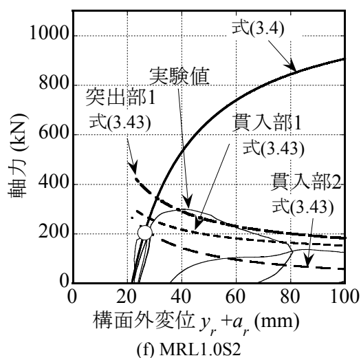
図 3.14 実験値と提案式の比較(軸力—面外変位関係)
