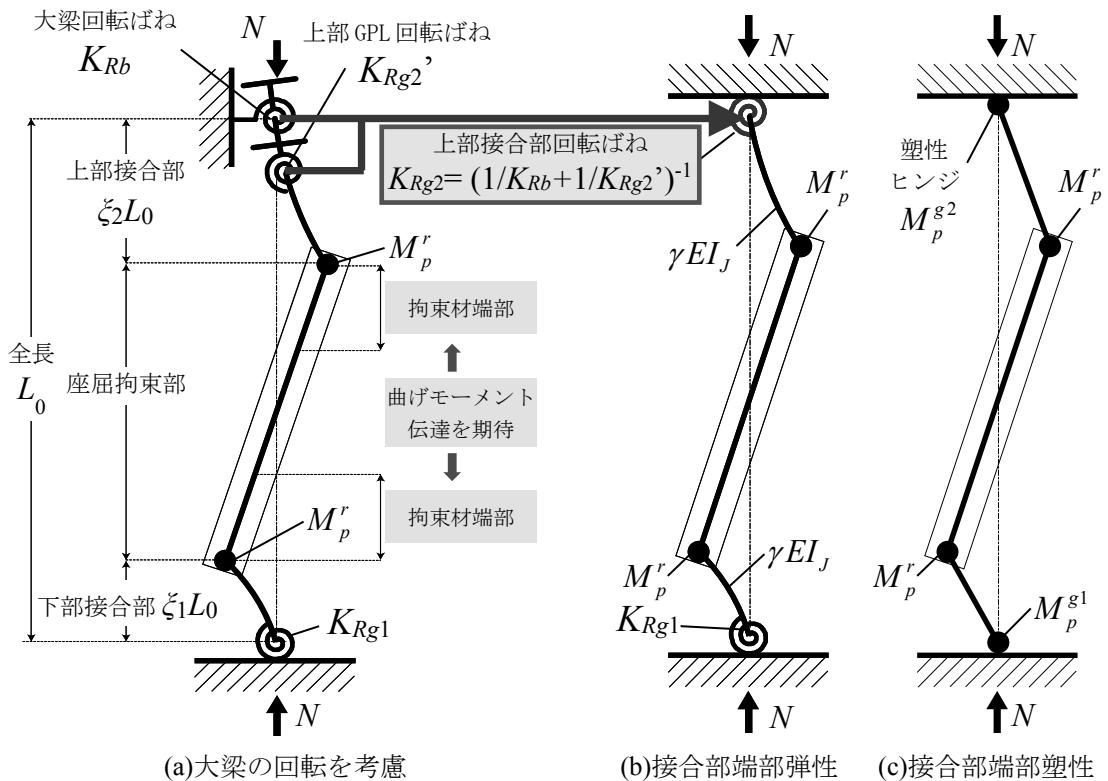
図 6.2.1 K型配置された座屈拘束ブレースの崩壊メカニズム
