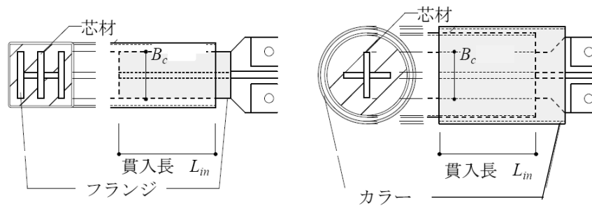
図 7.11 芯材突出部の補剛例
