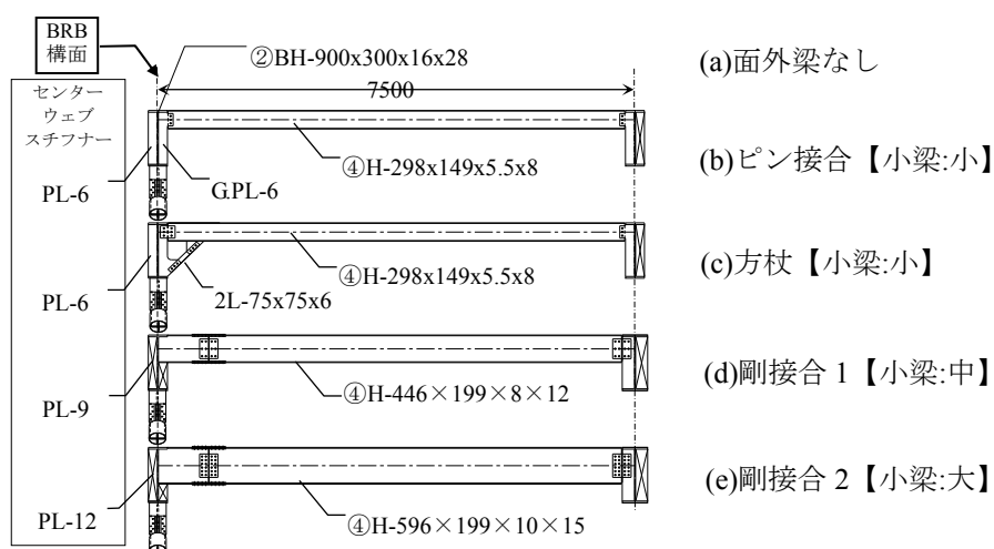
図 6.4.3 面外梁の取付き詳細
