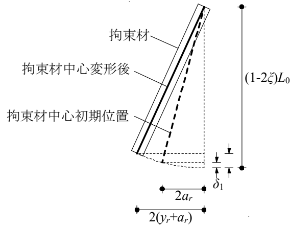
付図 3.1 拘束材の回転
