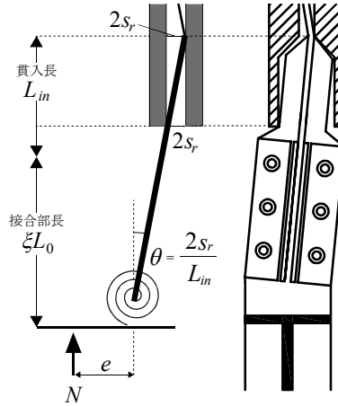
図 5.14 初期不整値 a_r のモデル化
