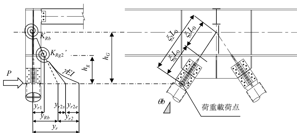
図 6.4.7 大梁の回転に伴う変位を含む接合部の力学モデル
