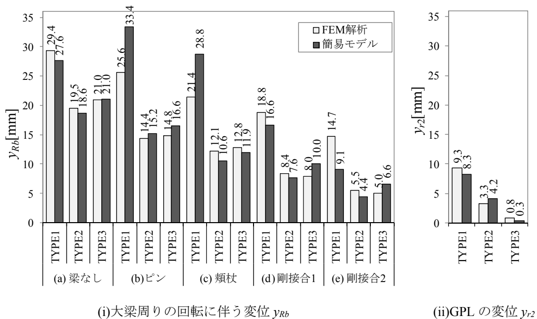
図 6.5.8 載荷点の変位の比較
