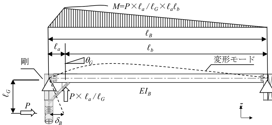
図 6.5.4 面外梁(方杖タイプ)の力学モデル
