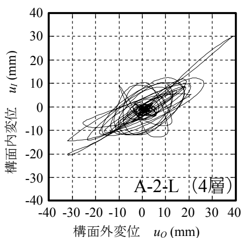
(iii) BRB 応答
