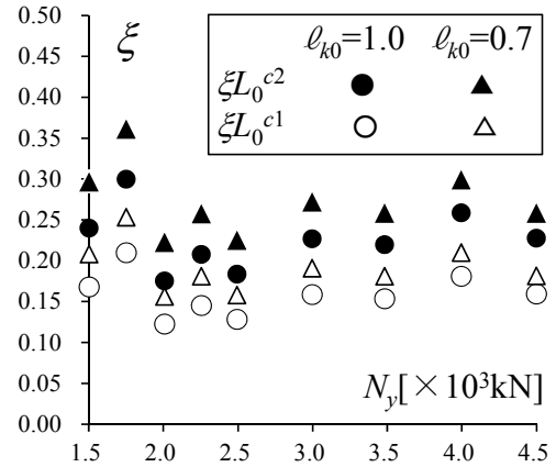
図 5.5 接合部長さ比 \xi の分布
