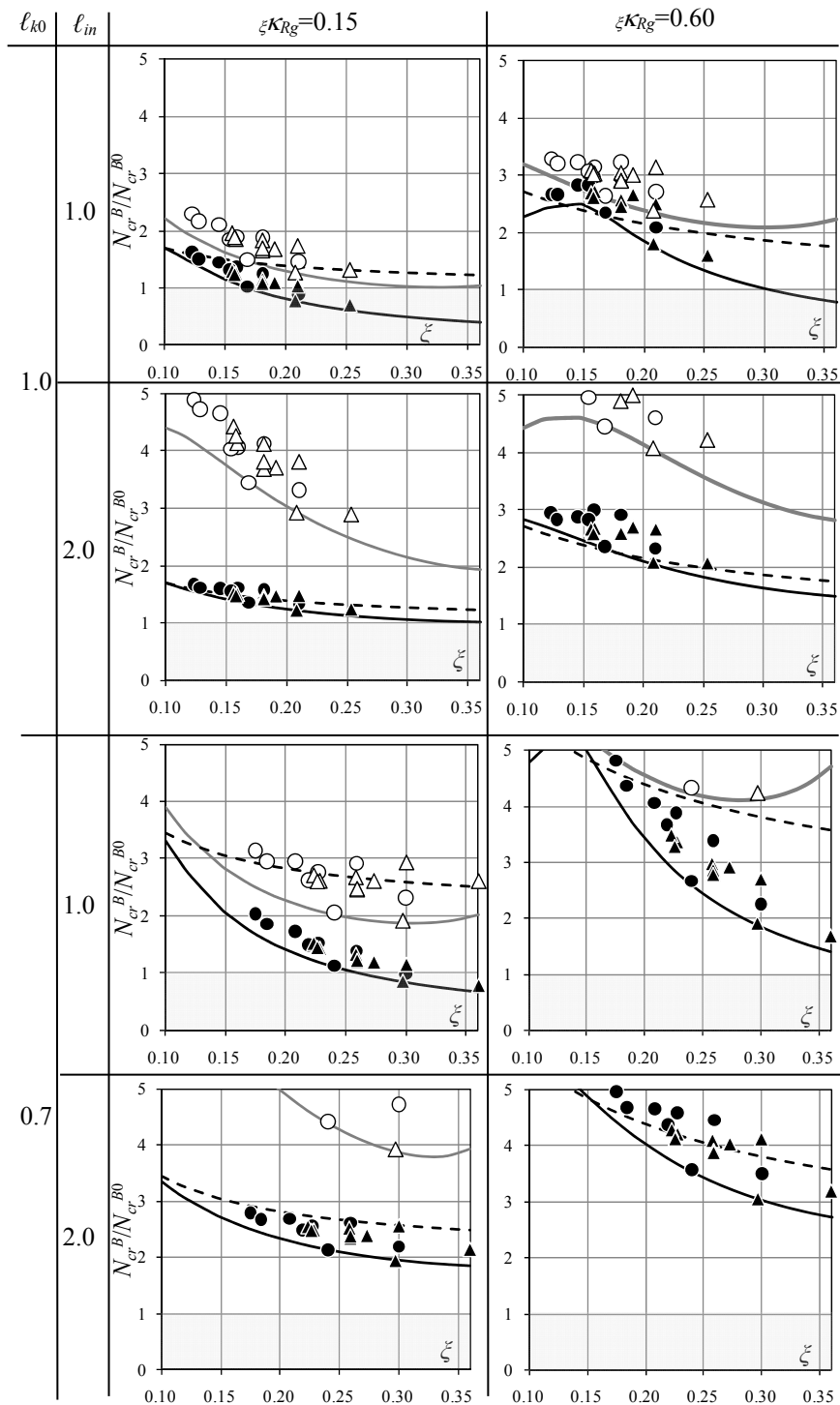
図 5.13 両端ピン座屈荷重に対する各モデルの弾性全体座屈荷重
