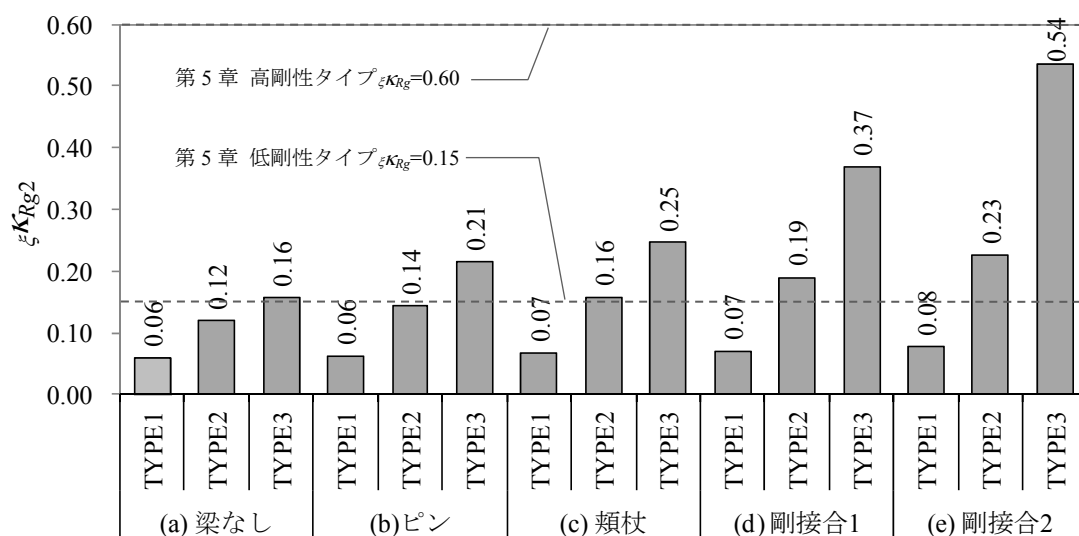
図 6.4.9 上部接合部の無次元化回転ばね剛性比
