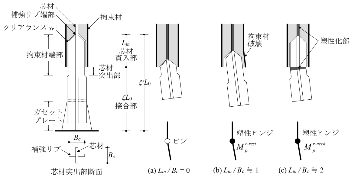
図 3.3 拘束材端部の曲げモーメント伝達機構
