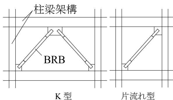
図 2.2 BRB 配置図
