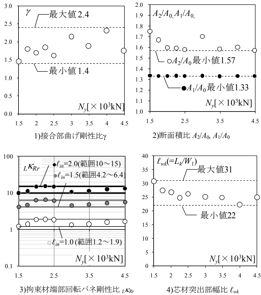
図 5.2 標準部材の評価用特性値の分布
