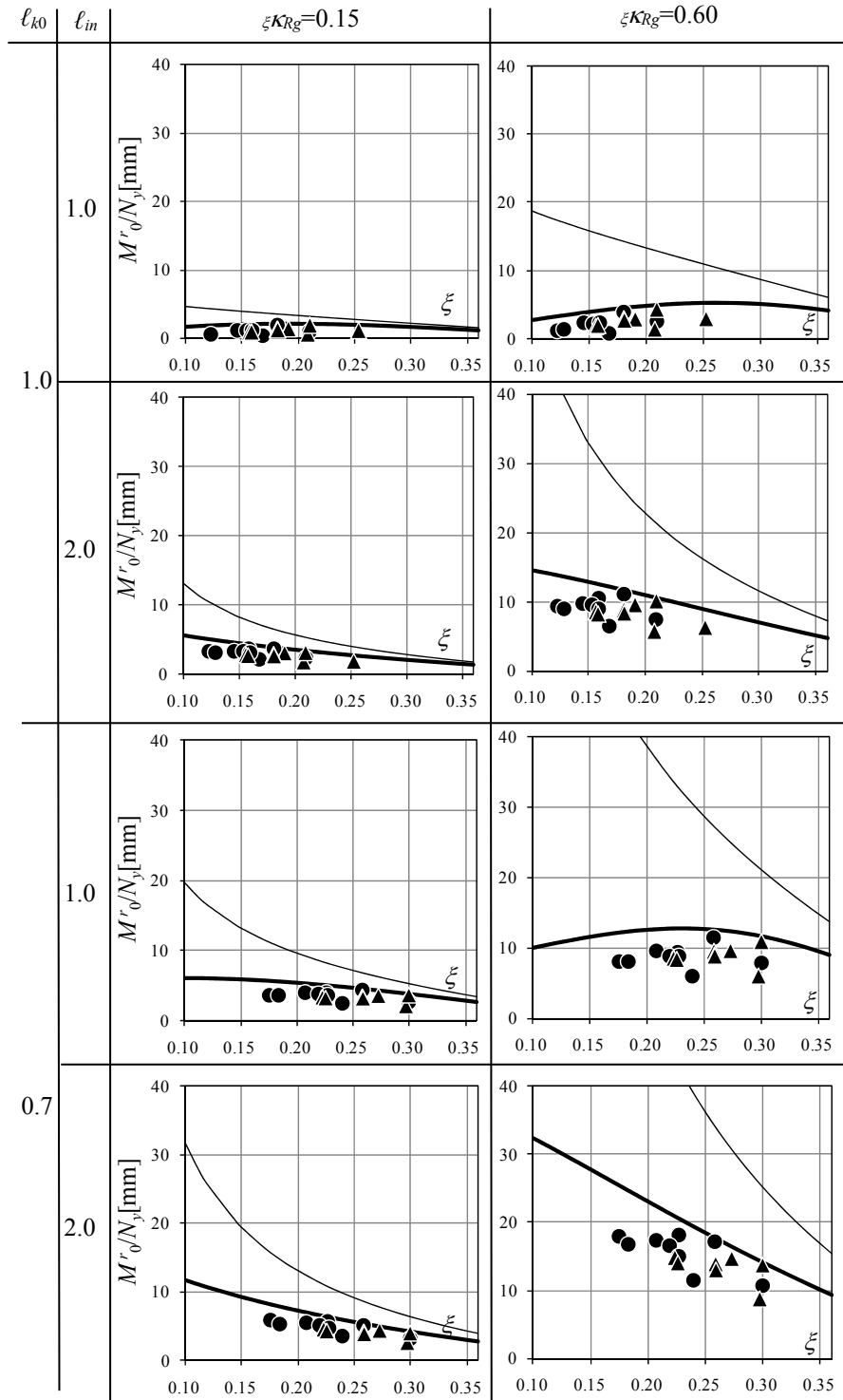
図 5.21 各モデルの設計用付加曲げモーメント M_0^r/N_y
