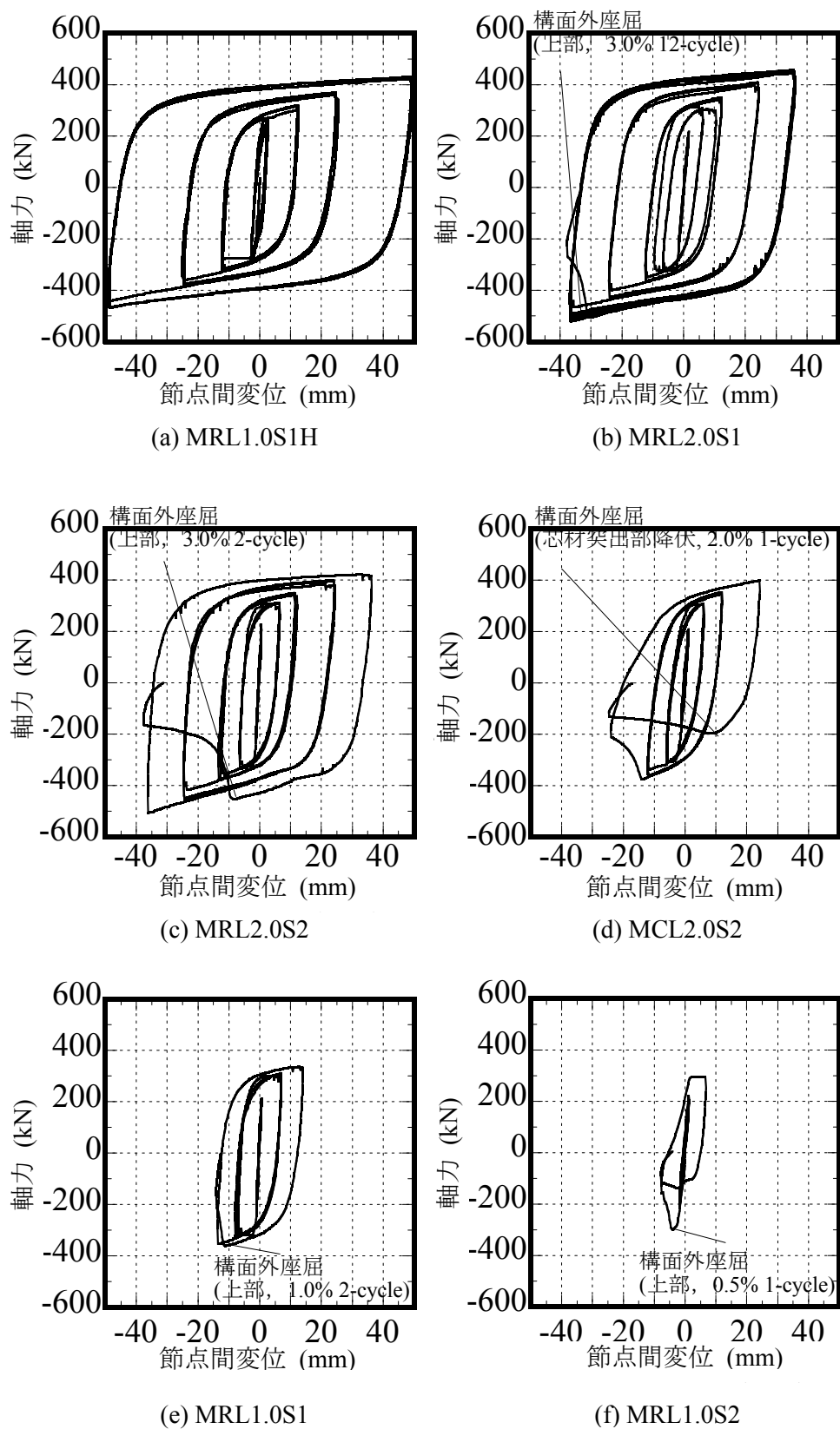
図 3.13 軸力－節点間変位関係
