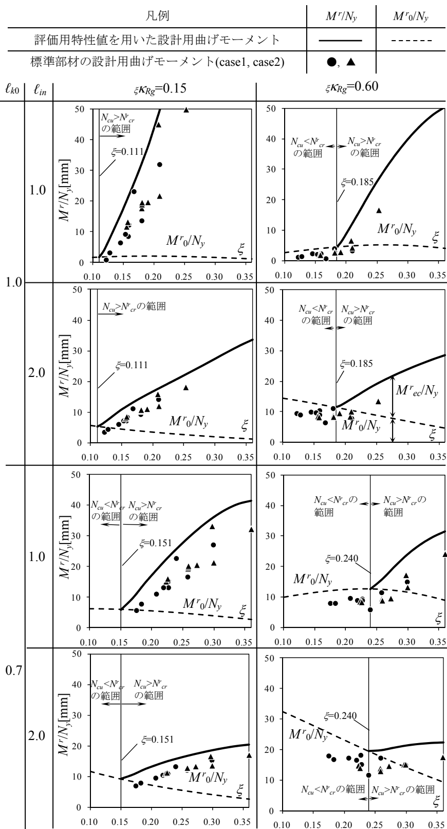
図 5.22 芯材突出部の設計用曲げモーメント
