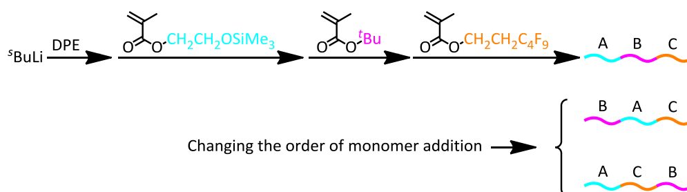
Scheme 1- 1. 同程度の反応性を有するモノマーを用いたトリブロック共重合体の合成
