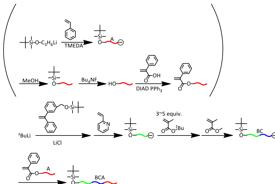
Scheme 2- 4. BCA トリブロック共重合体の合成
