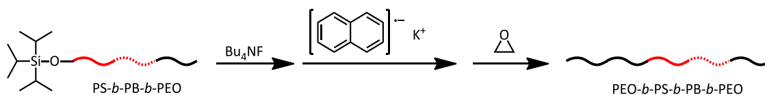
Scheme 1- 8. 末端ブロックの鎖長の非対称なテトラブロック共重合体の合成
