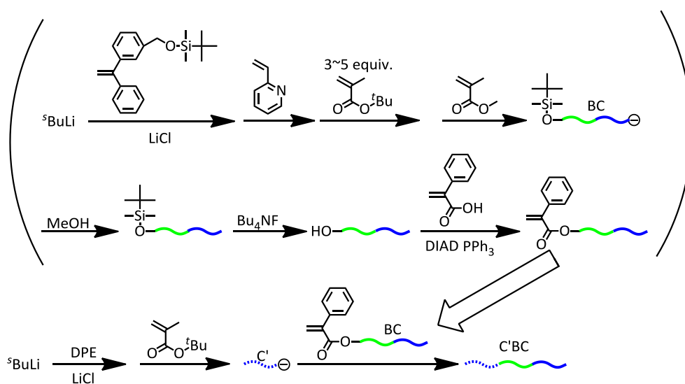
Scheme 3- 7. C'BC トリブロック共重合体の合成
