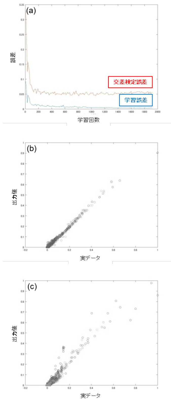
図 6-03. 第一段階目におけるバックプロパゲーション学習をした結果 ; (a) はオートエンコーダ学習時の誤差推移プロット、(b) は交差検定に基づく学習データ(80%)に対する実測値を横軸に予測値を縦軸にとったプロット、(c) 交差検定に基づく検定データ(残り 20%)に対する実測値を横軸に予測値を縦軸にとったプロット
