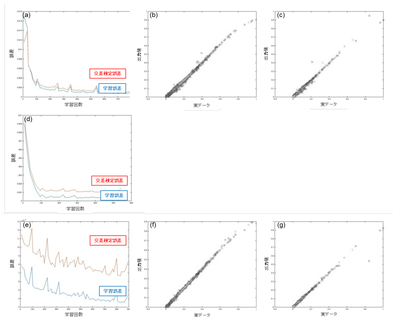
図6-09. 1500種類の香気化合物の構造パラメータに対してオートエンコーダーを用いた構造情報空間の圧縮；(a) は第一段目の学習におけるオートエンコーダ学習時の誤差推移プロット、(b) は第一段目の学習における交差検定に基づく学習データ(80%)に対する実測値を横軸に予測値を縦軸にとったプロット、(c) は第一段目の学習における交差検定に基づく検定データ(残り20%)に対する実測値を横軸に予測値を縦軸にとったプロット (d) は第二段目の学習におけるオートエンコーダ学習時の誤差推移プロット、(e) は第三段目の学習におけるオートエンコーダ学習時の誤差推移プロット、(f) は第三段目の交差検定に基づく学習データ(80%)に対する実測値を横軸に予測値を縦軸にとったプロット、(g) は第三段目の交差検定に基づく検定データ(残り20%)に対する実測値を横軸に予測値を縦軸にとったプロット
