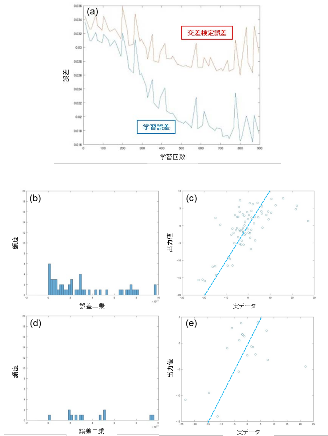
図 6-08. 80 次元まで圧縮した香気パラメータをもとにしたニューラルネットワークを用いた応答予測; (a)バックプロパゲーション学習過程におけるエラー推移、(b)トレーニングデータ(予測値-実測値) 2 ヒストグラム、(c) トレーニングデータ予測値-実測値プロット、(d)交差検定(予測値-実測値) 2 ヒストグラム、(e) 交差検定予測値-実測値プロット
