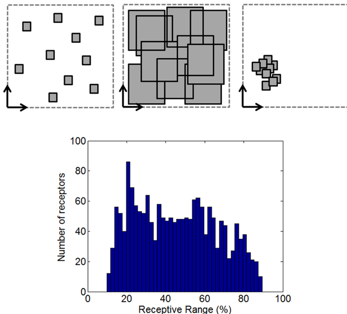
図 1-27. 複数の嗅覚受容体の相関関係とシステムの受容範囲選択性の相互関係；(A)抽象的な受容範囲、選択性と嗅覚受容体の相関関係、(B)1778 ピクセルの受容範囲の分布 [076]
