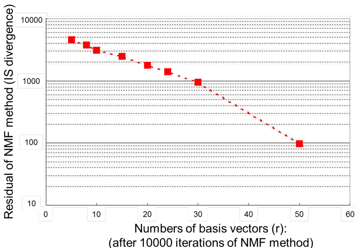
図 3-02. 要素臭の数とデータ \mathbf{V} 近似行列 \mathbf{WH} の残差の関係 (各基底数に対し NMF における距離演算は IS ダイバージェンス, 収束計算の繰り返し回数はいずれも 10000 回行い、残差を算出)
