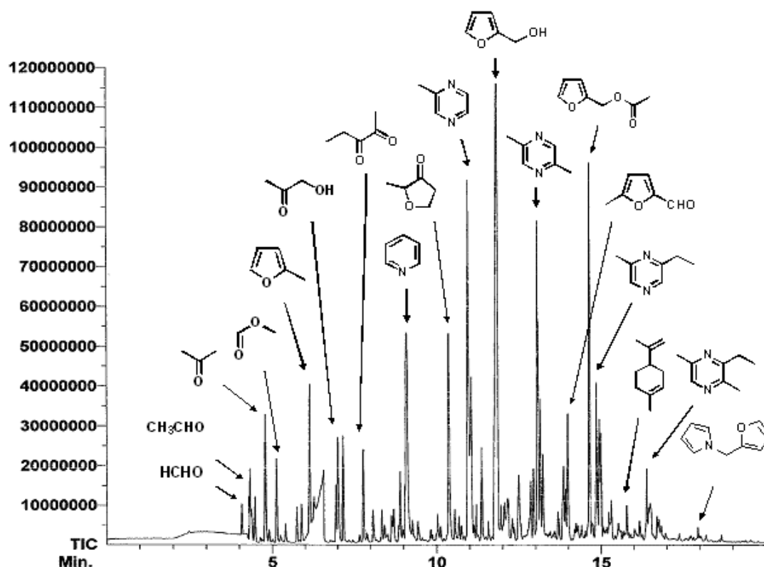
図 1-15. 香気成分の分析例 [041]
