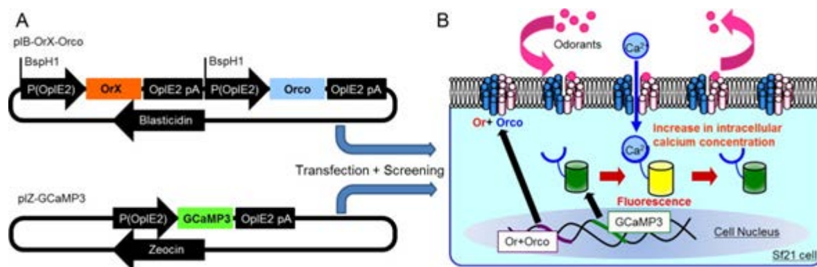
図 1-19.昆虫のレセプター遺伝子を導入した、バイオセンサー細胞の作製；(A) Sf21 母細胞へヘテロ遺伝子発現させる発現ベクター、(B) 安定株種細胞の動作 [061]
