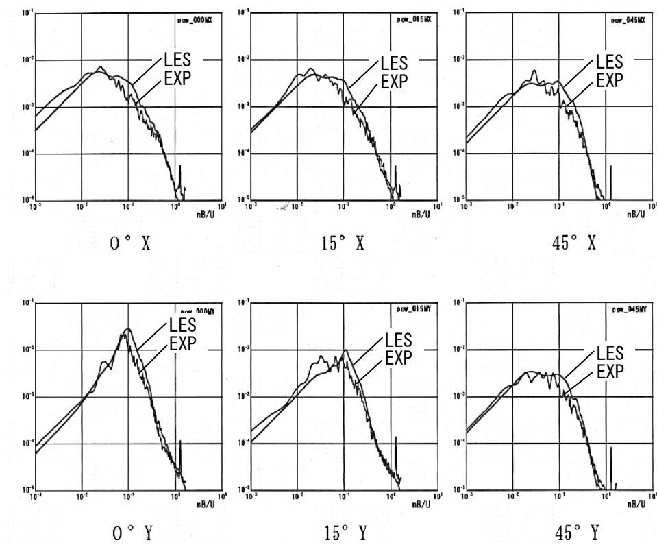
付図 1.2 一般化風力係数のパワースペクトル
