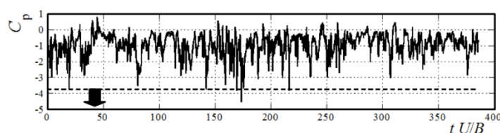
図 6.16 外圧係数時刻歴およびサンプリングレベル
