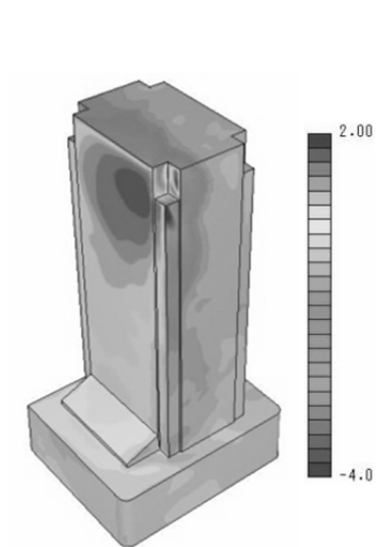
図 6.19 外圧係数の面分布
