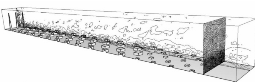
図 4.4 流入変動風作成モデル
