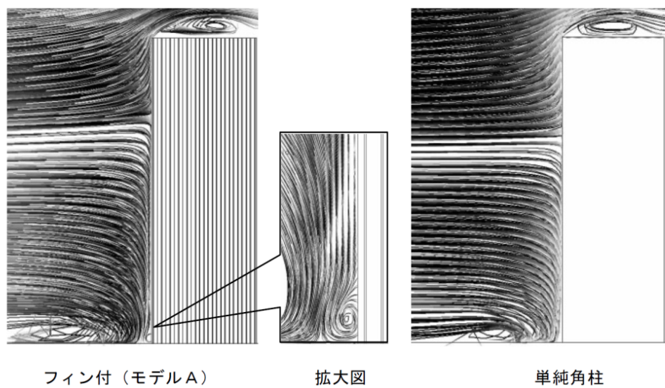
図 5.28 中央断面における流れのパターン
