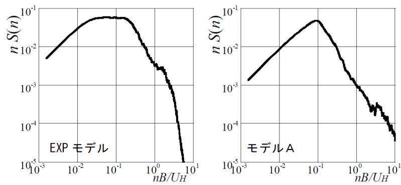
図 5.16 負圧変動のパワースペクトル
