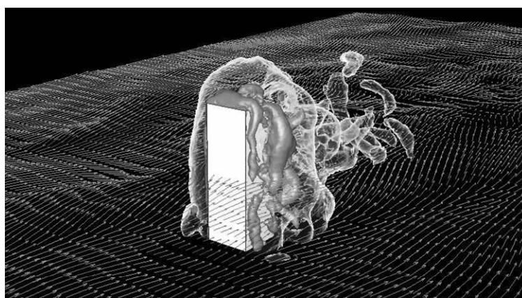
図 3.8 角柱周囲の瞬間流れ場（ベクトル分布）と瞬間圧力場（負圧等値面）
