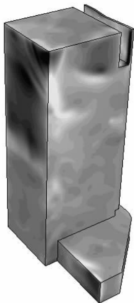
図 7.10 瞬間圧力分布
