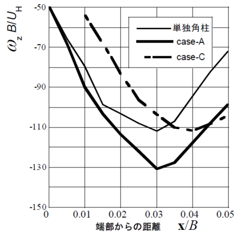
図 4.34 隅角部における渦度分布
