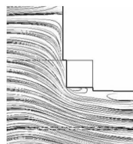
図 6.18 隅角部の渦構造
