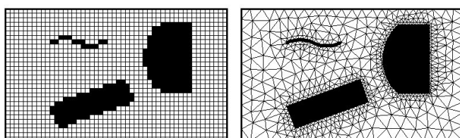
構造格子（直交格子） 非構造格子（テトラ要素）
