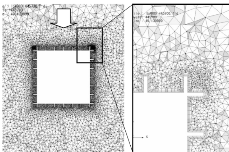
図 5.5 計算格子
