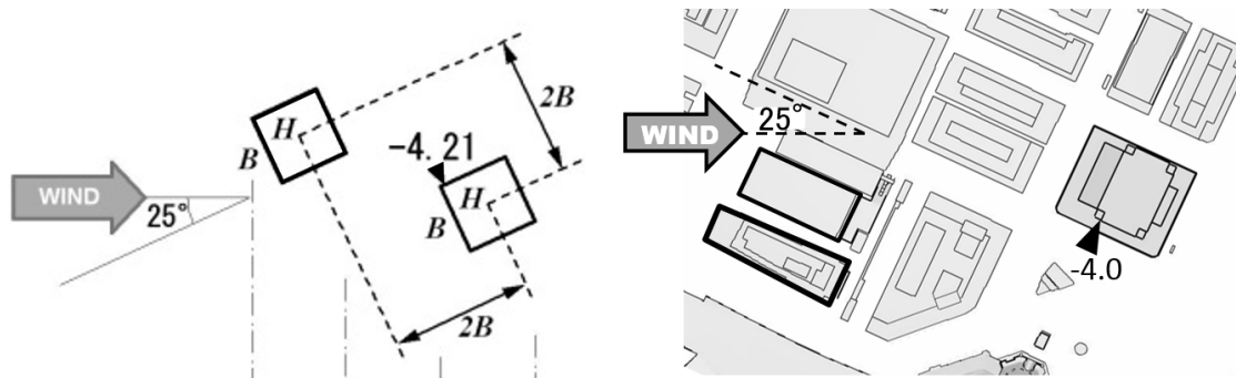
図 6.22 ピーク負圧発生に関する建物配置および風向角の類似性
