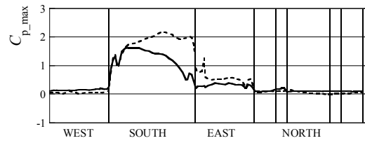
正圧側ピーク風圧係数
