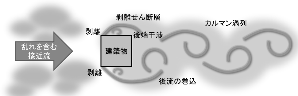
図 3.6 角柱周囲の乱流構造に関する概要図
