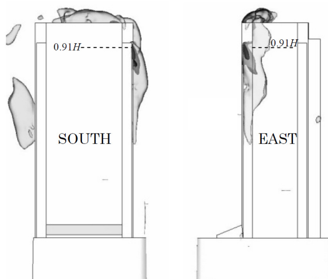
図 6.20 負圧等値面
