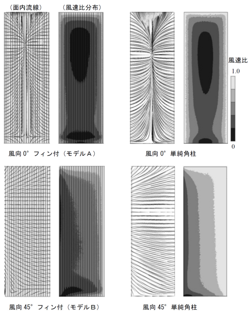
図 5.25 風上面近傍における平均風速分布
