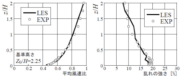
図 4.5 流入変動風のプロファイル
