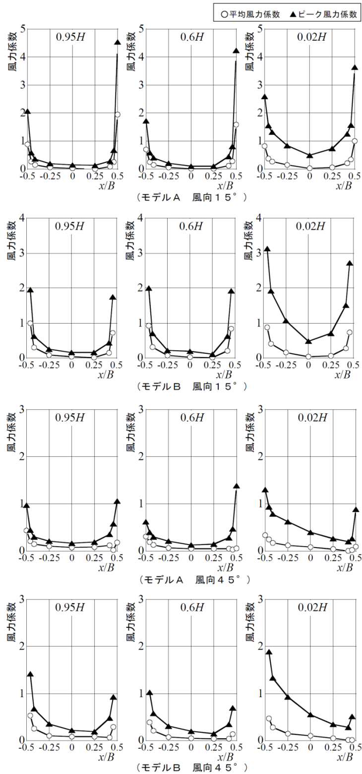
図 5.22 風力係数の水平分布
