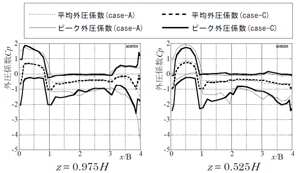
図 4.31 外圧係数の水平分布
