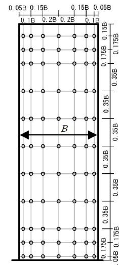
図 3.3 測定点配置
