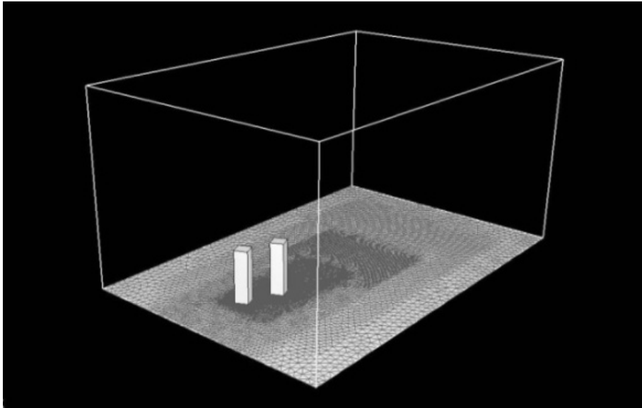
図 4.7 計算領域
