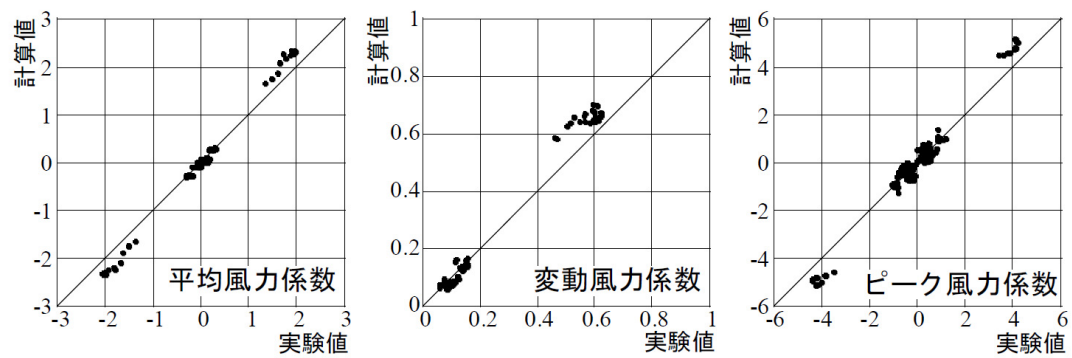
図 5.6 風力係数に関する実験値と計算値の相関図
