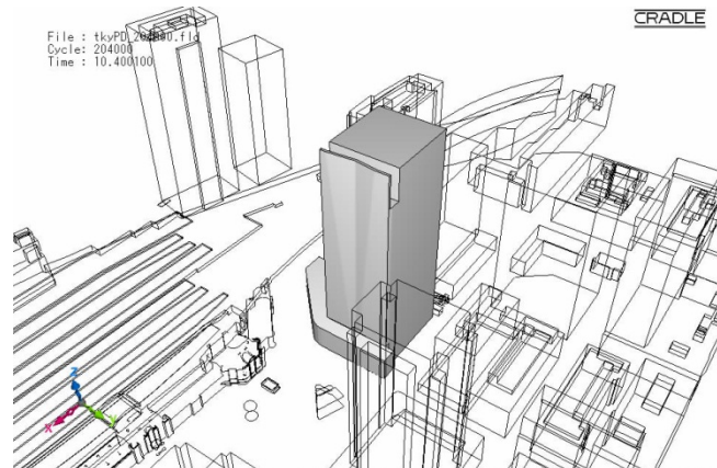
図 7.5 計算モデル形状
