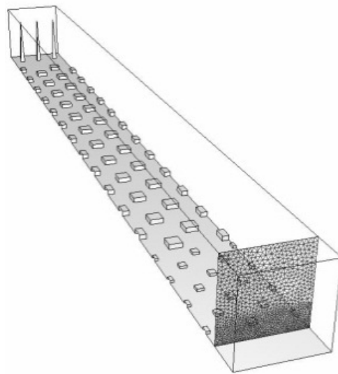
図 5.2 流入変動風作成モデル
