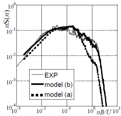
図 4.11 風圧係数のパワースペクトル
