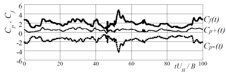
図 5.23 端部フィンにおける風圧係数および風力係数の時刻歴波形
