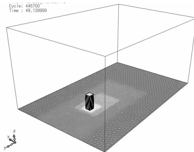
図 5.4 計算領域
