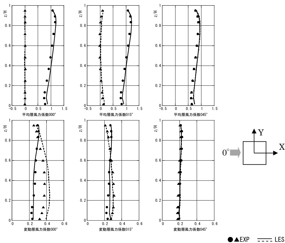
付図 1.1 層風力係数の高さ方向分布
