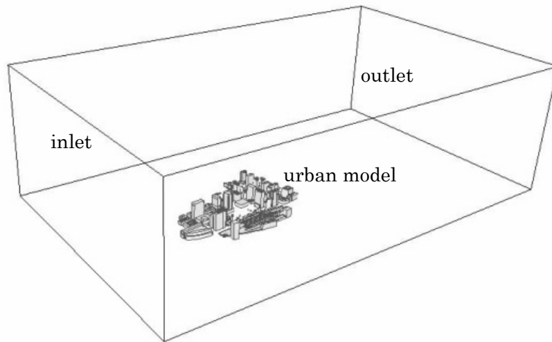
図 6.5 計算領域
