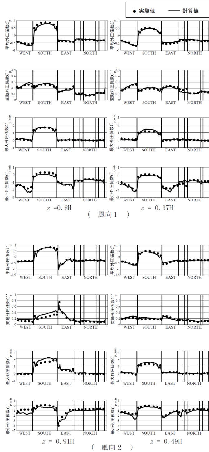
図 6.15 外圧係数の水平分布
