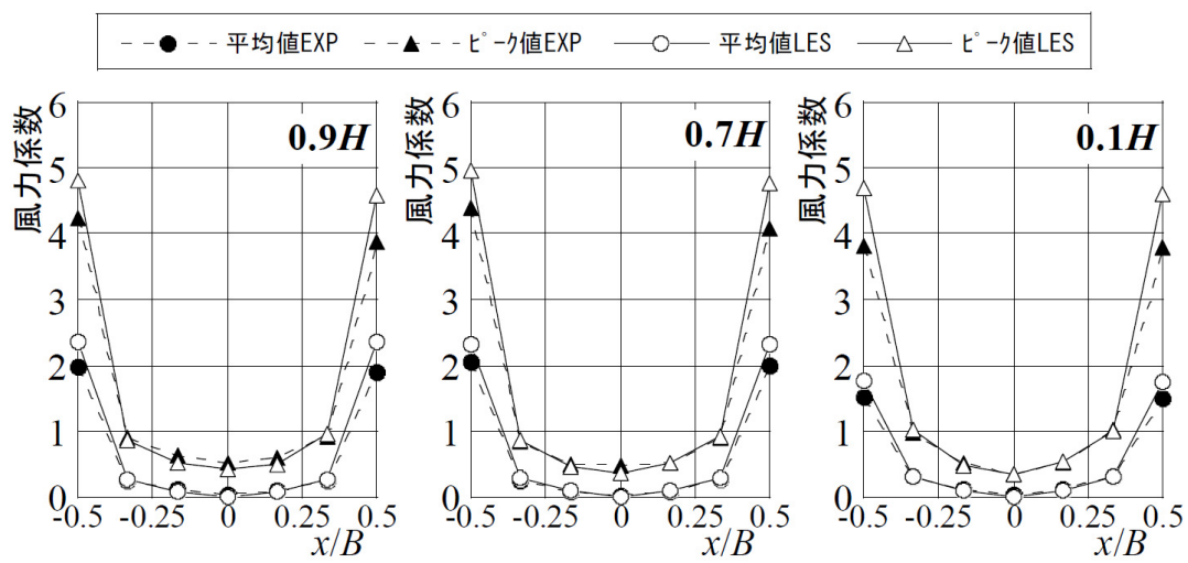
図 5.7 風力係数の水平分布
