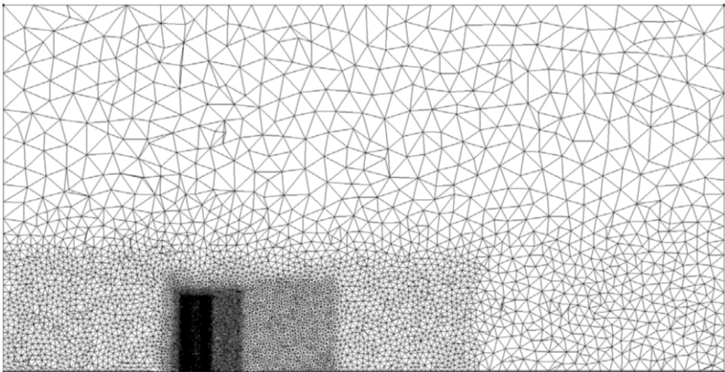
鉛直断面
