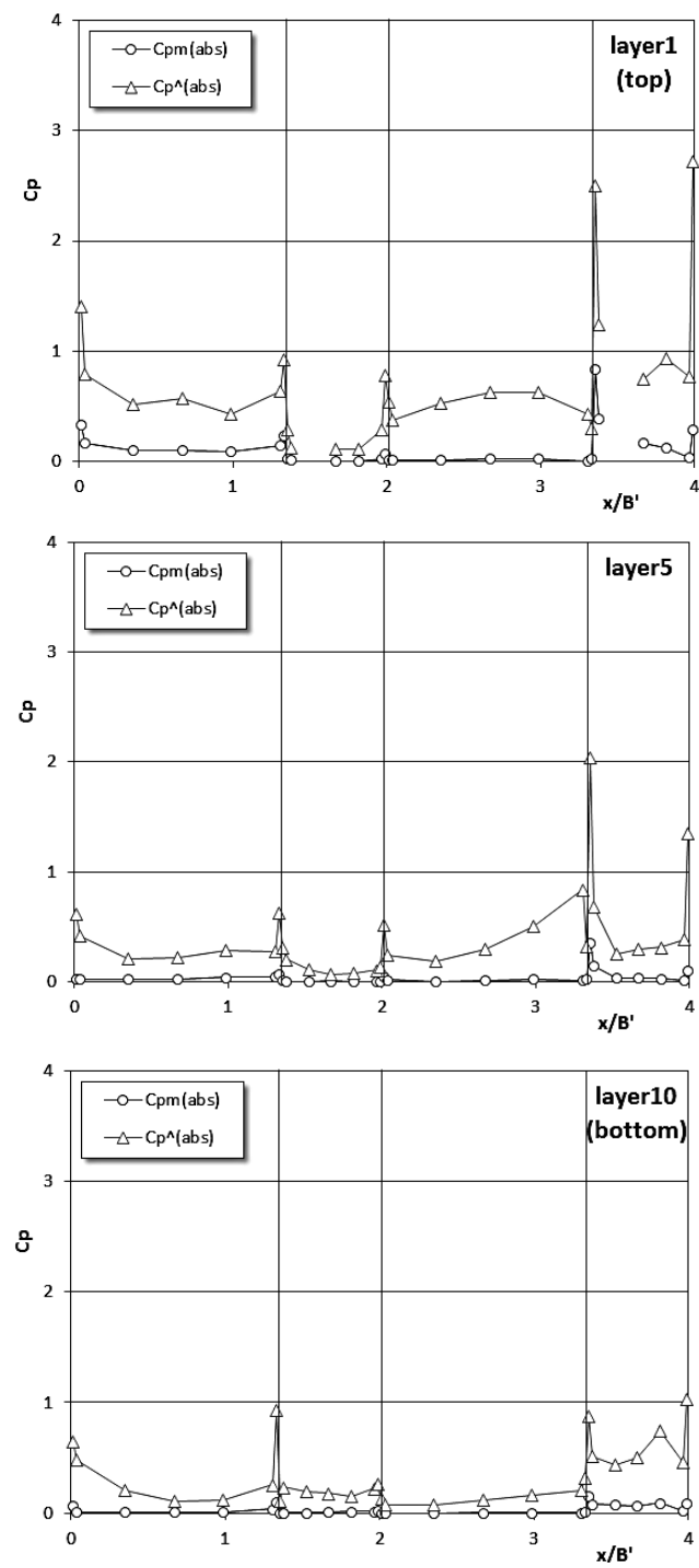
図 7.21 フィンの風力係数に関する水平分布
