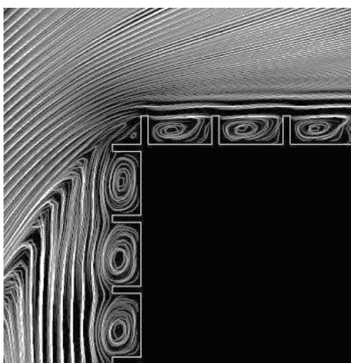
図 5.13 建物およびフィン周囲の流れ場
