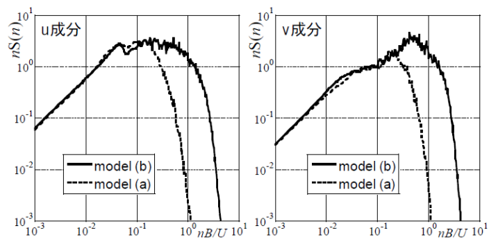
図 4.10 変動風速のパワースペクトル
