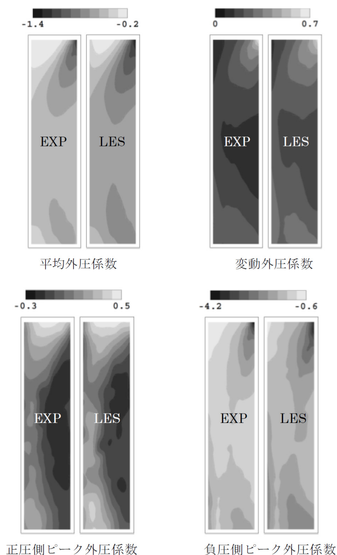
図 4.18 外圧係数の面分布 (case-A)
