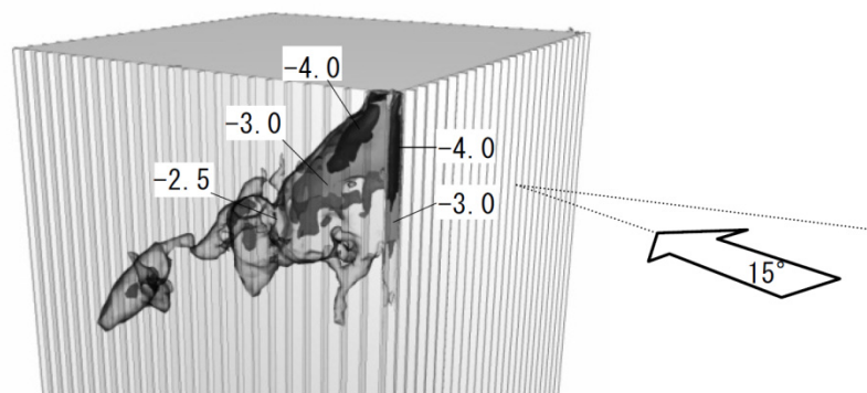
図 5.24 負圧場の等値面
