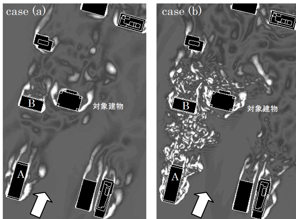
図 6.7 瞬間渦度分布
