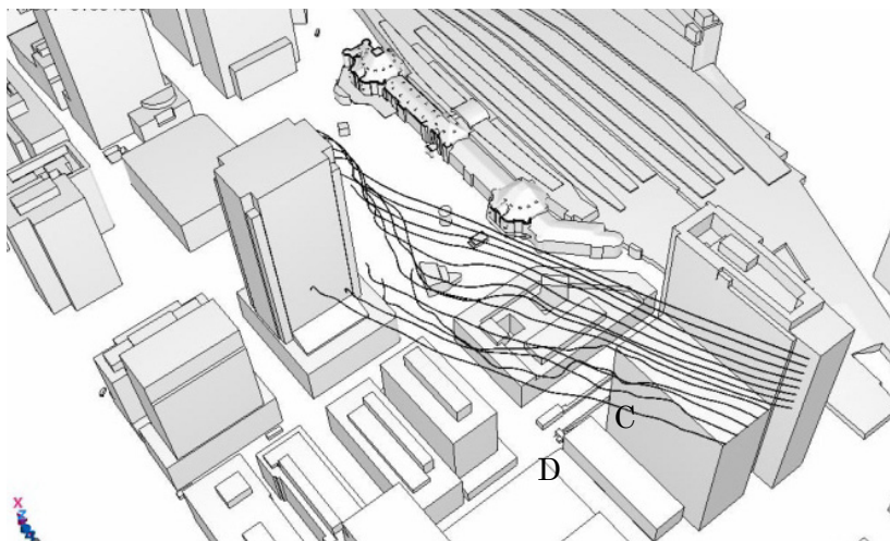
図 6.23 風上建物からの流線
