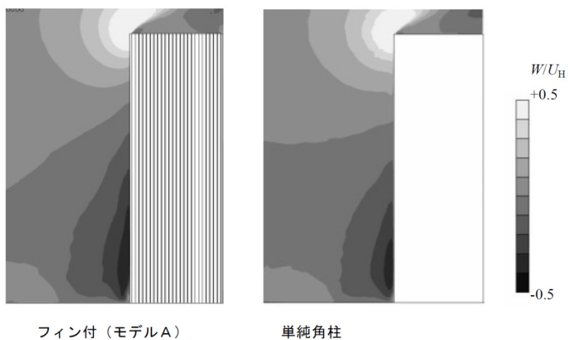
図 5.27 中央断面における風速分布 (鉛直成分)
