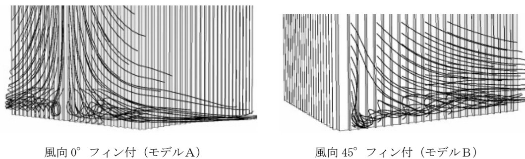
図 5.26 地上付近に発生する渦構造
