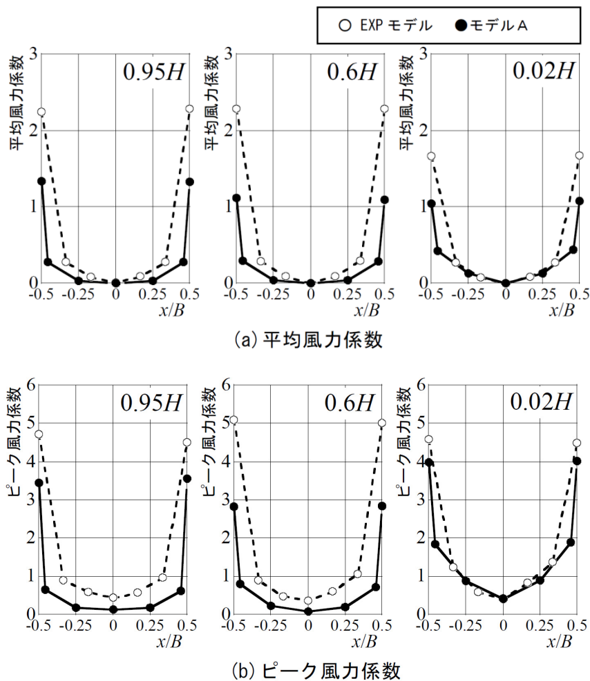
図 5.11 風力係数の水平分布
