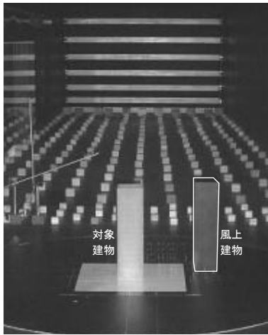
図 4.1 風洞実験
