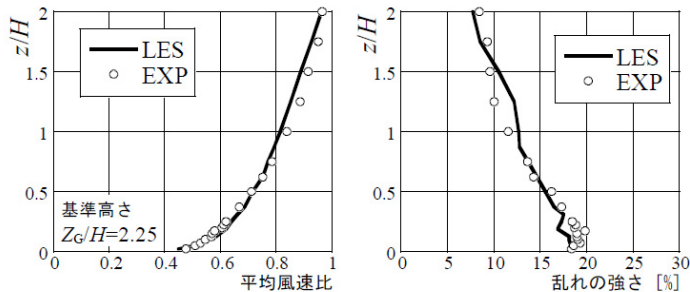
図4.5 流入変動風のプロファイル
