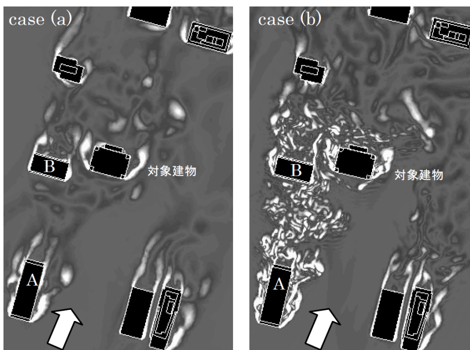
図 6.7 瞬間渦度分布
