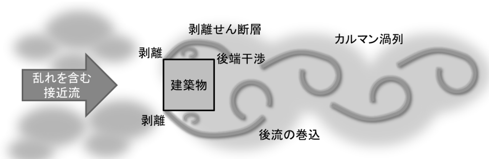
図 3.6 角柱周囲の乱流構造に関する概要図
