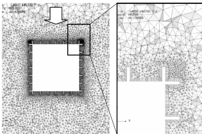
図 5.5 計算格子
