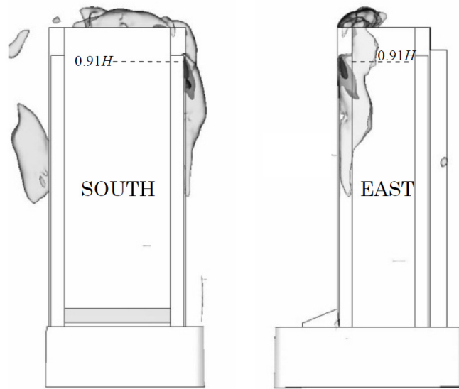
図 6.20 負圧等値面
