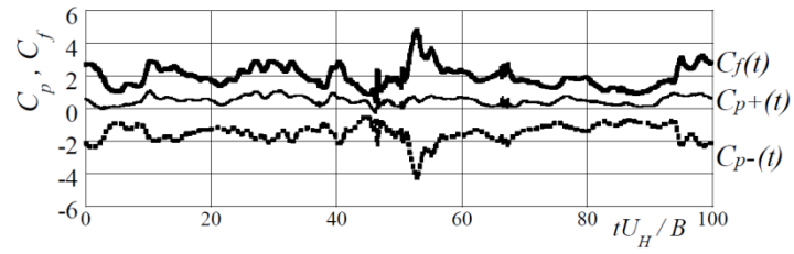
図 5.23 端部フィンにおける風圧係数および風力係数の時刻歴波形
