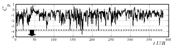
図 6.16 外圧係数時刻歴およびサンプリングレベル
