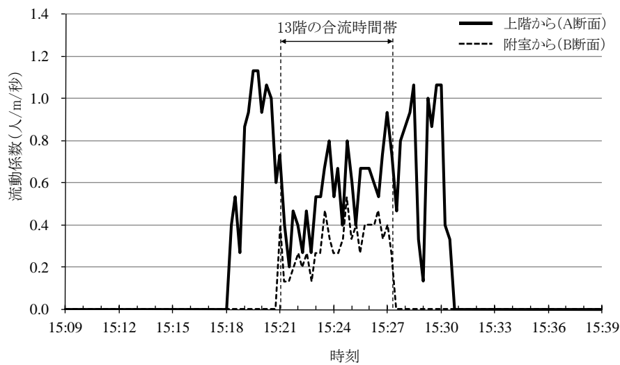
図3-20 13階の階踊り場の流動係数(階段避難シミュレーションの結果)
