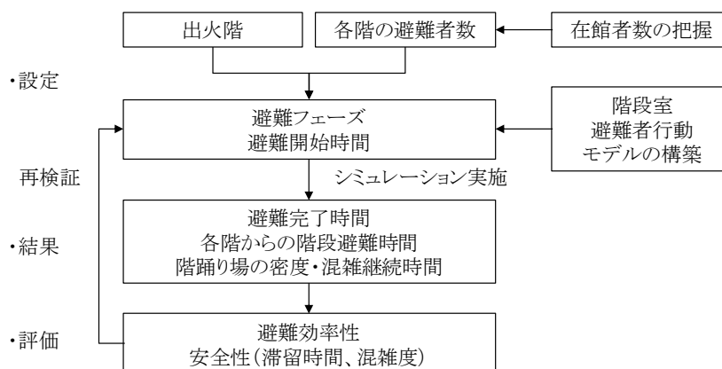
図4-10 階段避難シミュレーションによる検証手順
