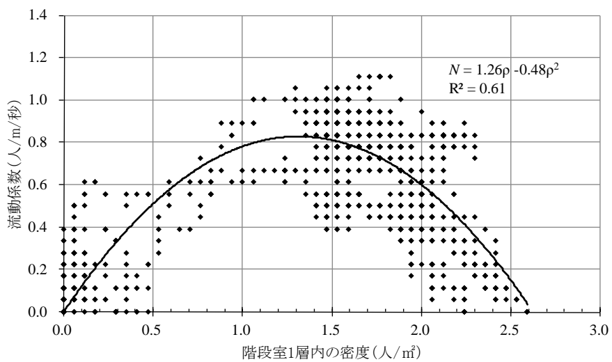
図 2-33 11 階階段室 1 層内の密度と流動係数の関係
