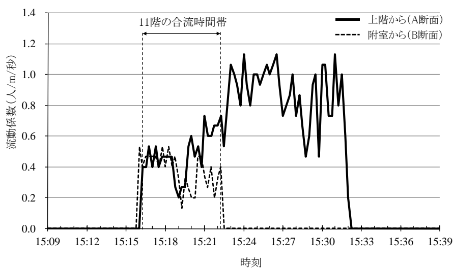
図3-19 11階の階踊り場の流動係数 (階段避難シミュレーションの結果)
