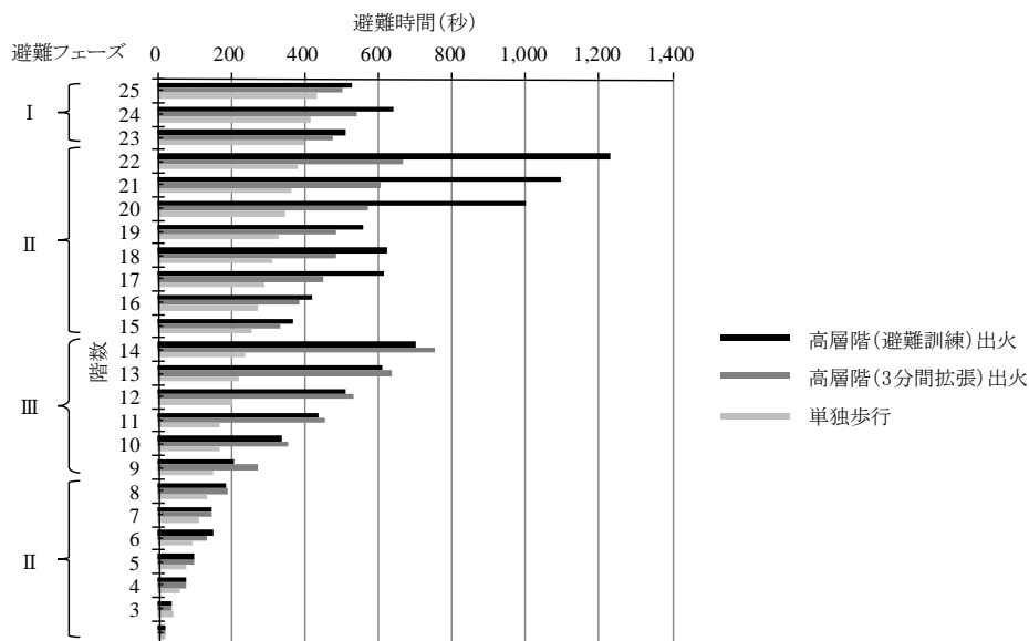
図 4-28 各階からの平均階段避難時間（出火階が高層階の場合）
