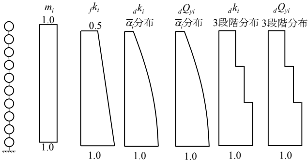
図 2 解析モデル
