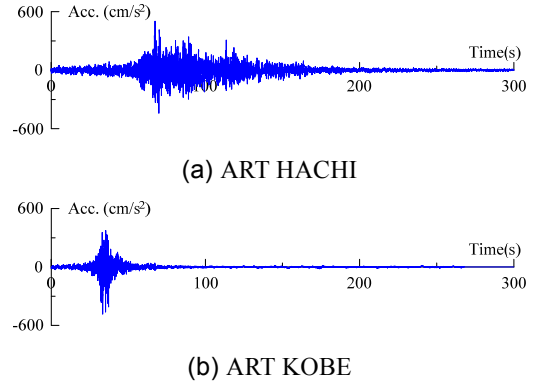
図 5 入力加速度波形 (レベル 2)
