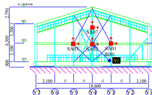
図1 東立面図
