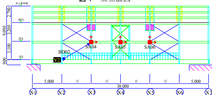
図2 北立面図
