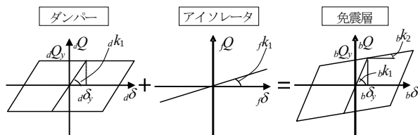
図 2 免震層の復元力特性 Fig. 2 Hysteresis properties of seismic-isolation layer
