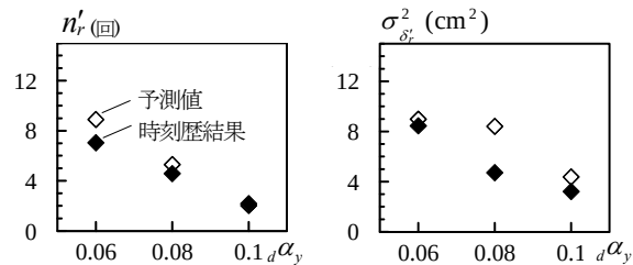
(a) シフトの発生回数 (a) Occurrence count of shift (b) シフト変位の分散 (b) Variance of shift
