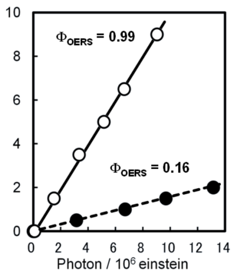
図 2 [\text{Si-WPOM}]^- 生成量の吸収光子数に対するプロット (○: [(\text{RuP})_2\text{Zn}]\text{-POM} ; ●: RuP と Si-WPOM の混合溶液)。
