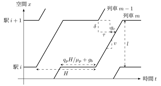
(a) 自由流状態 ( v = v_f , g_c > 0 )
