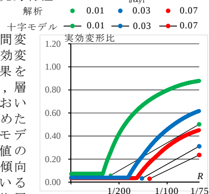
図 5 層間変形角 R と実効変形比の関係
