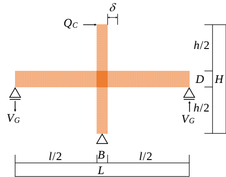
図 1 柱梁接合部の十字モデル概要
