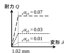
図 4 せん断パネルの復元力特性
