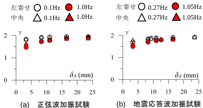
図 3 ダンパー設置位置の違いによる実効変形比の比較
