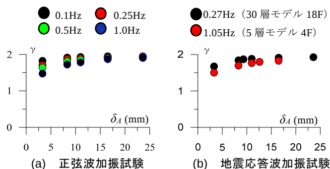
図 1 左寄せフレーム加振試験の実効変形比
