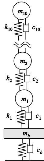
図2 免震を有する11自由度系のモデル
