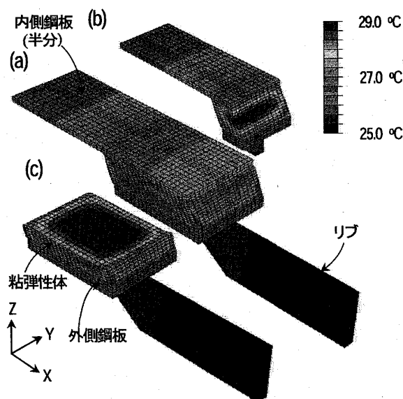
図5 3次元有限要素解析より得られた3000秒での温度分布
