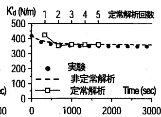
図4 貯蔵剛性の比較
