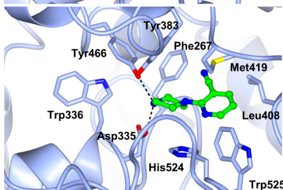
Figure 2-8 化合物 11 から 14 の複合体結晶構造
