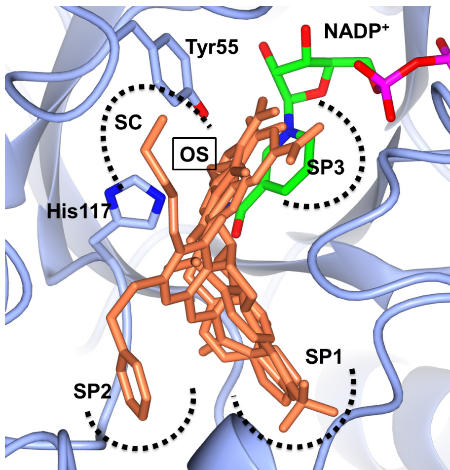
Figure 4-2 化合物 27 から 30 と 17β-HSD5、NADP + の 3 者複合体の重ね合わせ 橙のスティックモデルが化合物を、緑のスティックモデルが NADP + を示す。オキシア ニオンサイト (OS) の位置を文字で示す。サブポケット 1 から 3 (SP1 から 3)、ステロ イドチャネル (SC) の位置を点線で示す。
