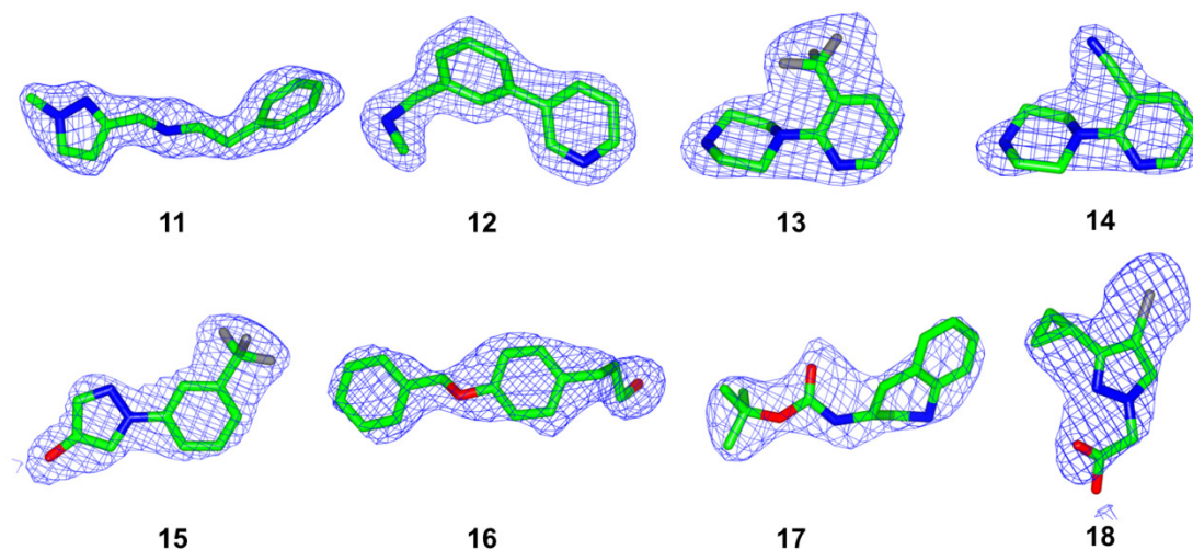
Figure 2-7 フラグメント化合物の F_o - F_c オミット電子密度マップ (2.5 \sigma )
