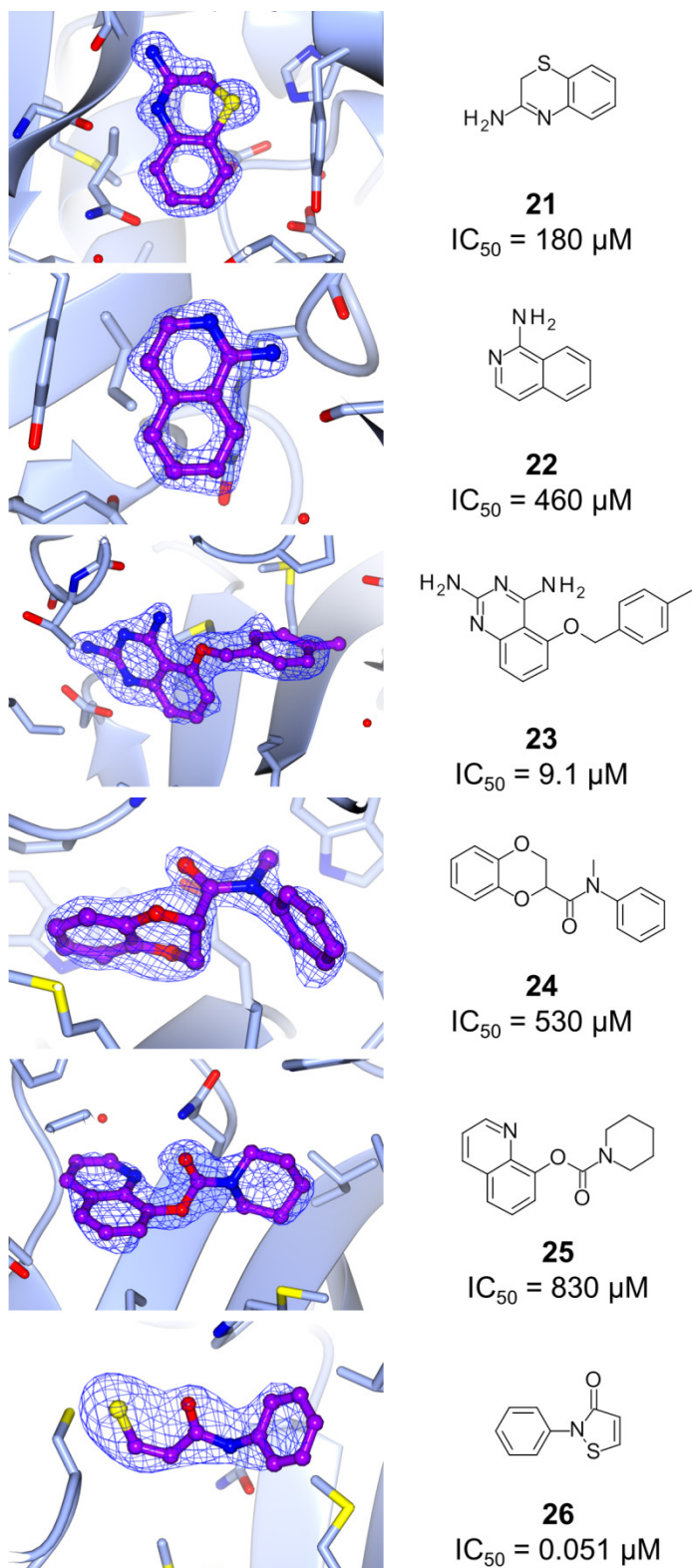
Figure 3-4 化合物 21 から 26 の F_o - F_c オミット電子密度マップ ( 2.5 \sigma ) および構造式 化合物は紫のボール&スティックモデル、タンパク質は水色のリボン図とスティックモデルで示す。阻害活性評価における IC_{50} 値を併せて表示した。
