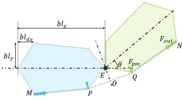
図 4 関節が曲がった時に外側にある人工筋肉の経路と力の関係を表したモデル図
