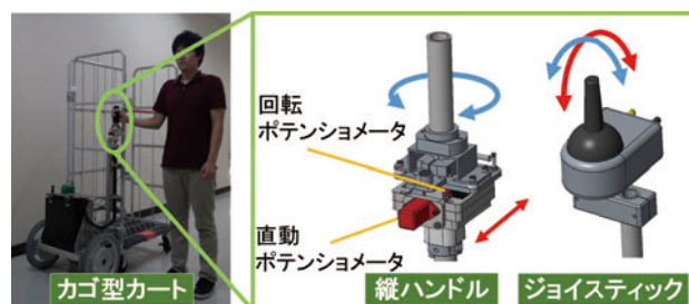
図3: 縦ハンドル/ジョイスティック式インターフェース
