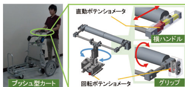
図2: 横ハンドル/グリップ式インターフェース
