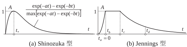
図4 地動の振幅包絡関数
