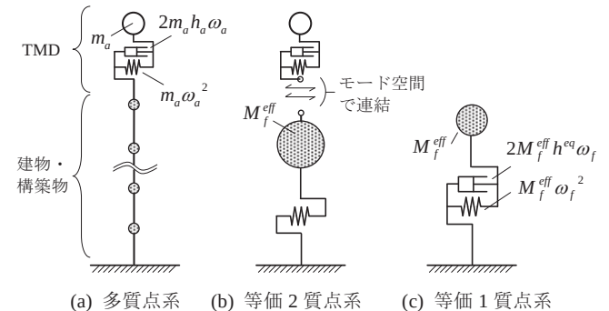
図 1 建物と TMD から構成される全体系のモデル化
