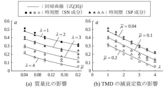
図 12 TMD の最大変形と応答スペクトル特性の関係
