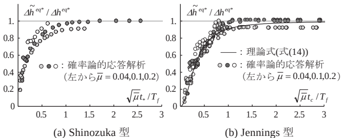
図5 等価付加減衰定数の推定
