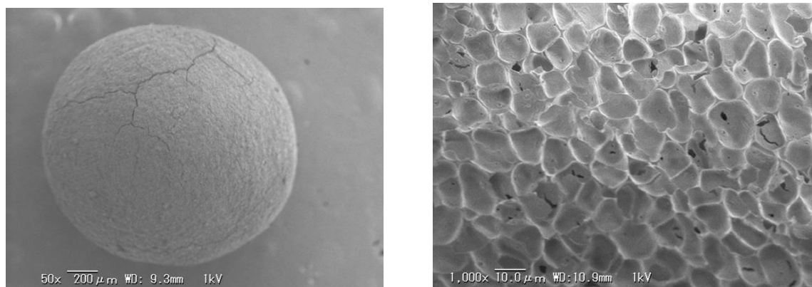
Fig. 5-1 A. オートクレーブ処理前後の FT-IR による化学構造の比較； B. SEM によるオートクレーブ処理後の構造観察
