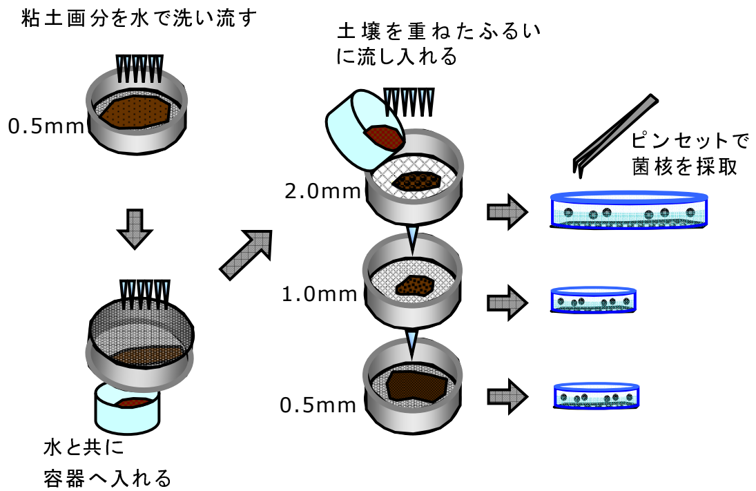
Fig. 2-4 改変 wet sieving 法
