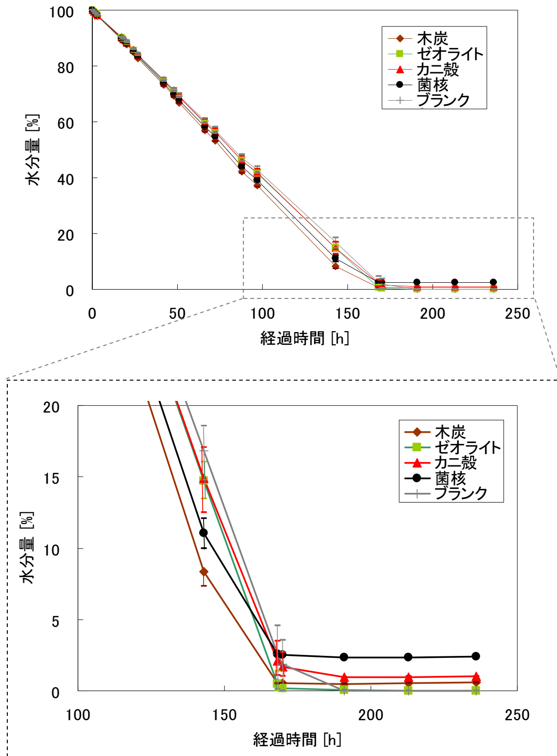
Fig.5-7 微生物担体と菌核の水分量の変化
