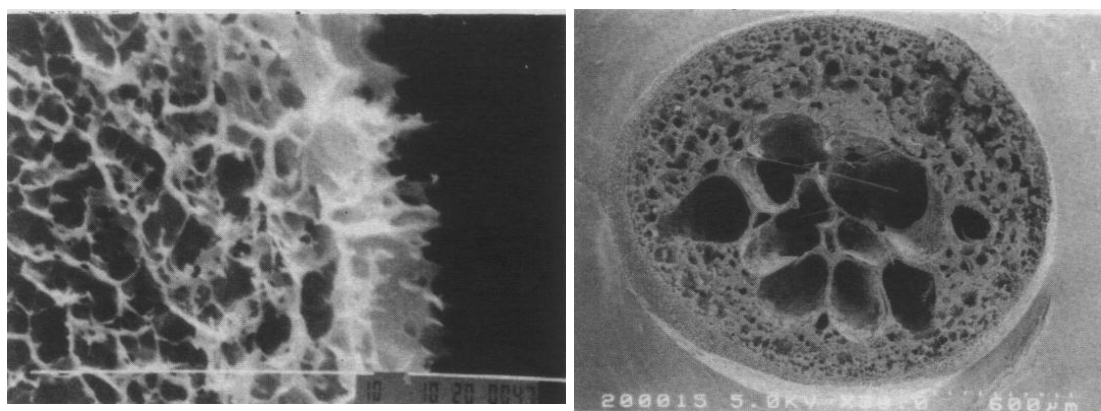
Fig. 6-2 キトサンビーズの SEM 写真
