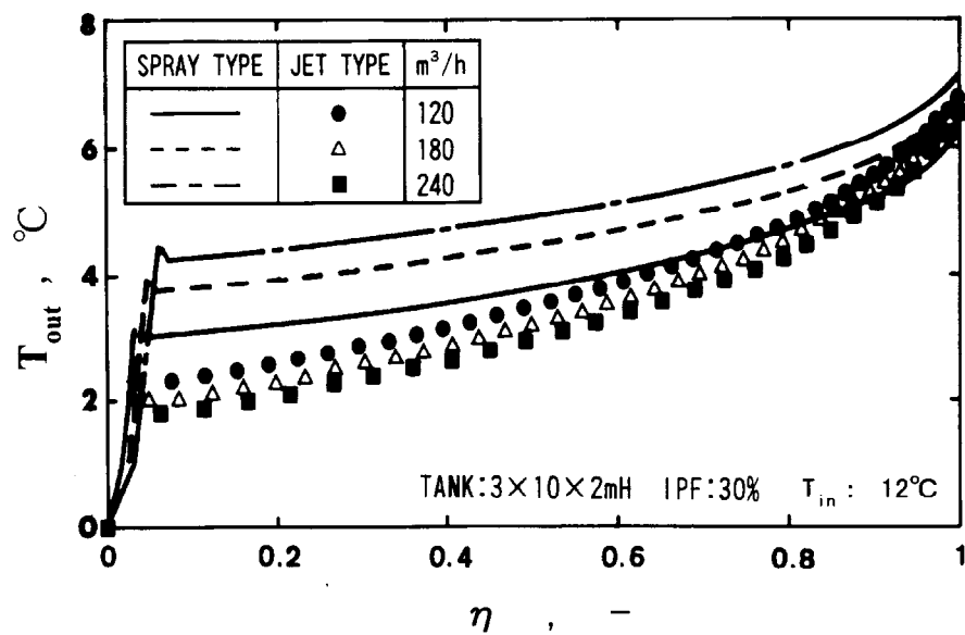
図 4-2-5 伝熱特性による解氷方式の比較
