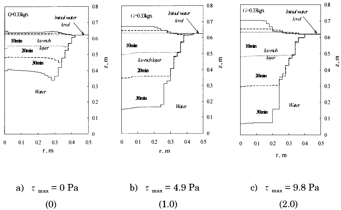
図 3-4-4 セン断応力のしきい値の浮遊氷層形状への感度
