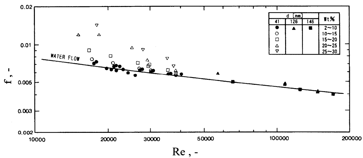
図2-3-8 管内の氷水二相流のRe数と管摩擦係数の関係
