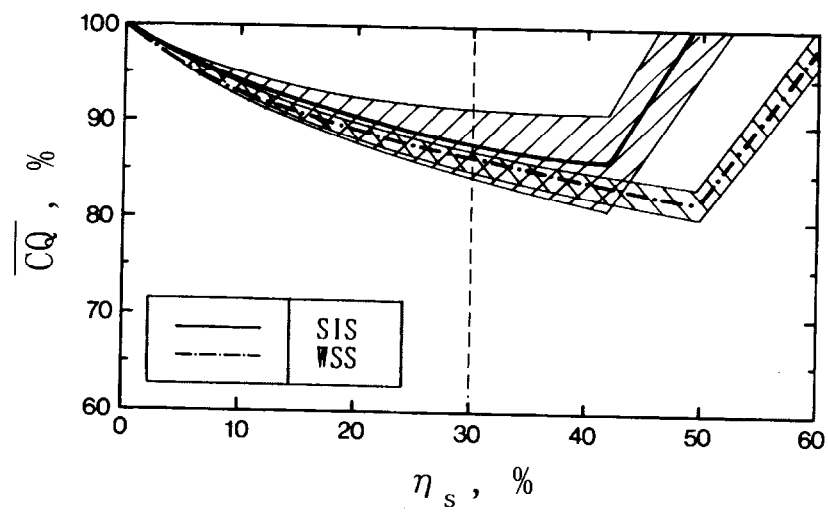
図2-4-5 蓄熱槽からの冷熱で処理する熱負荷の割合 \eta_s と年間経常費の割合 \overline{CQ} の関係
