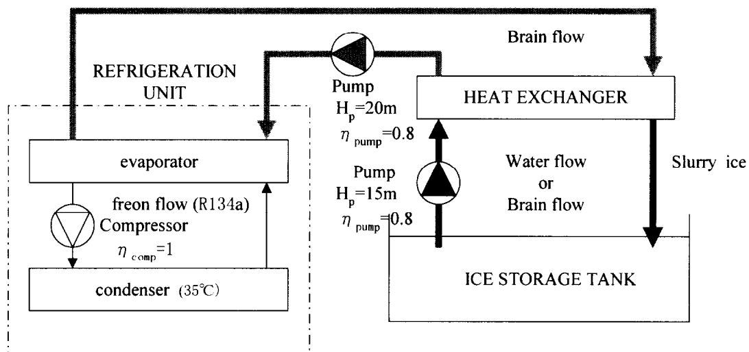
図2-3-1 想定した冷却サイクル
