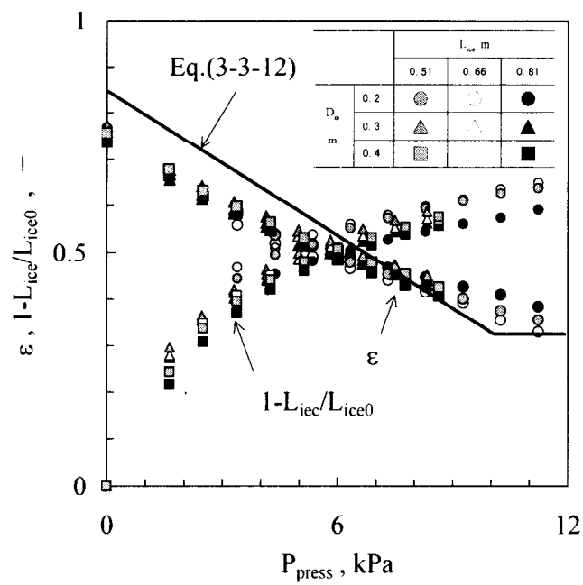
図 3-3-5 氷層の圧密実験の結果 (応力 P_{press} と氷層の空隙率 \epsilon との関係)
