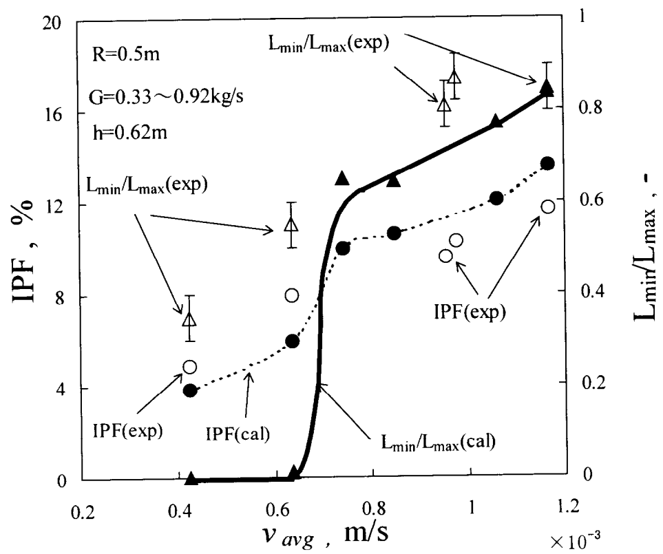
図 3-4-6 円筒氷蓄熱槽における容積の利用効率
