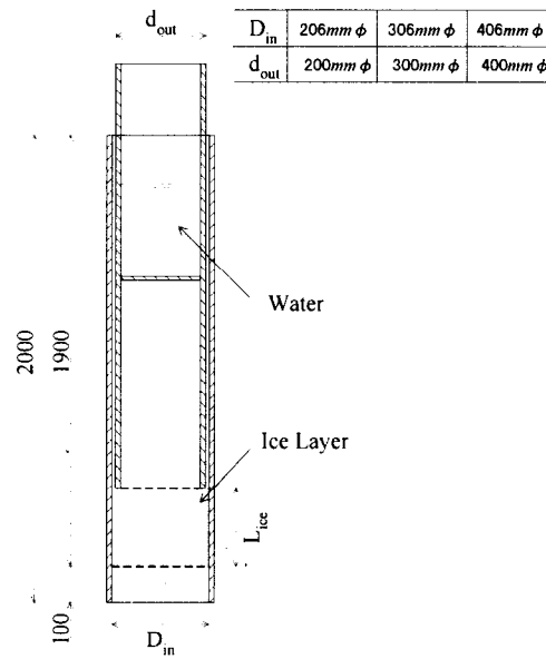
図 3-3-4 氷層の圧密実験に用いた容器
