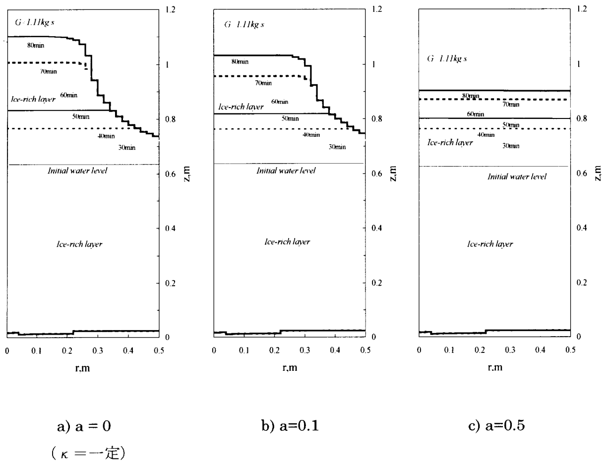
図 3-4-5 空隙率の変化に伴う透過係数 \kappa の変化の堆積氷層形状への感度
