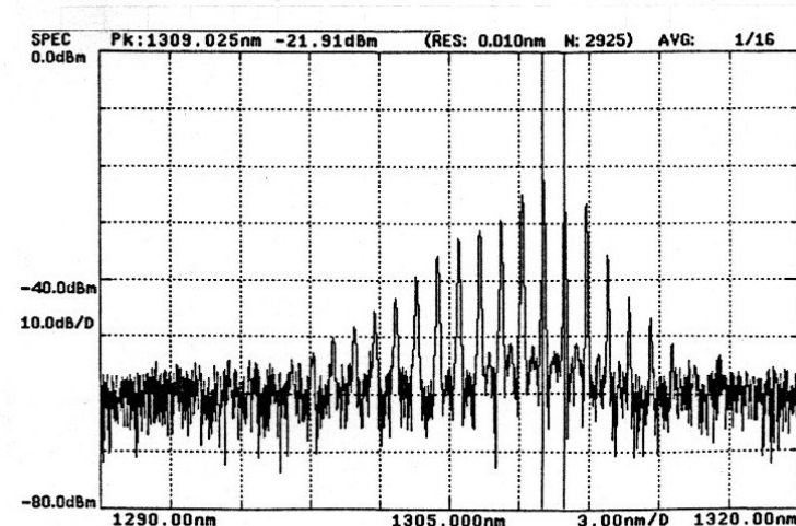
図5-2 1.3 \mu m帯FP-LDの光信号のスペクトル分布
