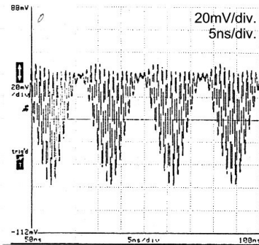
図6-7 LDに入力する単極性AM信号の振幅を変化させたときの光スペクトル分布と入力信号の時間波形(Ⅱ)
