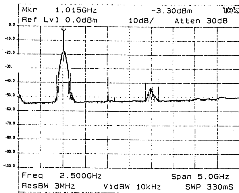
(b) ASK信号のスペクトル分布
