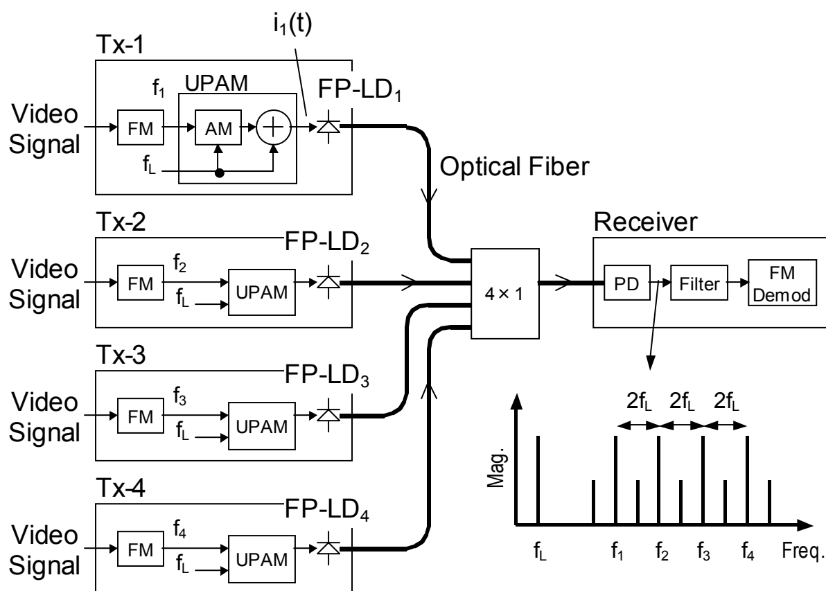
図5-1 SCMアクセスネットワークの構成
