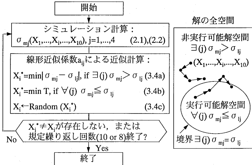
図 3.2: 強制操作アルゴリズム
