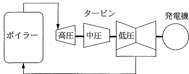
図 2.1: 発電プラントの基本構成
