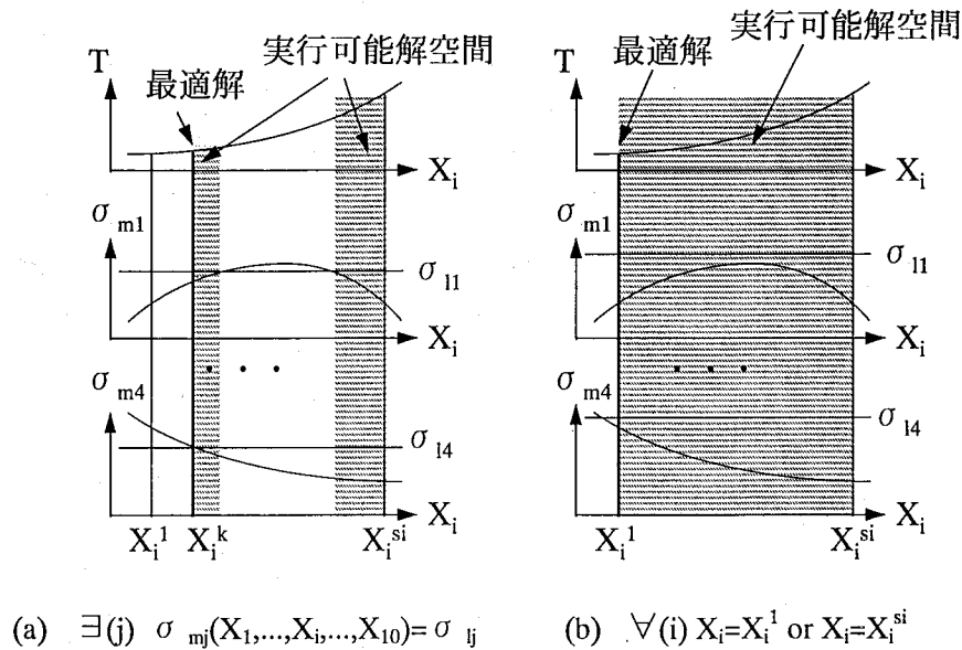
図 3.1: 実行可能解空間の境界上に最適解の存在例
