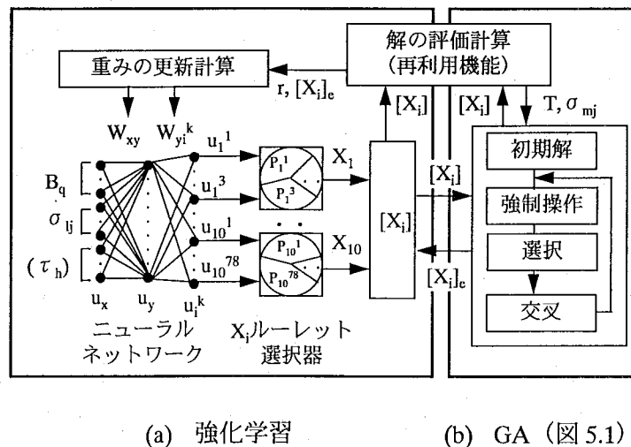
図 5.2: GA と強化学習の融合モデル
