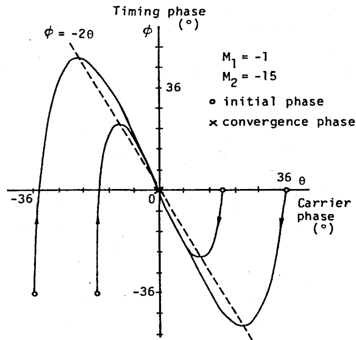
図 3-7 位相平面上の制御軌跡
