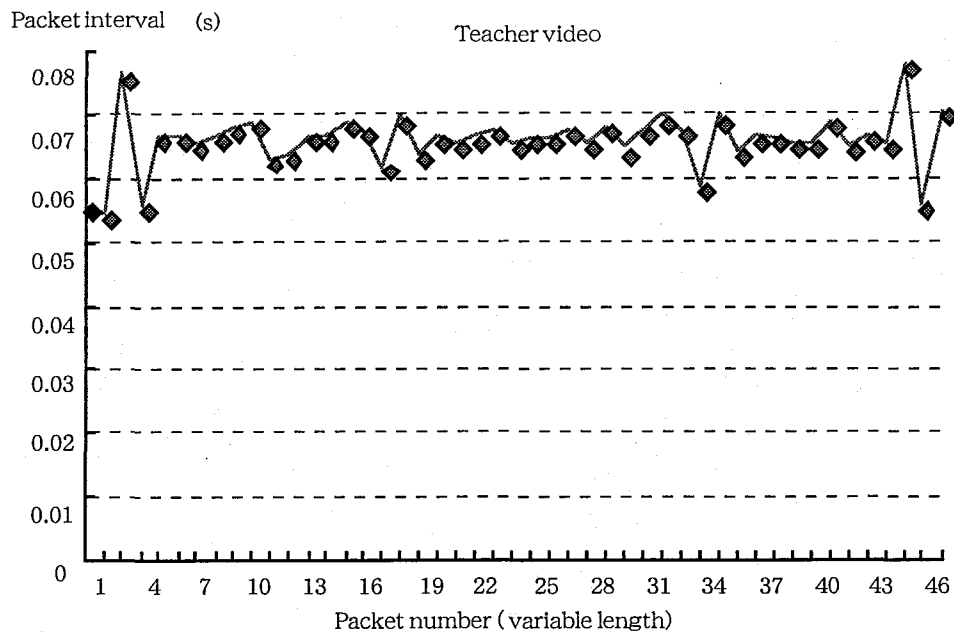
図 4-25 講師映像のパケット転送間隔
