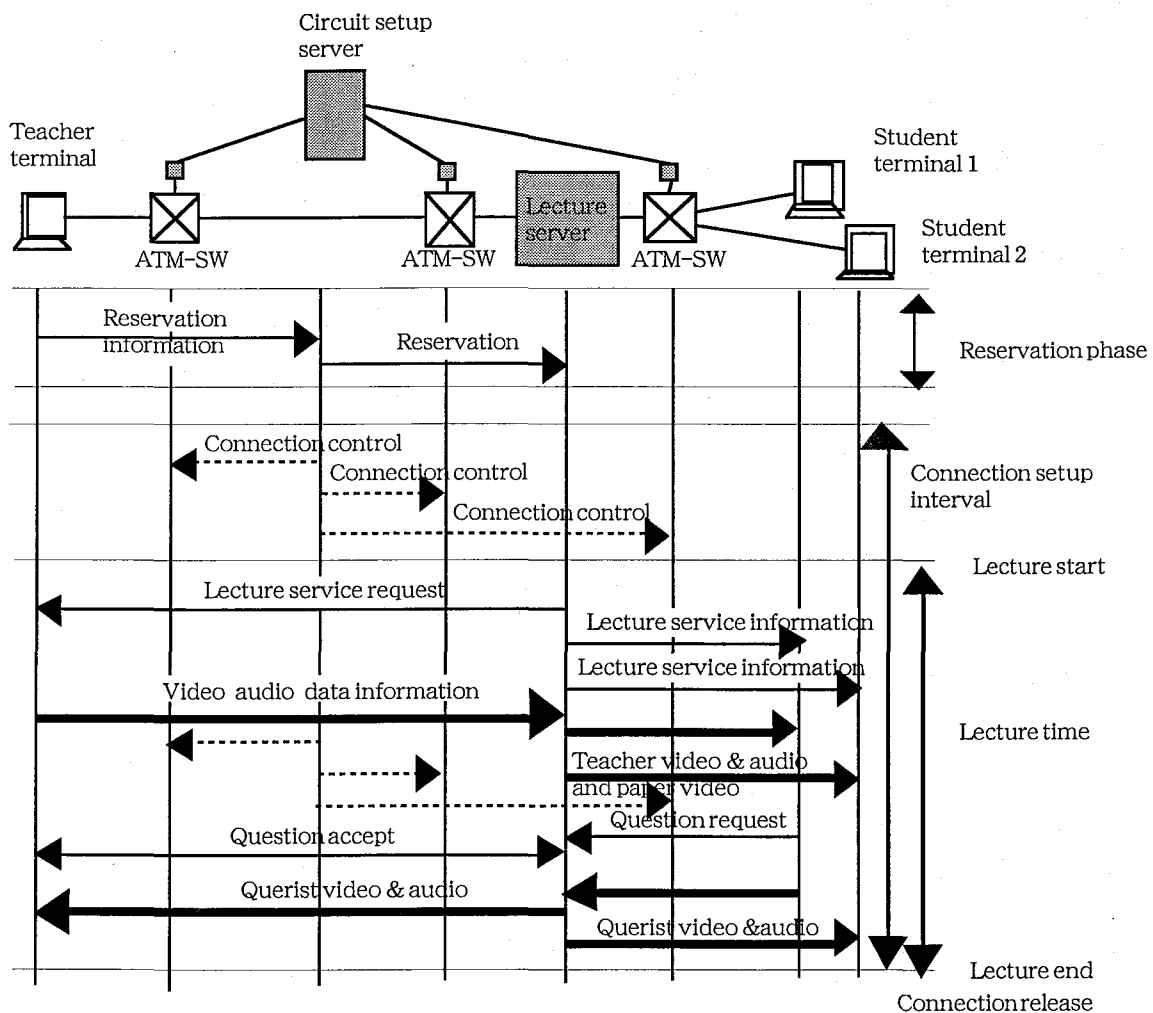
図4-19 遠隔講義サービスの動作シーケンス
