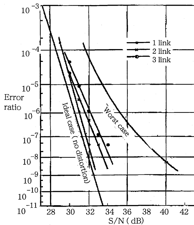
図 3-16 S/Nに対する誤り率特性
