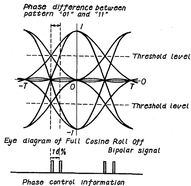
図2-2 2乗余弦波形のアイパターン
