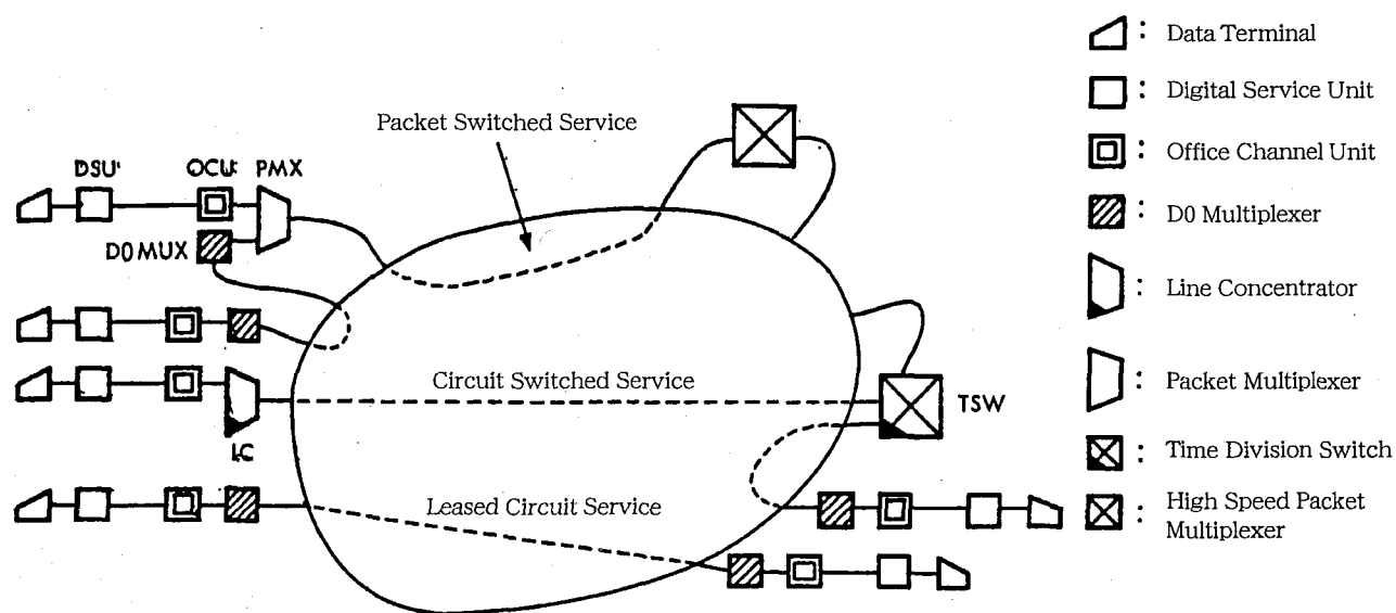
図2-1 デジタルデータ網の加入者線伝送方式の構成図
