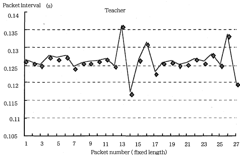
図 4-26 講師音声のパケット転送間隔
