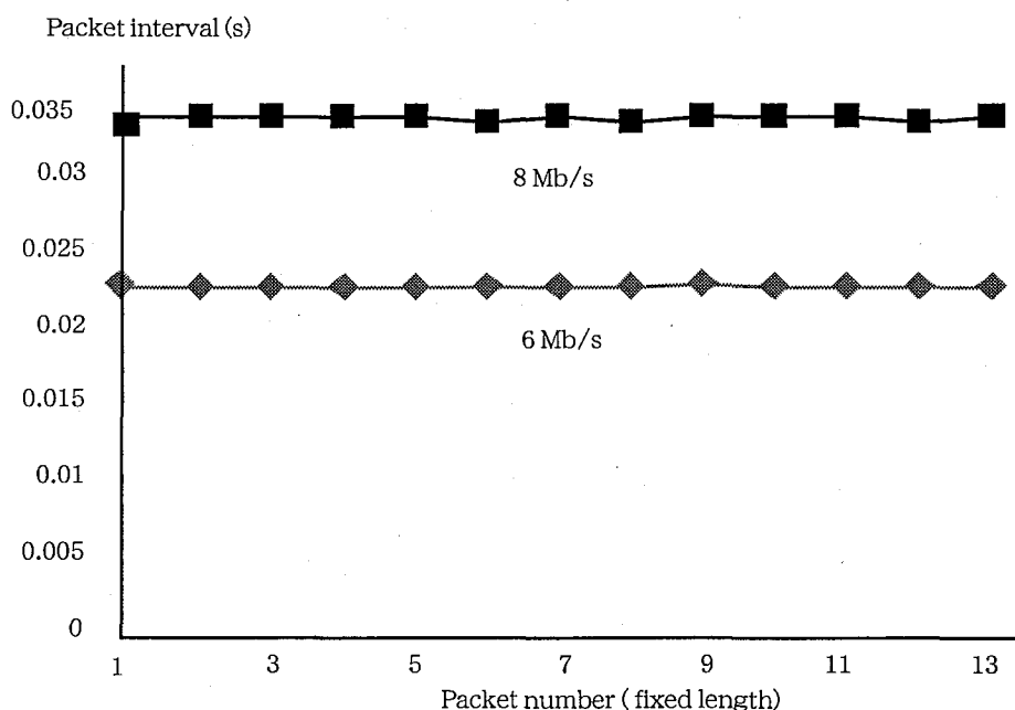
図 4－29 MPEG2 CODECの映像信号パケット転送間隔
