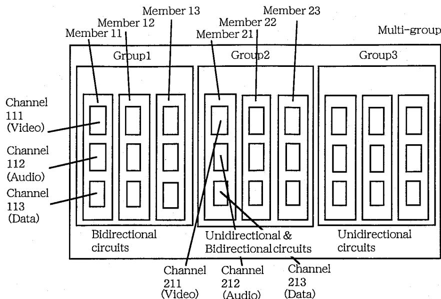
図 4 - 6 マルチグループ通信のチャネル構成例
