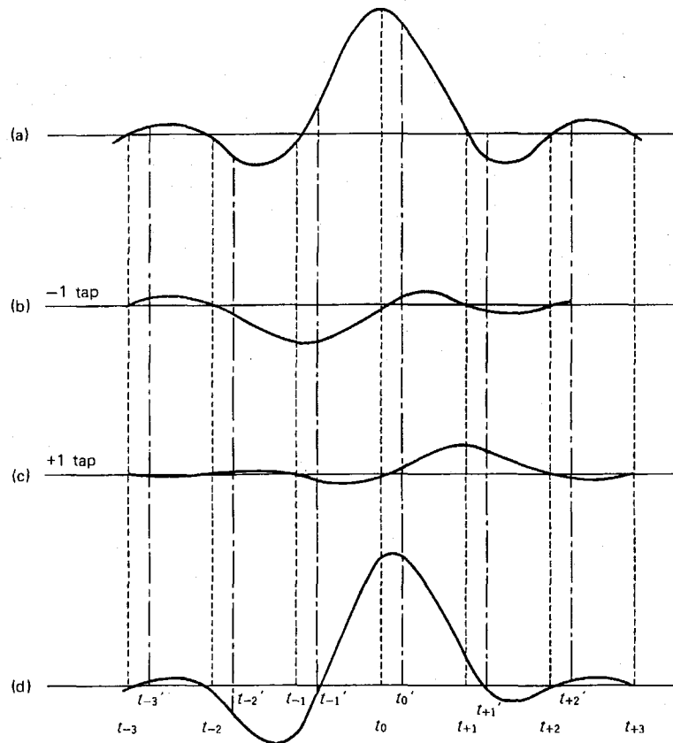
図 3-4 タイミング自動位相制御の原理
