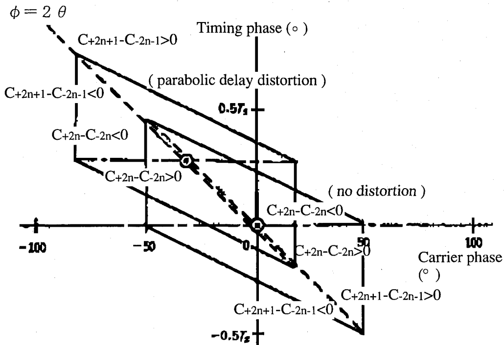
図 3-14 位相制御情報と自動等化器の引き込み範囲
