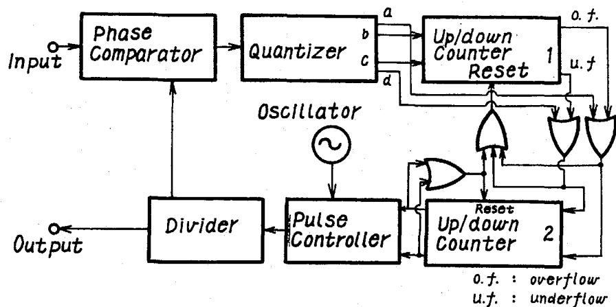
図 2 - 4 カウンタ段数切替型DPLLの構成
