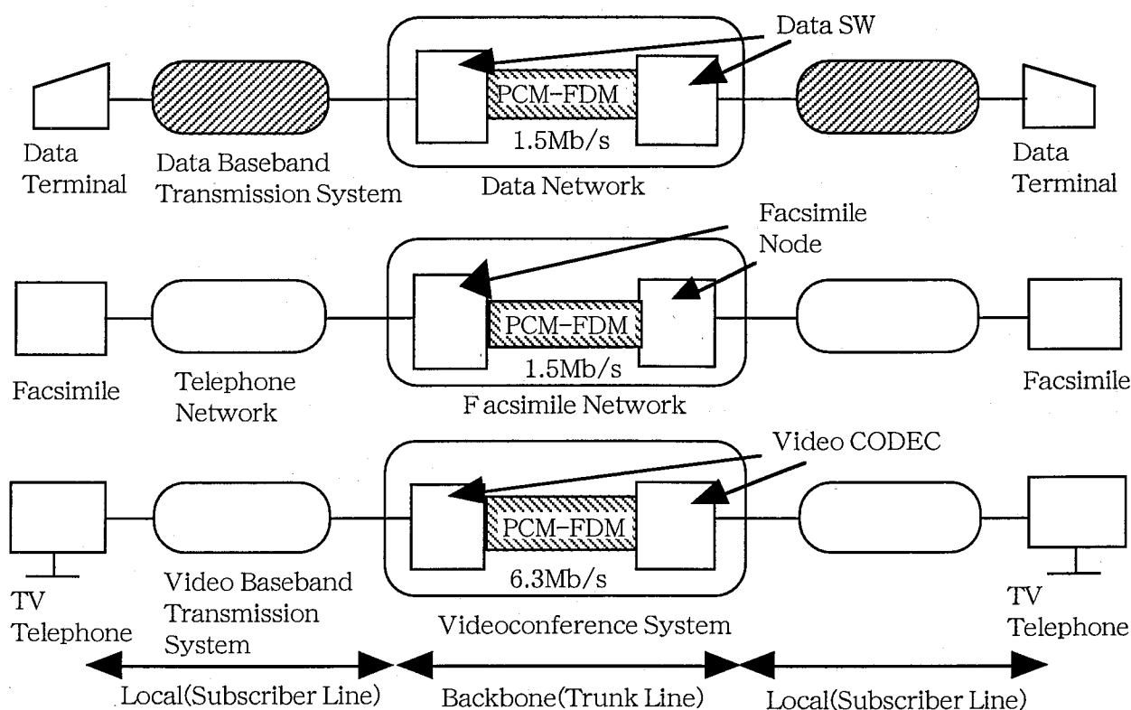
図1-1 各種サービスの加入者線伝送方式と基幹伝送系のPCM-FDM方式
