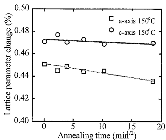
Fig.4.1-a x 軸は保持時間 Fig.4.1-b x 軸は保持時間の 1/2 乗 Fig.4.1 B 4 C 添加 SiC の 150°C 等温アニールにおける格子定数の変化
