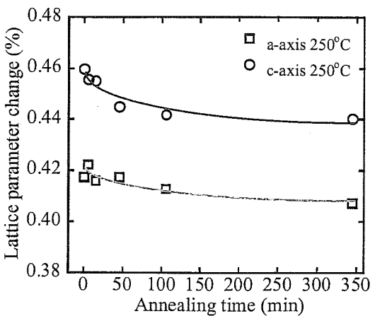
Fig.4.3-a x 軸は保持時間 Fig.4.3-b x 軸は保持時間の 1/2 乗 Fig.4.3 B 4 C 添加 SiC の 250°C 等温アニールにおける格子定数の変化
