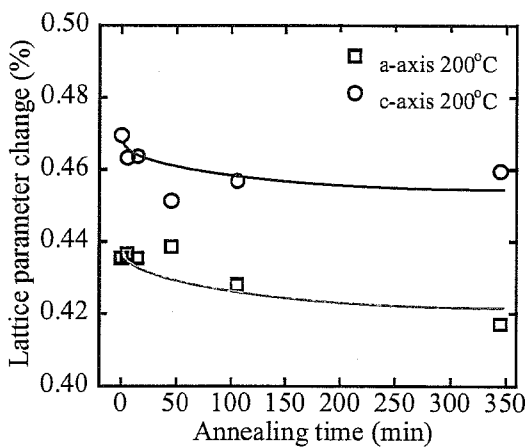
Fig.4.2-a x 軸は保持時間 Fig.4.2-b x 軸は保持時間の 1/2 乗 Fig.4.2 B 4 C 添加 SiC の 200°C 等温アニールにおける格子定数の変化
