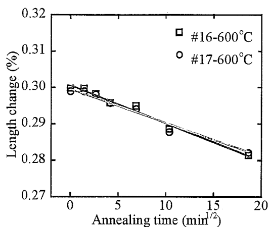
Fig.2.36-b x 軸は保持時間の 1/2 乗
