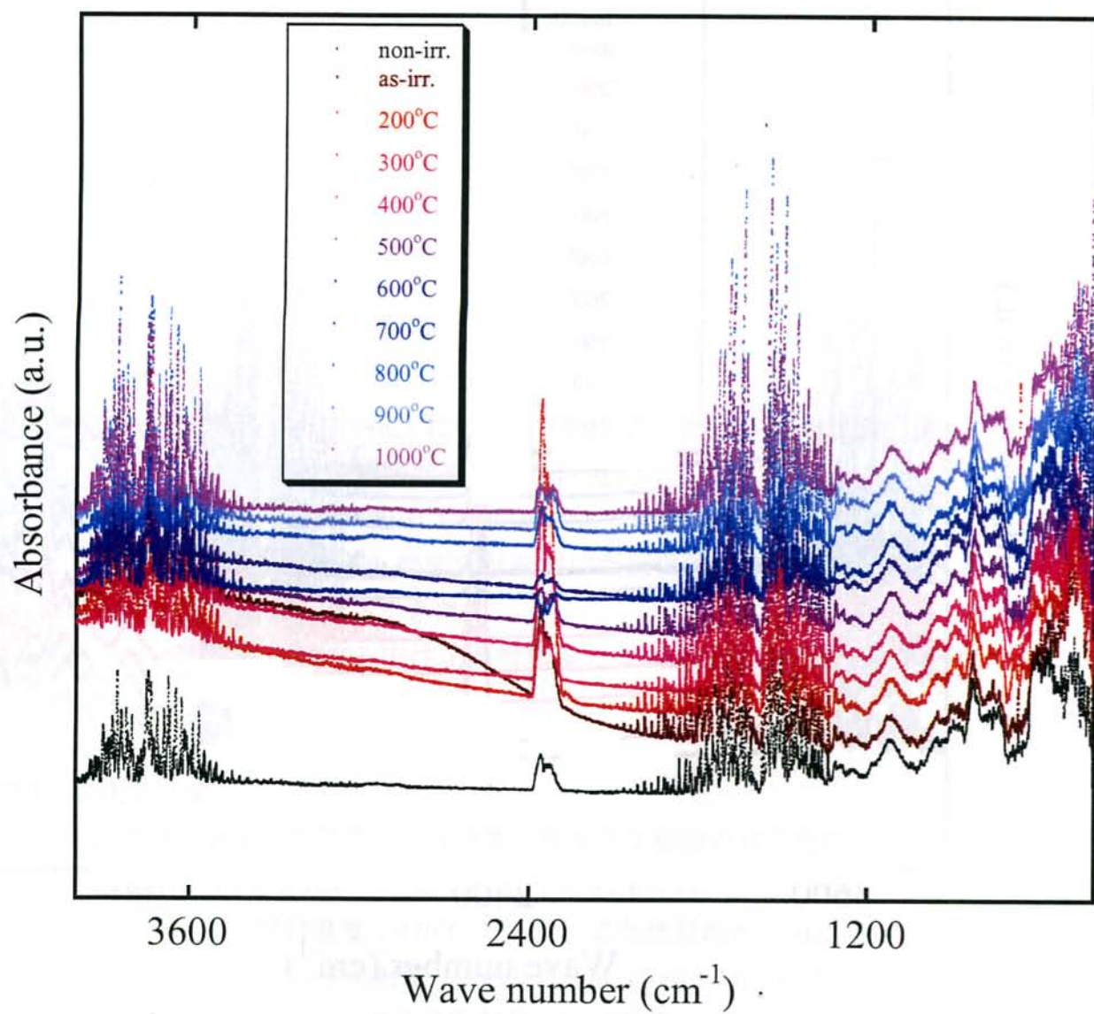
Fig6.5-1 中性子照射 Si (照射量 : 3.0 \times 10^{23} n/m 2 、照射温度 : 120~150°C) の測定範囲全域 (400-4000 cm -1 ) における赤外吸収スペクトル。温度はアニール温度を示す。
