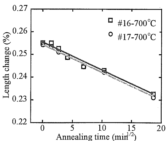
Fig.2.38-b x 軸は保持時間の 1/2 乗
