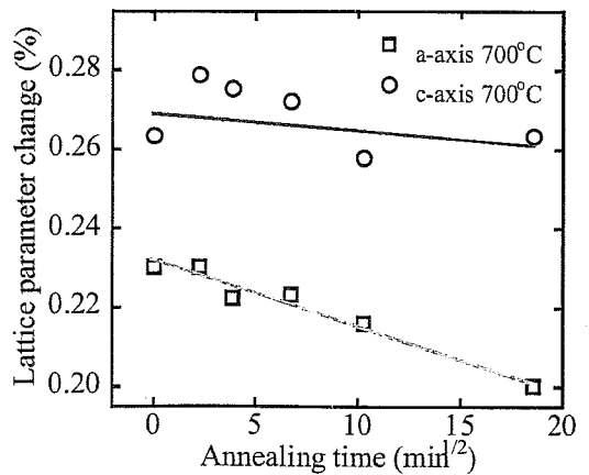
Fig.4.12-b x 軸は保持時間の 1/2 乗
