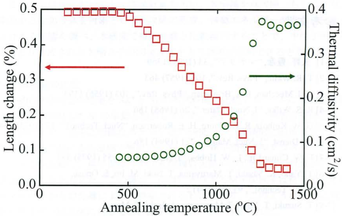
Fig.7.1 \text{Al}_2\text{O}_3 添加 SiC において、熱膨張計を用いて測定した巨視的寸法変化と、熱拡散率の変化を同時にプロットした 6 時間等時アニールによる回復挙動
