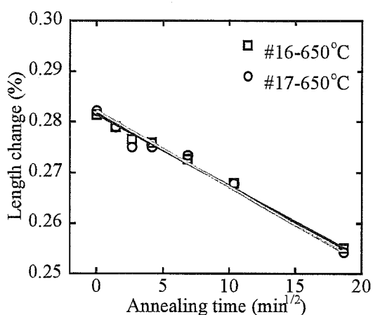
Fig.2.37-b x 軸は保持時間の 1/2 乗
