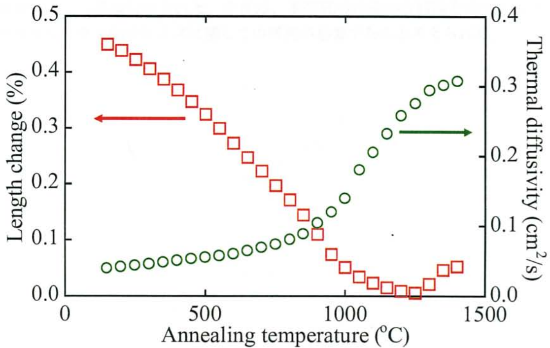
Fig.7.2 \text{B}_4\text{C} 添加 SiC において、熱膨張計を用いて測定した巨視的寸法変化と、熱拡散率の変化を同時にプロットした 6 時間等時アニールによる回復挙動
