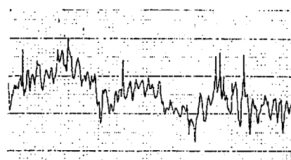
図26 研削粒子の粒度の違いによる摩耗促進試験前後の断面(P1)曲線
