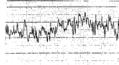
図25 研削粒子の粒度の違いによる摩耗促進試験前後の断面(P1)曲線
