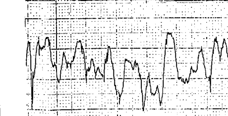
図20 研削粒子の粒度の違いによる摩耗促進試験前後の断面(P1)曲線 <セラミックタイル1>
