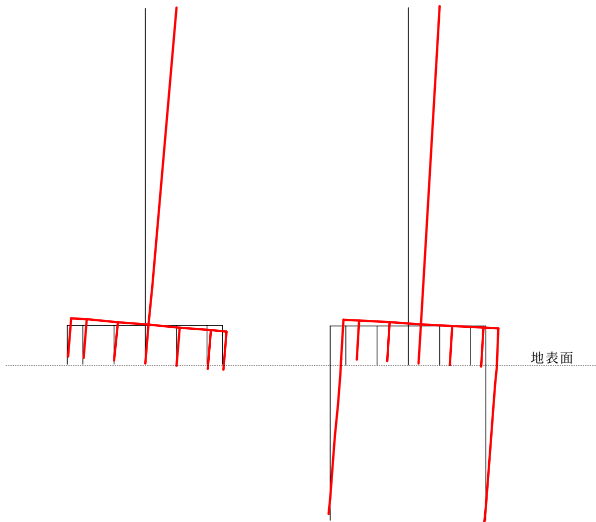
(a) 直接基礎 (HF2L-11) (b) シートパイル基礎 (HS3L-1113) 図-5.7 室内模型の水平載荷実験に対するシミュレーション結果 ( \delta=20\text{mm} 時の変形図)
