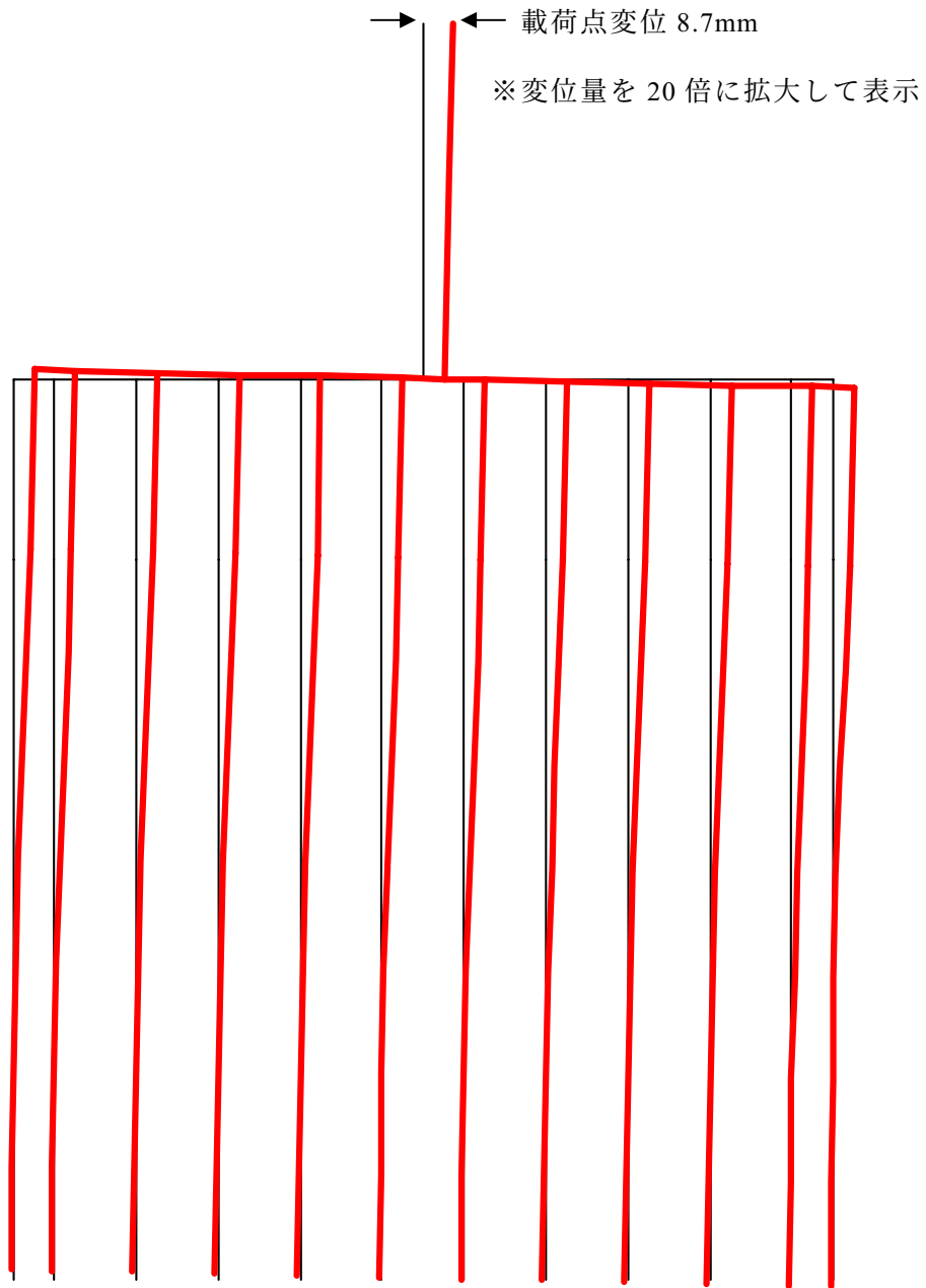
図-6.13 提案モデルによる解析結果（P9 橋脚， P=3600\text{kN} 時，変位図）
