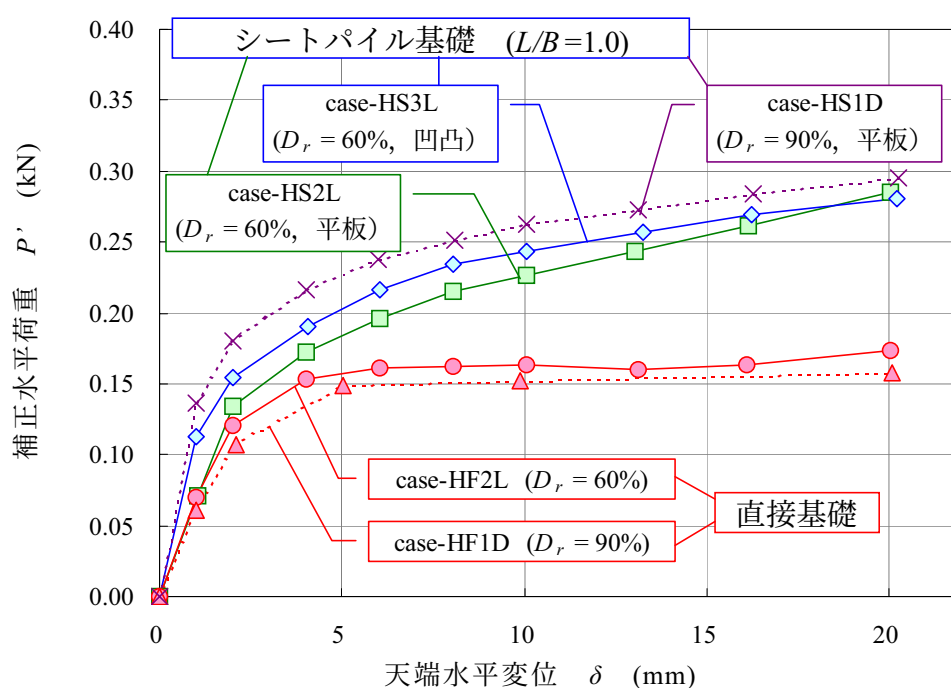
(b) シートパイル剛性および地盤密度の影響比較
