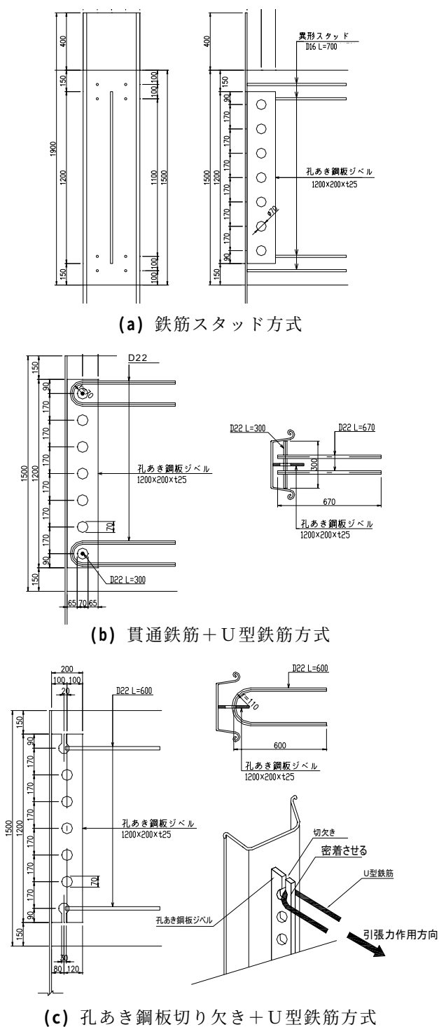
図-4.2 シートパイルとフーチングの接合構造（単位：mm）
