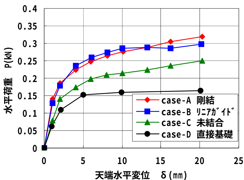
図-A.4 P-\delta 関係（骨格曲線）
