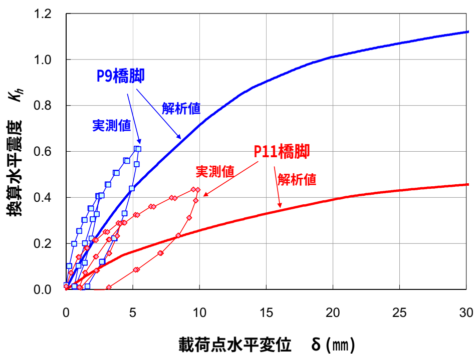
(a) 換算水平震度 K_h ～載荷点水平変位 \delta 関係
