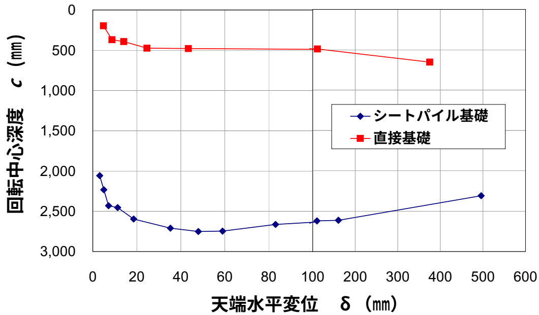
図-4.12 回転中心深度ー天端水平変位関係
