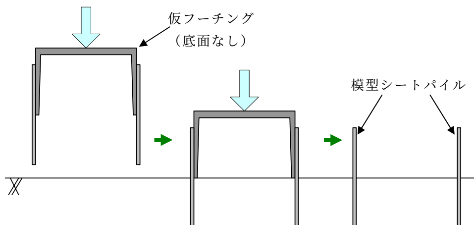
(a) 手順<1> 模型シートパイルの貫入
