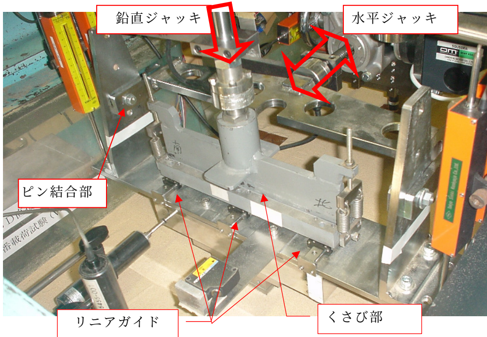
(c) 荷重装置 写真
