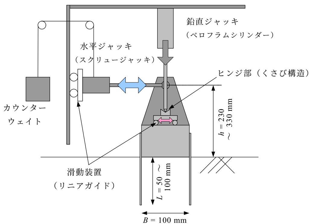
図-3.1 水平載荷実験装置
