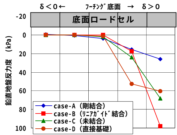
b) 天端水平変位 \delta = 10\text{mm} 時
