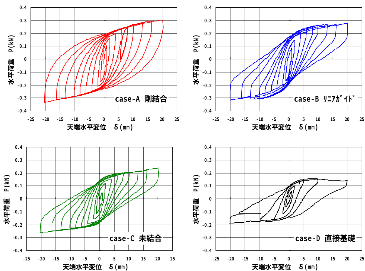
図-A.3 P-\delta 関係（履歴曲線）
