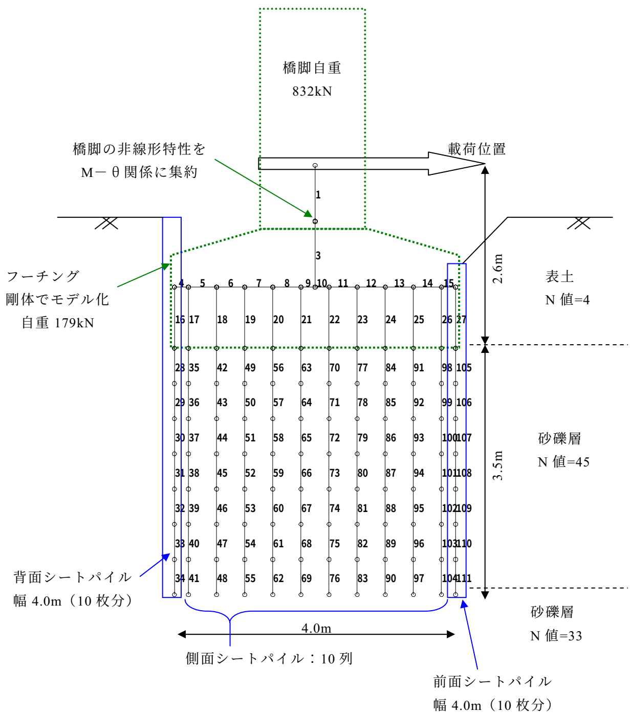
図-6.11 载荷試験シミュレーション用の骨組み解析モデル (P9 橋脚, 要素番号図)
