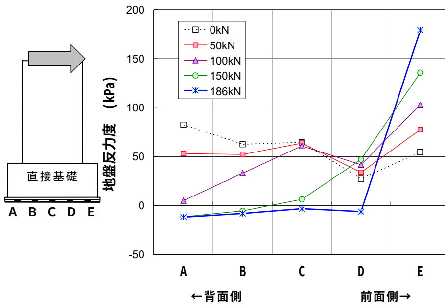
(a) 直接基礎
