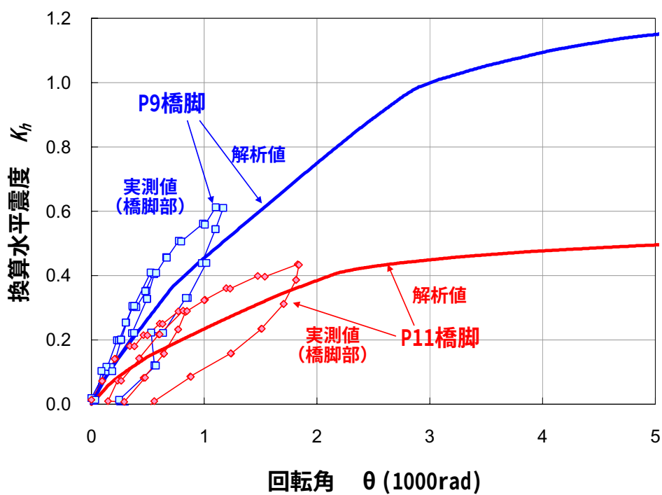
(b) 換算水平震度 K_h ～回転角 \theta 関係
