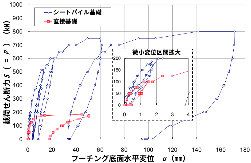
図-4.11 荷重せん断力ーフーチング底面水平変位関係 ( S - u 関係)
