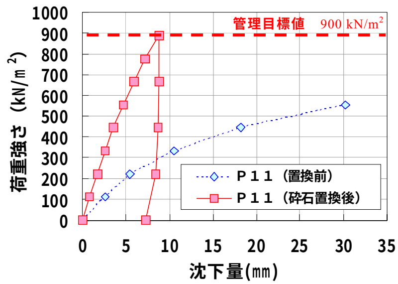
図-6.3 平板載荷試験結果
