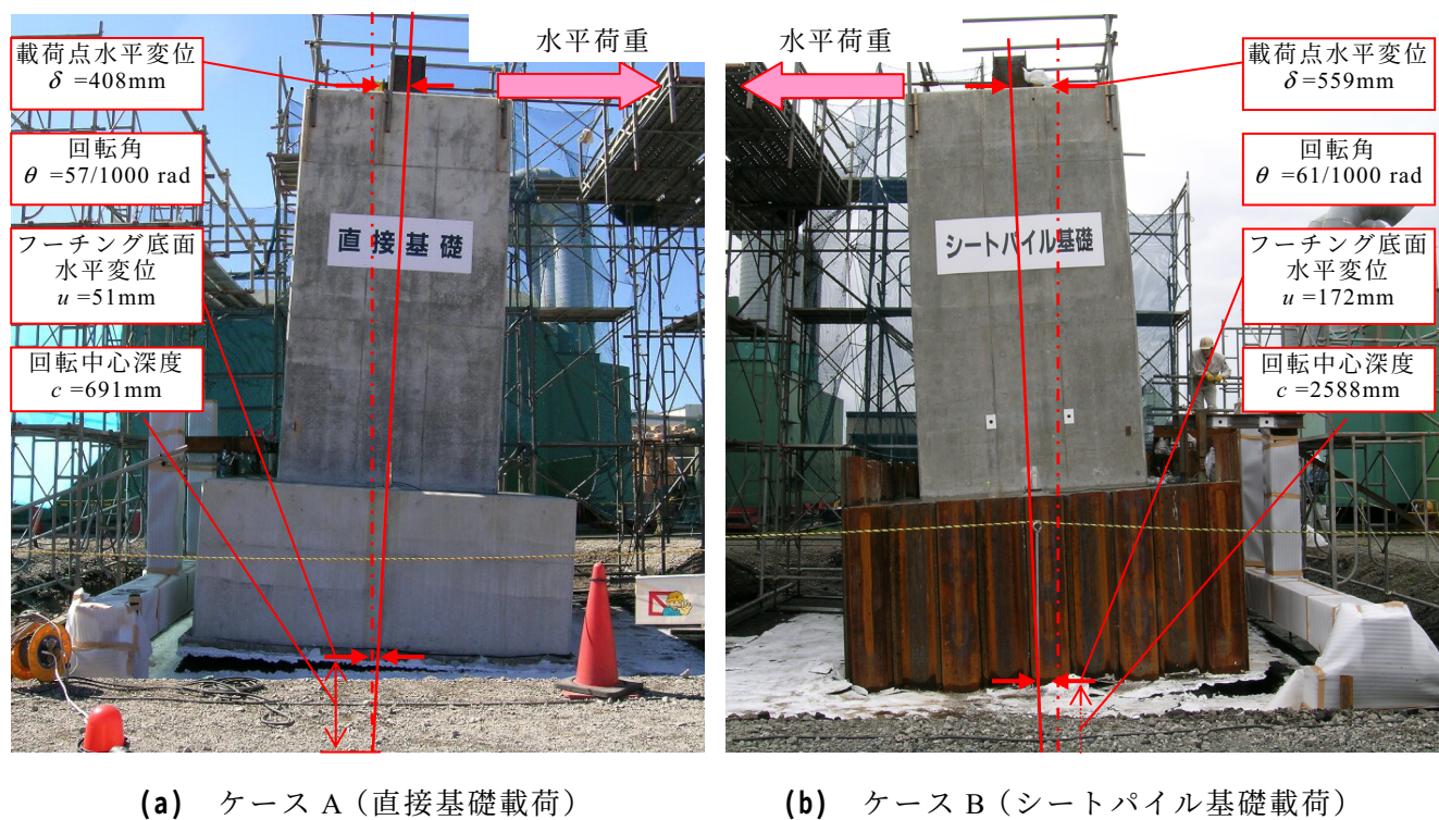
図-4.5 試験体の変形状況 (最大変位時)
