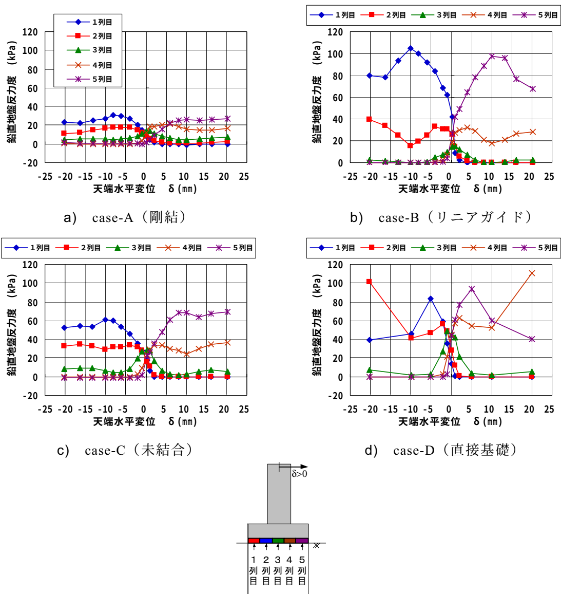
図-A.10 天端水平変位一底面鉛直反力度関係
