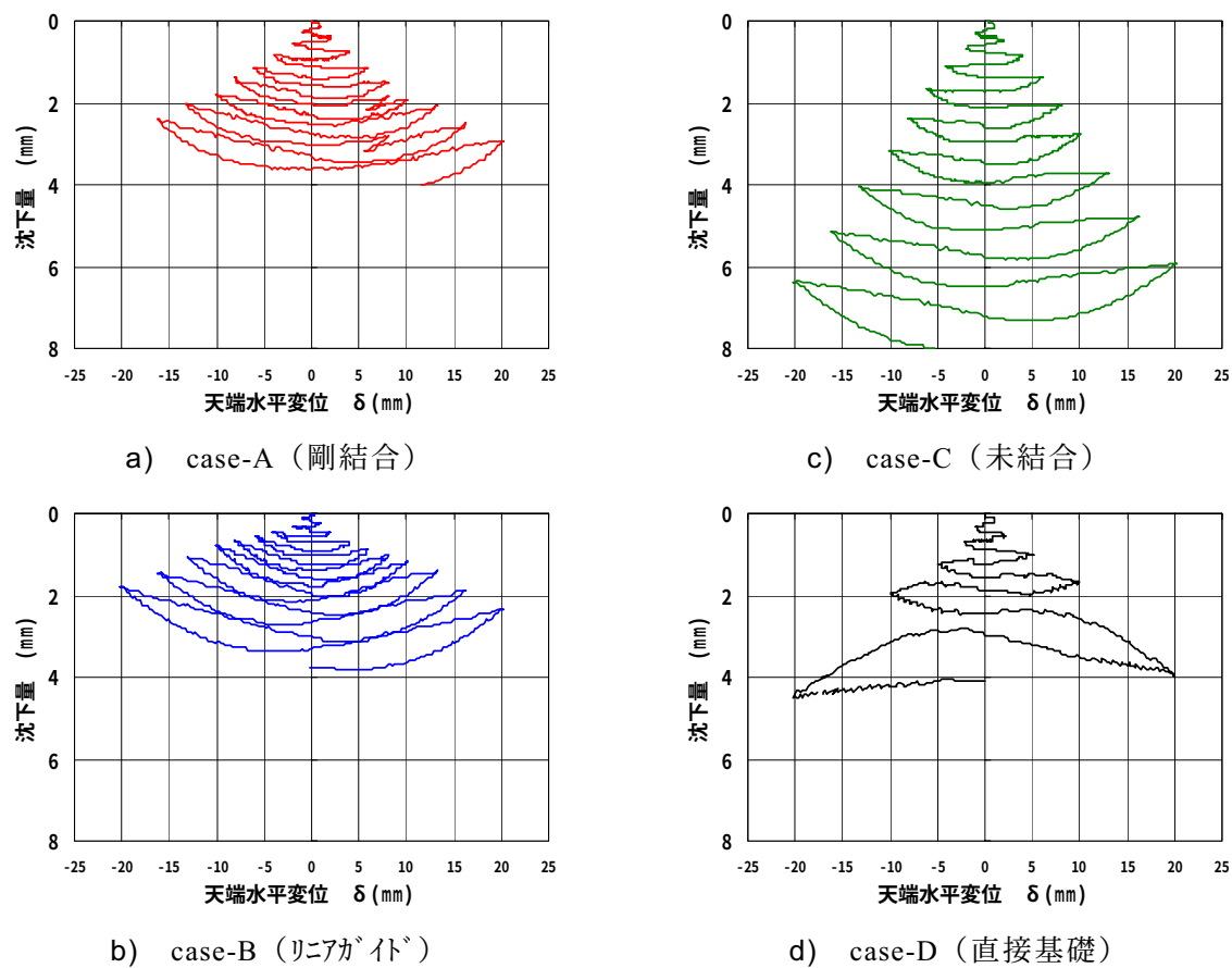
図-A.11 天端水平変位—沈下量関係
