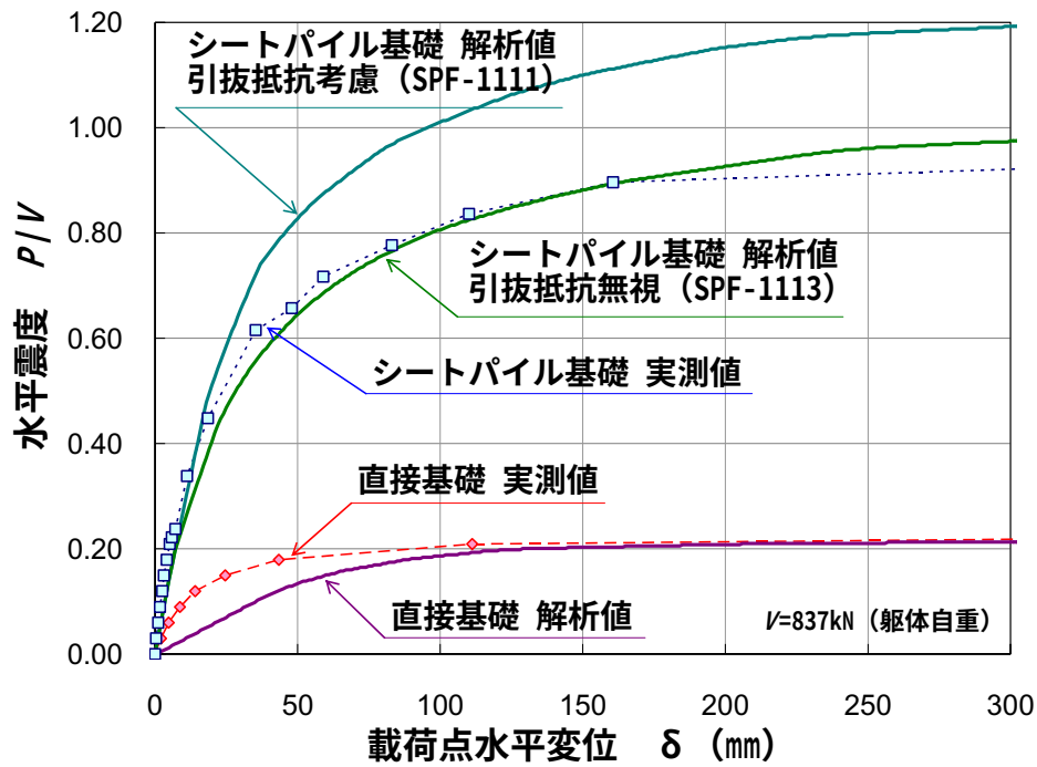
(a) 水平震度～載荷点水平変位関係
