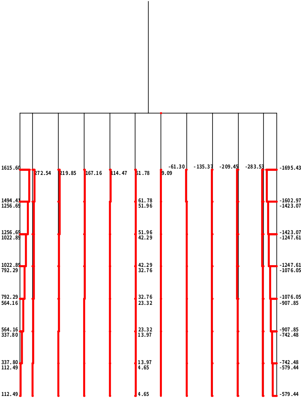
図 -6.14 提案モデルによる解析結果 (P9 橋脚, P=3600kN 時, 軸力図)
