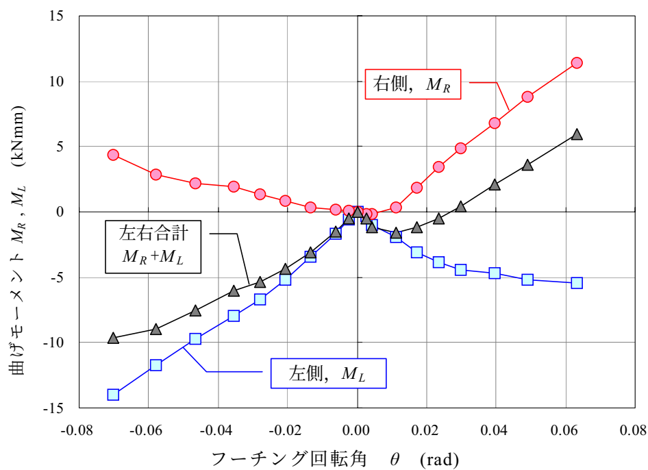
図-3.21 曲げモーメント～水平変位関係 (case-HS3L)
