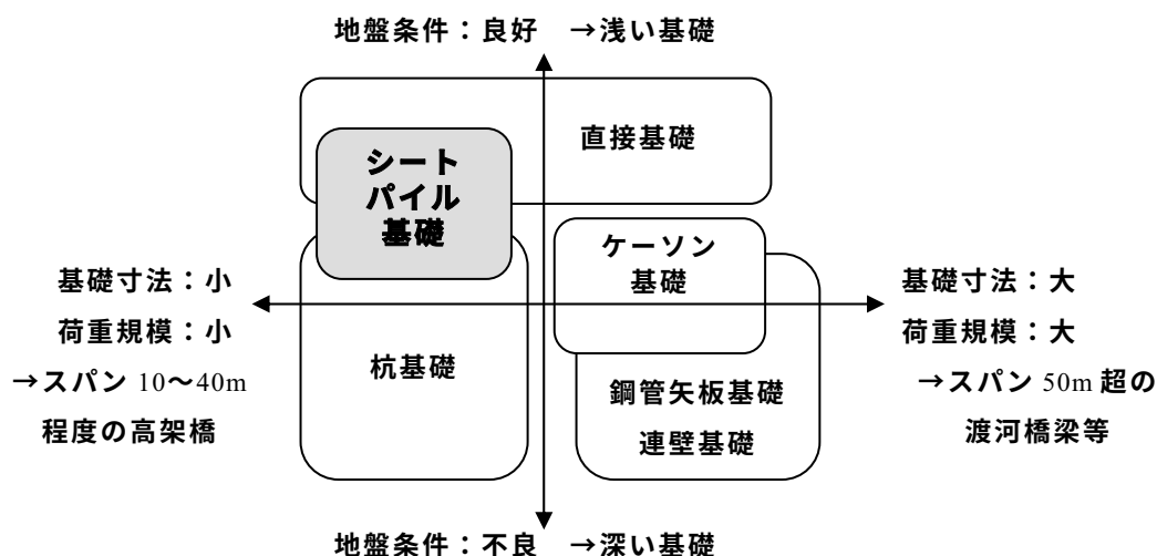
図-1.3 シートパイル基礎と既存基礎形式との適用区分
