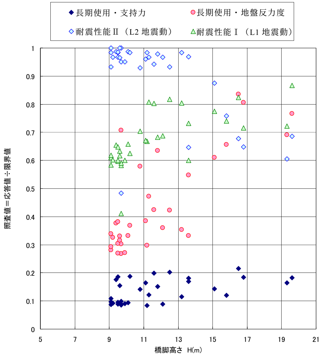
図-5.1 現状の直接基礎設計事例の調査値の傾向
