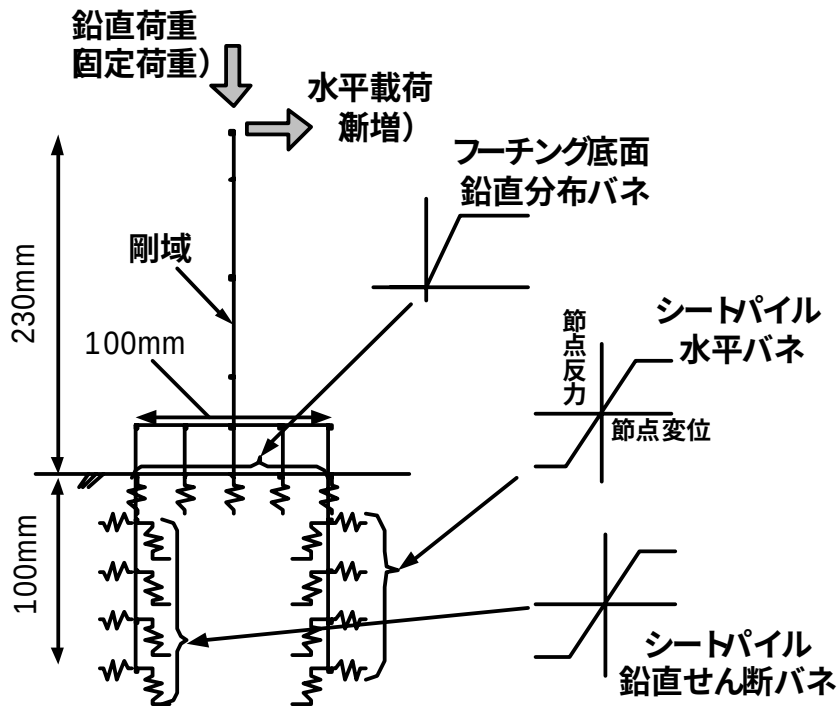
図-5.5 室内模型の水平載荷実験に対するシートパイル基礎の骨組み解析モデル
