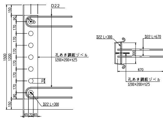
(b) 貫通鉄筋+U型鉄筋方式
