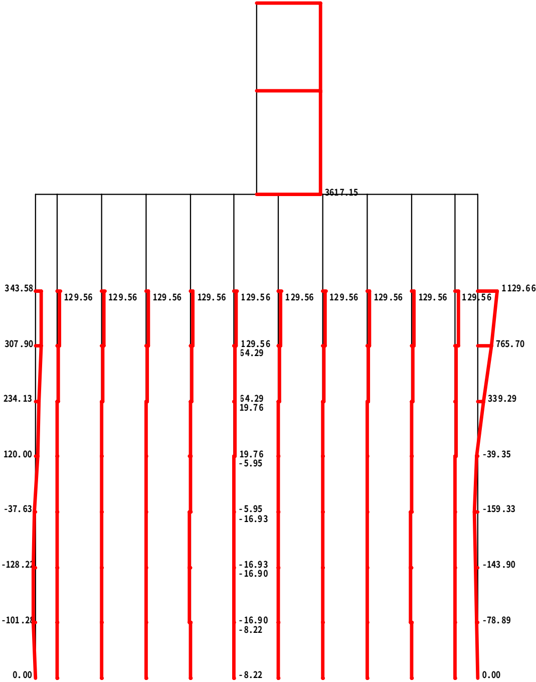
図-6.16 提案モデルによる解析結果（P9 橋脚， P=3600\text{kN} 時，せん断力図）
