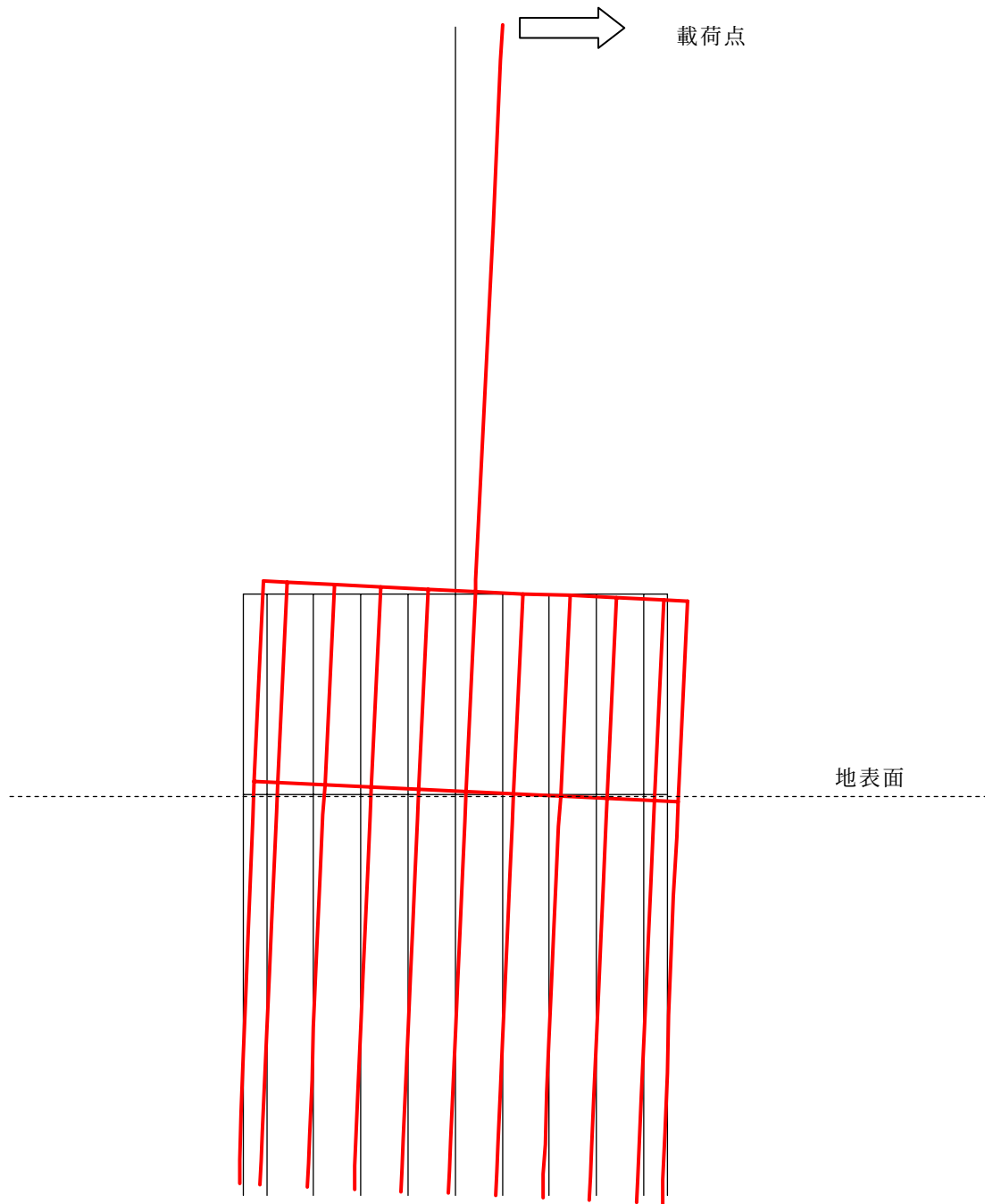
図-5.12 \delta = 500\text{mm} 時の変形図（ケース SPF-1111：引抜き抵抗考慮）
