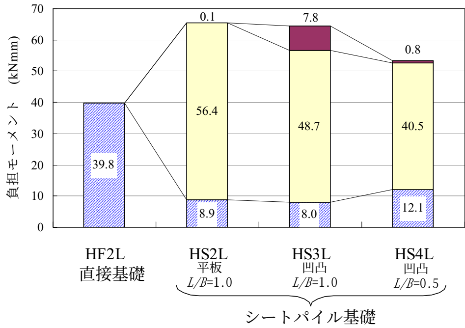
図-3.22 負担比率の比較
