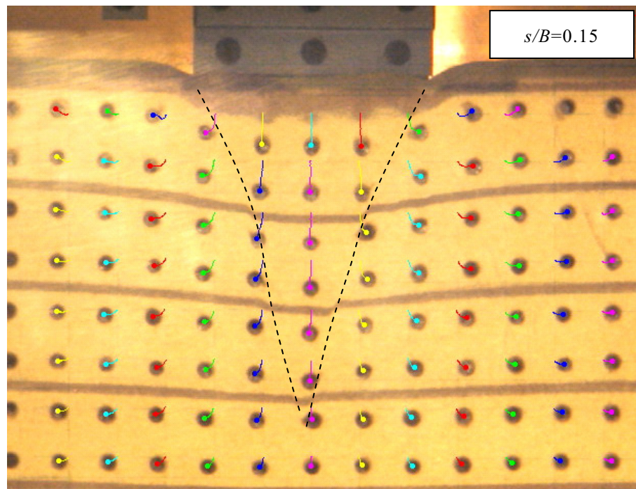
(a) case-VF1 (直接基礎)
