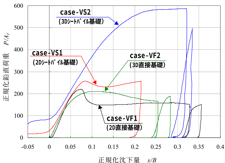
(a) case-VF1,VF2,VS1,VS2 : D_r=90\%
