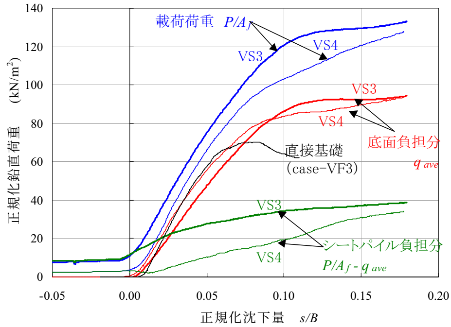
図-2.8 負担箇所別の荷重変位関係
