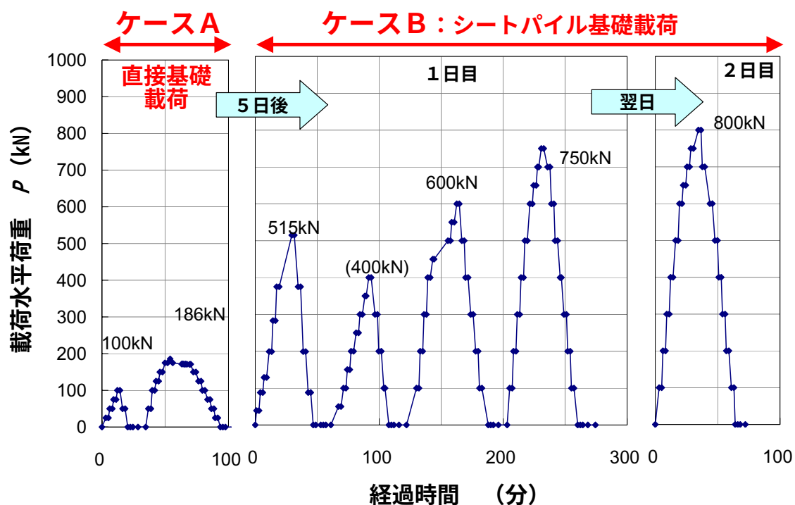
図-4.4 載荷サイクル
