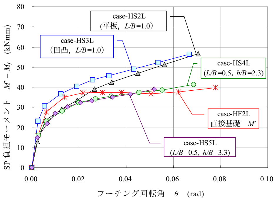
図-3.20 シートパイル負担モーメント～回転角関係
