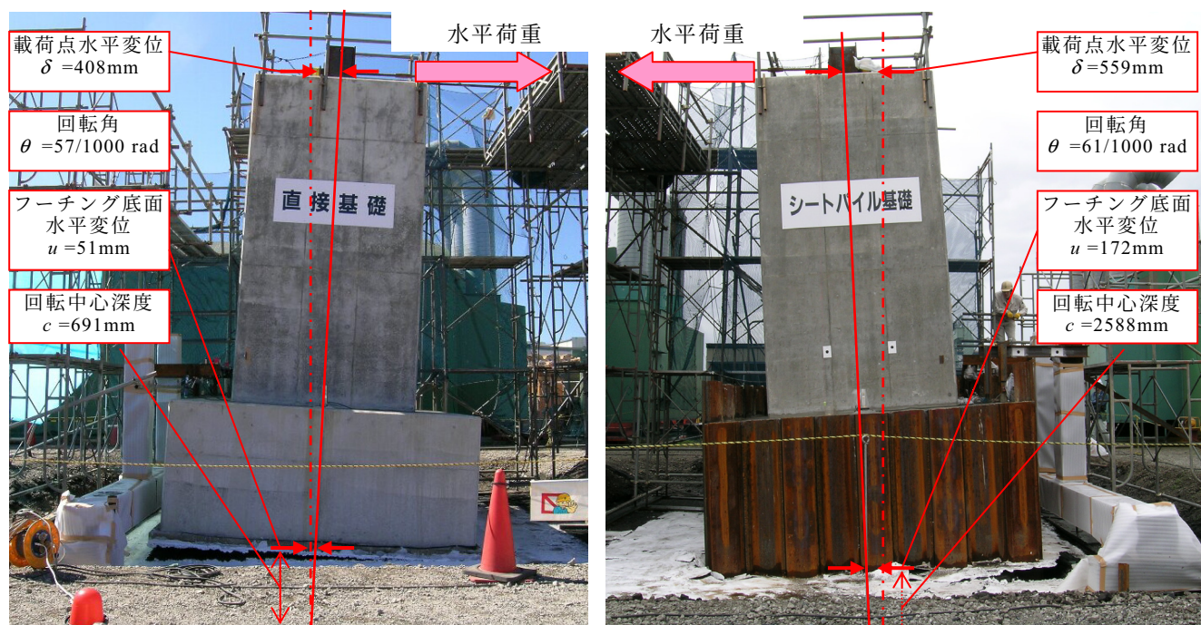
図-4.5 試験体の変形状況（最大変位時）
