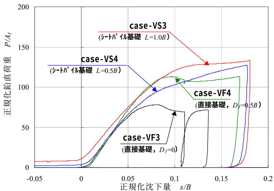
(b) case-VF3,VF4,VS3,VS4 : D_r=60\%
