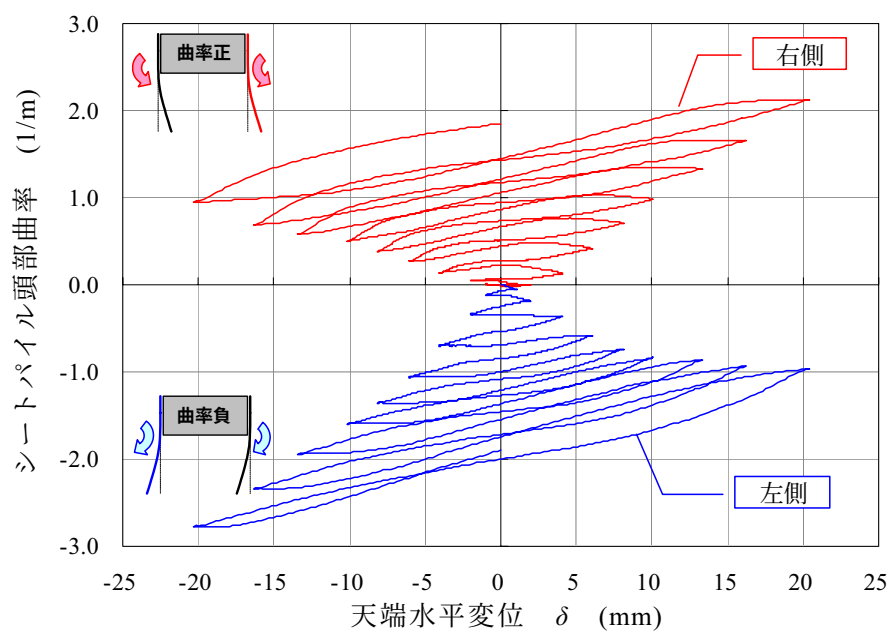
図-3.15 頭部曲率～水平変位関係 (case-HS3L)
