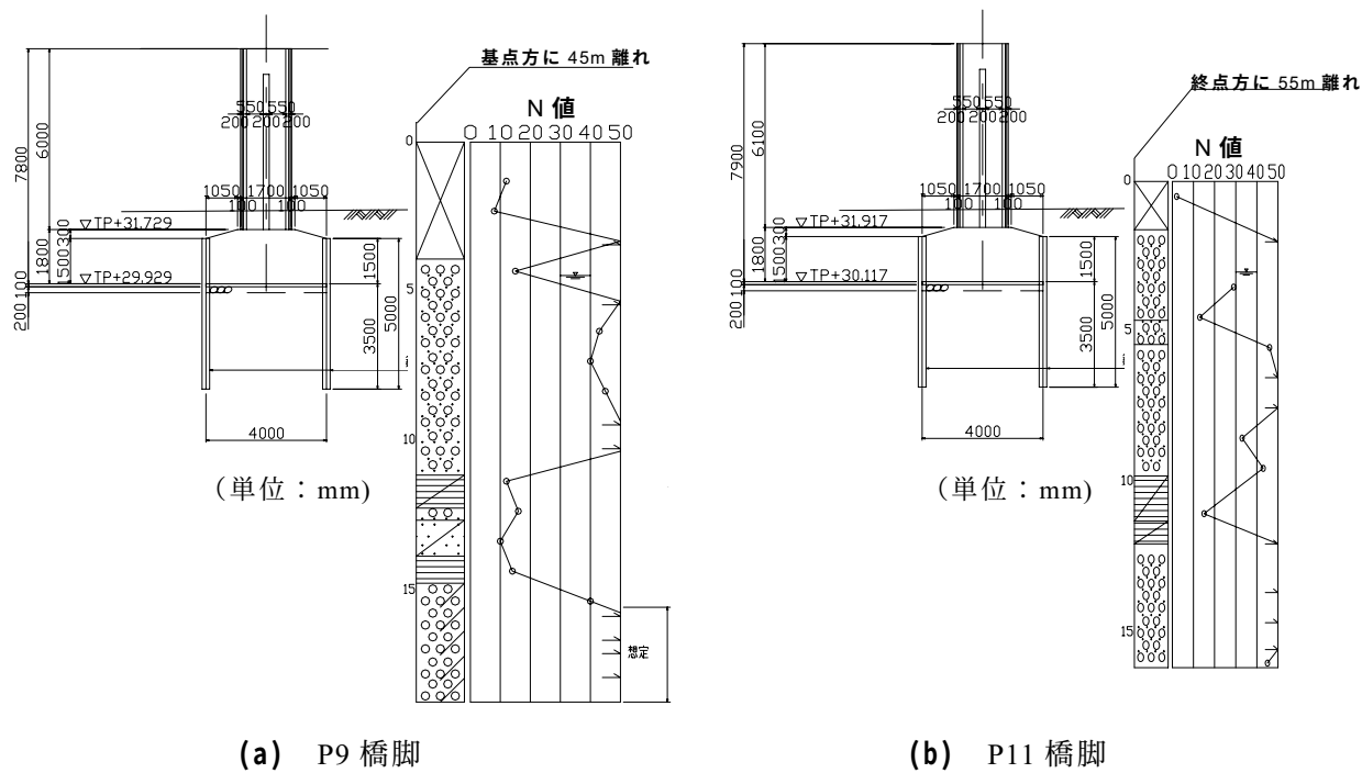
図-6.1 試験対象橋脚と土質柱状図
