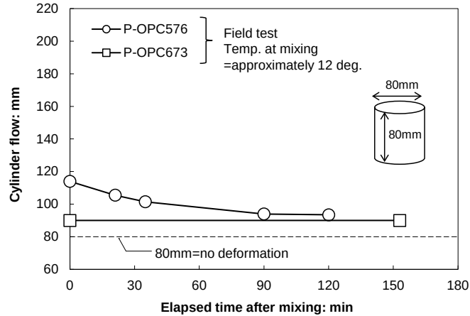
図-3.11 シリンダーフロー値の経時変化（高分子系 OPC）
