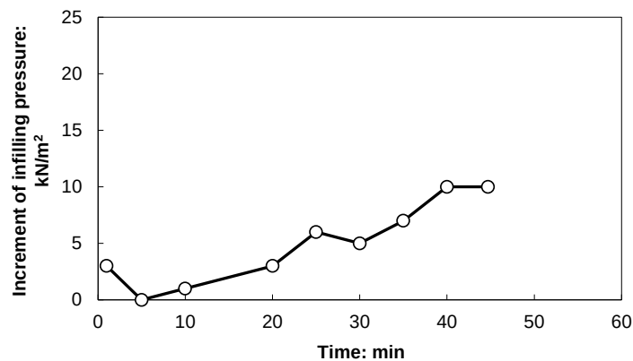
図-5.15 圧入圧の経時変化
