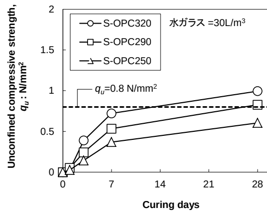
(c) 一軸圧縮強さの材齢変化
