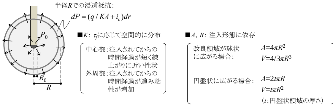
図-4.14 注入圧算定式 の概念
