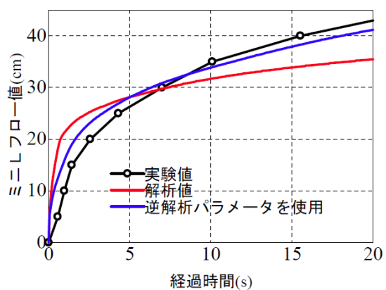
図-2.10 L字フロー試験結果と解析シミュレーションの比較
