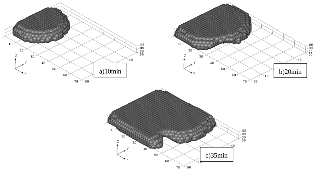
図-3.55 解析で得られた充填の進展（圧入空間内の起伏の影響）
