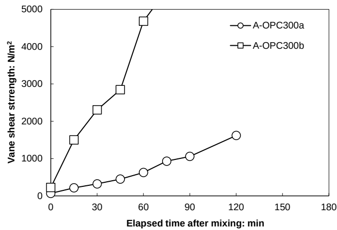
図-3.16 ベーンせん断抵抗の経時変化（アルミニウム系 OPC）
