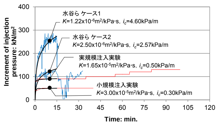
図-4.17 注入圧のフィッティングによる同定結果
