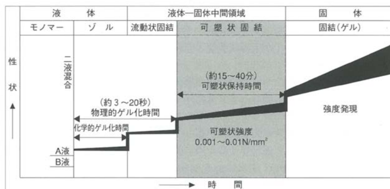
図-3.10 三木らが示した可塑性グラウト強度の経時変化の概念（文献 8 より）
