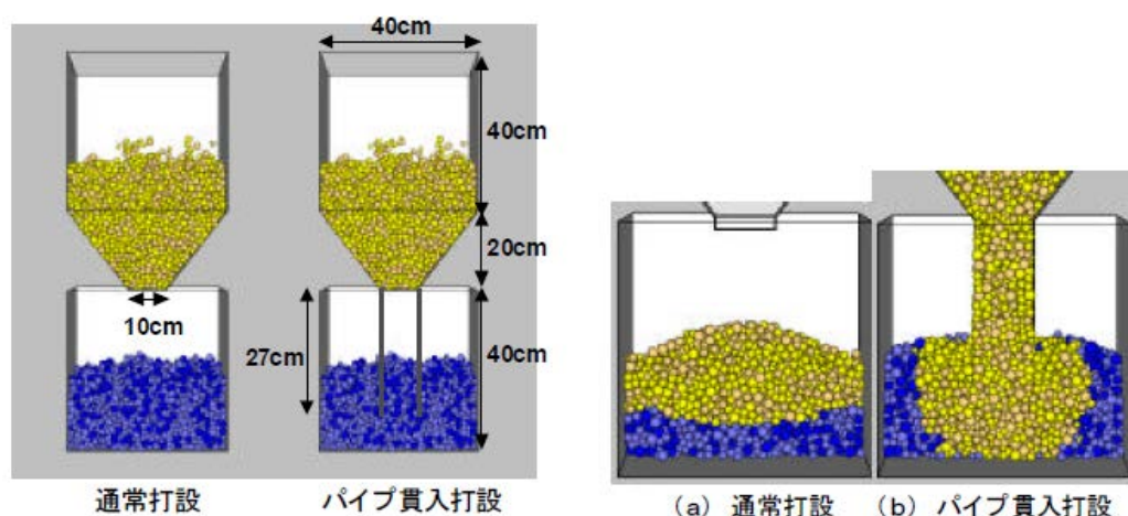
図-2.11 コンクリートの打重ねを対象とした解析検討（左：解析モデル，右：解析結果）
