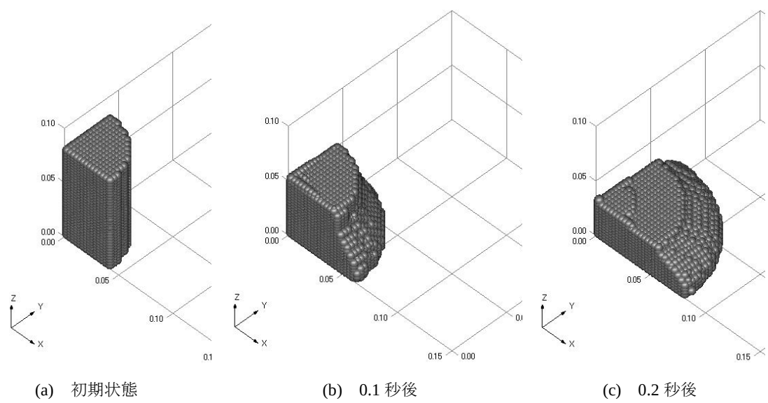
図-3.35 解析で再現したスランプ挙動 ( \eta=200\text{N/m}^2 )
