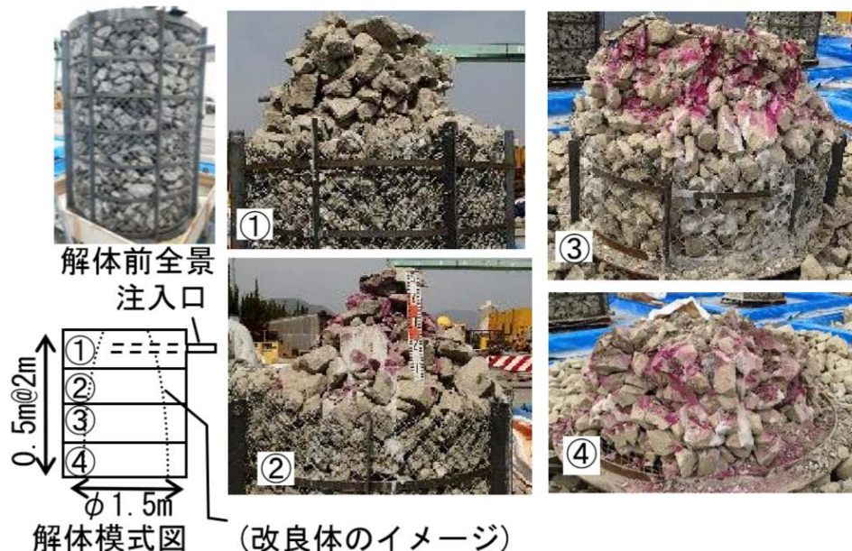
図-2.38 岩ズリ盛土の沈下防止対策に関する充填実験の結果
