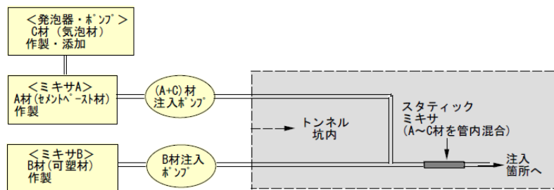
図-2.16 可塑性グラウトの配管輸送システムの例 23
