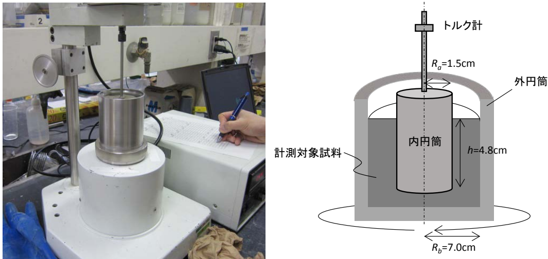
図-3.5 回転粘度計によるレオロジー特性の測定
