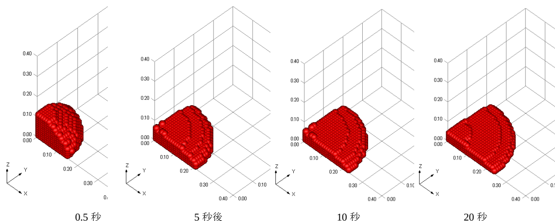
図-3A.6 解析結果 (高流動コンクリートのフロー挙動)
