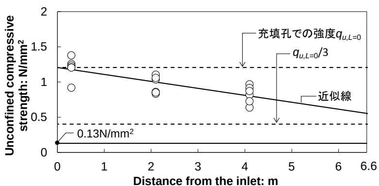
図-5.17 一軸圧縮強さの分布 (28 日材齢)
