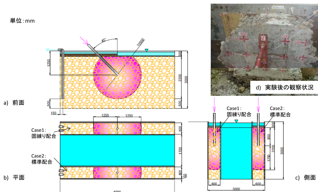
図-2.37 実験概要と掘出し確認された固化体
