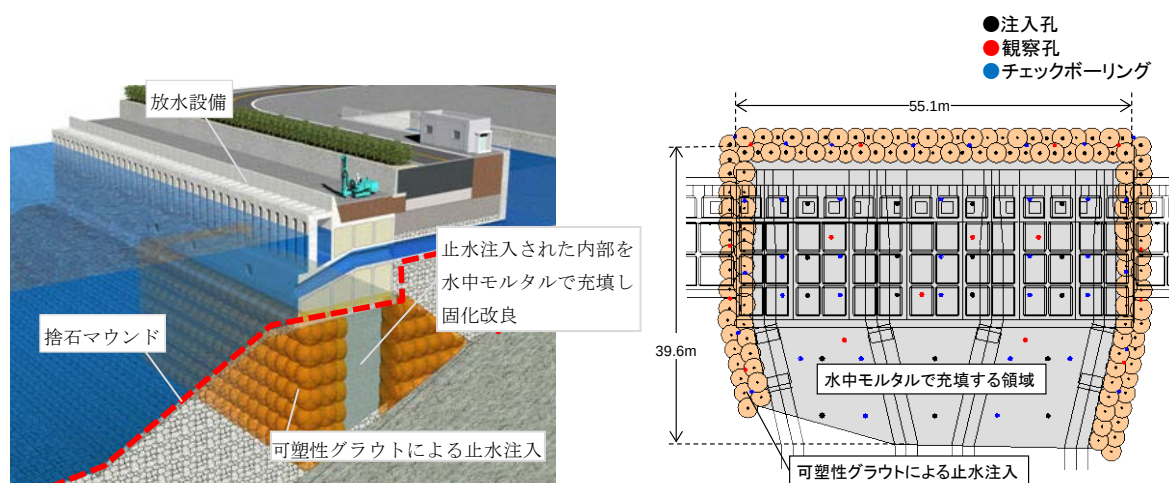
図-2.31 可塑性グラウトを併用した捨石マウンドの耐震補強
