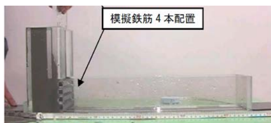
図-2.8 L字フロー試験状況
