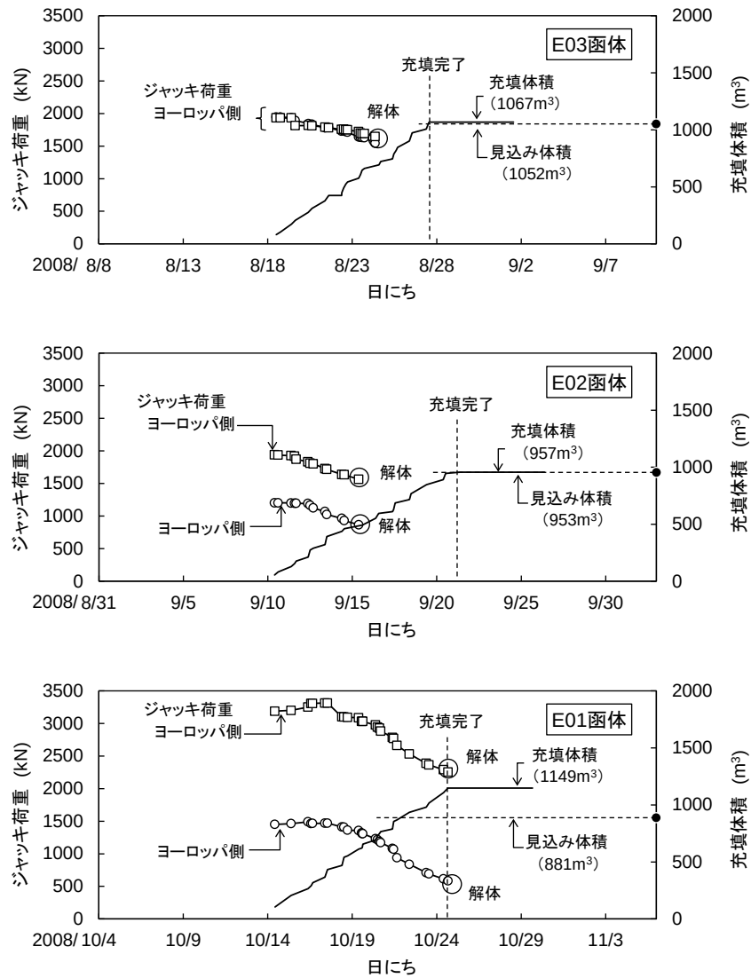
図-5.33 充填中のジャッキ荷重の変化 (E03～E01 函体)
