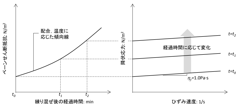
図-3.31 可塑性グラウトのせん断抵抗の時間変化と提案モデル
