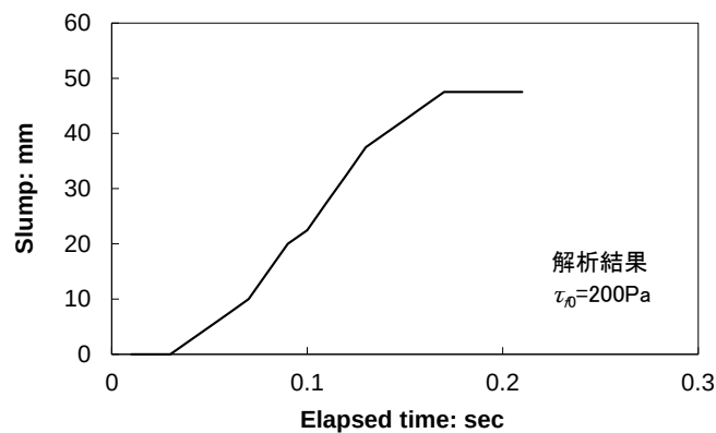
図-3.34 スランプの経時変化（ \tau_0=200\text{Pa} ）
