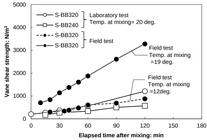
図-3.14 ベーンせん断抵抗の経時変化（水ガラス系 BB）
