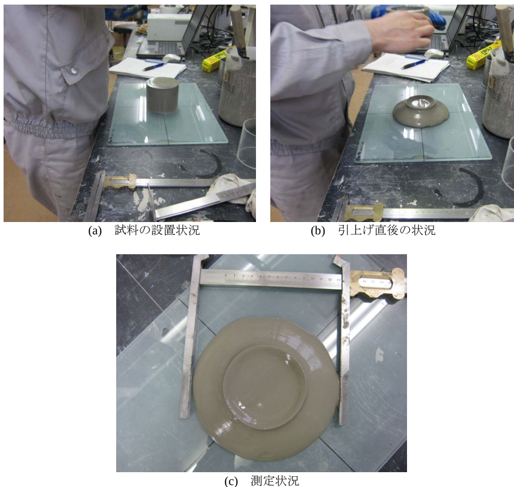
図-3.6 可塑性グラウトのシリンダーフロー測定状況
