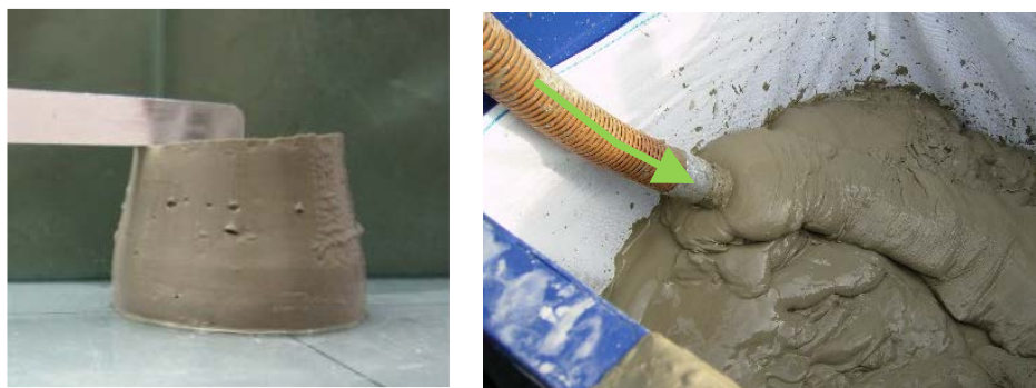
図-1.1 可塑性グラウト（左：形状を保持した状態、右：供給圧で容易に押し出される状況）
