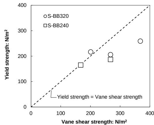
図-3.30 ベーンせん断抵抗と降伏応力の関係
