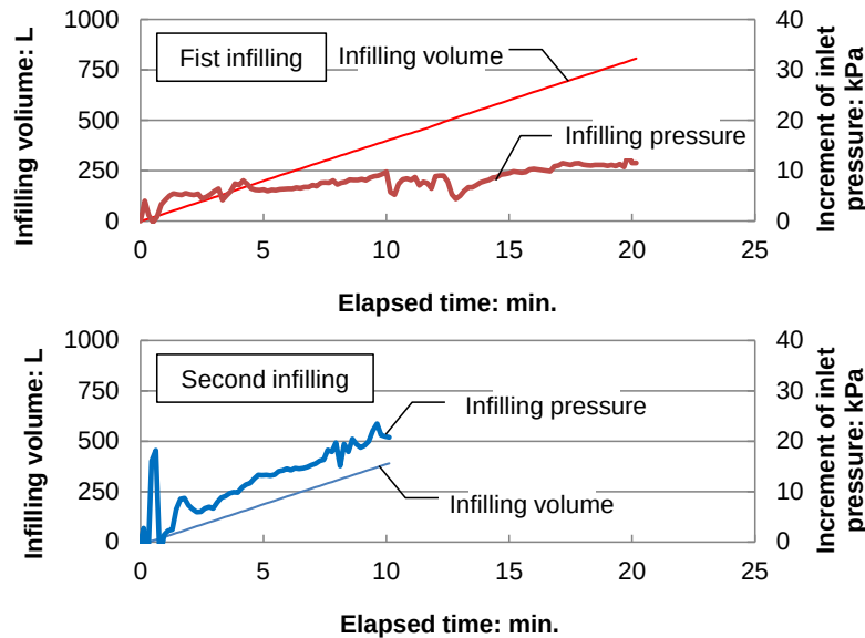
図-3.47 供給量，供給圧の実測推移(先行・後行充填)
