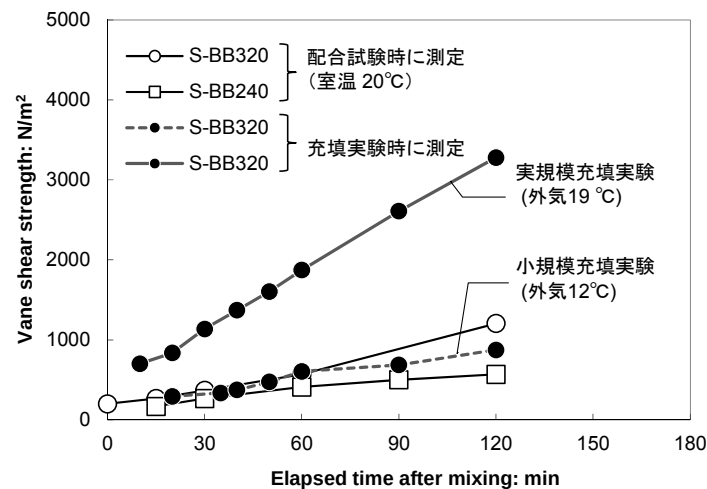
図-4.20 ベーンせん断抵抗の経時変化（水ガラス系 BB，図-3.14 を再掲）
