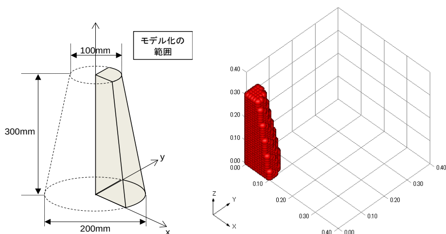
図-3A.5 解析モデル（高流動コンクリートのフロー挙動）
