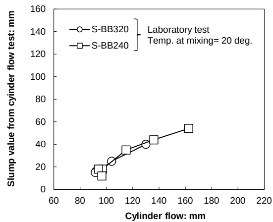
図-3.26 シリンダーフロー値とスランプ値の関係（水ガラス系 BB）
