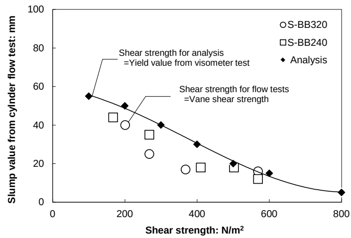
図-3.38 降伏応力・ベーンせん断強度とスランプの関係
