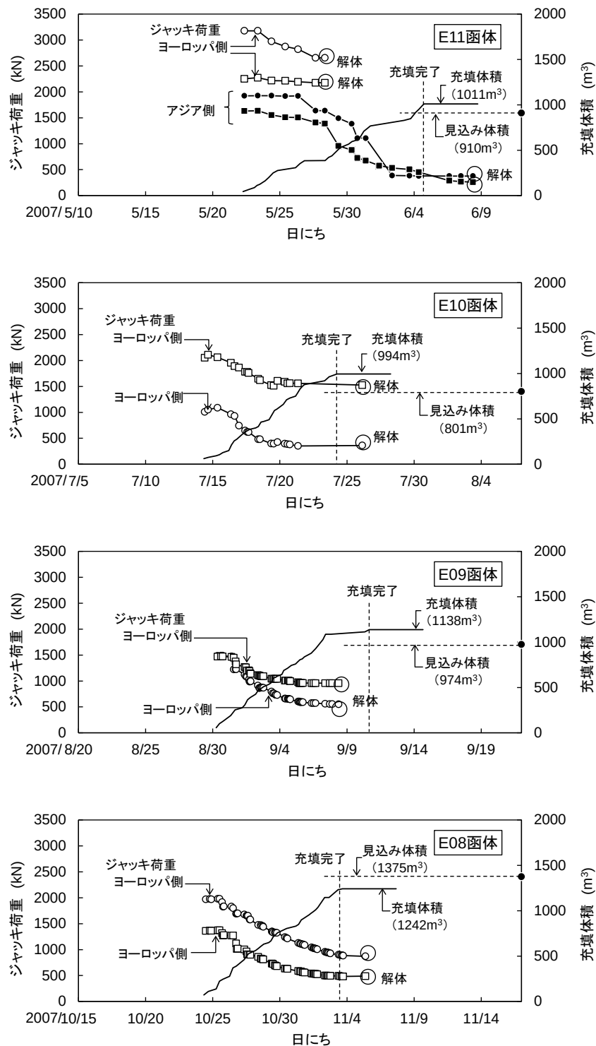
図-5.31 充填中のジャッキ荷重の変化 (E11～E08 函体)
