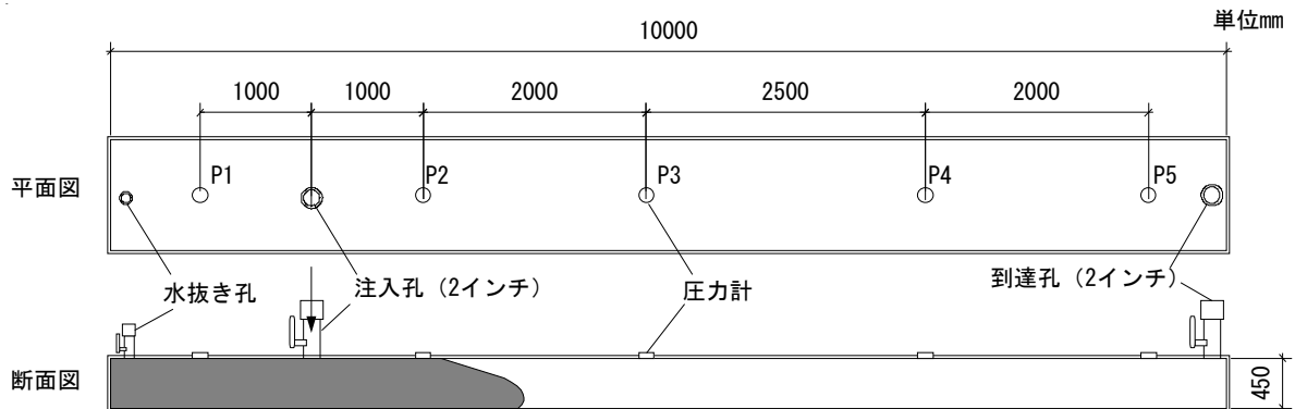
図-3.58 実験概要（粘性変化の影響）
