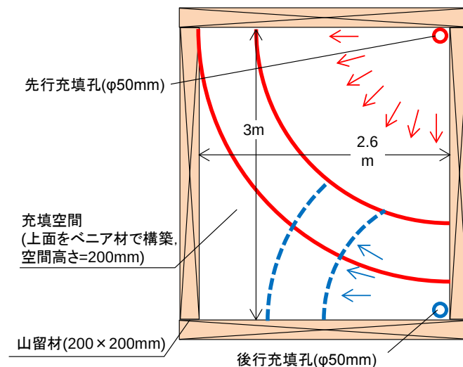
図-3.39 実験概要 (平面図)
