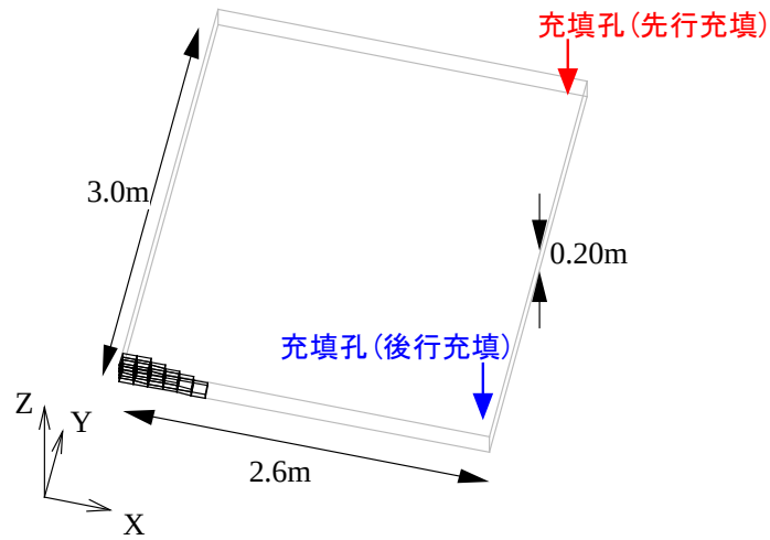
図-3.48 解析モデル（段階的な空洞圧入）
