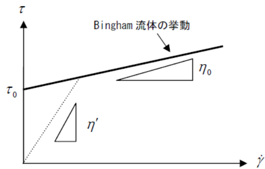
図-2.1 ビンガムモデルのひずみ速度と応力の関係
