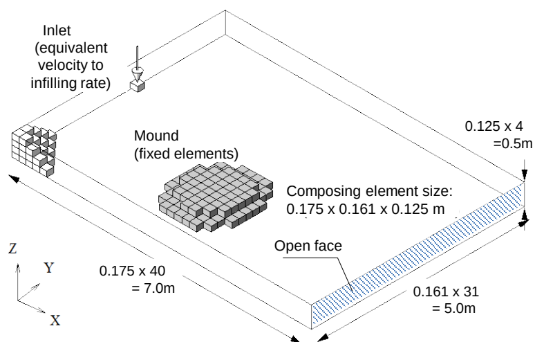
図-3.54 解析モデル
