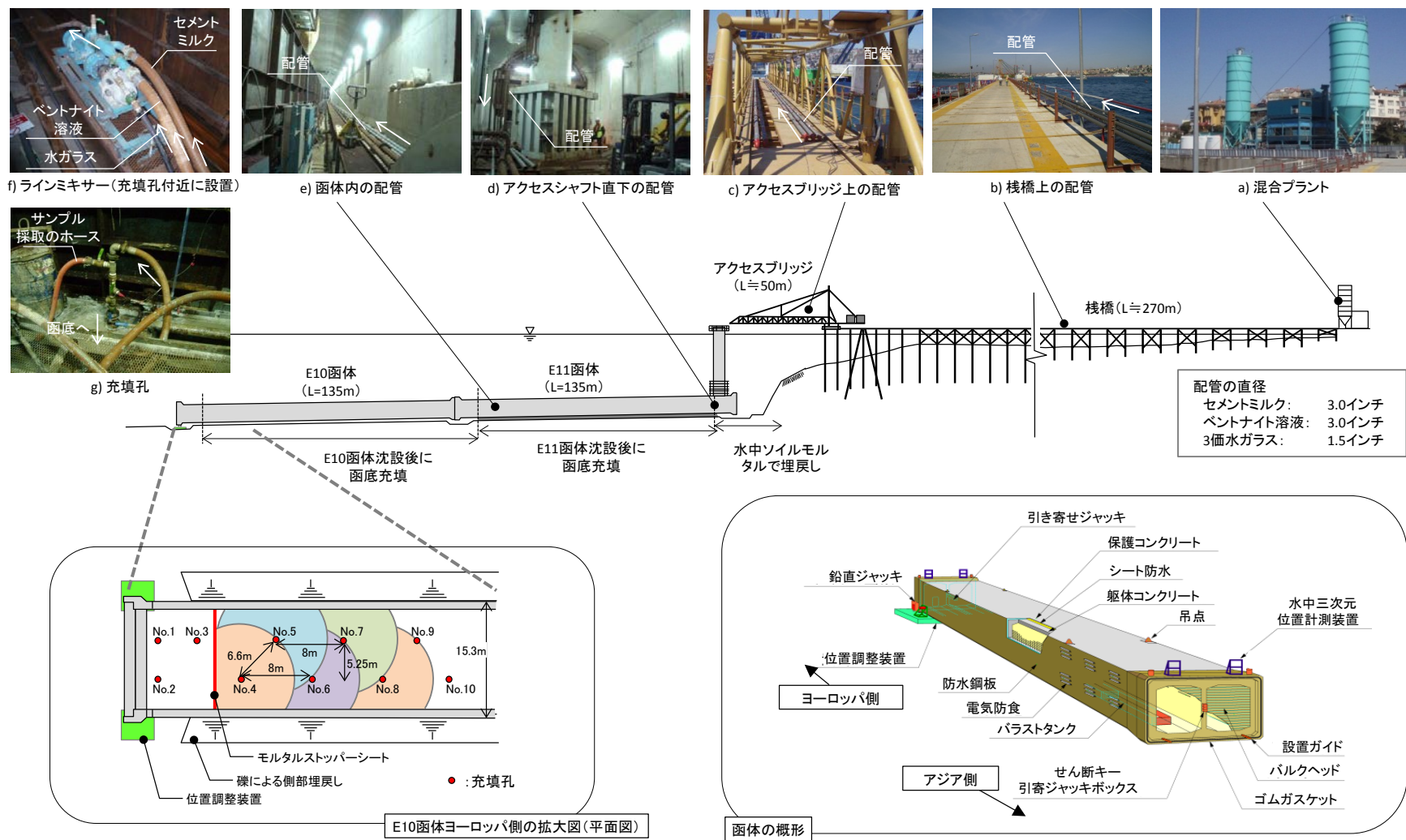
図-5.22 製造プラントを含む全体配置と函底充填部分の平面・断面図 (E10 函体施工時の状況)
