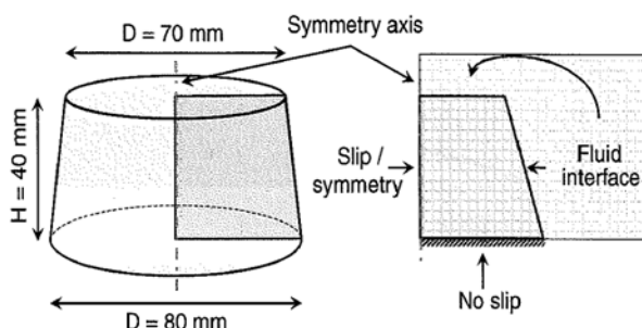
図-2.3 セメントミルクの流動挙動解析モデル
