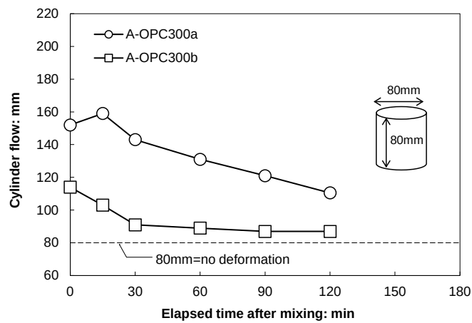
図-3.12 シリンダーフロー値の経時変化（アルミニウム系 OPC）
