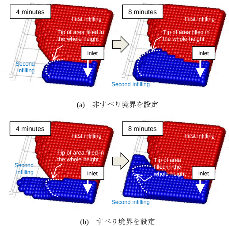
図-3.51 充填状況の進展（解析結果）
