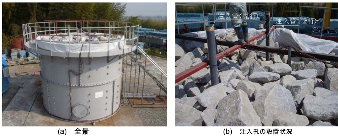
図-4.8 実験準備状況 (実規模注入実験)
