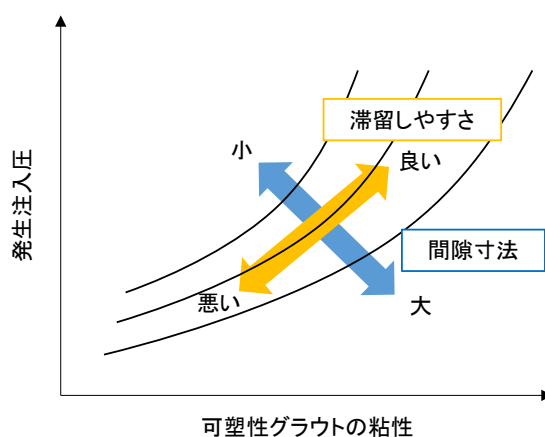
図-6.9 可塑性グラウトの粘性と発生注入圧の概念
