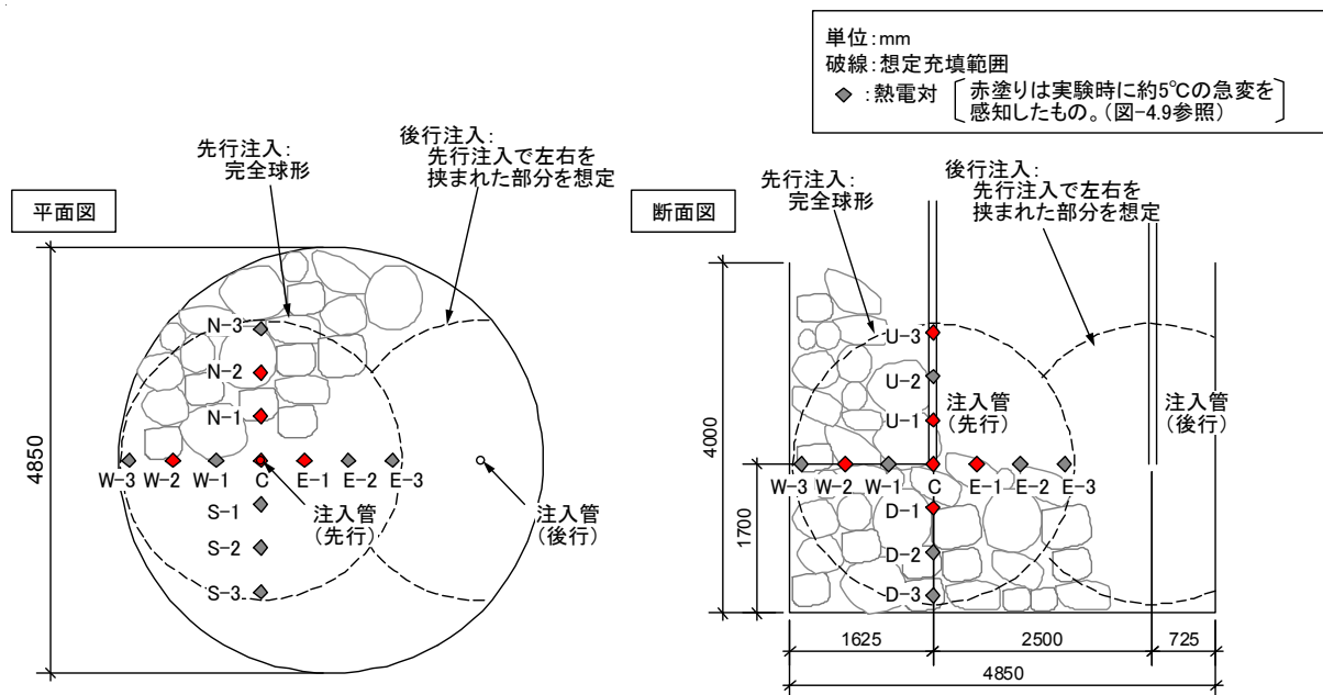
図-4.7 実験概要 (実規模注入実験)
