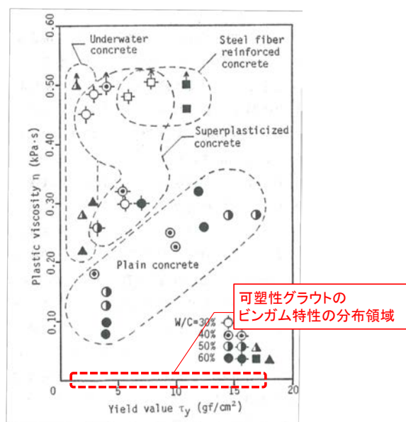
図-3.32 ビンガム定数の比較
