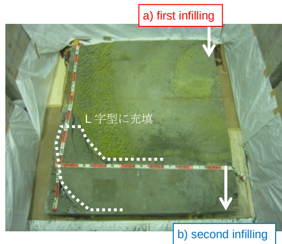
図-3.45 充填後の観察状況（左：先行充填後，右：後行充填後）
