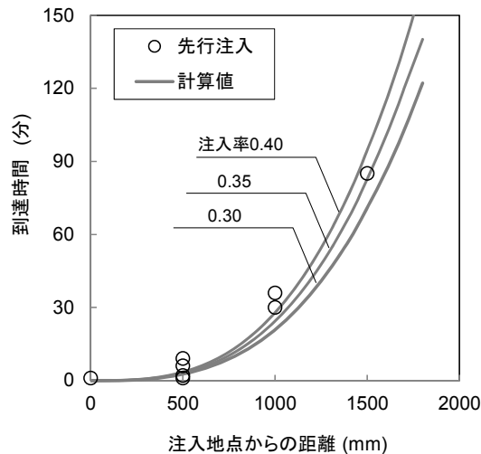
図-4.10 注入孔からの距離と到達時間の関係（実規模注入実験）
