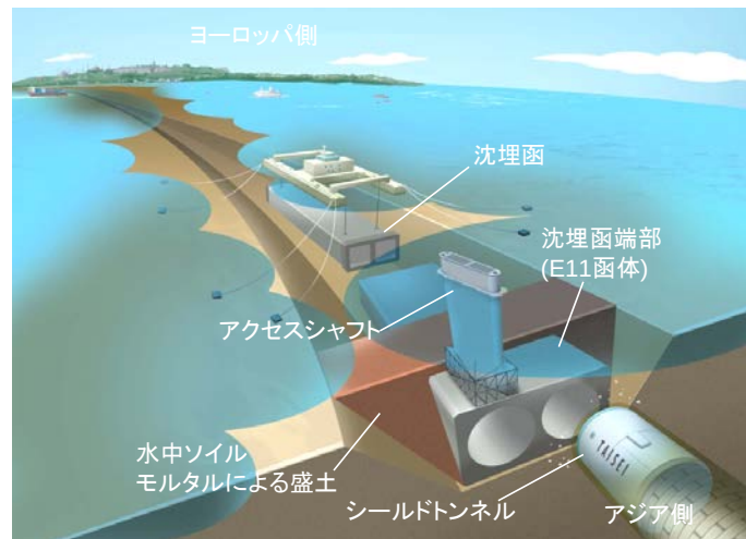
図-5.2 アジア側沈埋トンネル端部の概要図
