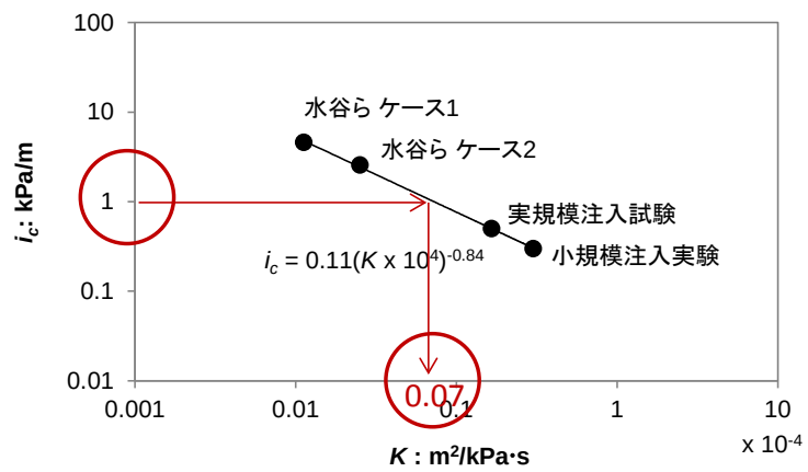
図-6.10 注入係数と降伏圧力勾配の関係
