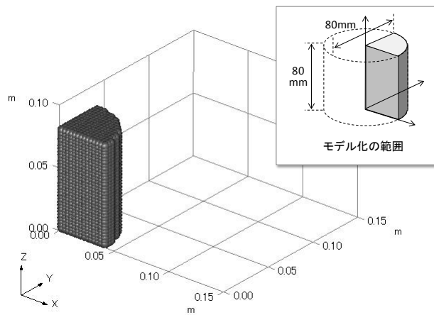
図-3.33 解析モデル (シリンダーフローのシミュレーション)
