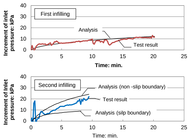
図-3.50 充填圧の経時変化（実測および解析結果）
