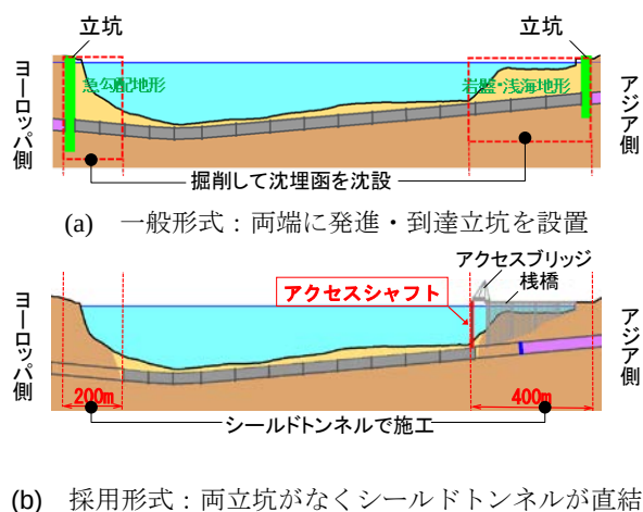
図-5.1 沈埋トンネルの設置方法（縦断面図）
