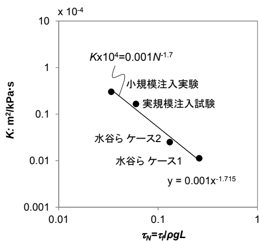
図-4.18 注入仕様に関する無次元量と注入係数の関係
