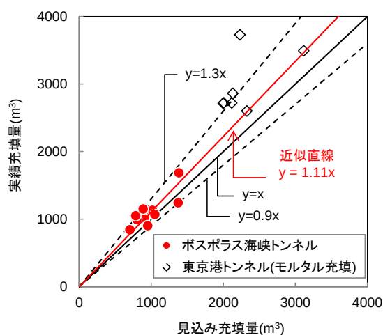
図-5.34 見込み充填量と実績充填量の関係(全 11 函体)
