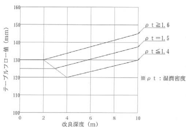
図-6.4 浅層・中層混合処理工法に対する推奨テーブルフロー値
