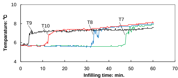
図-5.12 温度センサーによる到達状況の感知（T7～10）
