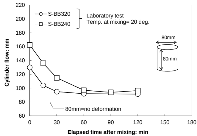
図-3.8 シリンダーフロー値の経時変化（水ガラス系 BB）
