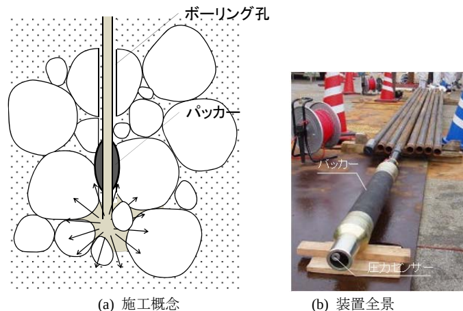
図-4.23 大型パッカー付き注入装置
