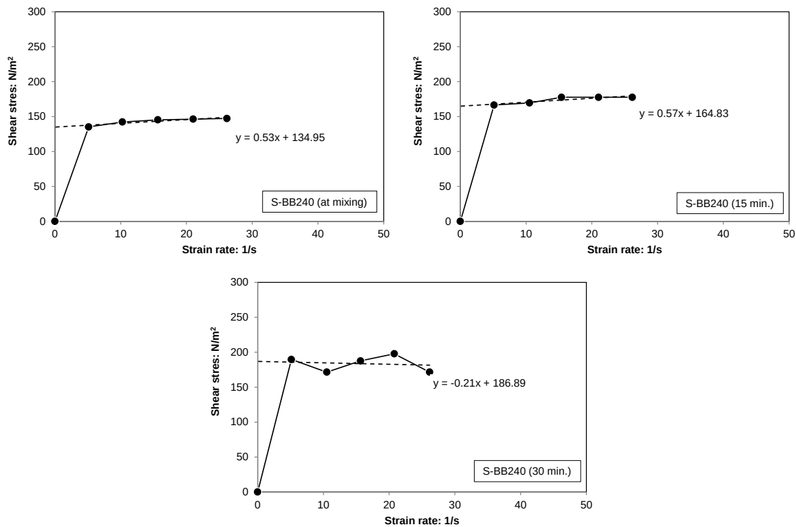
図-3.18 ひずみ速度～応力の関係とせん断抵抗（S-BB240，混合直後・15分後・30分後）
