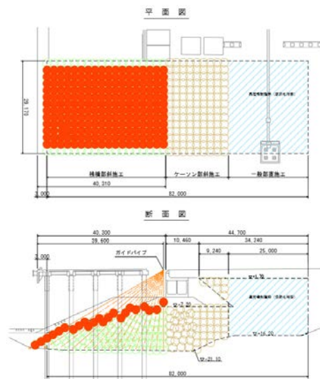
図-5 表層改良範囲図
