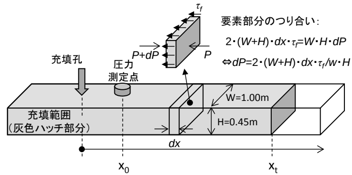
図-5.18 充填圧と周面抵抗とのつり合いの想定
