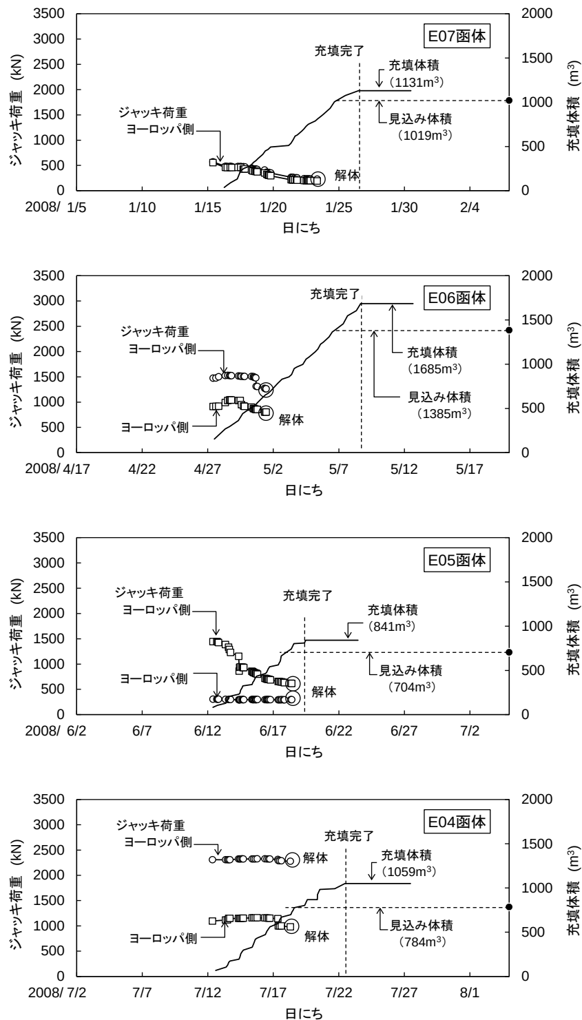
図-5.32 充填中のジャッキ荷重の変化 (E07～E04 函体)
