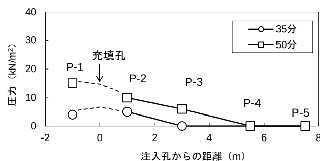
図-5.8 充填性確認実験での圧力分布
