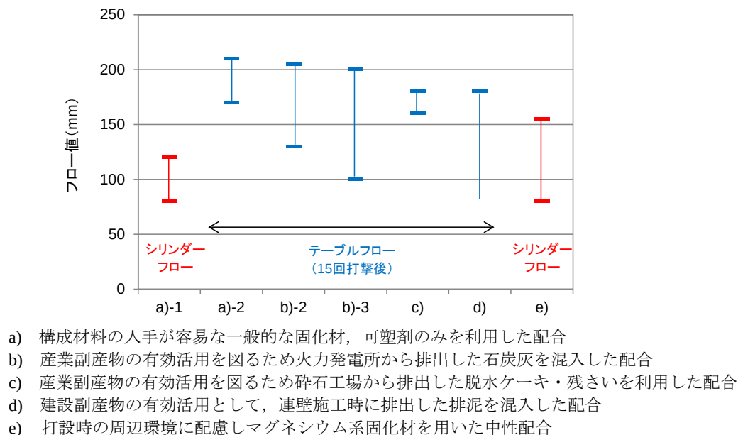
図-2.20 可塑性充填材のフロー値の実績
