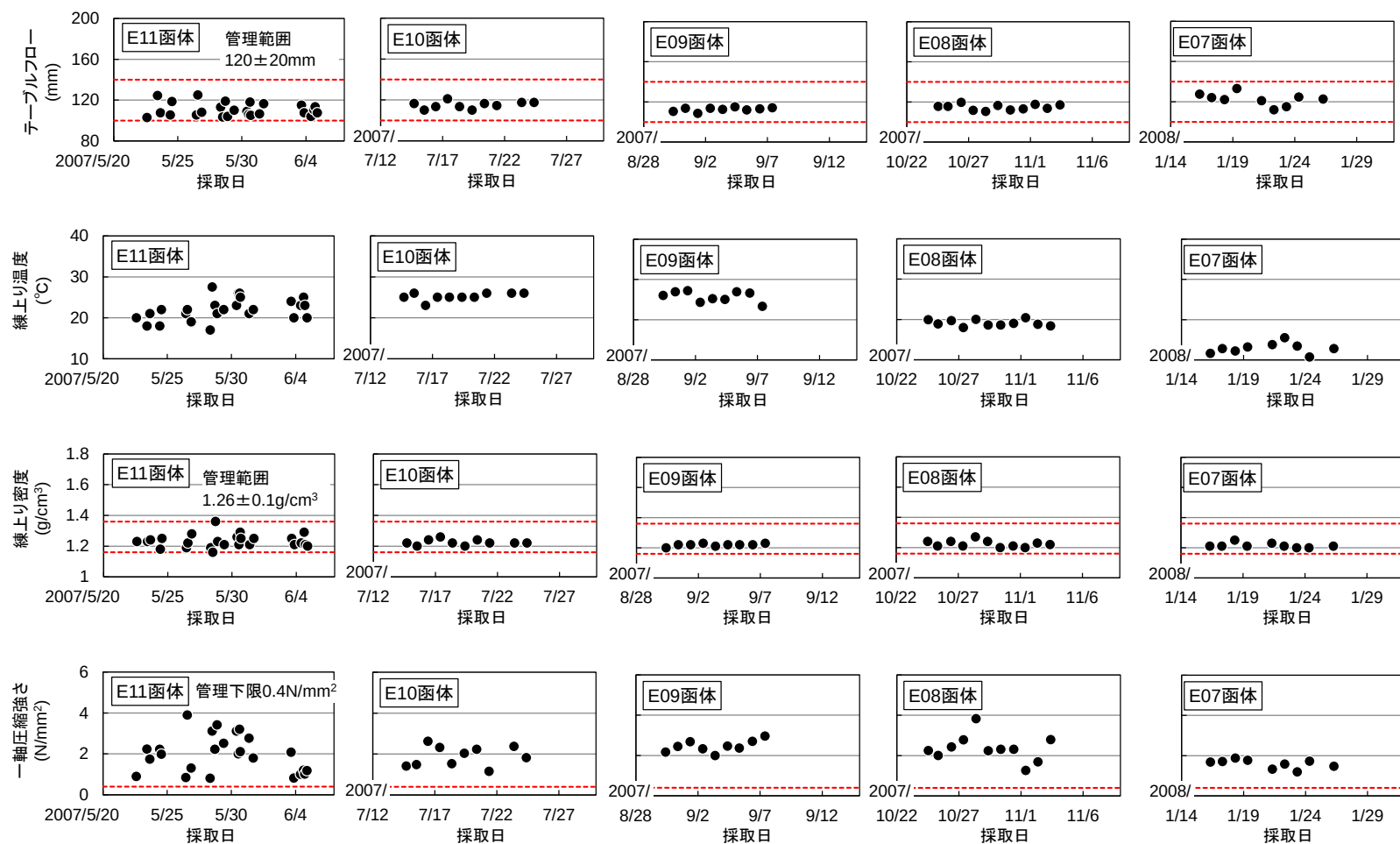
図-5.24 テーブルフロー，練上り温度，温度，一軸圧縮強さ（E11，E10，E09，E08，E07 函体）
