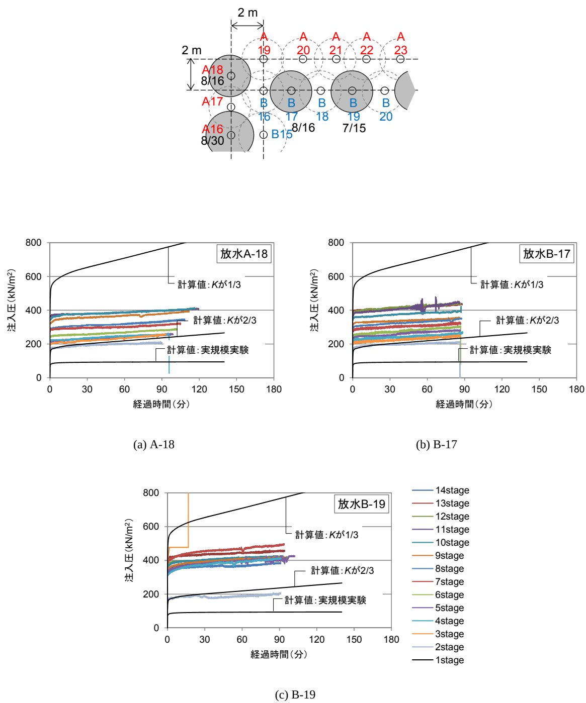
図-4.28 注入圧の比較（角部1次注入：A-18, B-17, B-19）
