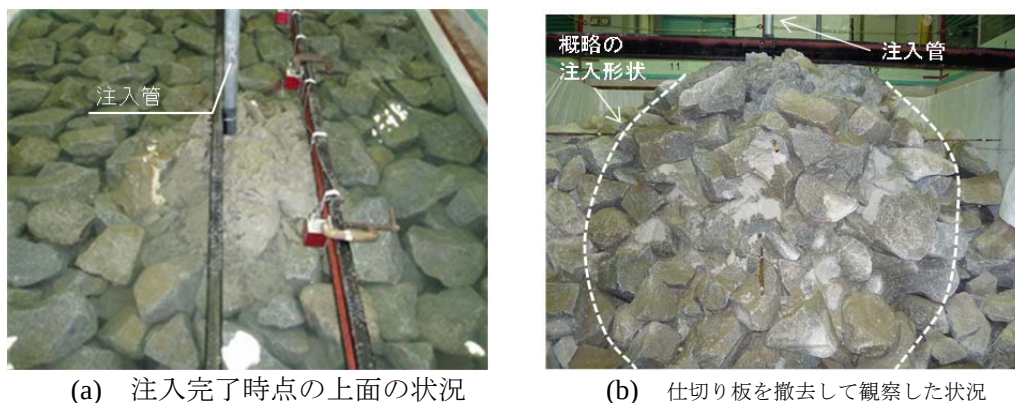
図-4.5 注入実験後の観察（小規模注入実験）
