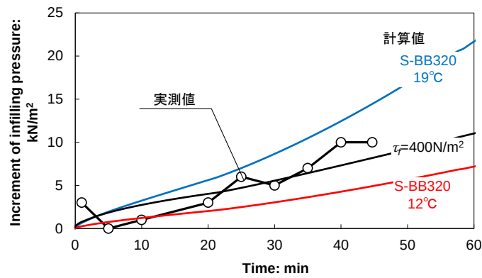
図-6.13 実大実験で得られた充填圧と計算値（水平到達距離約 6m）
