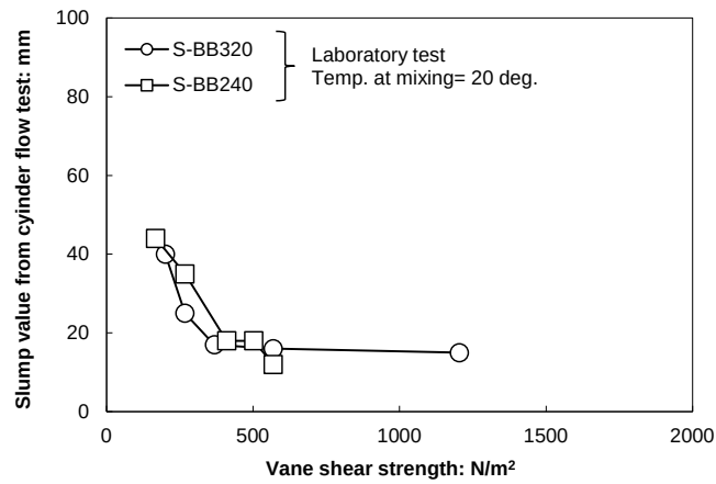
図-3.28 ベーンせん断抵抗とスランプ値の関係（水ガラス系 BB）
