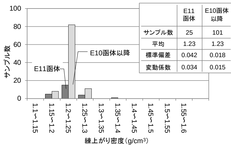
図-5.27 練上がり密度の頻度分布
