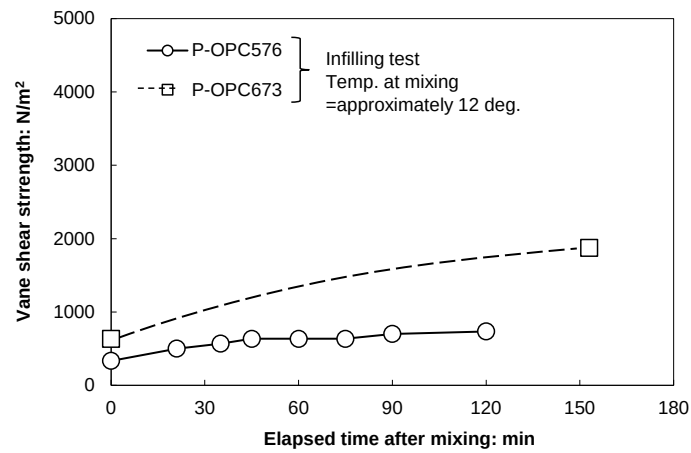
図-3.15 ベーンせん断抵抗の経時変化（高分子系 OPC）
