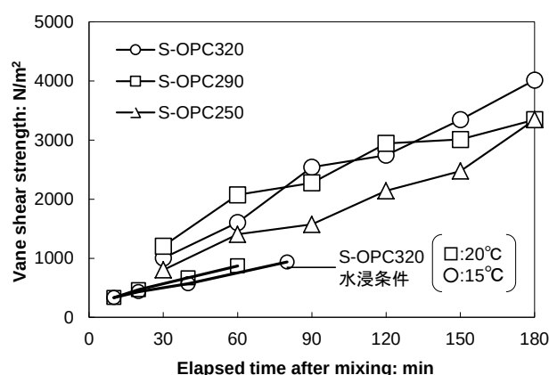
図-3.13 ベーンせん断抵抗の経時変化（水ガラス系 OPC）
