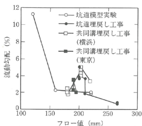
図-6.2 流動化処理土に対する流動勾配とフロー値の関係
