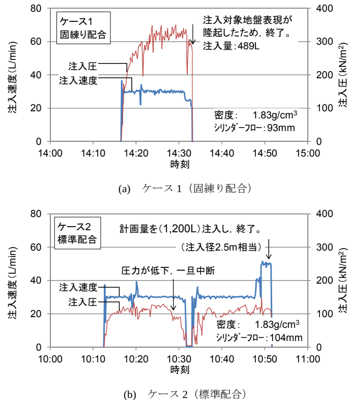
図-4.16 既往の注入実験での注入速度・注入圧（水谷らの文献に加筆）
