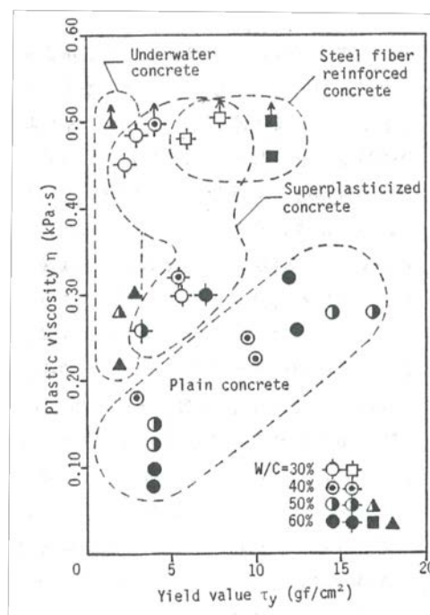
図-2.2 各種コンクリートのビンガム定数の関係 10
