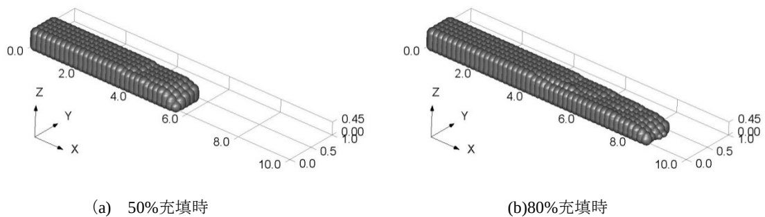
図-3.62 解析で得られた充填範囲の変化（粘性変化の影響）
