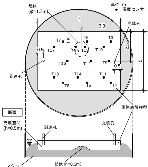
図-3.52 充填実験の概要
