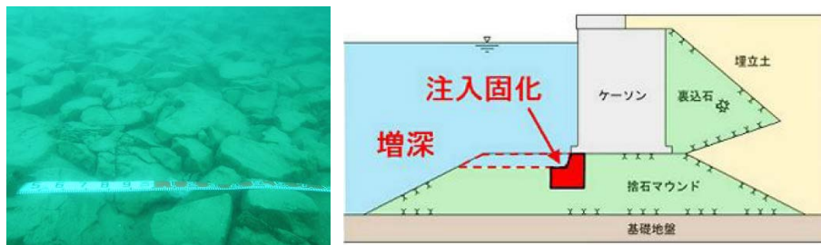
図-2.36 検討対象の捨石マウンドと既設岸壁の増深構造
