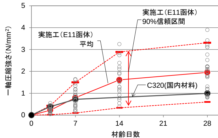
図-5.29 一軸圧縮強さの材齢変化(E11 函体)
