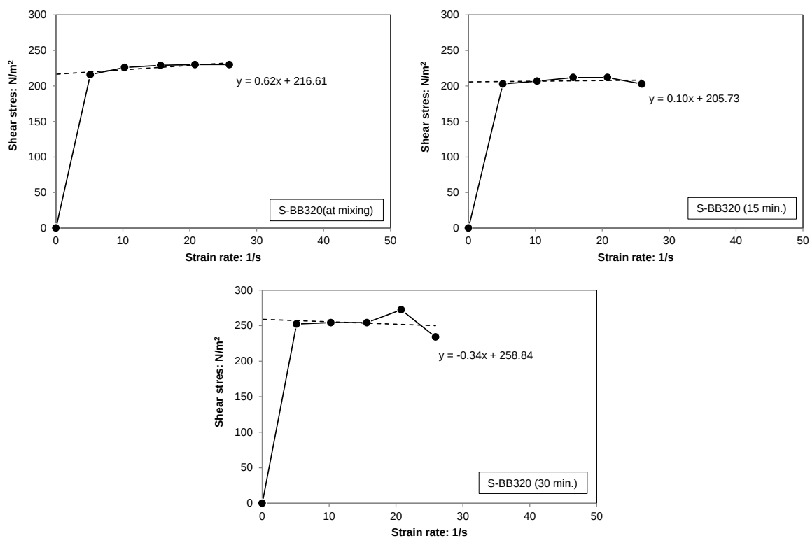
図-3.17 ひずみ速度～応力の関係とせん断抵抗（S-BB320，混合直後・15分後・30分後）
