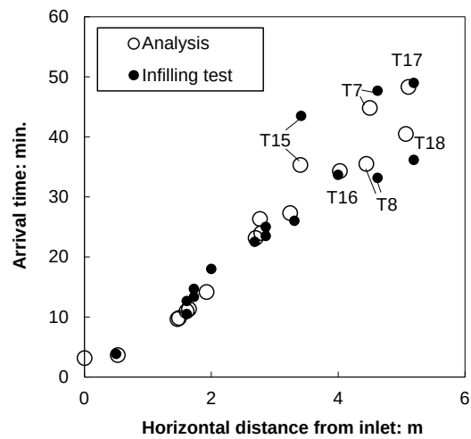
図-3.56 実測・解析による充填孔からの距離と到達時間の関係（圧入空間内の起伏の影響）
