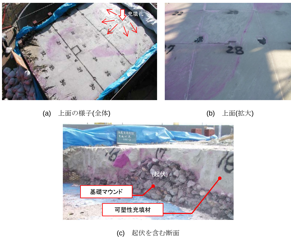
図-5.16 充填状況の確認状況
