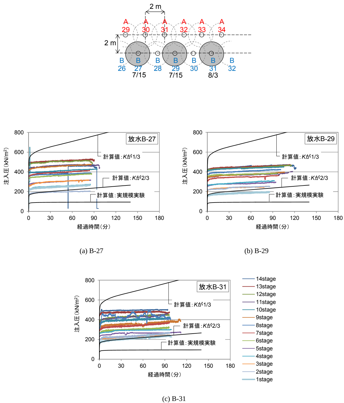
図-4.31 注入圧の比較（中央部 1 次注入：B-27, B-29, B-31）
