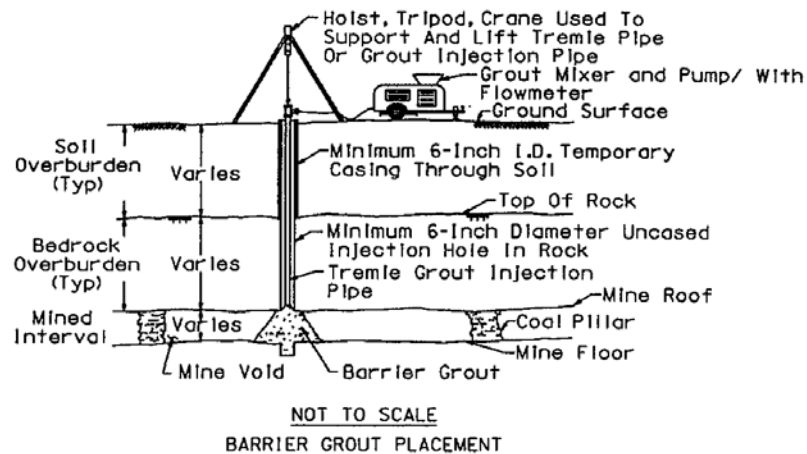
図-2.25 高速道路下の廃坑埋戻しにおける Barrier Grout の活用
