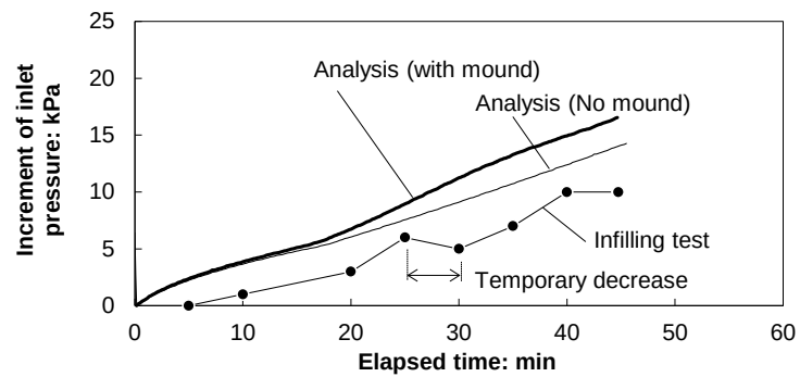
図-3.57 実測・解析による充填圧力の経時変化（圧入空間内の起伏の影響）
