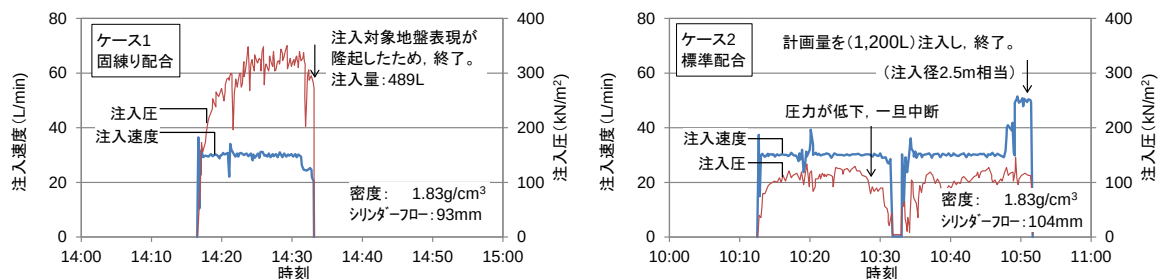
図-6.6 巨石地盤を対象とした可塑性グラウトの注入実験結果（注入速度と注入圧、文献5に基づき整理）
