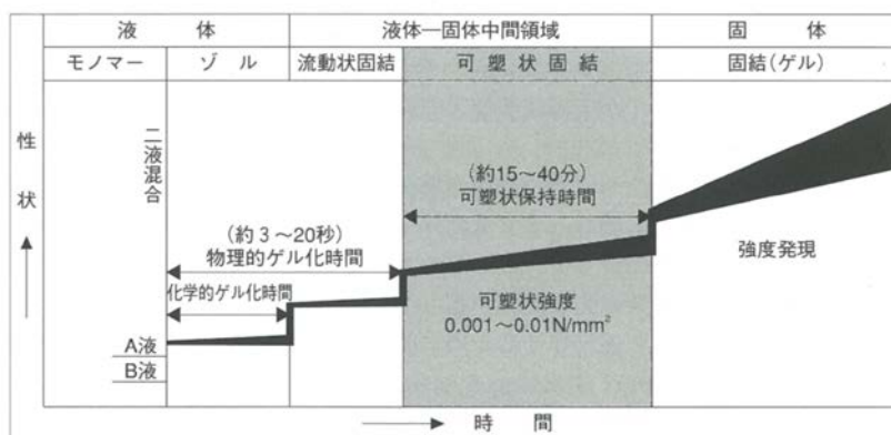
図-1.4 可塑性グラウトの粘性変化の概念（参考文献 2 より）
