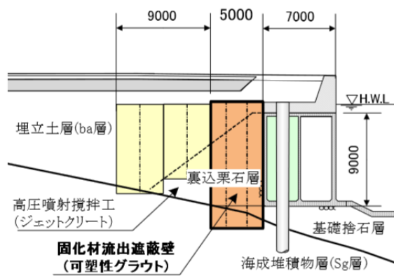
図-2.33 可塑性グラウトによる間隙充填計画
