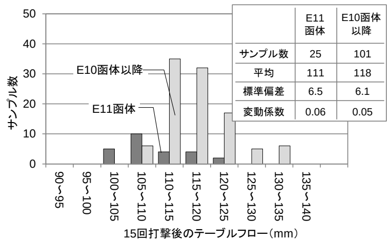
図-5.26 テーブルフローの頻度分布
