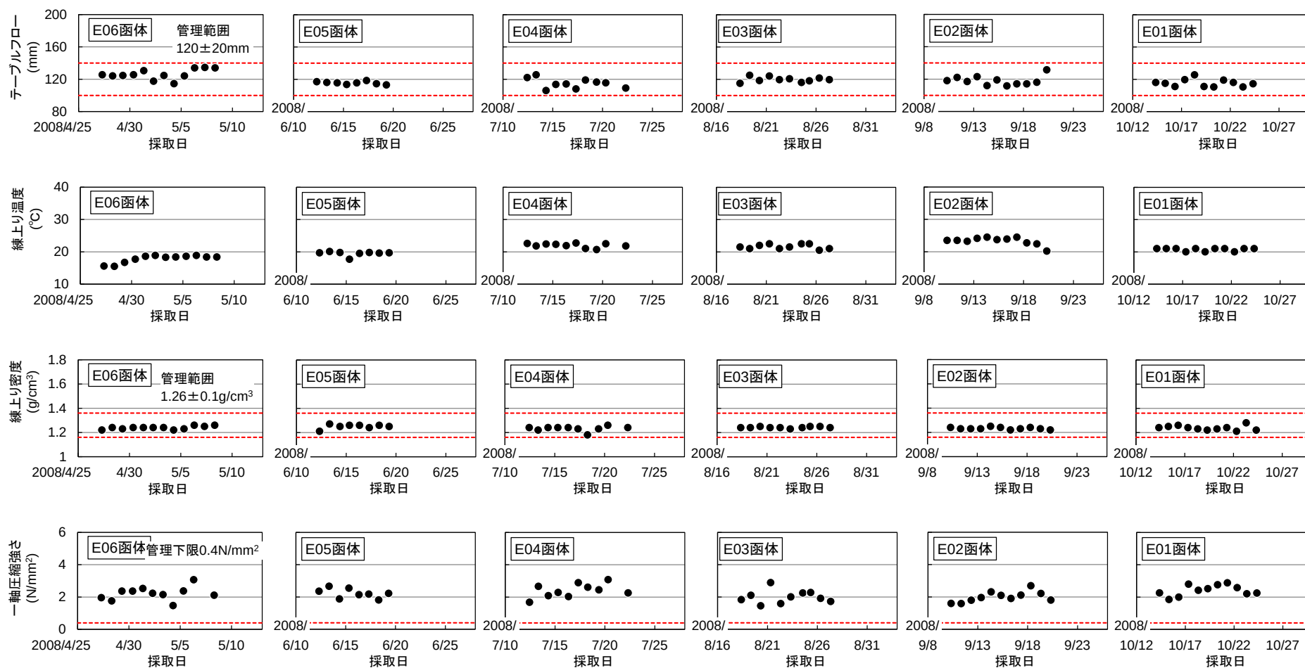
図-5.25 テーブルフロー，練上り温度，温度，一軸圧縮強さ（E05，E04，E03，E02，E01 函体）
