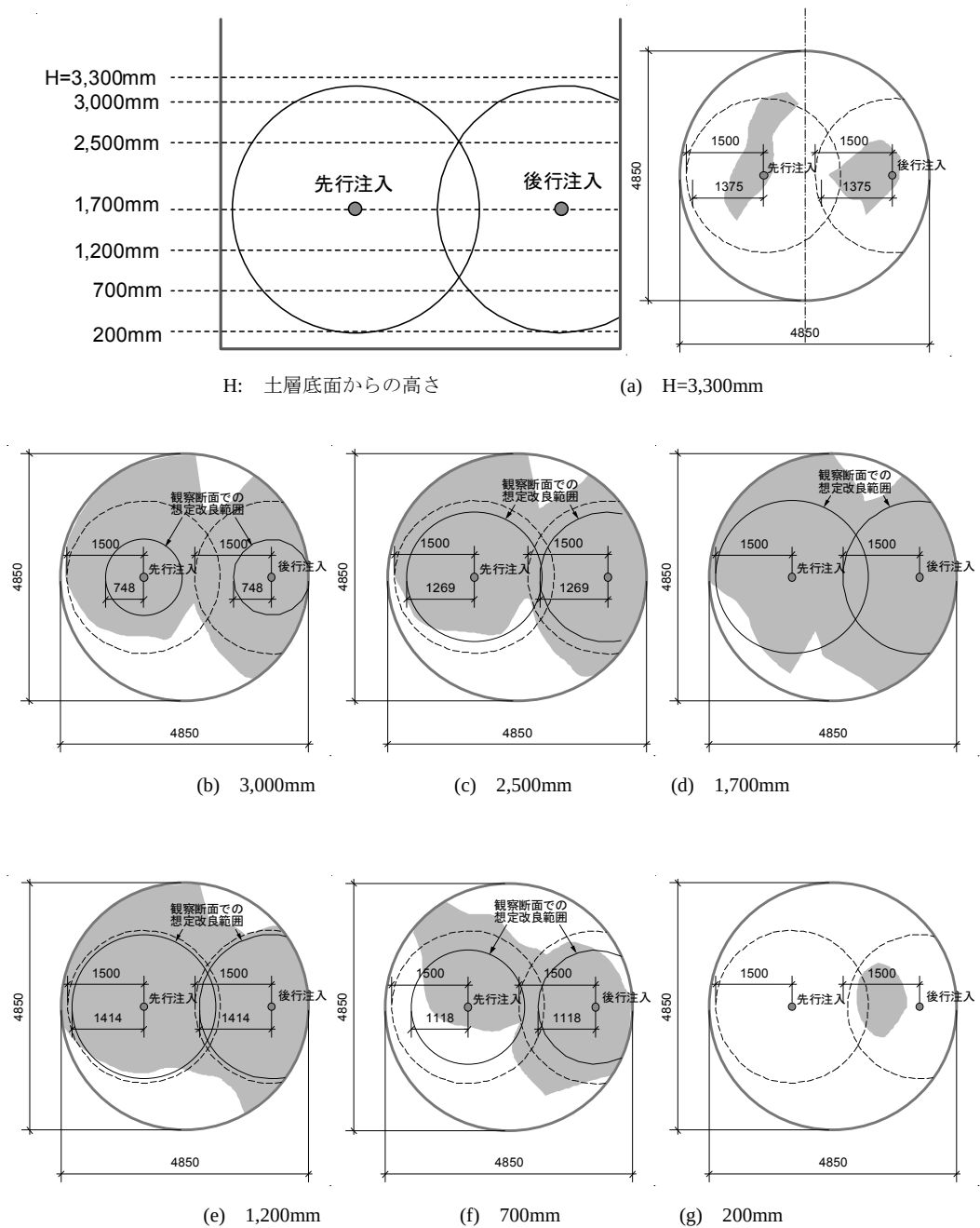
図-4.12 注入範囲の観察スケッチ（実規模注入実験）
