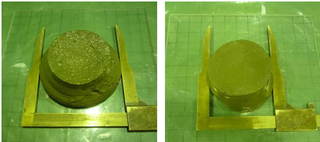
図-3.43 フロー値の確認状況（左：先行充填 TF：124mm，右：後行充填 TF:95mm）
