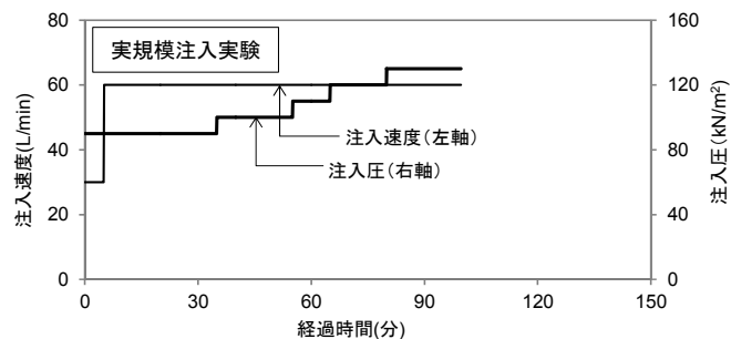
図-4.11 注入速度、注入圧の経時変化（実規模注入実験）
