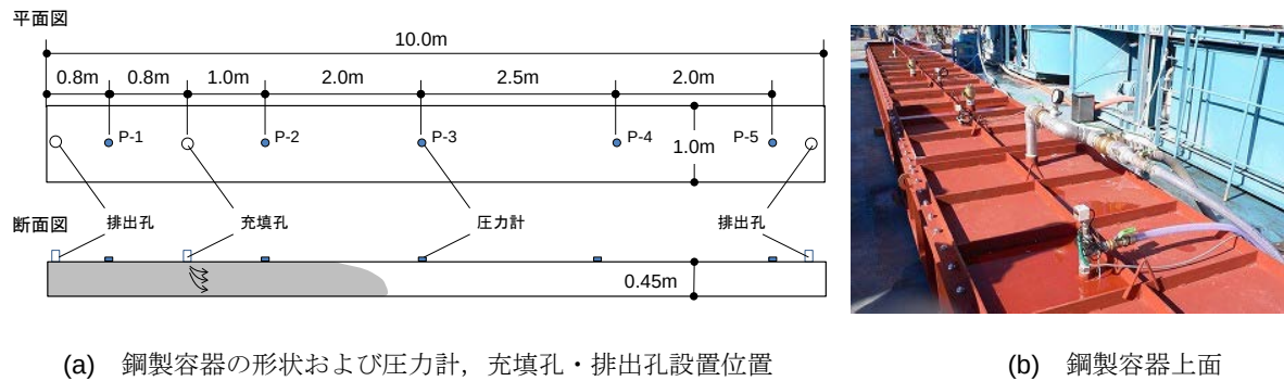
図-5.6 充填性確認実験
