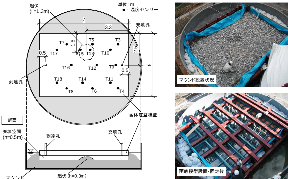
図-5.10 実規模実証試験の概要
