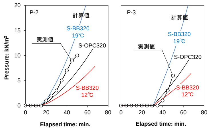
図-5.20 圧力の経時変化 (P-2, P-3)
