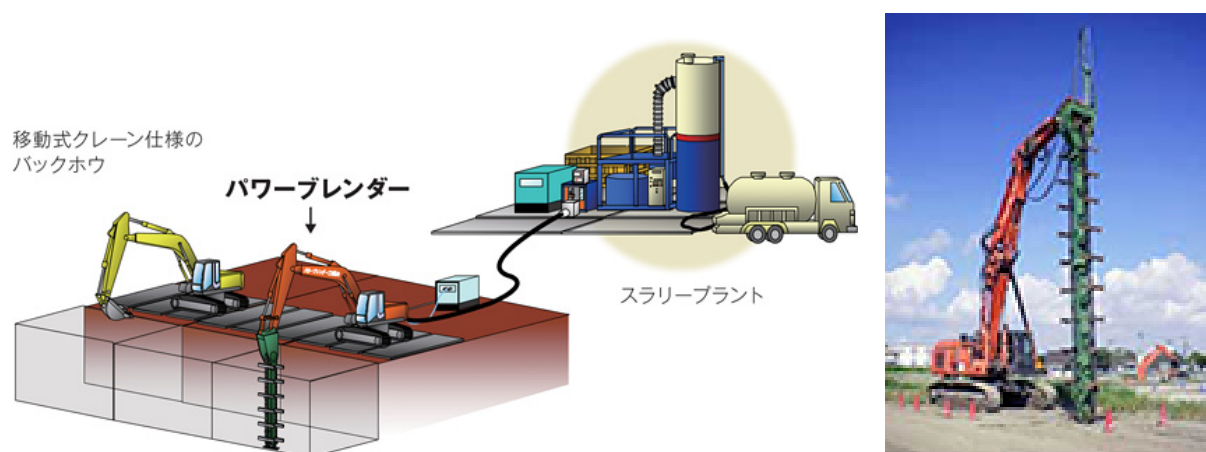
図-6.3 パワーブレンダー工法の概要とトレンチャー式攪拌混合機
