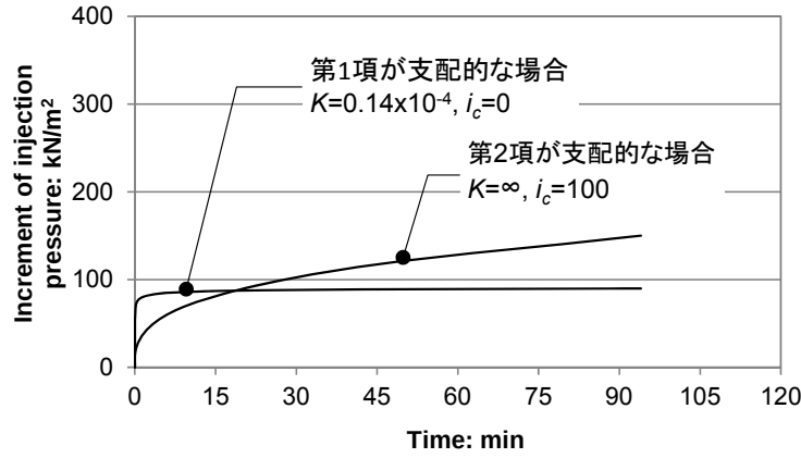
図-4.15 注入圧 P_0 の経時変化に対するパラメータの影響
