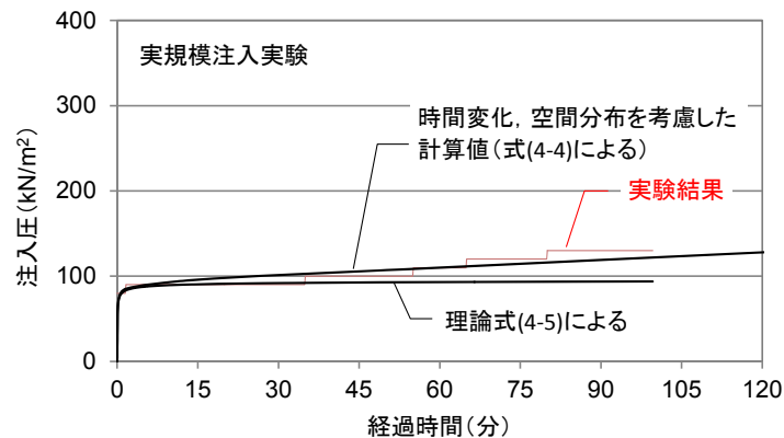
図-4.21 可塑性グラウトの粘性増加を考慮した注入圧力の計算値
