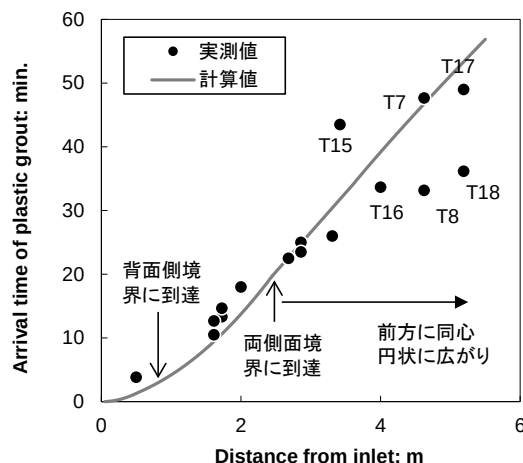
図-5.13 充填孔からの距離と到達時間の関係
