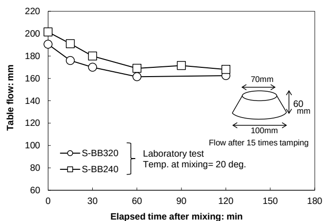
図-3.7 テーブルフロー値の経時変化（水ガラス系 BB）
