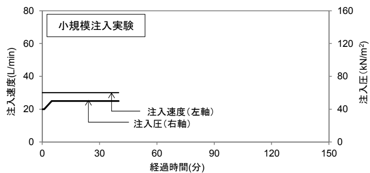
図-4.4 注入速度，注入圧の経時変化（小規模注入実験）
