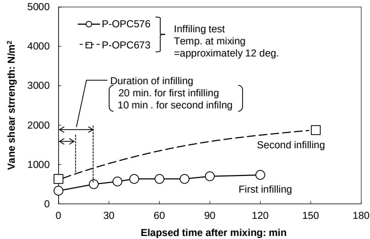
図-3.49 ベーンせん断抵抗の変化と圧入期間（段階的な空洞圧入）
