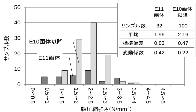
図-5.28 一軸圧縮強さ（28日材齢）の頻度分布
