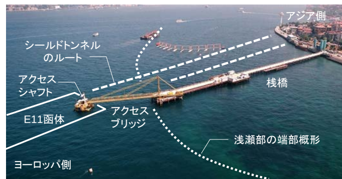
図-5.3 アジア側沈埋トンネル端部の航空写真
