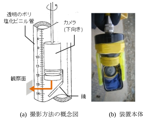
図-4.24 モニタリングカメラ
