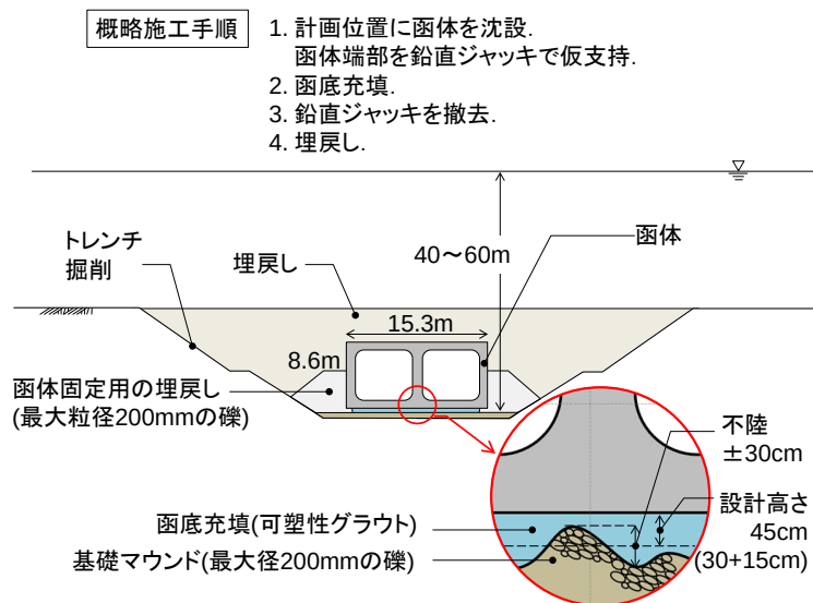
図-5.4 ポスボラス海峡横断鉄道プロジェクトにおける沈埋トンネルの断面（横断面図）
