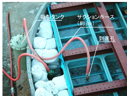
図-5.11 到達孔での排出確認実験の準備状況
