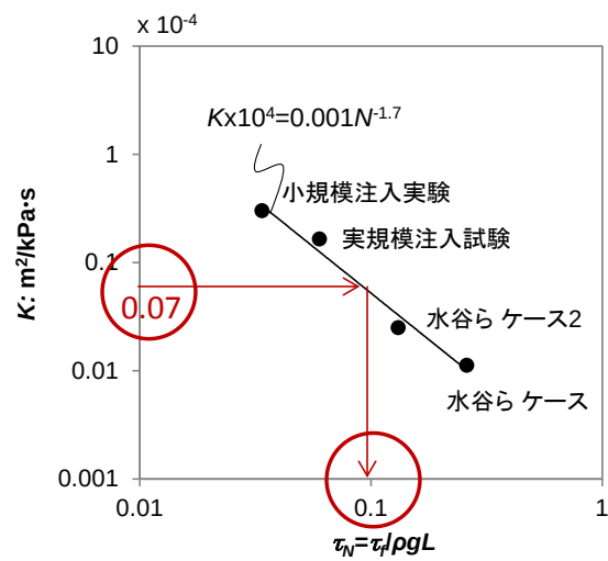
図-6.11 注入仕様に関する無次元量と注入係数の関係
