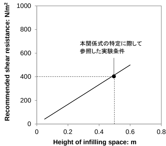
図-6.14 充填空間高さに応じて推奨される可塑性グラウトのせん断抵抗
