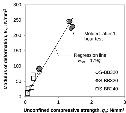
図-3.24 q_u と E_{50} の関係
