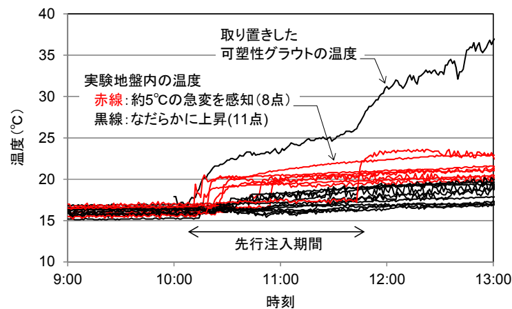
図-4.9 試験中に測定された温度変化（実規模注入実験）
