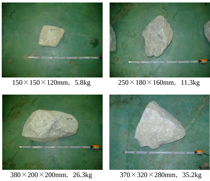
図-4.2 実験に用いた巨石（小規模注入実験）
