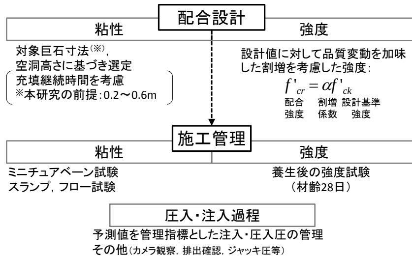
図-6.16 可塑性グラウトの配合設計と施工管理の体系
