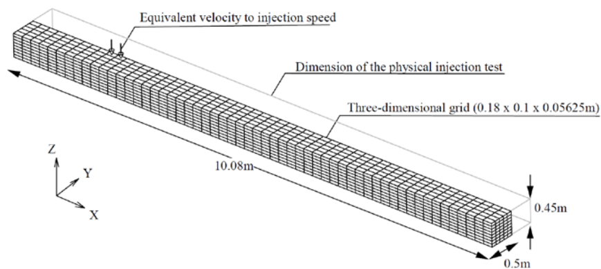
図-3.60 解析モデル（粘性変化の影響）
