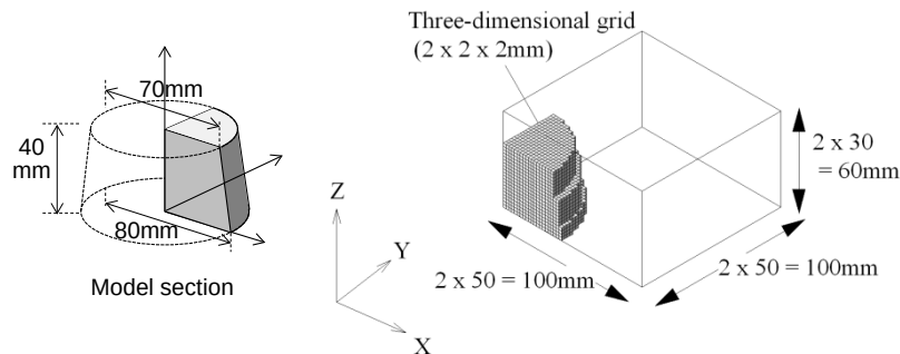
図-3A.3 解析モデル (セメントグラウトのフロー挙動)
