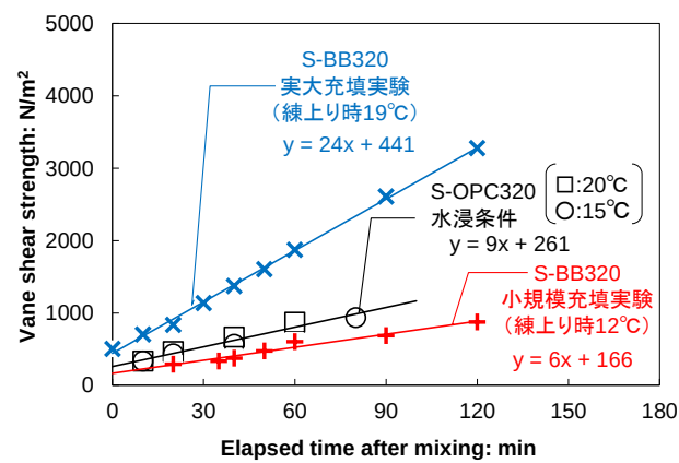
図-5.19 圧力算定で参照したベーンせん断強さの経時変化
