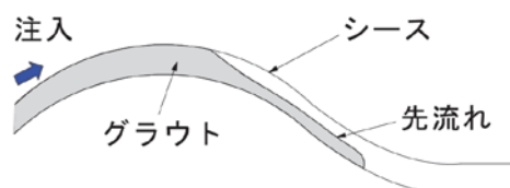
図-2.5 PC グラウトの注入状況と先流れ
