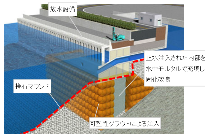
図-4.1 捨石マウンドにおける止水注入（文献1に加筆）
