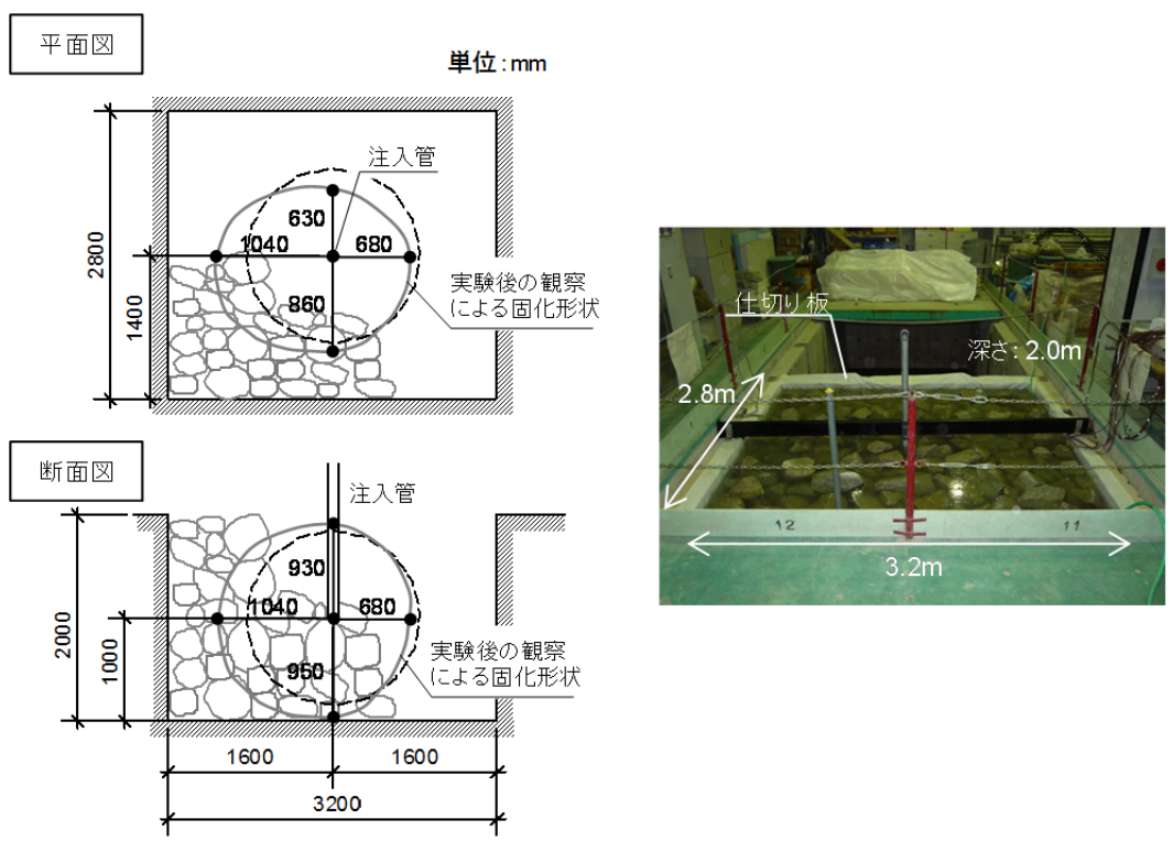
図-4.3 実験概要（小規模注入実験）
