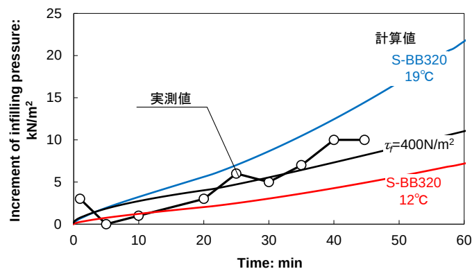
図-5.21 充填圧の変化
