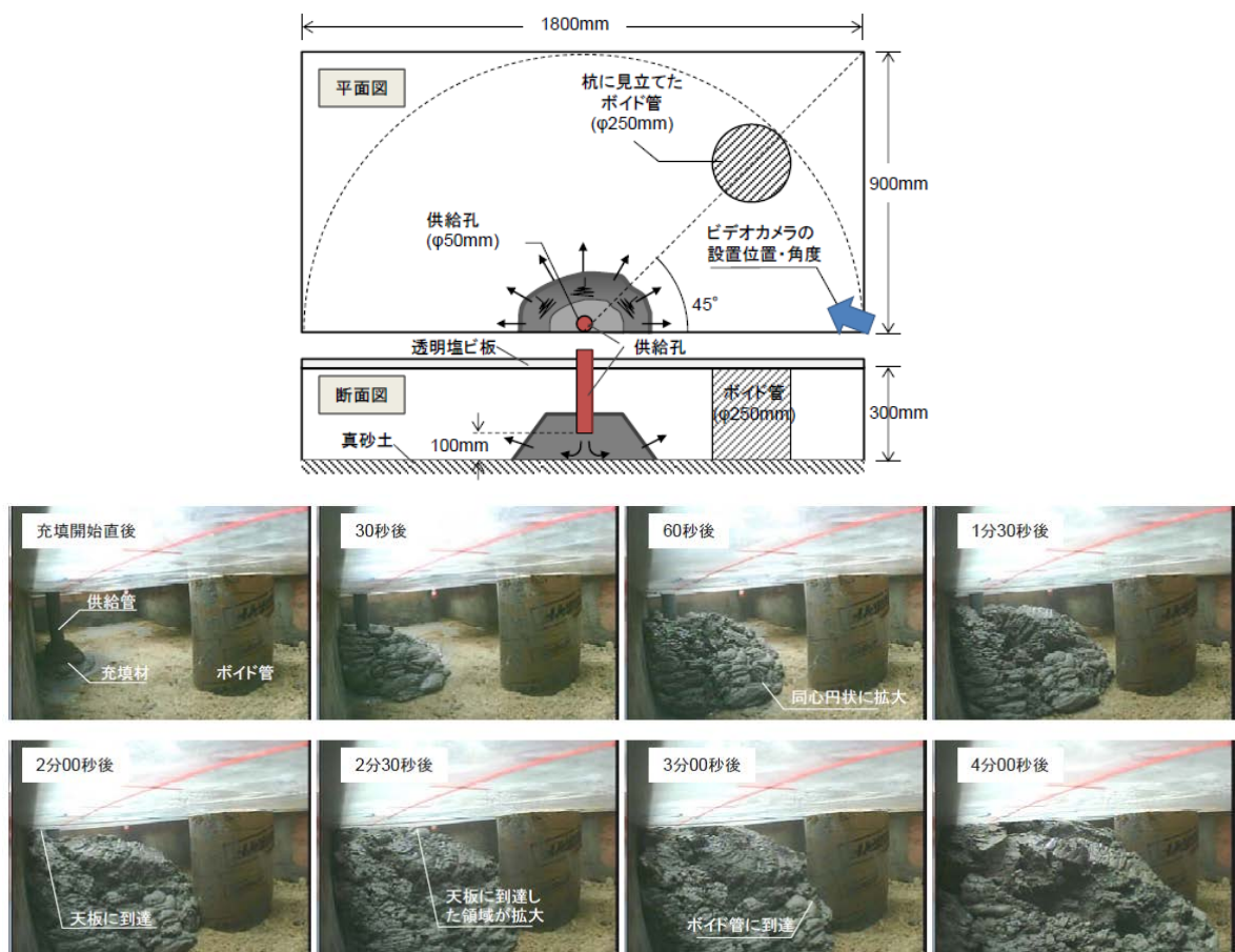
図-2.28 隔離堤構築を想定した充填状況の確認
