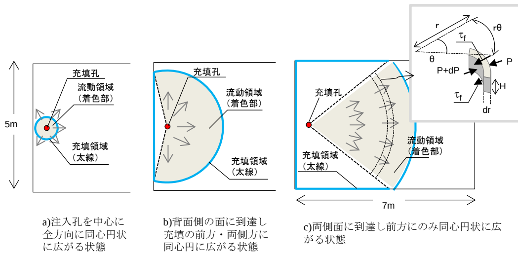
図-5.14 充填領域・流動領域の想定（平面図）
