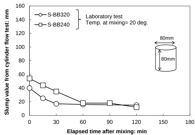
図-3.9 シリンダーフロー試験で測定したスランプ値の経時変化（水ガラス系 BB）
