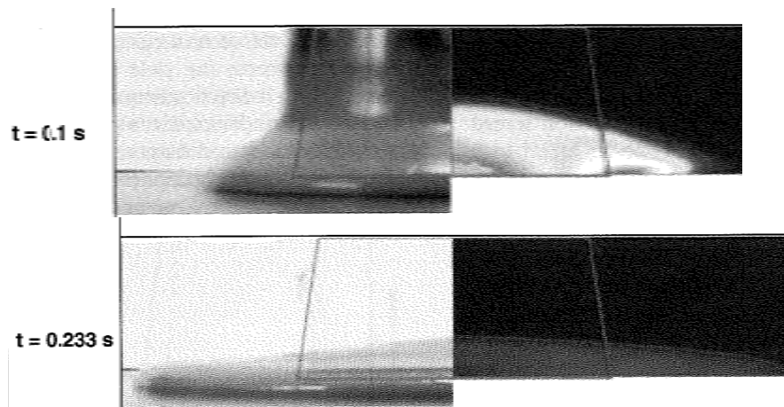
図-2.4 セメントミルクの流動と解析結果の比較
