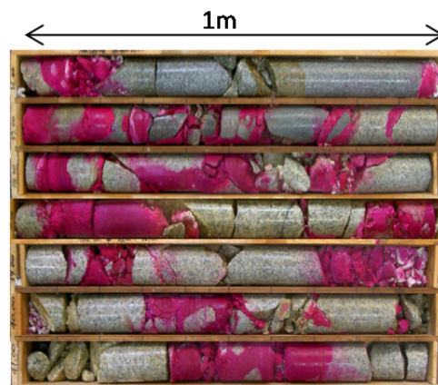
図-4.34 チェックボーリングで確認した改良状況例
