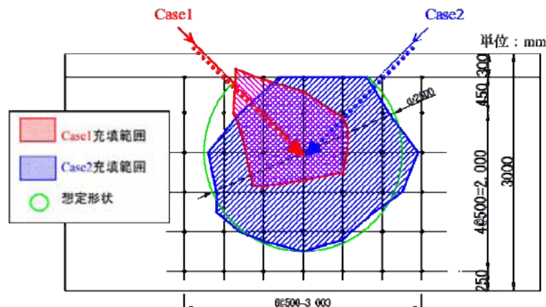
図-6.7 巨石地盤を対象とした可塑性グラウトの注入実験結果（注入範囲）
