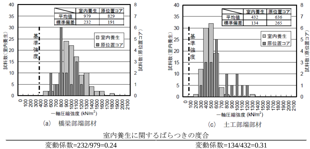
図-5.30 過去の事例における一軸圧縮強さの記録
