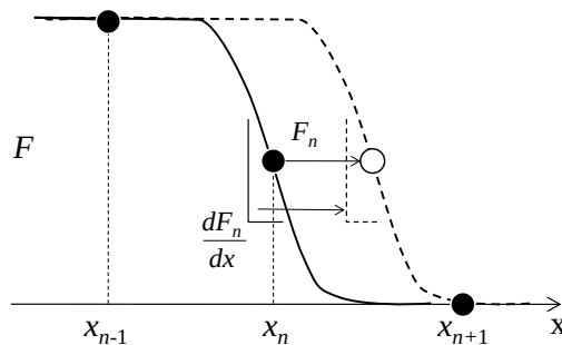
図-3A.1 CIP法のイメージ
