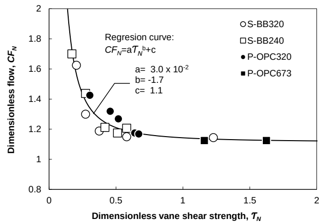
図-3.29 無次元量 T_N と CF_N の関係
