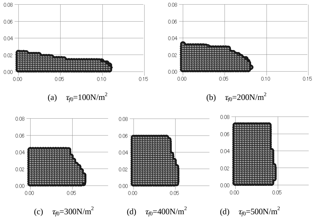
図-3.37 解析で再現したスランプ形状 (0.2 秒後)
