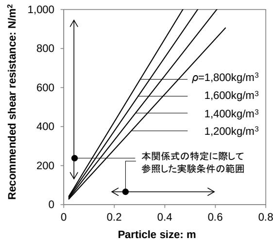
図-6.12 代表粒径に応じて推奨される可塑性グラウトのせん断抵抗
