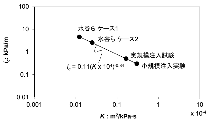
図-4.19 注入係数と降伏圧力勾配の関係
