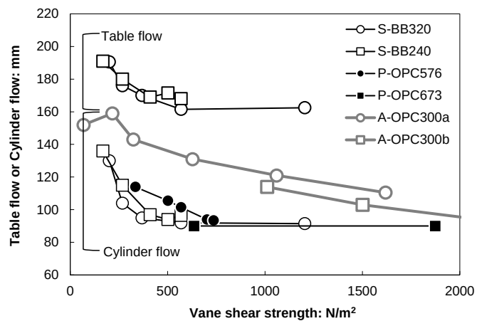
図-3.27 ベーンせん断抵抗とフロー値の関係（水ガラス系 BB，高分子系 OPC）
