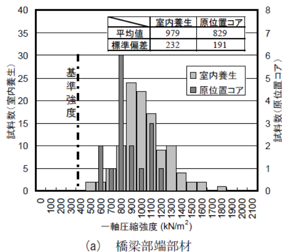
図-2.22 廃坑埋め戻しでの端部充填における品質管理結果
