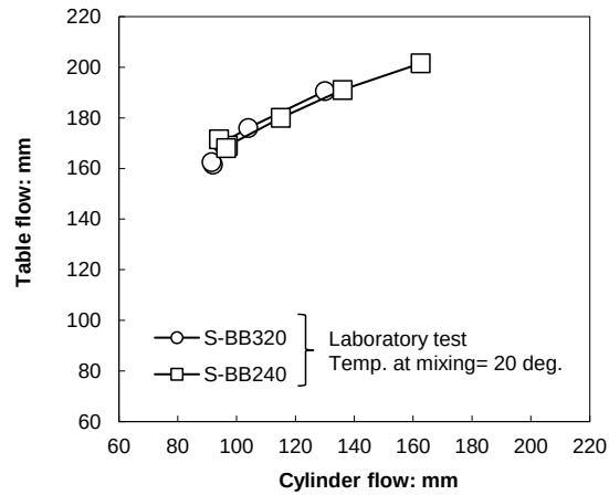
図-3.25 シリンダーフロー値とテーブルフロー値の関係（水ガラス系 BB）
