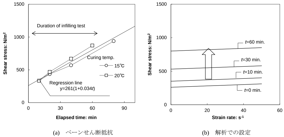
図-3.61 解析に反映したベーンせん断抵抗の変化
