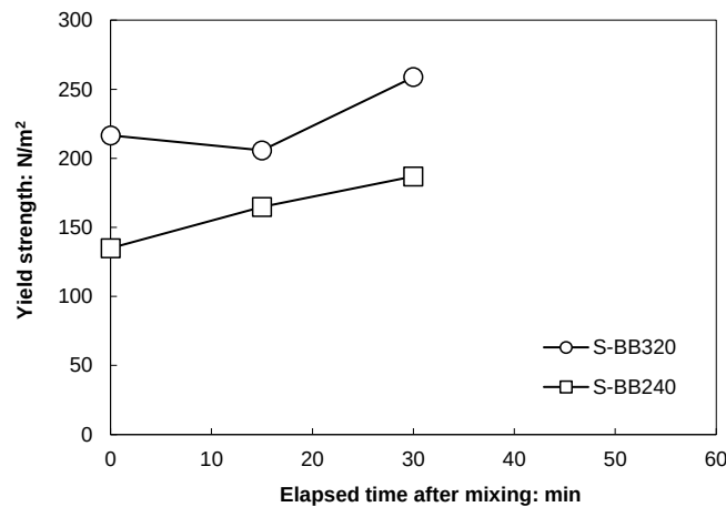
図-3.19 降伏応力の経時変化 (S-BB320, S-BB240)
