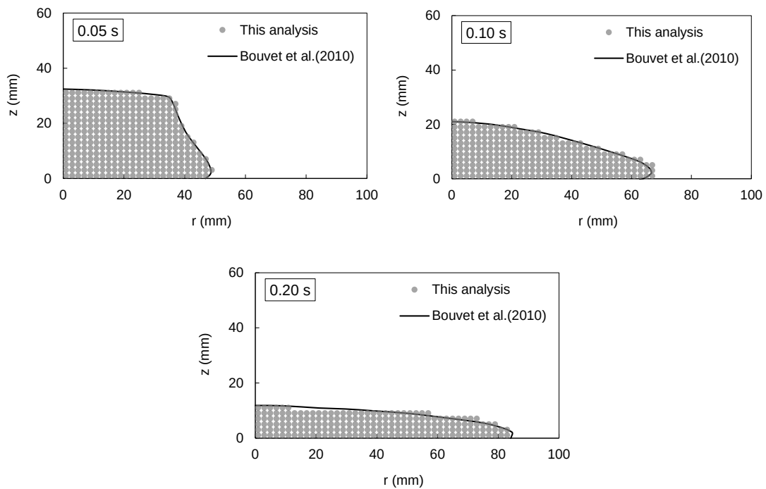
図-3A.4 解析結果（セメントグラウトのフロー挙動）
