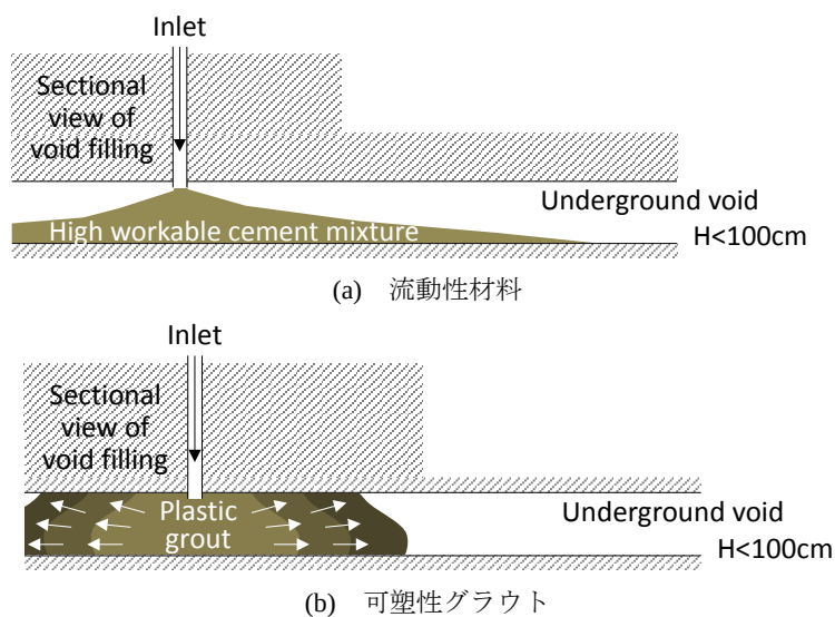
図-2.15 流動イメージの比較
