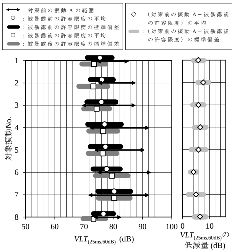
図 7.5.1 対策前の振動 A 暴露後の許容限度
