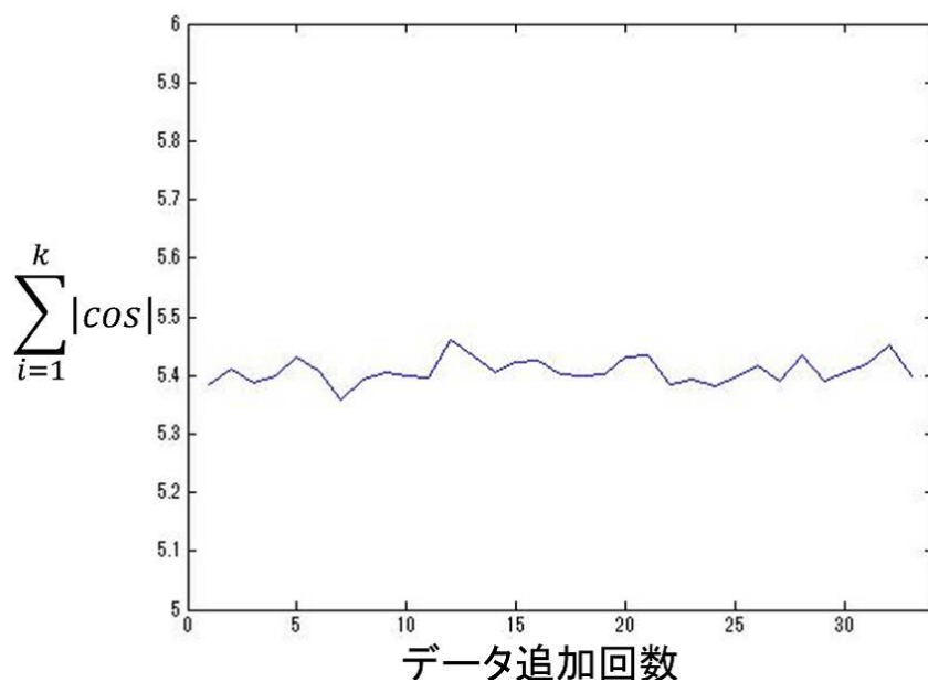
図 5.2 データ追加に基づく独立話題分析を LA Times に適用して抽出した話題と、全てのデータを使用して抽出した話題とのコサインの絶対値の総和. 初期データとして LA Times のデータの 50% を使用し、残ったデータを追加データとして 100 ずつ追加していった. 横軸はデータの追加回数, 縦軸は全てのデータを使用して抽出した話題とのコサインの絶対値の総和であり, 最大値は話題数が 6 であるため 6 となる.
