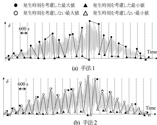
図2 最大値最小値波形の模式図 ( \hat{D} )
