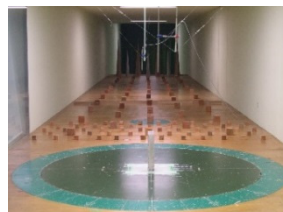
図7 風洞実験概要
