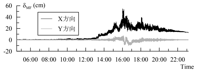
図12 免震層変位の時刻歴波形 ( d\alpha_y=0.02, fT=5.0\text{s} , 第1波)
