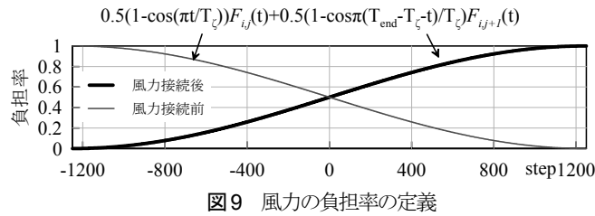
図9 風力の負担率の定義
