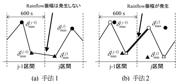
図3 提案手法1と2の振幅の比較
