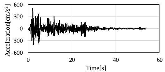
a) El Centro NS
