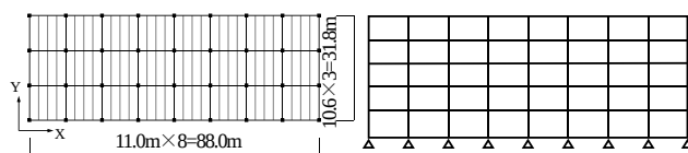
図 2 基準階伏図
