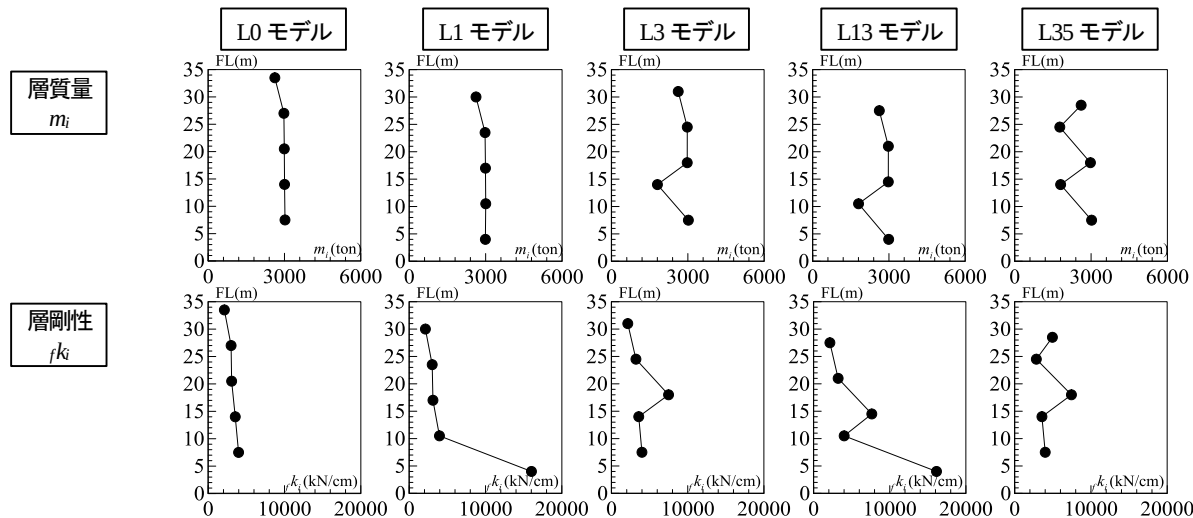
図 4 層質量 m_i と層剛性 f_{k_i}
