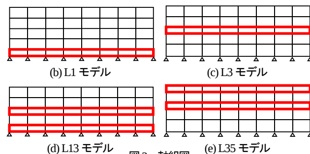
図 3 軸組図
