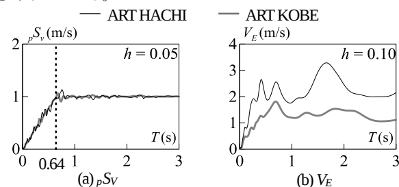
図 1 擬似速度応答スペクトル pS_v と エネルギー Spektral V_E
