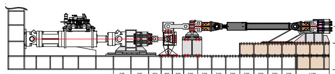
図3 粘性ダンパーセットアップ図
