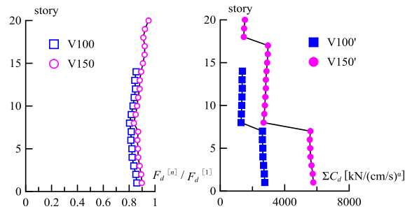
附図 1 特性値低下率
