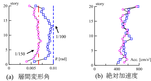
図 9 時刻歴応答結果 (ART HACHI 入力時)
