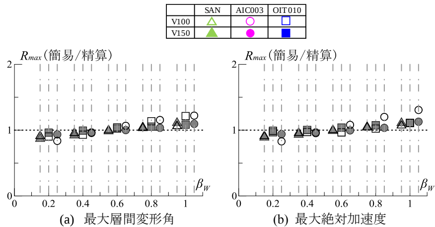
図 14 エネルギー低減係数を用いた簡易手法と精算手法の比較
