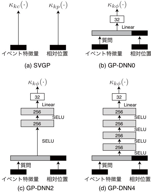
図 2 実験における SVGP および GP-DNN の特徴抽出の比較
