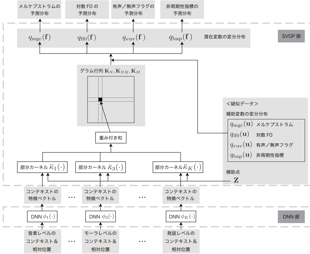
図 1 GP-DNN ハイブリッドモデルに基づく音響モデリングの枠組み
