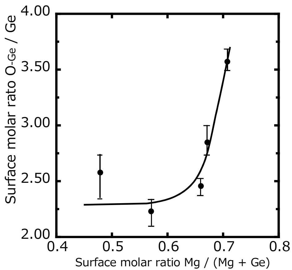
Fig. 3.18 Ge-タルクにおける表面原子比 \text{Mg} / (\text{Mg} + \text{Ge}) が \text{O}_{\text{peak1}} / \text{Ge} に及ぼす影響
