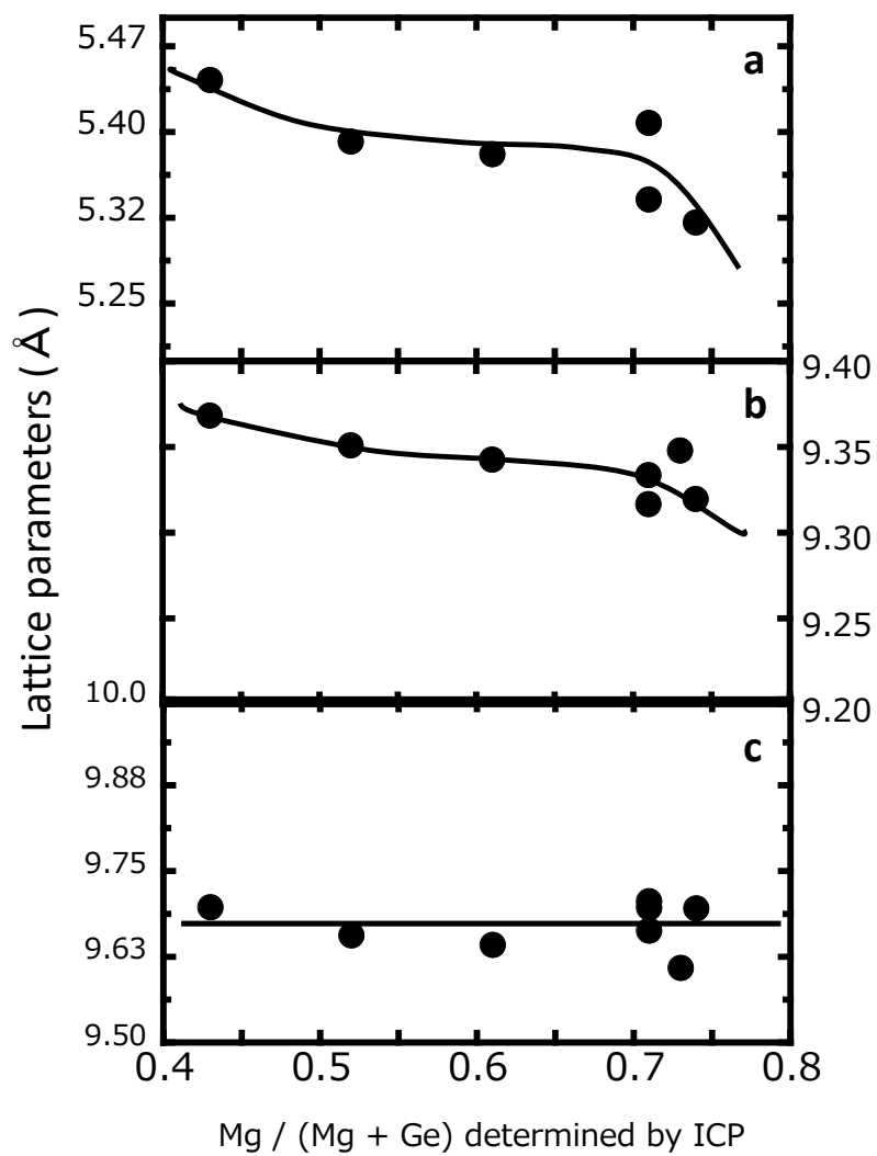
Fig.3.17 合成した Ge-タルクにおける ICP 測定による バルクの原子比 \text{Mg} / (\text{Mg} + \text{Ge}) が格子定数に及ぼす影響
