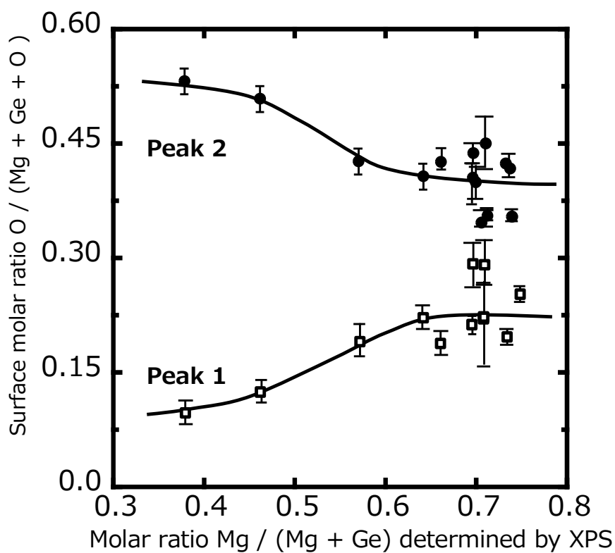
Fig. 3.16 Ge-タルクにおける表面原子比 \text{Mg} / (\text{Mg} + \text{Ge}) が \text{O} / (\text{Mg} + \text{Ge} + \text{O}) に及ぼす影響
