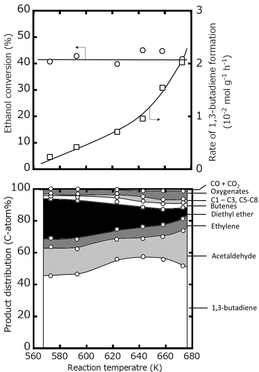
Fig. 2.13 Zn/タルクを触媒としたエタノール転化反応における反応温度が 1,3-ブタジエンの生成速度と生成物分布に及ぼす影響 エタノール分圧: 101.3 kPa
