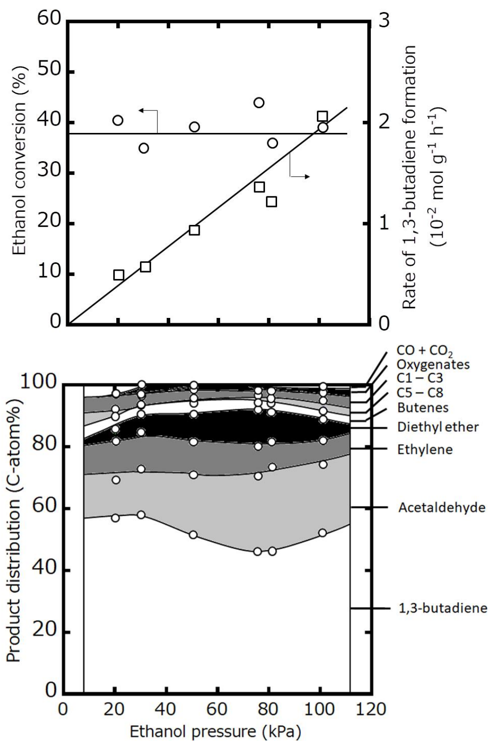
Fig. 2.14 Zn/タルクを触媒としたエタノール転化反応におけるエタノール分圧が 1,3-ブタジエンの生成速度と生成物分布に及ぼす影響 反応温度: 673K
