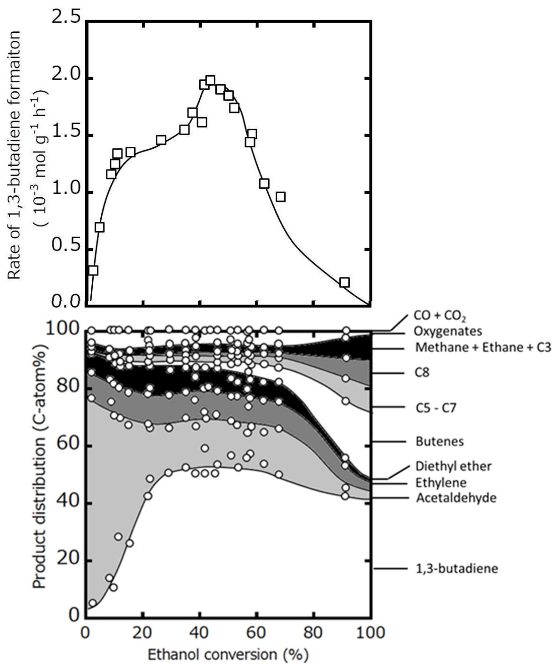
Fig. 2.6 Zn/タルクを触媒としたエタノール転化反応におけるエタノール転化率が 1,3-ブタジエンの生成速度と生成物分布に及ぼす影響 反応温度: 673K, エタノール分圧: 101.3 kPa
