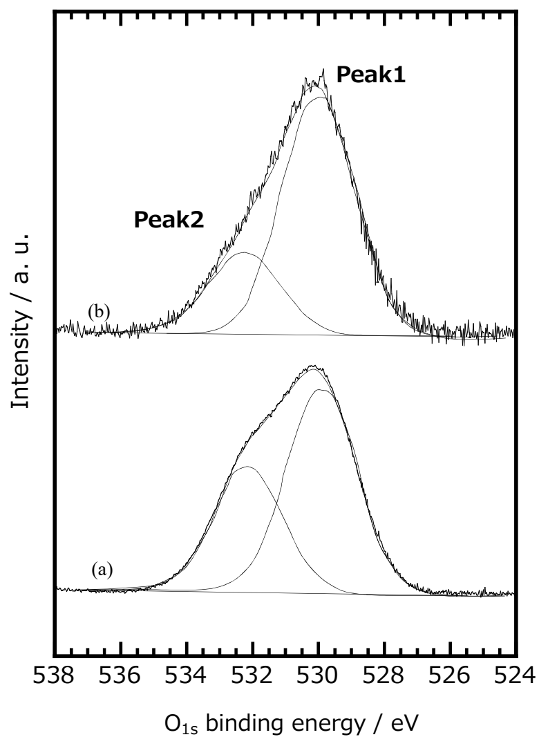
Fig. 2.4 加熱して水熱合成した MgO ht と加熱した MgO calc における O 1s 軌道の XPS スペクトル
