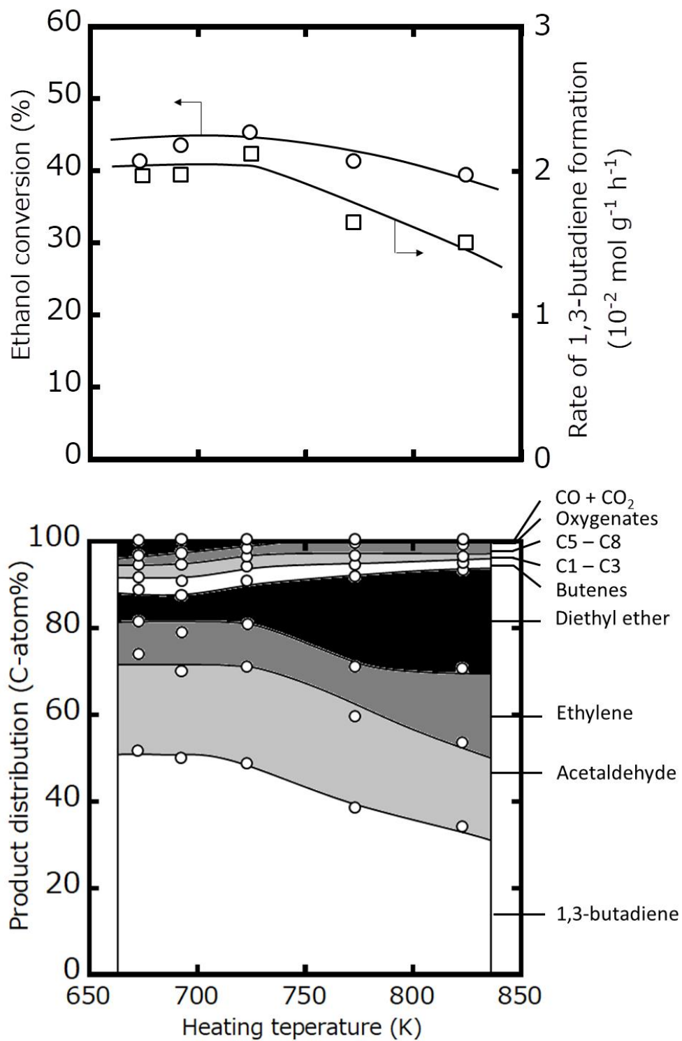
Fig. 2.11 Zn/タルクを触媒としたエタノール転化反応における反応温度が 1,3-ブタジエンの生成速度と生成物分布に及ぼす影響 反応温度: 673K, エタノール分圧: 101.3 kPa
