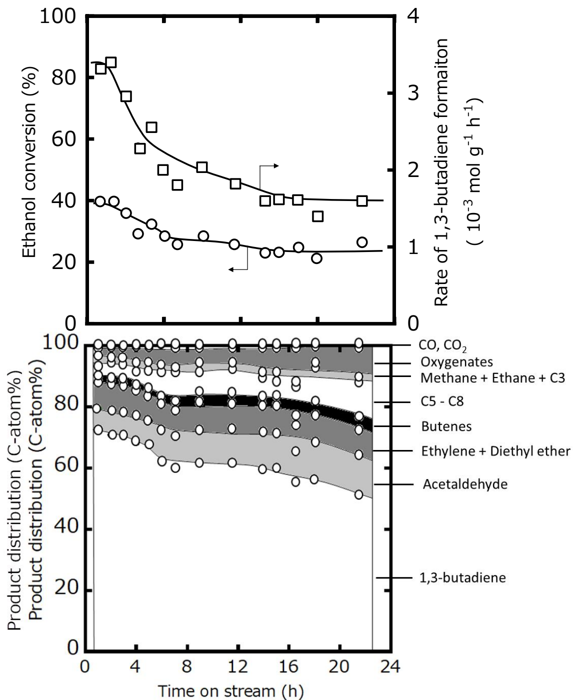
Fig.3.23 流通時間に対するエタノール転化反応
