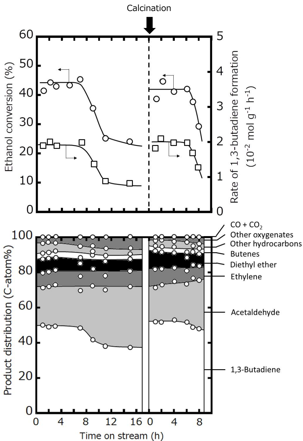
Fig. 2.15 Zn/タルクを触媒としたエタノール転化反応における流通時間が1,3-ブタジエンの生成速度と生成物分布に及ぼす影響 反応温度: 673K, エタノール分圧: 101.3 kPa Calcination: N 2 / O 2 = 90 / 10 (mol / mol), 室温から 693 K まで昇温, 693 K , 5 h で加熱
