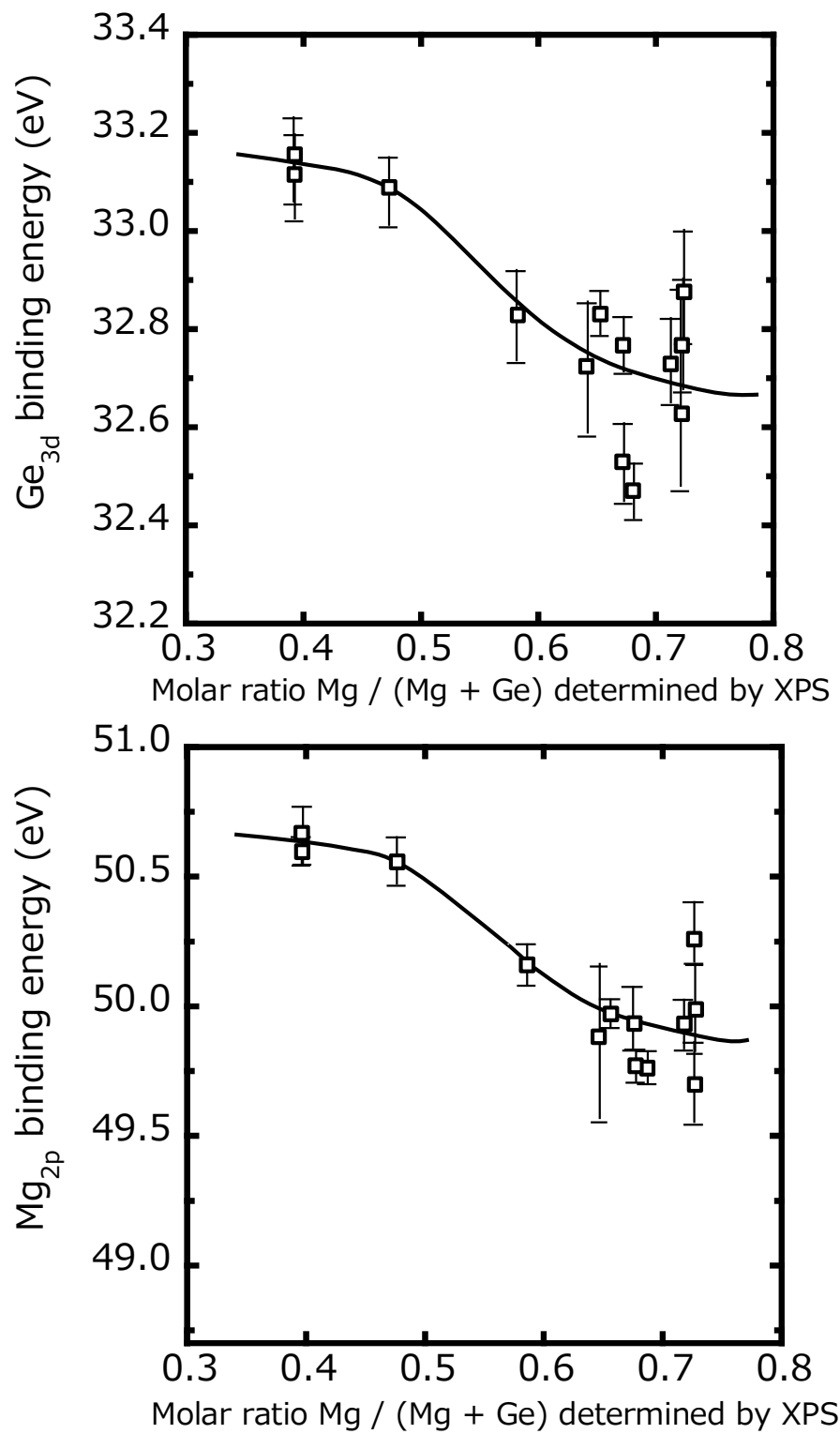
Fig. 3.14 Ge-タルクにおける表面原子比 \text{Mg} / (\text{Mg} + \text{Ge}) が \text{Mg}_{2p} と \text{Ge}_{3d} 軌道の電子の結合エネルギーに及ぼす影響
