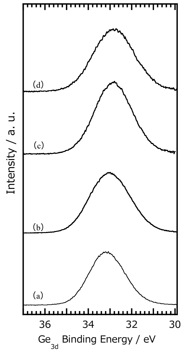
Fig. 3.11 表面原子比 \text{Mg} / (\text{Mg} + \text{Ge}) が 0.38 から 0.67 の範囲を示す Ge-タルクにおけ \text{Mg}_{2p} と \text{Ge}_{3ds} 軌道の XPS スペクトル
