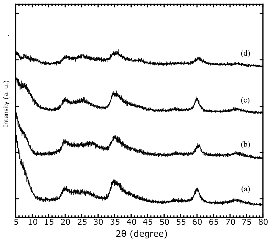
Fig. 2.9 原子比 \text{Mg} / (\text{Mg} + \text{Si}) が異なる Zn/タルクの XRD パターン
