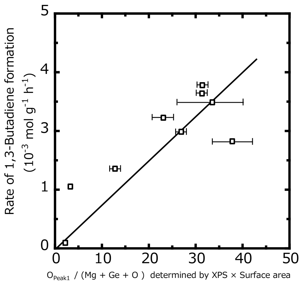
Fig. 3.22 Ge-タルクにおける M 原子近傍の酸素原子数に相当する \text{Mg} / (\text{Mg} + \text{Ge}) \times 比表面積がエタノールから 1,3-ブタジエンの生成速度に及ぼす影響 反応温度: 673K, エタノール分圧: 101.3 kPa
