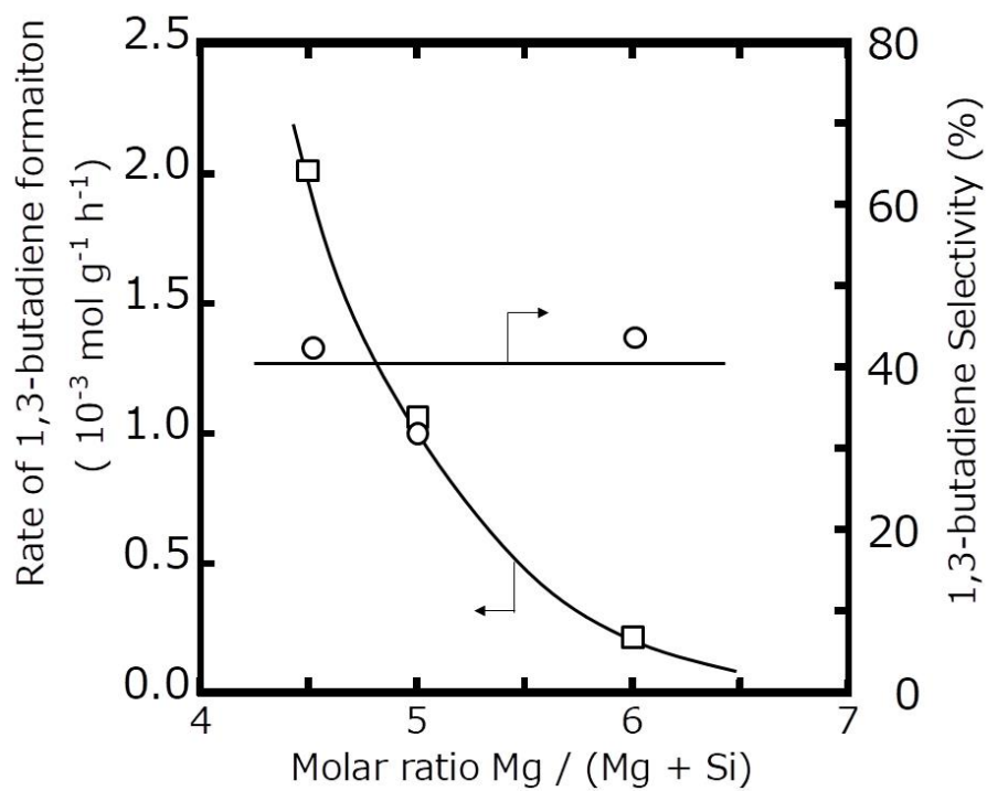
Fig. 2.10 Zn/タルクの原子比 \text{Mg} / (\text{Mg} + \text{Si}) が 1,3-ブタジエンの生成速度と選択率に及ぼす影響
