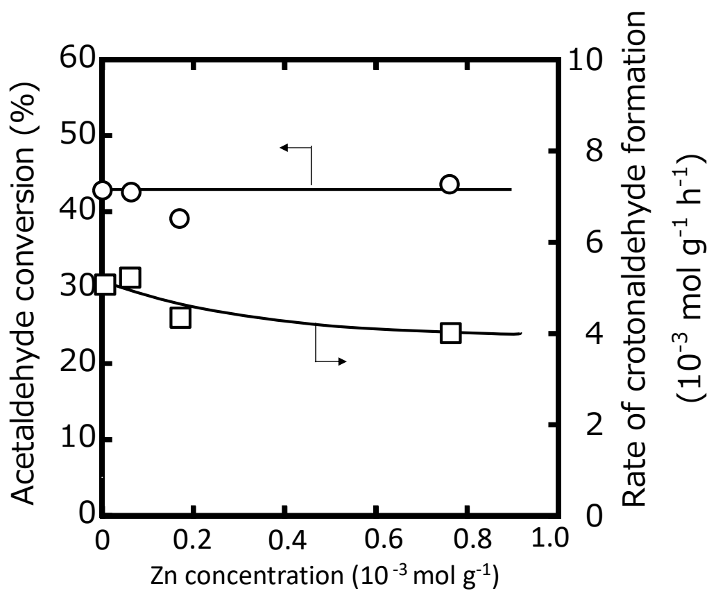
Fig. 2.8 Zn/タルクの Zn 含有量がアセトアルデヒドからのクロトンアルデヒドの生成速度と転化率に及ぼす影響
