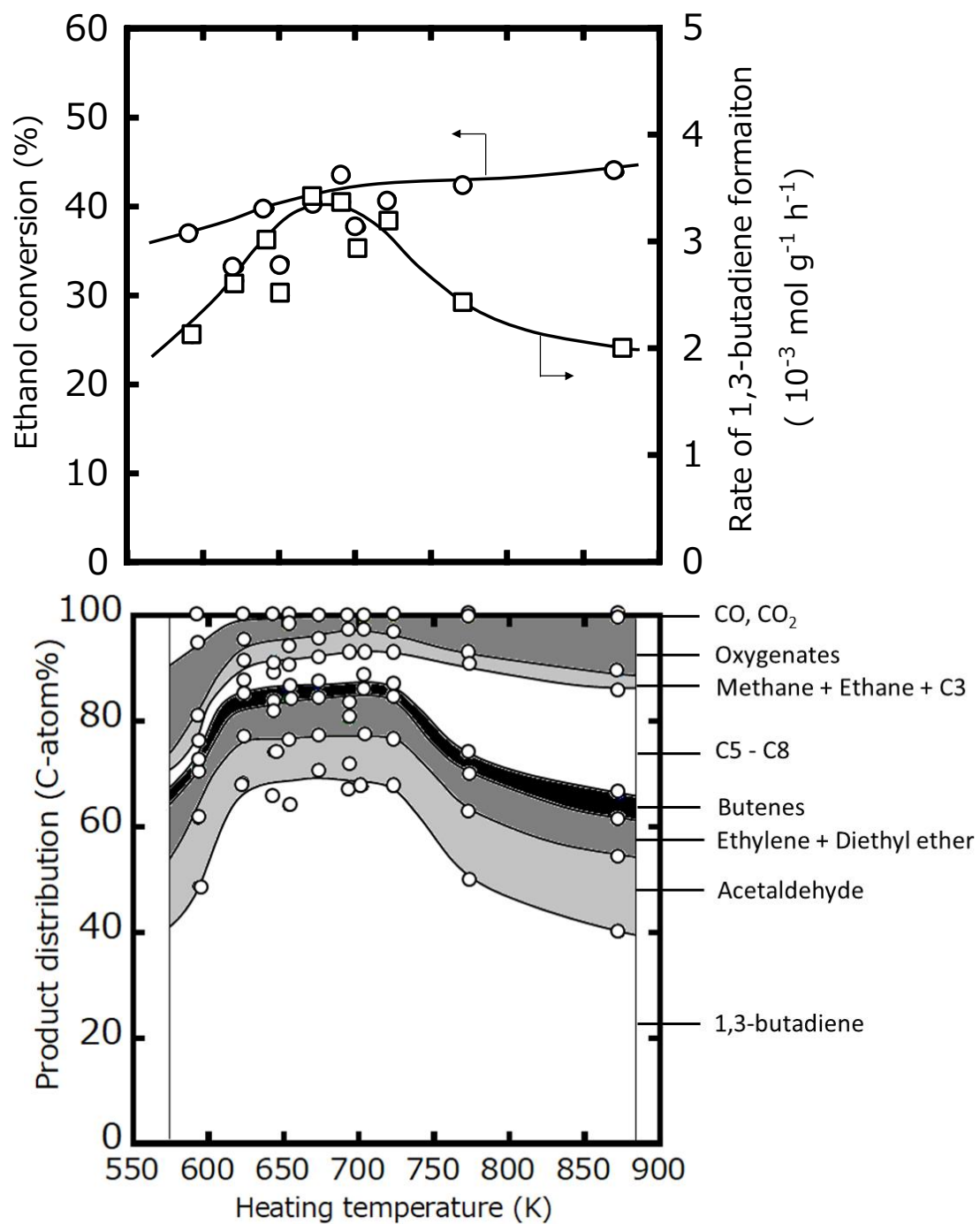
Fig. 3.6 加熱温度が 1,3-ブタジエンの生成速度と生成物分布に及ぼす影響
