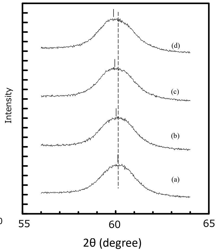
Fig. 2.17 Zn 含有量が異なる Zn/タルクの XRD パターン Zn 含有量 (a) 0, (b) 2.52 \times 10^{-4} , (c) 5.68 \times 10^{-4} , (d) 9.57 \times 10^{-4} \text{ mol g}^{-1}
