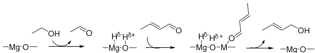
Scheme 1-2 MgO による水素転移反応 (1)
