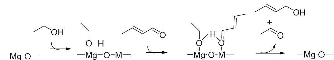
Scheme 1-3 MgO による水素転移反応 (2)
