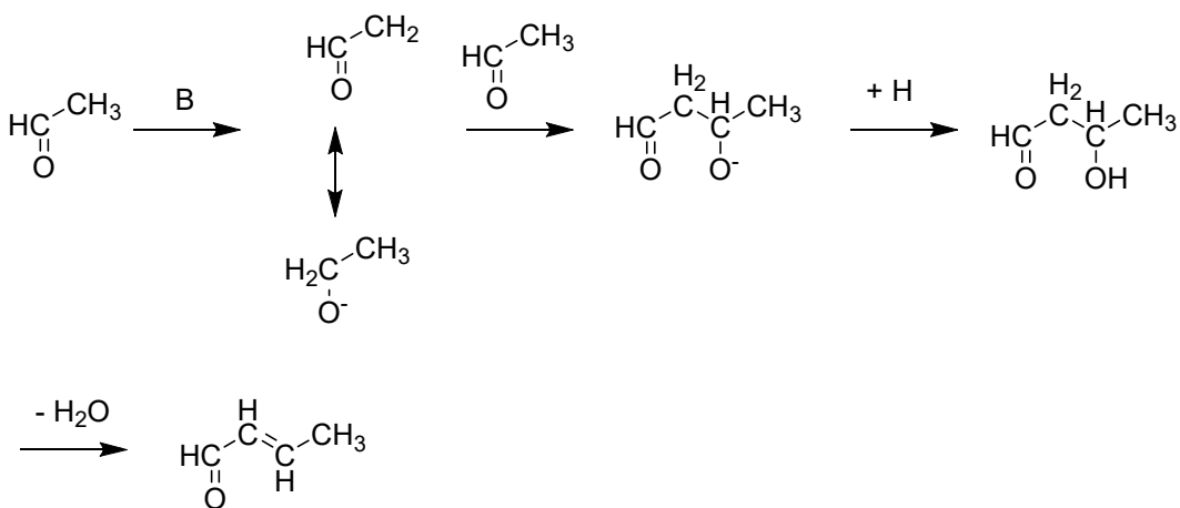
Scheme 1-1 塩基触媒によるアセトアルデヒドのアルドール縮合反応
