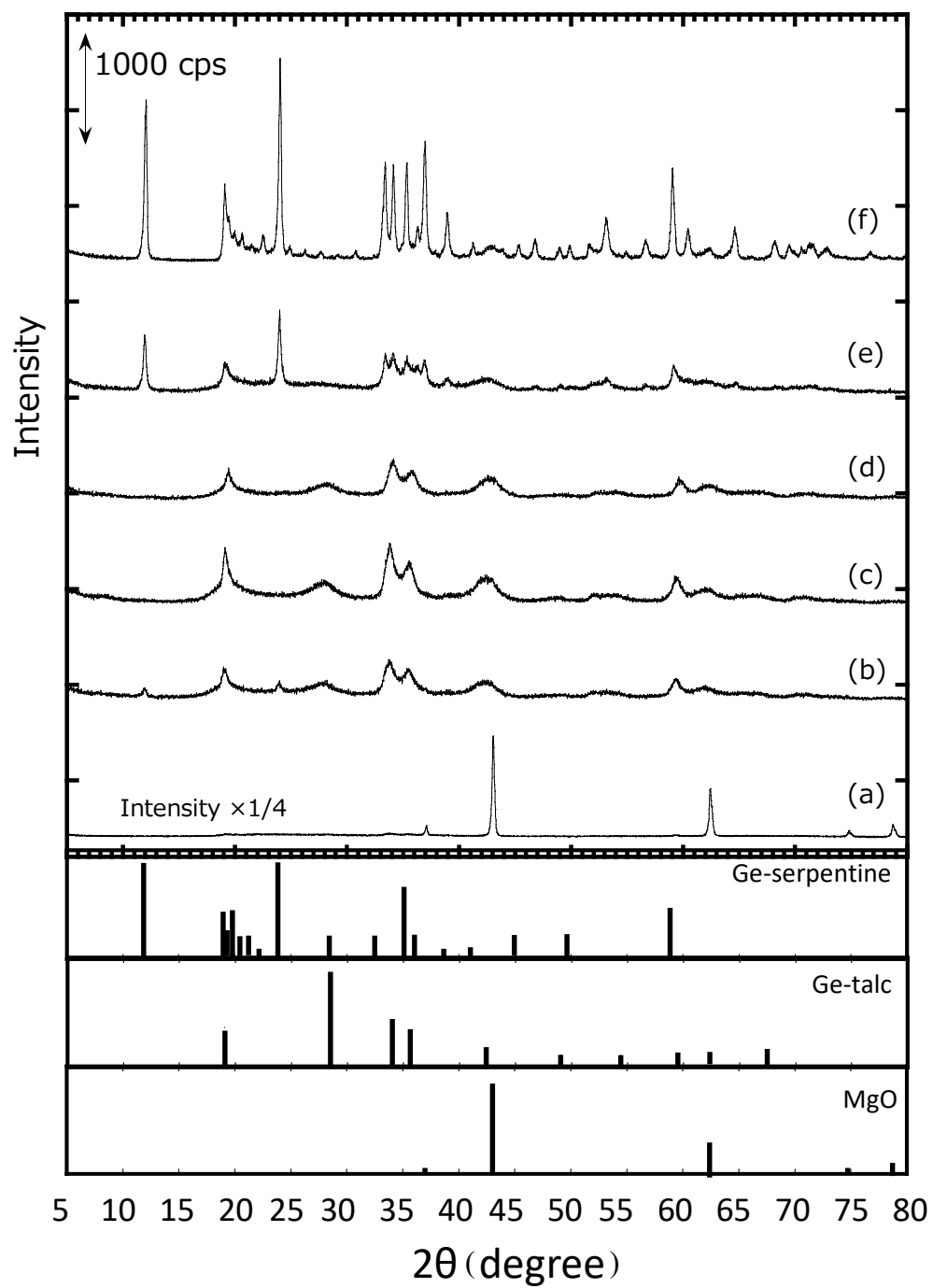
Fig. 3.1 水熱合成温度が Ge-タルク形成に及ぼす影響 水熱合成温度 (a) 333K, (b) 348K, (c) 353K, (d) 358K, (e) 363K, (f) 473K
