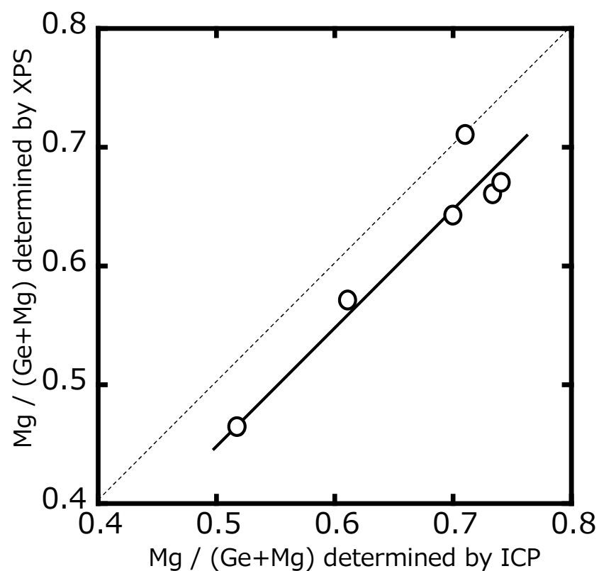
Fig.3.9 合成した Ge-タルクにおける ICP 測定によるバルク原子比 \text{Mg} / (\text{Mg} + \text{Ge}) と XPS 測定による表面原子比 \text{Mg} / (\text{Mg} + \text{Ge}) の関係
