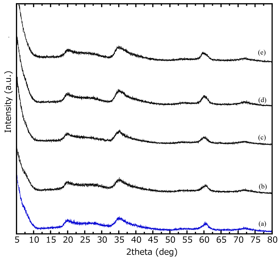
Fig. 2.5 合成したタルクと第三金属を含有したタルクの XRD パターン
