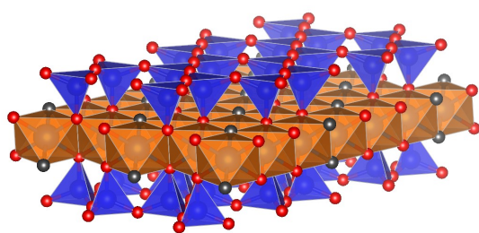
タルク Mg 3 Si 4 O 10 (OH) 2
