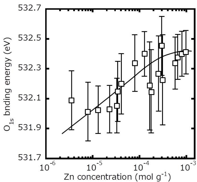
Fig. 2.20 Zn/タルクの Zn 含有量が O 1s 軌道の電子の結合エネルギーに及ぼす影響
