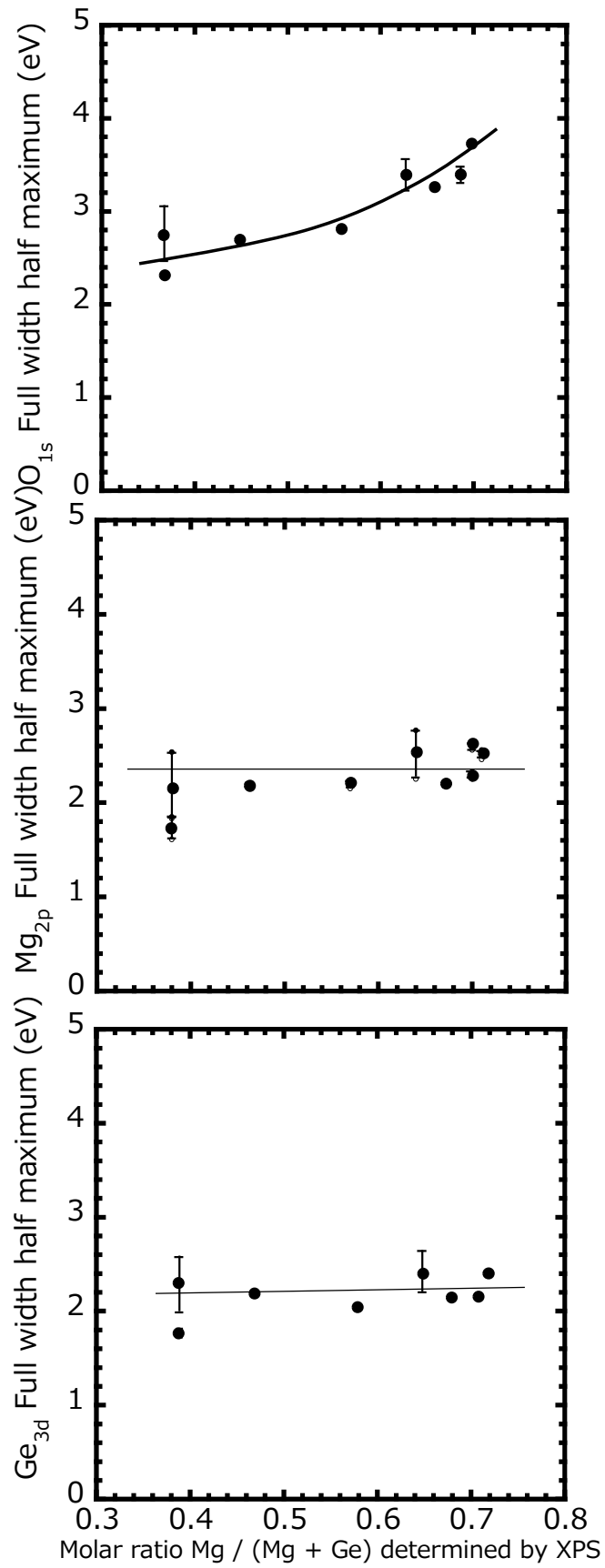
Fig. 3.13 合成した Ge-タルクにおける表面原子比 \text{Mg} / (\text{Mg} + \text{Ge}) が \text{Mg}_{2p} と \text{Ge}_{3d} , \text{O}_{1s} 軌道の半値幅に及ぼす影響
