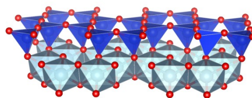
サーペンタイン Mg 3 Si 2 O 5 (OH) 4
