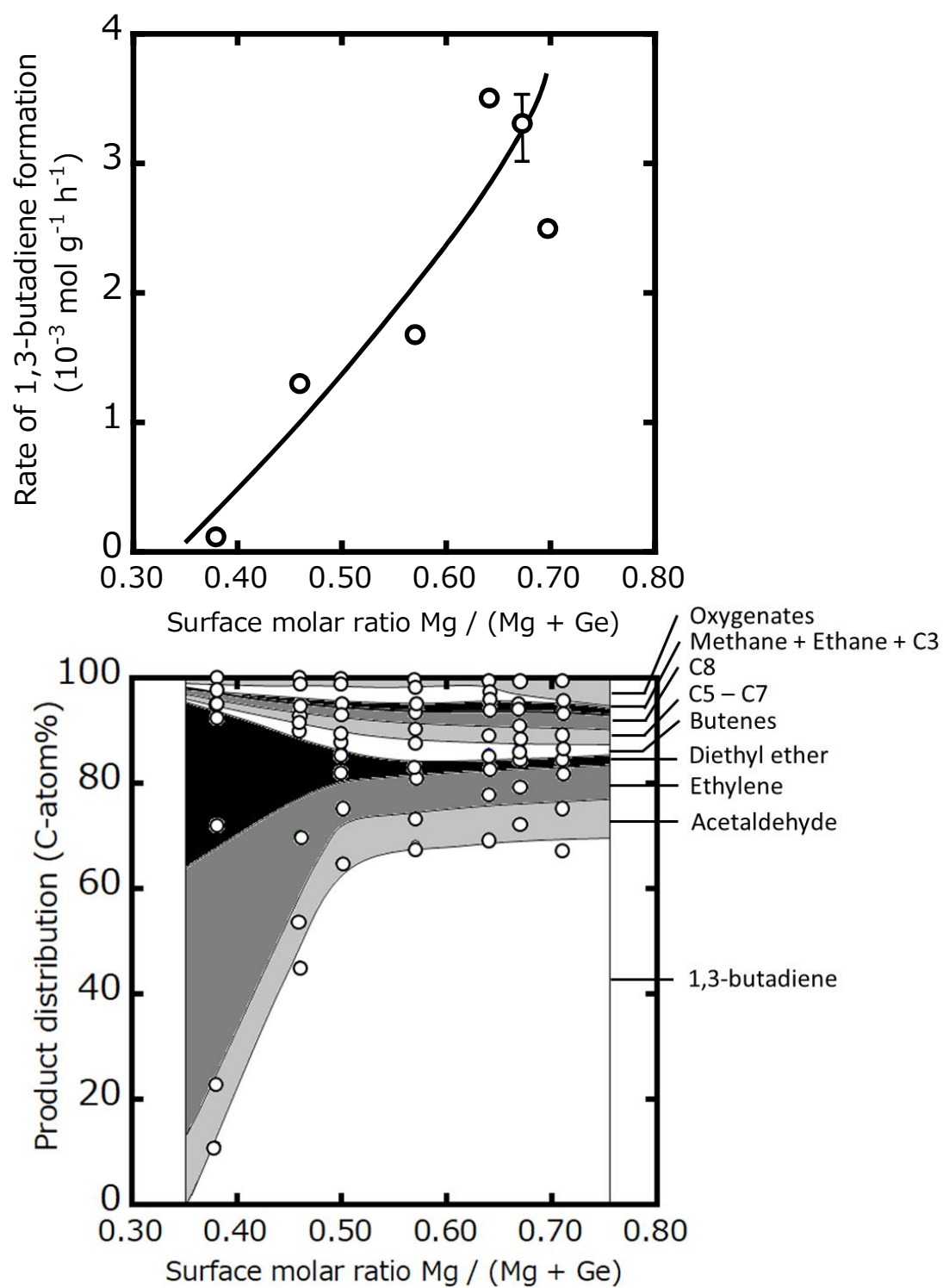
Fig. 3.21 合成した Ge-タルクにおける表面原子比 \text{Mg} / (\text{Mg} + \text{Ge}) がエタノールからの 1,3-ブタジエンの生成速度と生成物分布に及ぼす影響 反応温度: 673K, エタノール分圧: 101.3 kPa
