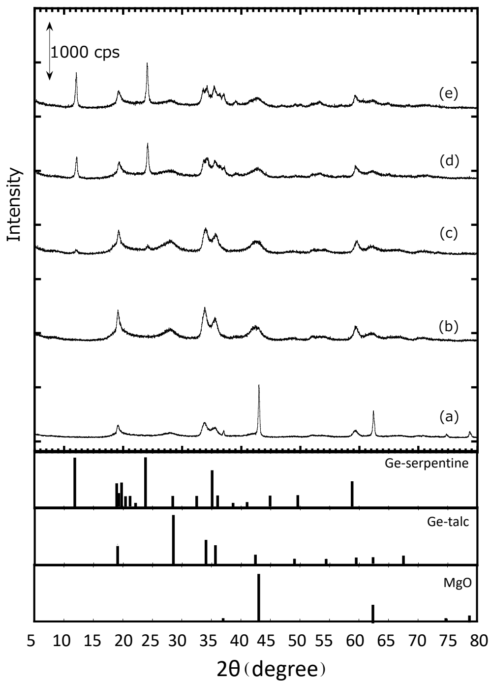
Fig. 3.2 水熱合成時間が Ge-タルク形成に及ぼす影響
