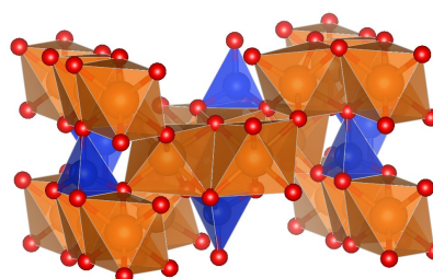
フォルステライト Mg 2 SiO 4
