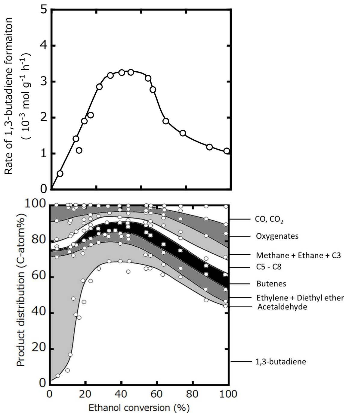
Fig. 3.20 合成した Ge-タルクにおけるエタノール転化率が 1,3-ブタジエンの生成速度と生成物分布に及ぼす影響
