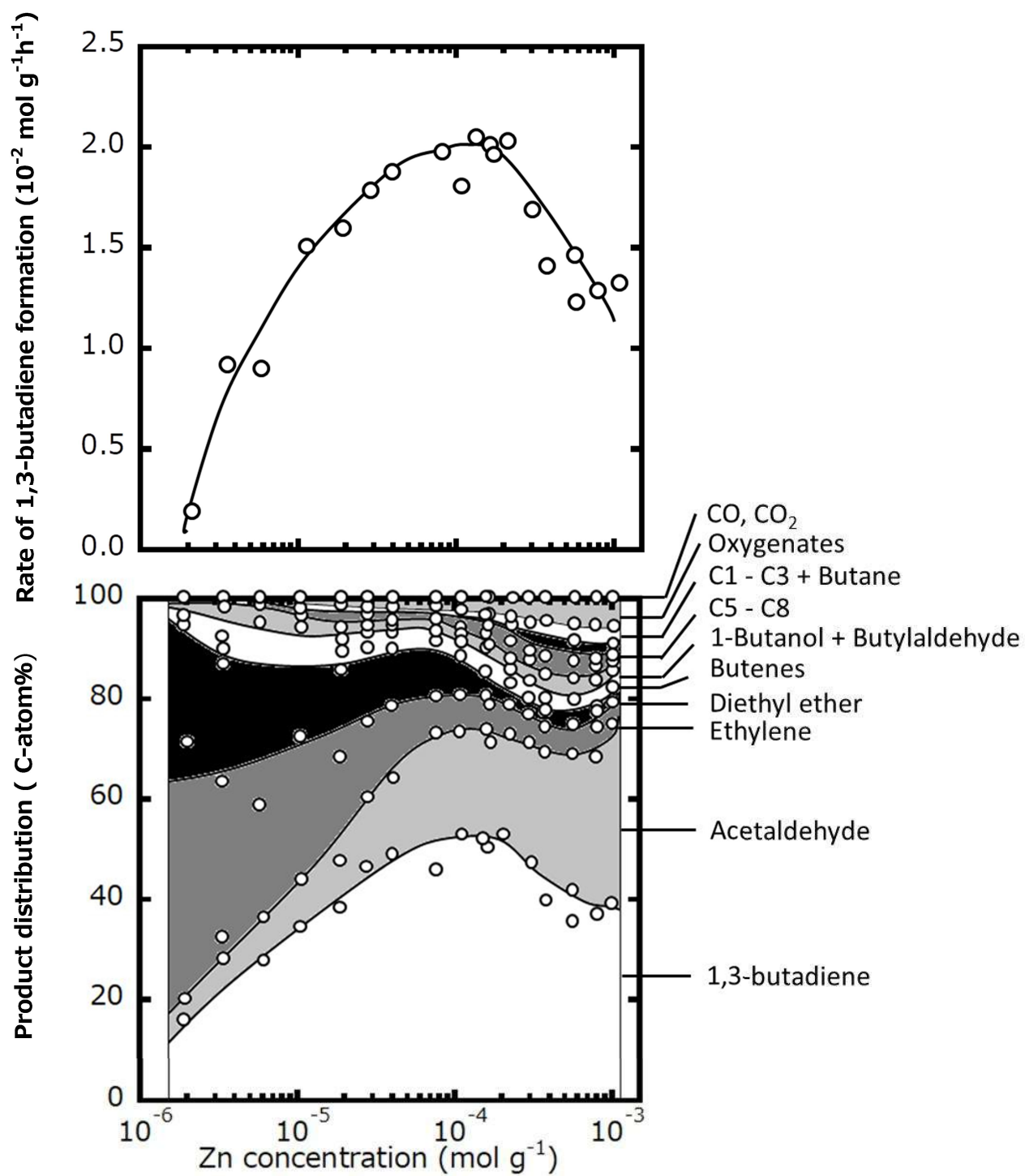
Fig. 2.7 Zn/タルクの Zn 含有量がエタノールからの 1,3-ブタジエンの生成速度と生成物分布に及ぼす影響
