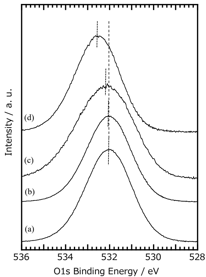
Fig. 2.19 Zn 含有量が異なる Zn/タルクの XPS スペクトル Zn 含有量 (a) 0, (b) 2.52 \times 10^{-4} , (c) 5.68 \times 10^{-4} , (d) 9.57 \times 10^{-4} \text{ mol g}^{-1}
