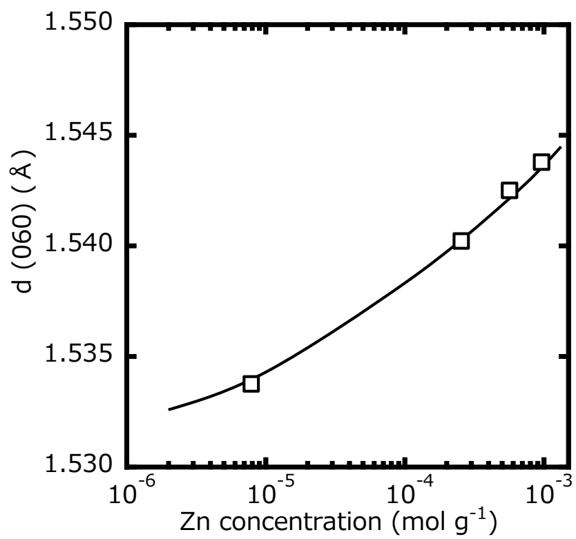
Fig. 2.18 合成したタルクにおける Zn 含有量と (060) 面の面間隔の関係
