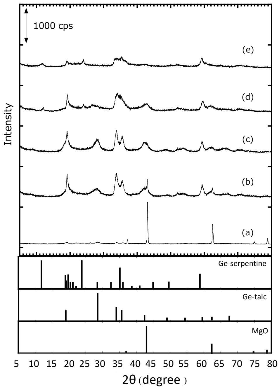
Fig. 3.3 原料である MgO の比表面積が Ge-タルク形成に及ぼす影響
