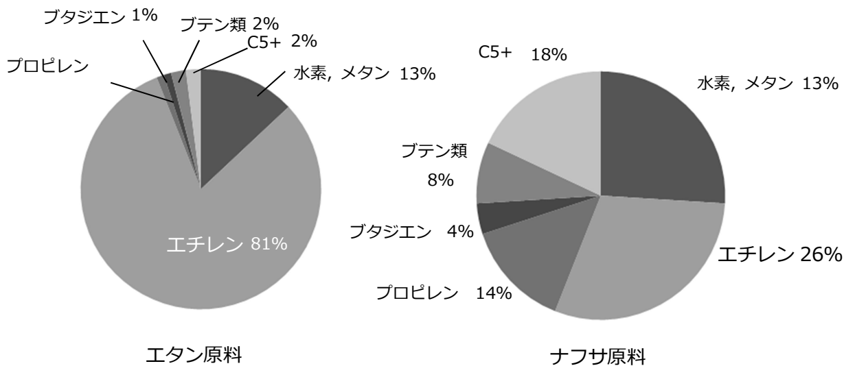
Fig. 1.1 熱分解における原料別の生成物分布 [10]
