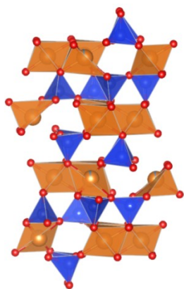
タルク Mg 3 Si 4 O 10 (OH) 2
