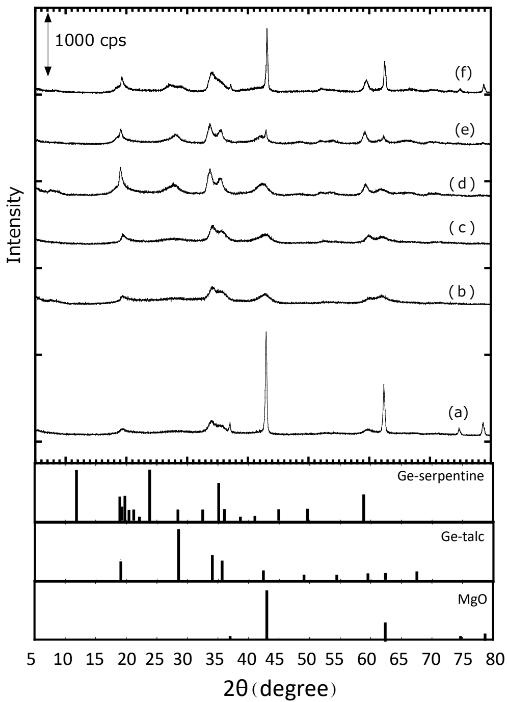
Fig. 3.4 水熱合成前の懸濁液の pH が Ge-タルク形成に及ぼす影響 水熱合成前の懸濁液の pH (a) 7.0, (b) 7.3, (c) 9.5, (d) 10.0, (e) 10.5, (f) 11.3
