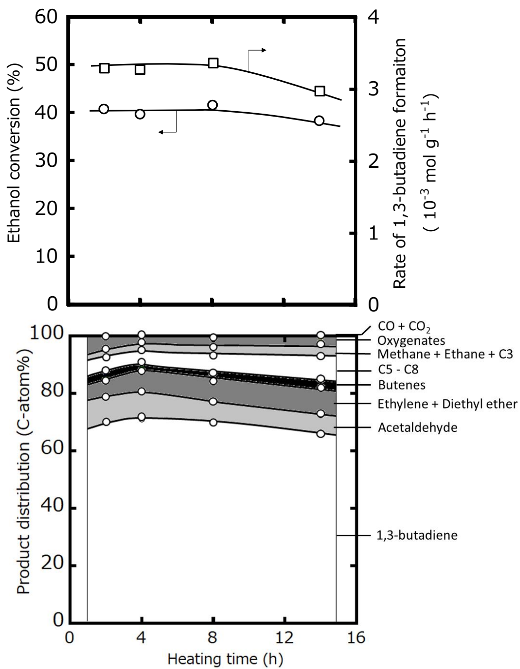
Fig. 3.7 加熱時間が1,3-ブタジエンの生成速度と生成物分布に及ぼす影響
