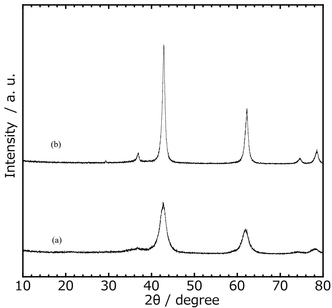
Fig. 2.2 加熱して水熱合成した \text{MgO}_{\text{ht}} と加熱した \text{MgO}_{\text{calc}} の XRD パターン
