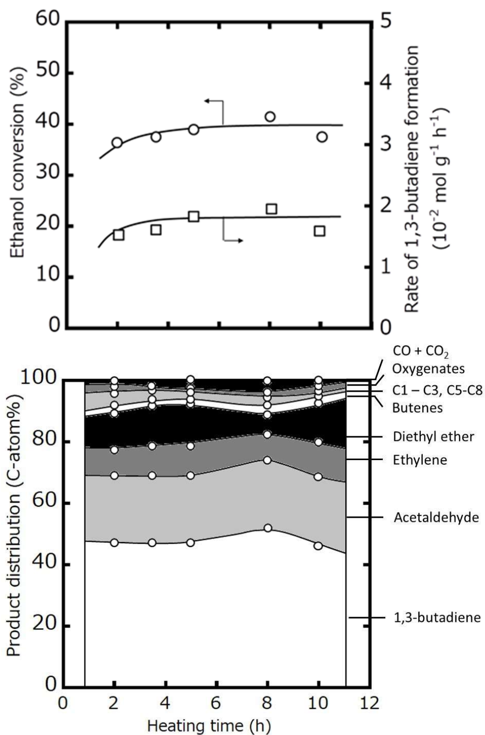
Fig. 2.12 Zn/タルクを触媒としたエタノール転化反応における
