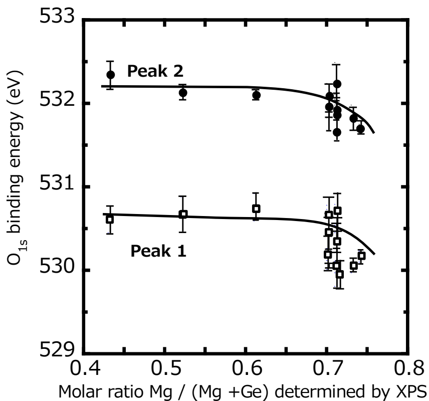
Fig. 3.15 Ge-タルクにおける表面原子比 \text{Mg} / (\text{Mg} + \text{Ge}) が \text{O}_{1s} 軌道の電子の結合エネルギーに及ぼす影響
