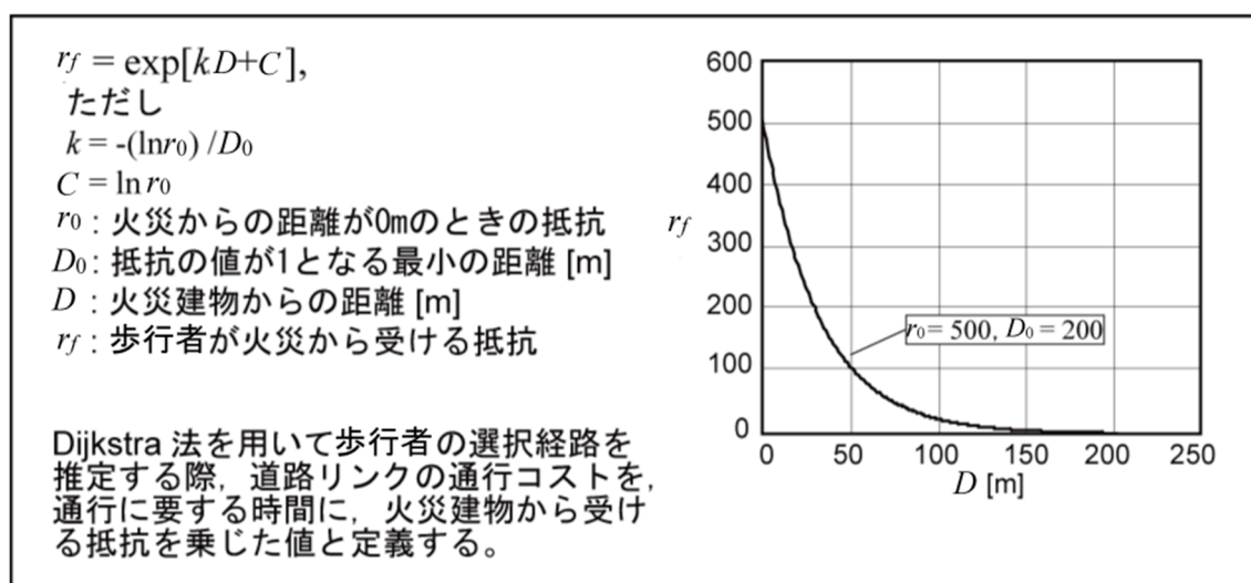
図 2.6.4 火災建物から受ける抵抗のモデル化 13 [30]
