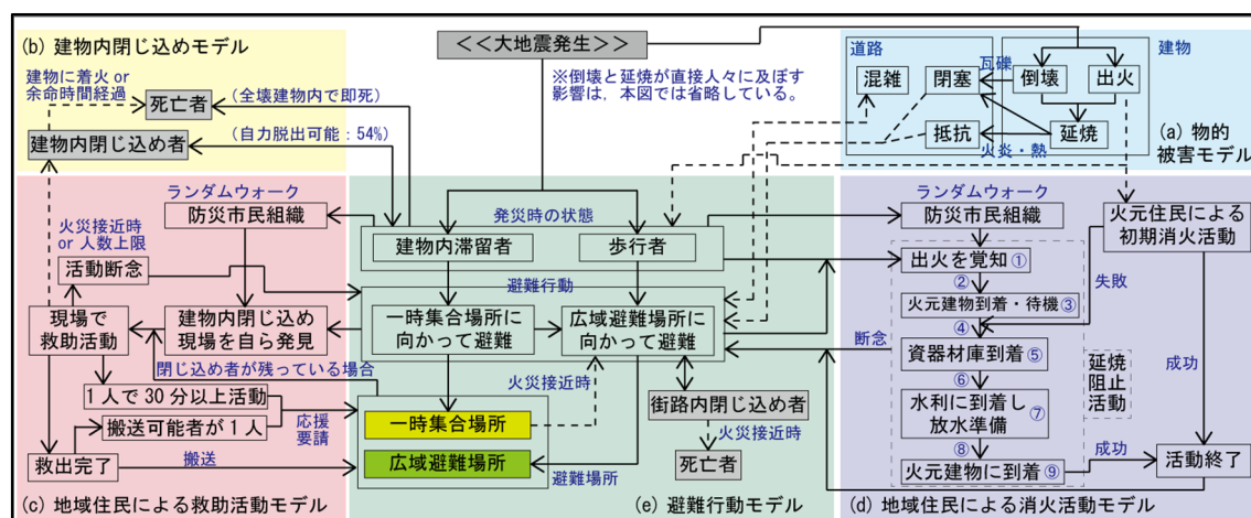
図 2.1.1 大地震時の物的被害・人間行動シミュレーションモデルの全体像 1,2[1]
