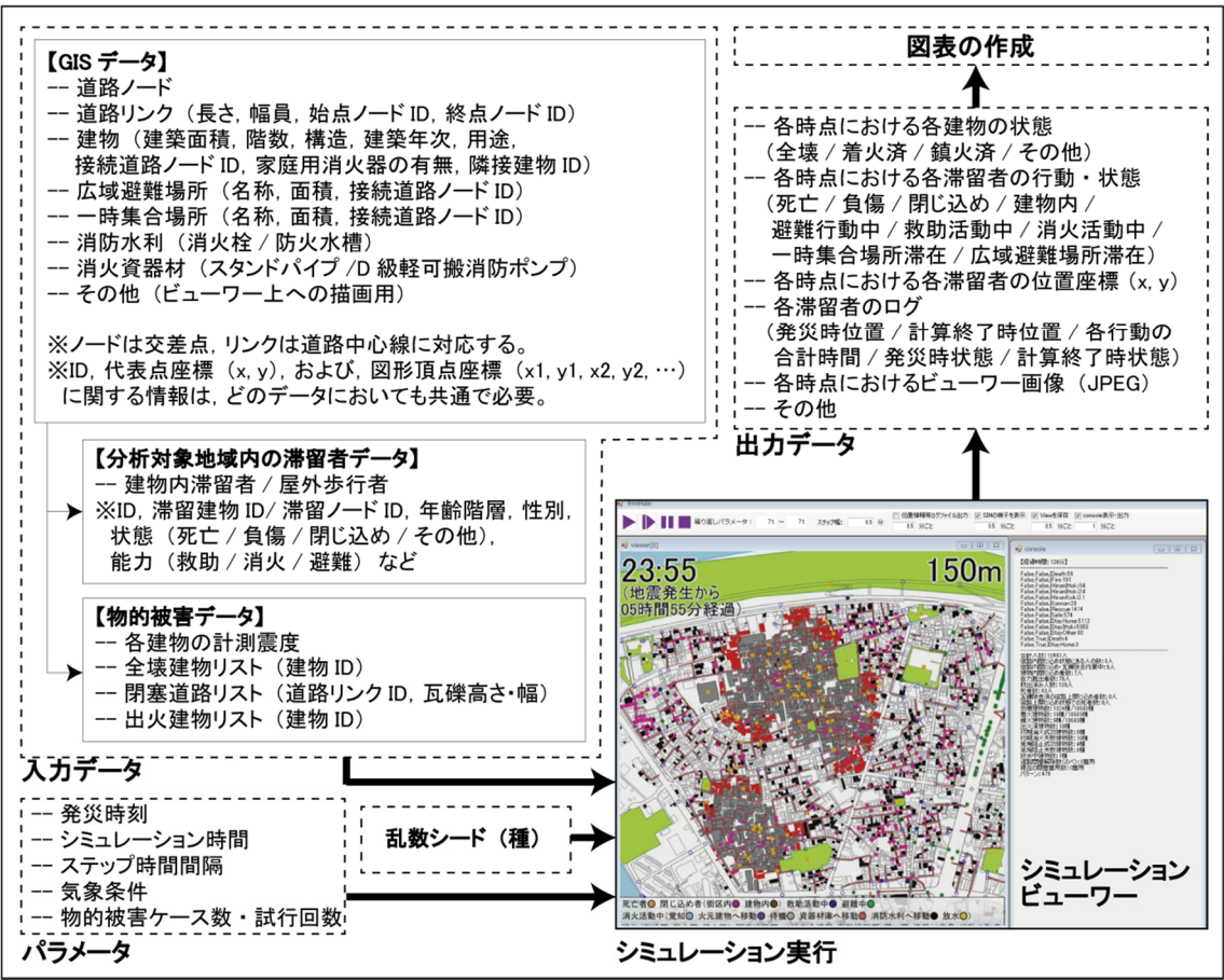
図 2.8.1 本論文のシミュレーション分析における処理プロセス[29]
