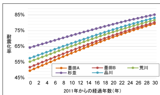
図 6.6.3 耐震化率の経年変化 ※物的被害100ケースのシミュレーションに基づく推定値
