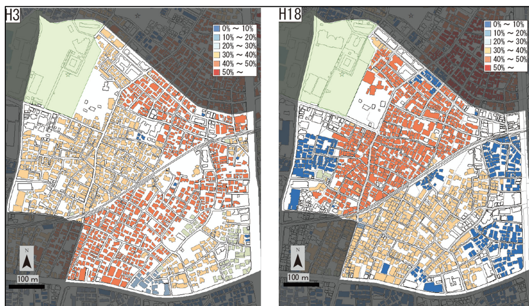
図 6.2.5 各建物の焼損率（100 回のうち各建物が焼損した回数の割合[推定値]）
