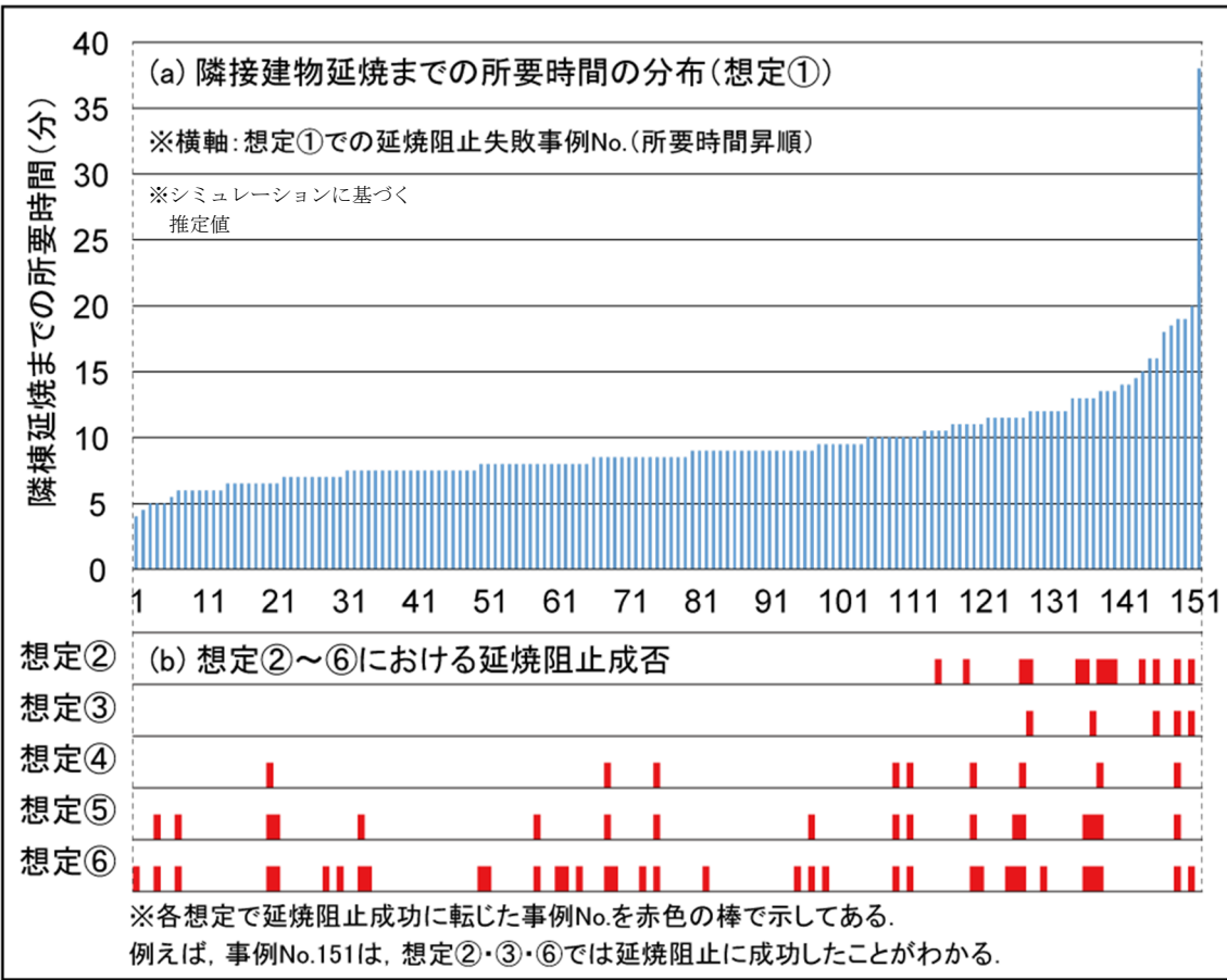
図 5.4.1 隣接建物延焼までの所要時間の分布と想定②～⑥における延焼阻止成否
