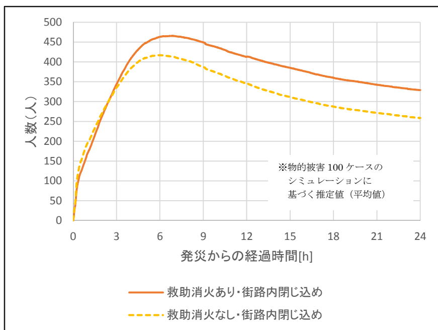
図 3.7.1 街路内閉じ込め者数の時間推移
