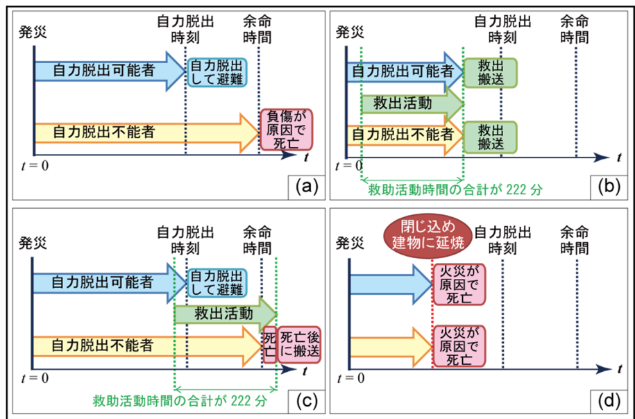
図 2.3.2 建物内閉じ込め者の脱出・救出・死亡
