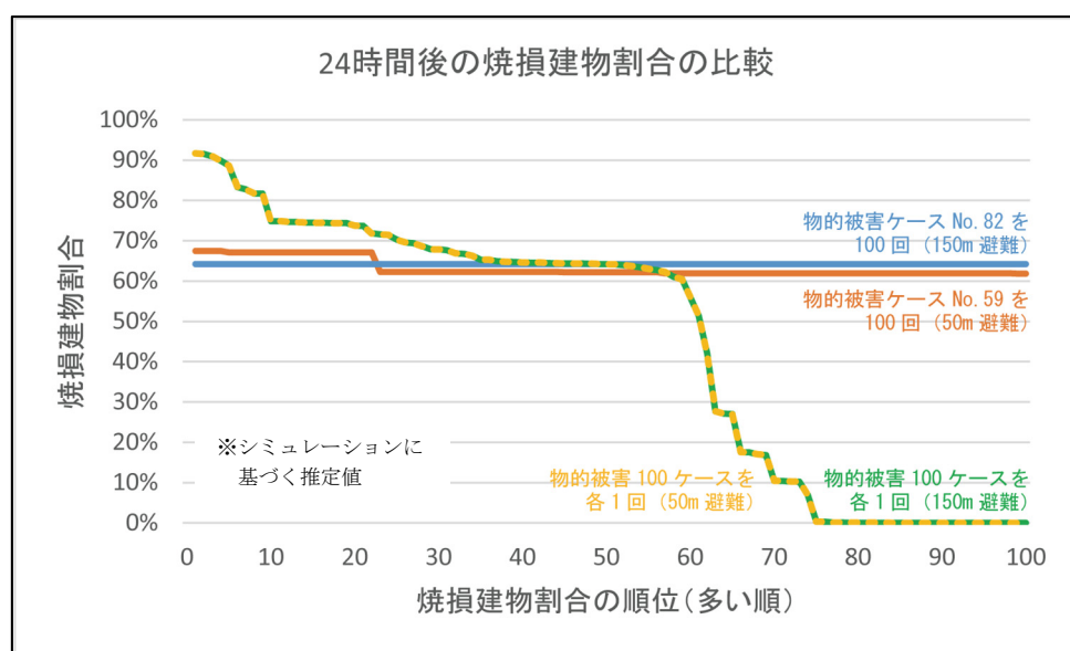
図 8.1.5 発災から 24 時間経過後の焼損建物割合の比較
