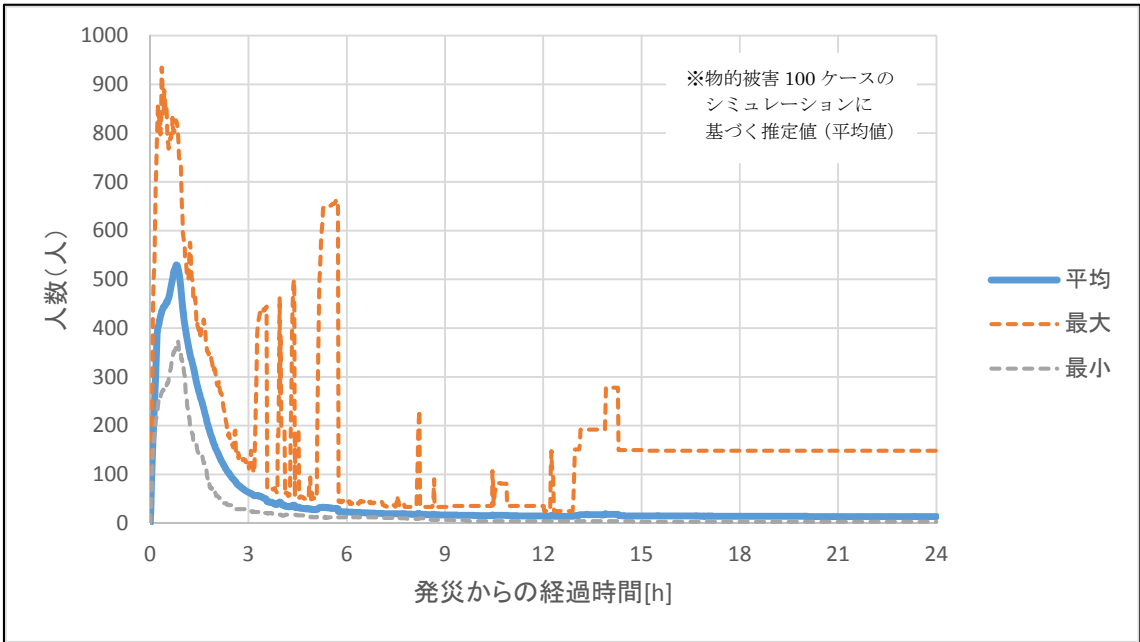
図 3.4.1 救助活動者数の時間推移
