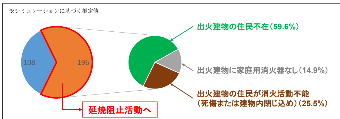
図 5.2.2 火元初期消火の成否
