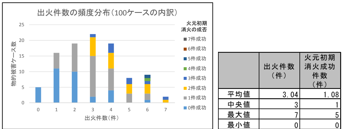
図 3.3.1 火元初期消火成功件数（物的被害 100 ケースの結果に基づく推定値）
