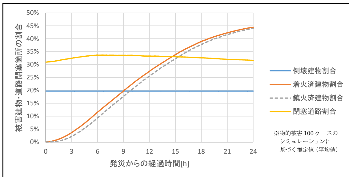
図3.2.1 物的被害箇所数の時間推移
