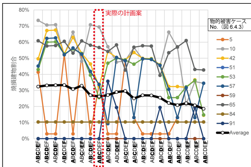
図 6.5.1 整備シナリオ別の焼損建物割合
