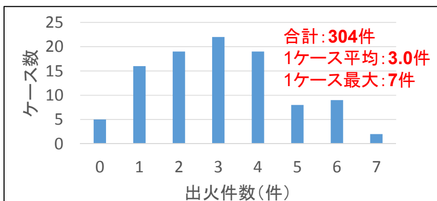
図 5.2.1 出火件数の頻度分布（物的被害 100 ケースの内訳）
