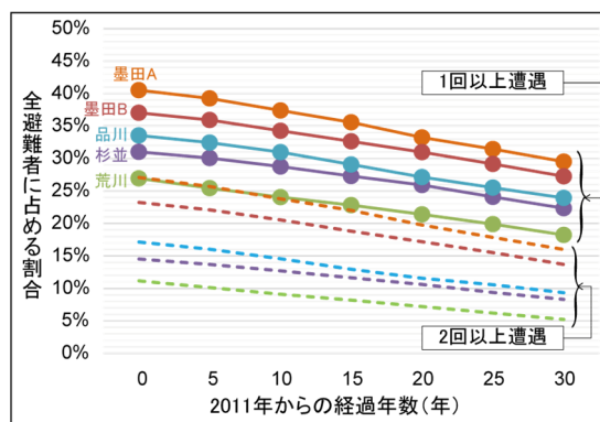
図 6.6.9 閉塞道路遭遇回数 ※物的被害 100 ケースのシミュレーションに基づく推定値
