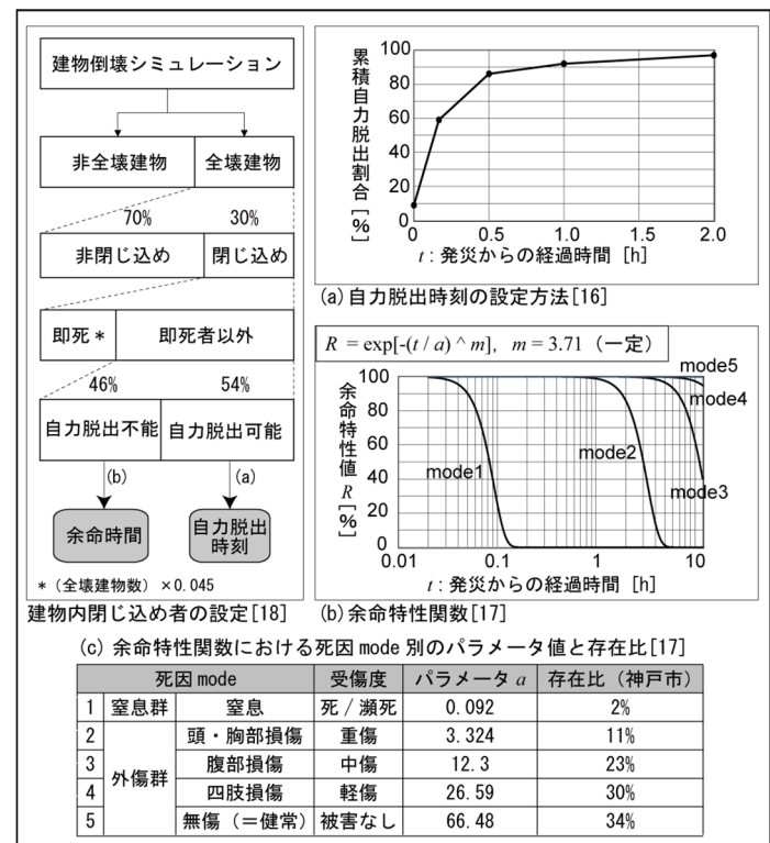
図 2.3.1 建物内閉じ込め者の設定方法[18]および自力脱出時刻と余命時間の設定方法[16, 17]
