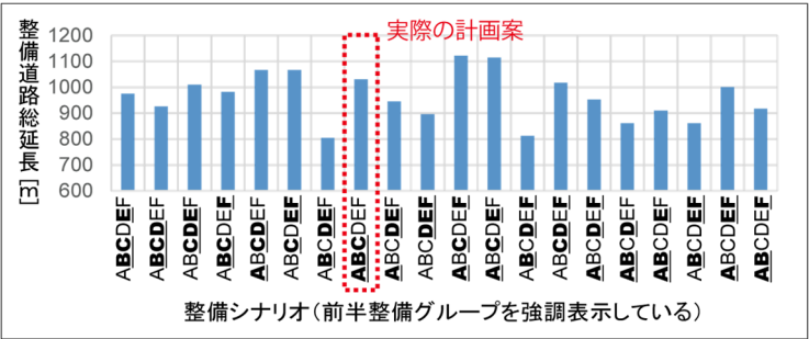
図 6.5.3 前半整備グループの整備道路総延長（整備シナリオ別）
