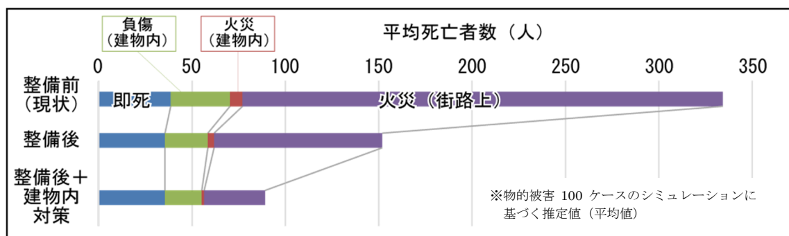
図 6.4.5 平均死亡者数の比較 (死因別・想定別)
