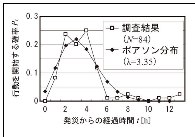
図 2.6.2 行動開始のタイミングの設定に用いる Poisson 分布[30]
