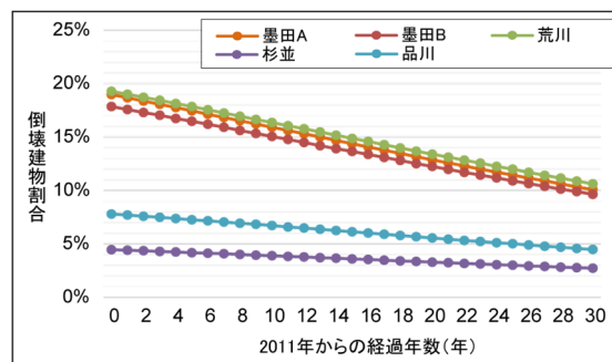
図 6.6.4 倒壊建物割合の経年変化 ※物的被害100ケースのシミュレーションに基づく推定値
