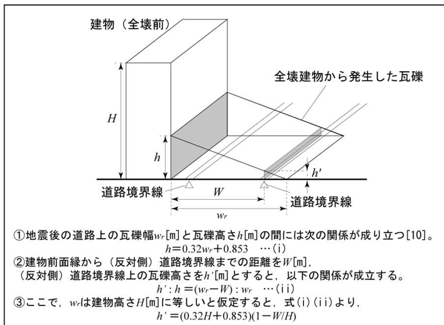
図 2.2.3 全壊建物から発生する瓦礫高さのモデル化
